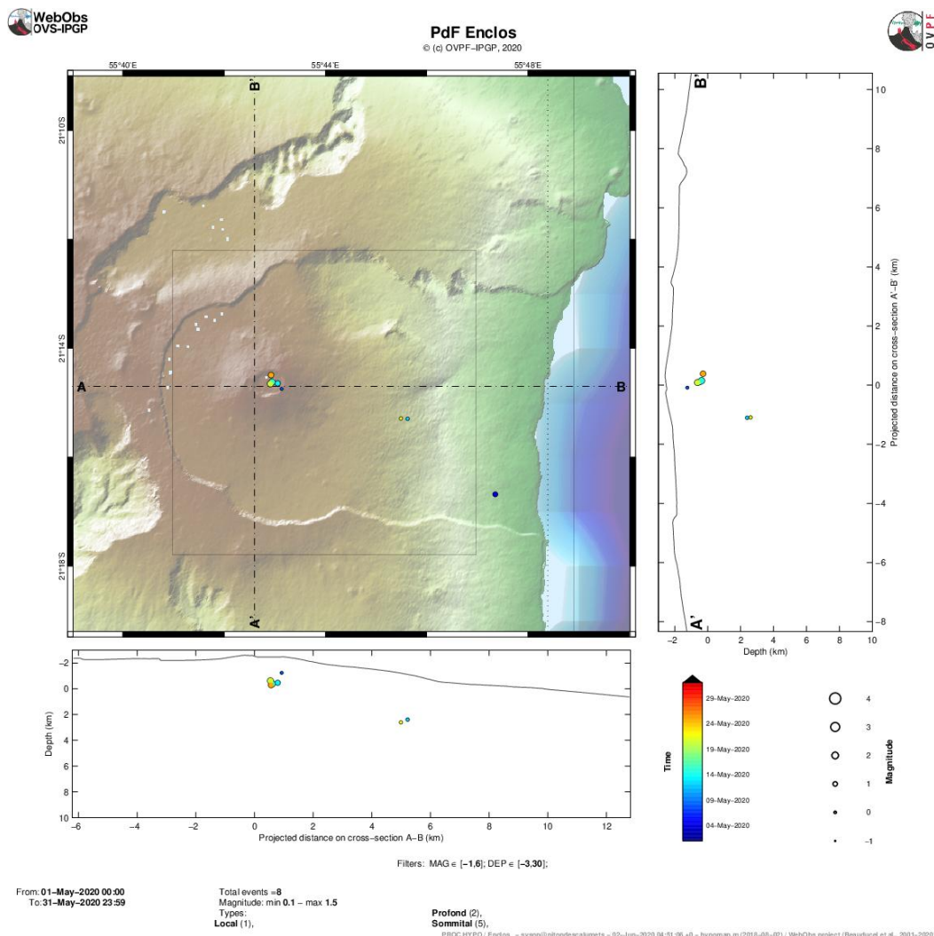
Figure 2 : Carte de localisation (épcentres) et coupes nord-sud et est-ouest (montrant la localisation en profondeur, hypocentres) des séismes enregistrés et localisés par l'OVPF-IPGP au mois de mai 2020 sous le massif du Piton de la Fournaise. Seuls les séismes localisables ont été représentés sur la carte. L'observatoire enregistre des événements sismiques non représentés sur cette carte car non localisables, en raison de leur trop faible magnitude (© OVPF-IPGP).
