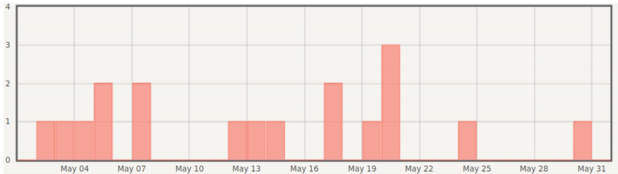
Figure 1 : Histogramme représentant le nombre de séismes volcano-tectoniques superficiels enregistrés en mai 2020 (© OVPF-IPGP).
