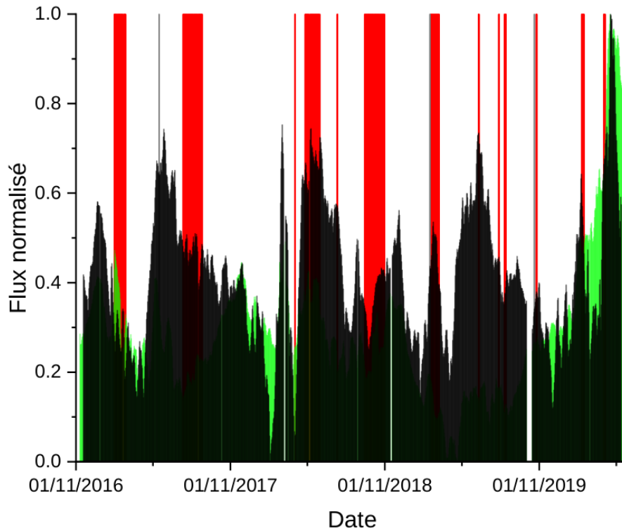
Figure 6 : Comparaison entre les moyennes normalisées des données de flux de CO 2 dans le sol, brutes (moyennées sur une fenêtre glissante de 15 jours, en vert) et corrigées (en noir), enregistrées sur les stations localisées en champ lointain depuis octobre 2016 (date d’installation de la dernière station). Les périodes éruptives sont représentées en rouge et les périodes intrusives en gris (© OVPF-IPGP).
