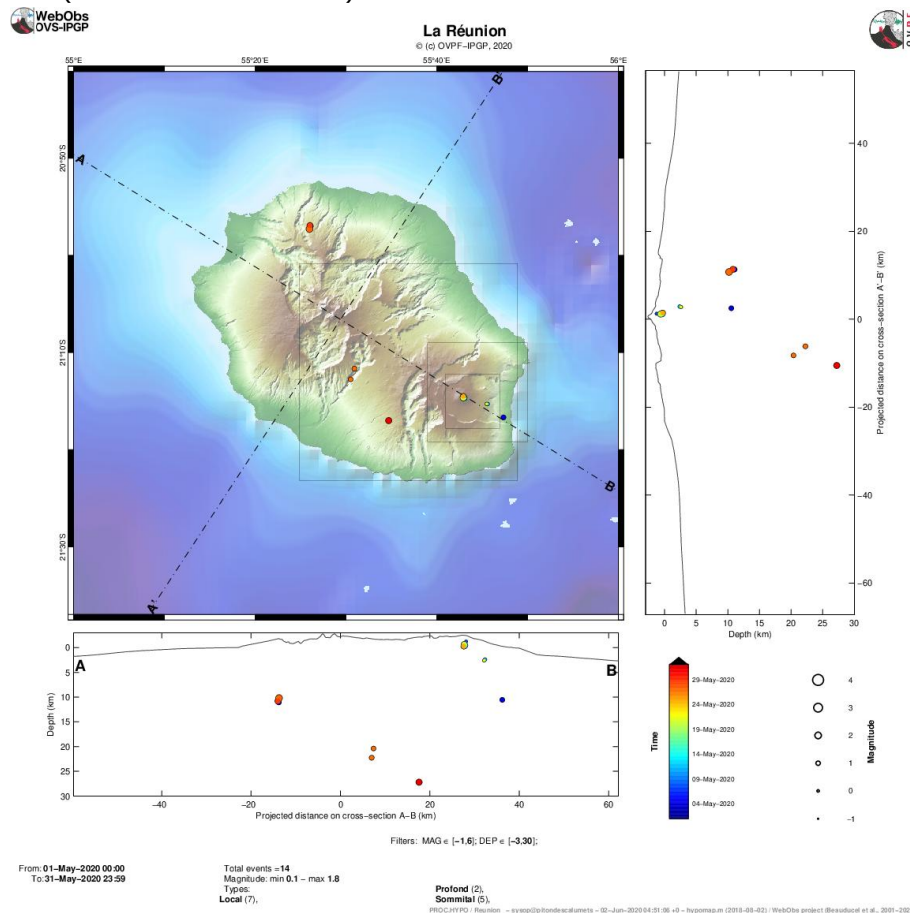
Figure 8 : Carte de localisation (épencentres) et coupes nord-sud et est-ouest (montrant la localisation en profondeur, hypocentres) des séismes enregistrés et localisés par l'OVPF-IPGP au mois de mai 2020 sous l'île de La Réunion. Seuls les séismes localisables ont été représentés sur la carte. L'observatoire enregistre des événements sismiques non représentés sur cette carte car non localisables, en raison de leur trop faible magnitude (@OVPF-IPGP).
