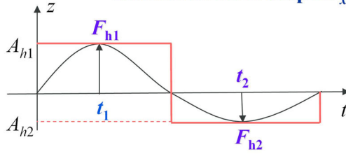
(d) Horizontal force drop \Delta F_x
