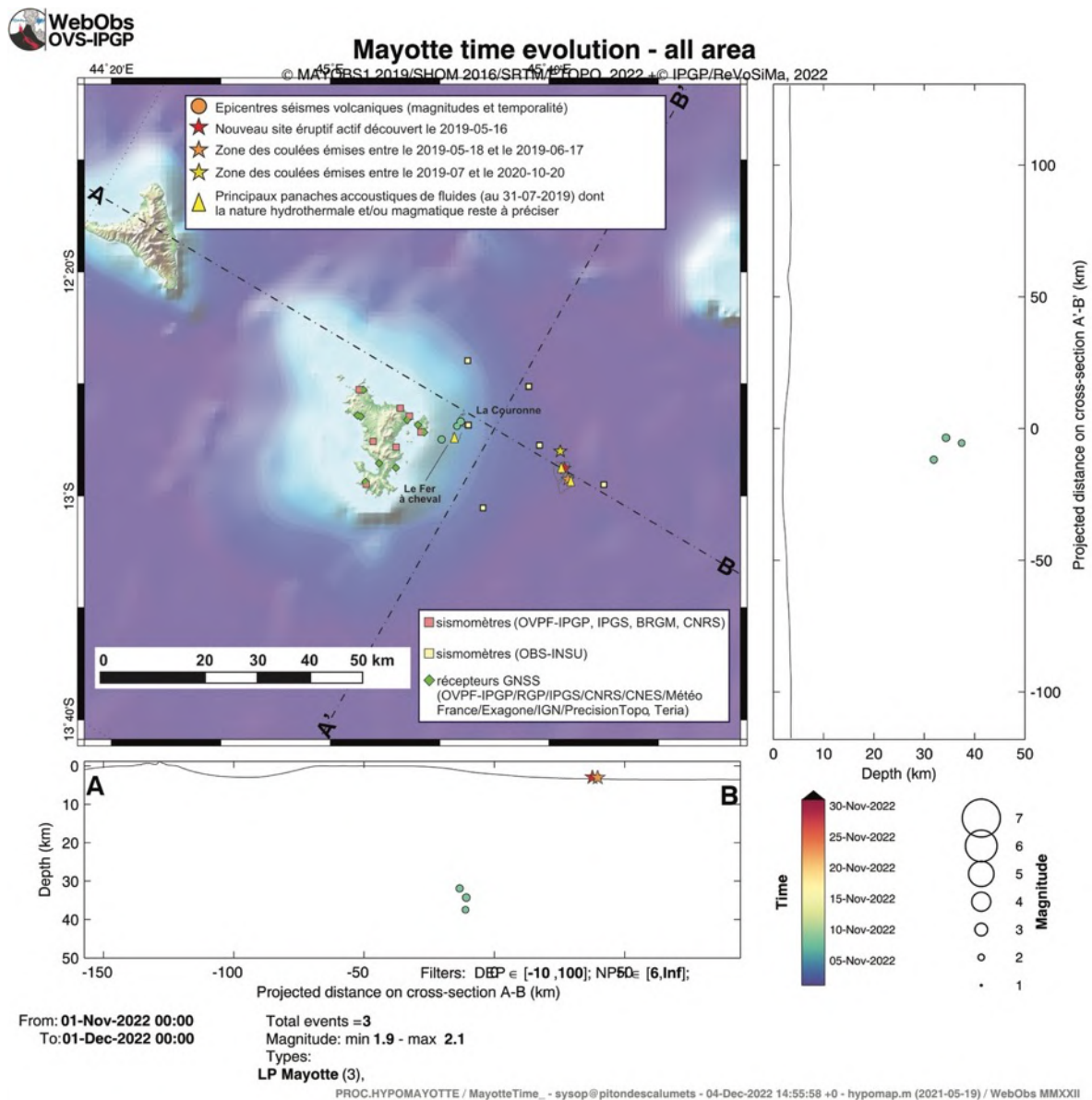
Figure 1b : Carte des épicentres ( \pm 5 km) des séismes longue période (LP) localisés avec les réseaux sismiques à terre (IPGP -CNRS-BRGM-BCSF-RENAISS, ITES) entre le 1 er et 30 novembre 2022 (échelle temporelle de couleur). Sont aussi représentées une projection des hypocentres des séismes le long de coupes transverses et axiales le long de la ride montrant la localisation estimée en profondeur (la précision varie entre \pm 5 km et \pm 15 km) des séismes en fonction de la magnitude (taille des symboles et de la date (échelle temporelle de couleur)). La localisation approximative des panaches acoustiques identifiés pendant les campagnes océanographiques (MD220-MAYOBS1, MD221-MAYOBS2, MD222-MAYOBS3, MD223-MAYOBS4, MAYOBS15, MAYOBS17) et dont la nature hydrothermale et/ou magmatique reste à préciser, est indiquée par des triangles jaunes, l'étoile rouge indique le site éruptif nouvellement identifié le 16 mai 2019, l'étoile orange la zone des coulées émises entre le 18/05/2019 et le 17/06/2019 et l'étoile jaune la zone des coulées émises entre juillet 2019 et le 18/01/2021. Les structures volcaniques de la zone dite de « La Couronne », du « Fer à cheval » sont indiquées en grisé tout comme les coulées de lave de Fani Maoré. Les stations sismiques du réseau terrestre, les sismomètres fond de mer (OBS) et les stations de positionnement par satellite GPS sont indiquées par des symboles (voir légende). (©OVPF-IPGP, BRGM, IFREMER, CNRS, BCSF-RENAISS, ITES / REVOSIMA).
