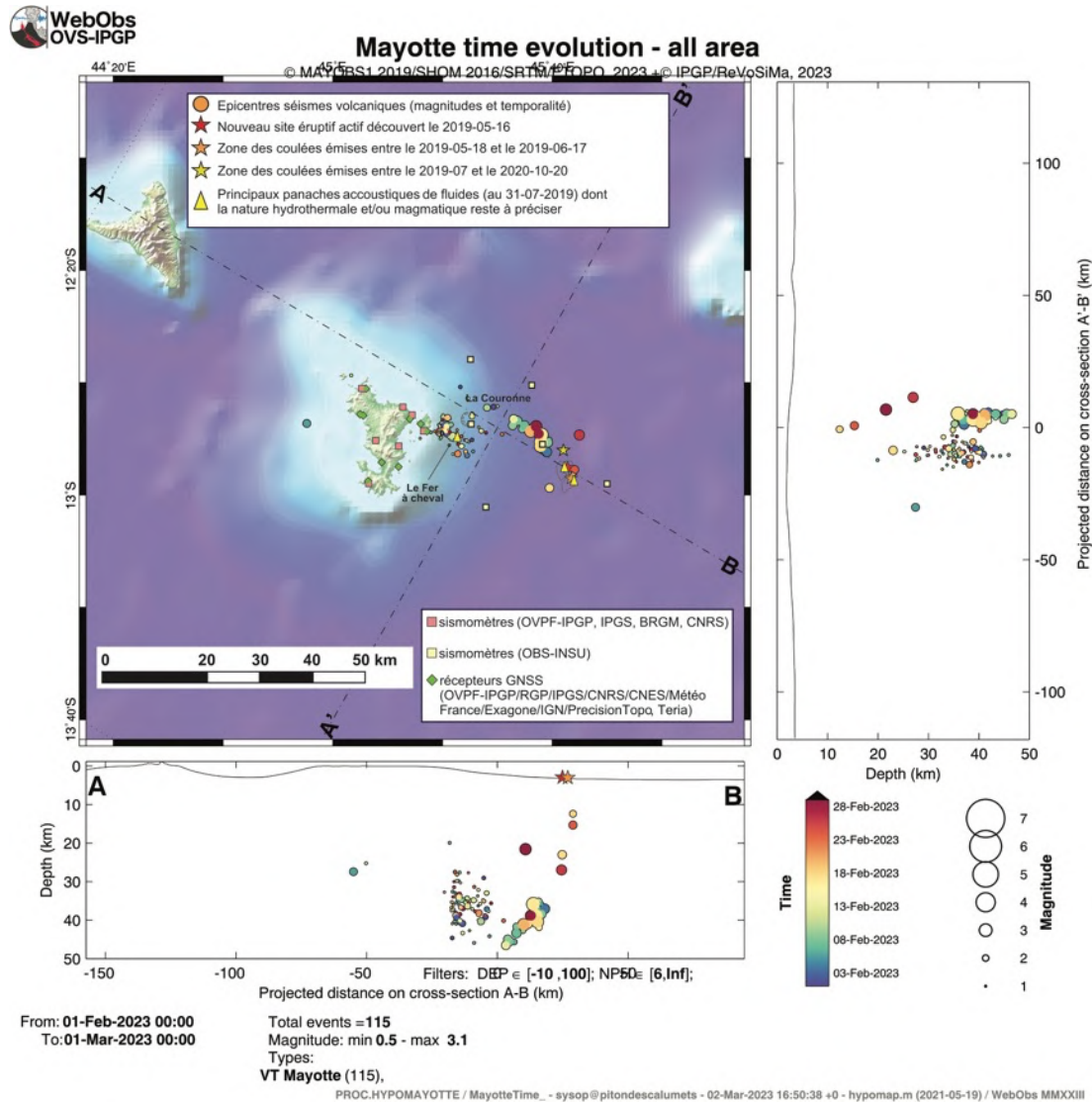
Figure 1a : Carte des épicentres ( \pm 5 km) des séismes volcano-tectoniques (VT) localisés avec les réseaux sismiques à terre (IPGP-CNRS-BRGM-BCSF-RENAISS, ITES) entre le 1 er et 28 février 2023 (échelle temporelle de couleur). Sont aussi représentées une projection des hypocentres des séismes le long de coupes transverses et axiales le long de la ride montrant la localisation estimée en profondeur (la précision varie entre \pm 5 km et \pm 15 km) des séismes en fonction de la magnitude (taille des symboles et de la date (échelle temporelle de couleur)). La localisation approximative des panaches acoustiques identifiés pendant les campagnes océanographiques (MD220-MAYOBS1, MD221-MAYOBS2, MD222-MAYOBS3, MD223-MAYOBS4, MAYOBS15, MAYOBS17) et dont la nature hydrothermale et/ou magmatique reste à préciser, est indiquée par des triangles jaunes, l'étoile rouge indique le site éruptif nouvellement identifié le 16 mai 2019, l'étoile orange la zone des coulées émises entre le 18/05/2019 et le 17/06/2019 et l'étoile jaune la zone des coulées émises entre juillet 2019 et le 18/01/2021. Les structures volcaniques de la zone dite de « La Couronne », du « Fer à cheval » sont indiquées en grisé tout comme les coulées de lave de Fani Maoré. Les stations sismiques du réseau terrestre, les sismomètres fond de mer (OBS) et les stations de positionnement par satellite GPS sont indiquées par des symboles (voir légende). (©OVPF-IPGP, BRGM, IFREMER, CNRS, BCSF-RENAISS, ITES / REVOSIMA).
