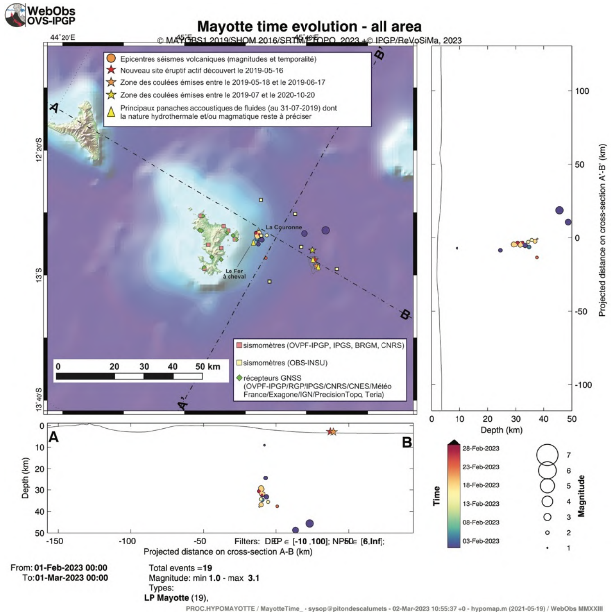
Figure 1b : Carte des épicentres ( \pm 5 km) des séismes longue période (LP) localisés avec les réseaux sismiques à terre (IPGP -CNRS-BRGM-BCSF-RENASS, ITES) entre le 1 er et 28 février 2023 (échelle temporelle de couleur). Sont aussi représentées une projection des hypocentres des séismes le long de coupes transverses et axiales le long de la ride montrant la localisation estimée en profondeur (la précision varie entre \pm 5 km et \pm 15 km) des séismes en fonction de la magnitude (taille des symboles et de la date (échelle temporelle de couleur)). La localisation approximative des panaches acoustiques identifiés pendant les campagnes océanographiques (MD220-MAYOBS1, MD221-MAYOBS2, MD222-MAYOBS3, MD223-MAYOBS4, MAYOBS15, MAYOBS17) et dont la nature hydrothermale et/ou magmatique reste à préciser, est indiquée par des triangles jaunes, l'étoile rouge indique le site éruptif nouvellement identifié le 16 mai 2019, l'étoile orange la zone des coulées émises entre le 18/05/2019 et le 17/06/2019 et l'étoile jaune la zone des coulées émises entre juillet 2019 et le 18/01/2021. Les structures volcaniques de la zone dite de « La Couronne », du « Fer à cheval » sont indiquées en grisé tout comme les coulées de lave de Fani Maoré. Les stations sismiques du réseau terrestre, les sismomètres fond de mer (OBS) et les stations de positionnement par satellite GPS sont indiquées par des symboles (voir légende). (©OVPF-IPGP, BRGM, IFREMER, CNRS, BCSF-RENASS, ITES / REVOSIMA).
