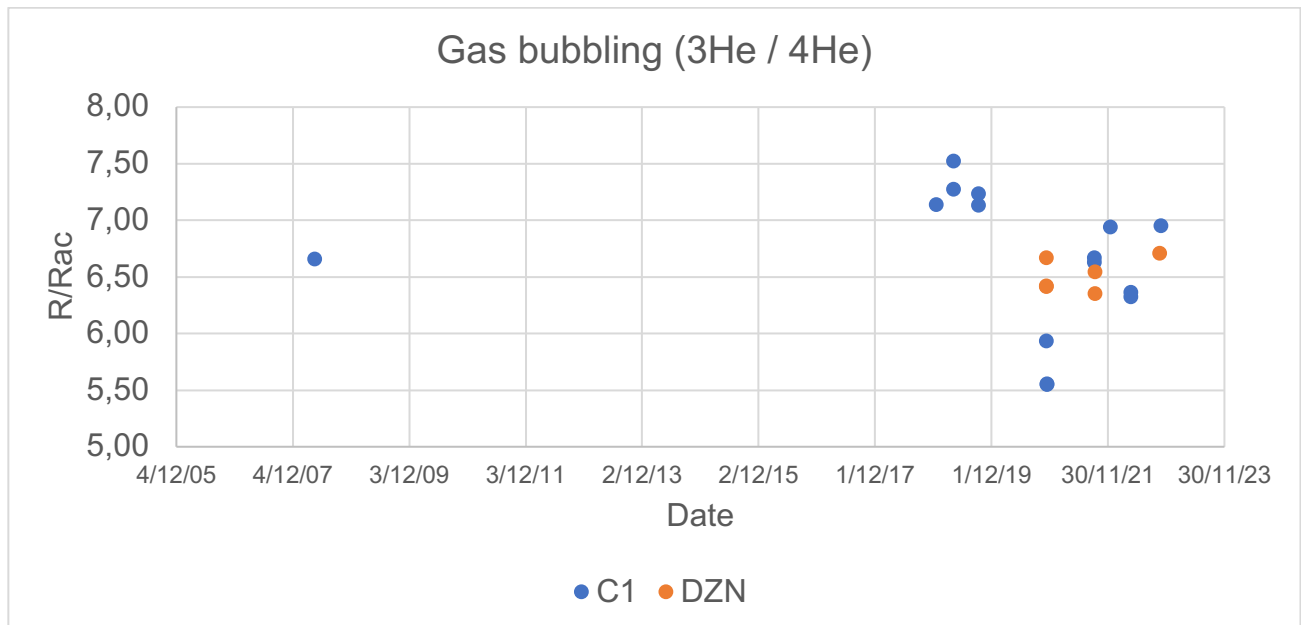
Figure 13 : Analyses isotopiques (gaz rares) des bullages aux points de contrôle C1 (estran de l'aéroport) et DZN (Lac Dziani). Une augmentation du R/R_{ac} (rapport isotopique de l'He normalisé à celui de l'atmosphère) est liée à une augmentation de la contribution des fluides profonds remontant du manteau. Erreur moyenne sur chaque analyse : 0.05 unité.
