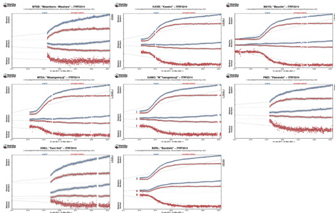
Figure 9 : Déplacements (en cm) enregistrés sur les 8 stations GPS localisés à Mayotte (MTSB, KAWE, MAYG, M TSA, GAMO, PMZI, KNKL, BDRL ; la station PORO a été retirée en 2021 et n'est donc plus affichée ici) entre le 1 er janvier 2017 et 28 février 2023 pour visualiser une longue série temporelle ante crise. En bleu les données brutes, en rouge les données corrigées du mouvement de la plaque. Les stations sont présentées dans un ordre géographique ; du nord au sud (de haut en base à et d'ouest en est (de gauche à droite). Post-traitement de ces données réalisé par l'IPGP (©OVPF-IPGP / REVOSIMA).
