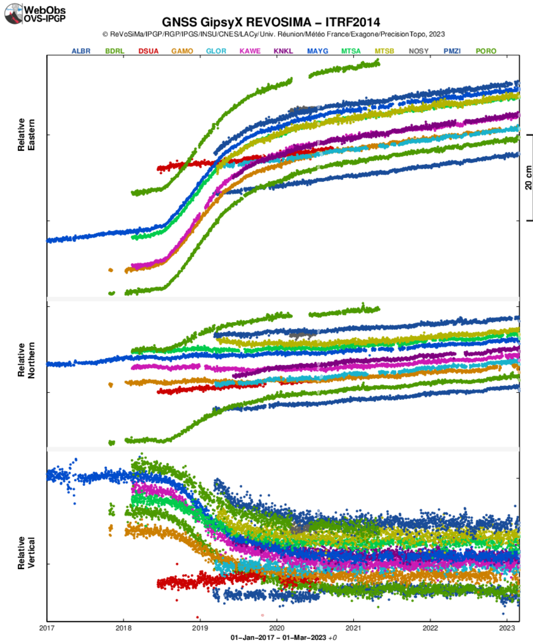
Figure 8 : Déplacements (en cm) enregistrés sur 9 stations GPS localisés à Mayotte (BDRL, GAMO, KAWE, KNKL, MAYG, MTSA, MTSB, PMZI, PORO), 1 station à Grande Glorieuse (GLOR), 1 station à Aldabra (ALBR) et 2 stations au nord de Madagascar à Diego Suarez (DSUA) et Nosy Be (NOSY) sur les composantes est (en haut), nord (au milieu) et vertical (en bas) entre le 1 er janvier 2017 et le 28 février 2023 pour visualiser une longue série temporelle ante crise. Post-traitement de ces données réalisé par l'IPGP (©OVVPF-IPGP / REVOSIMA).
