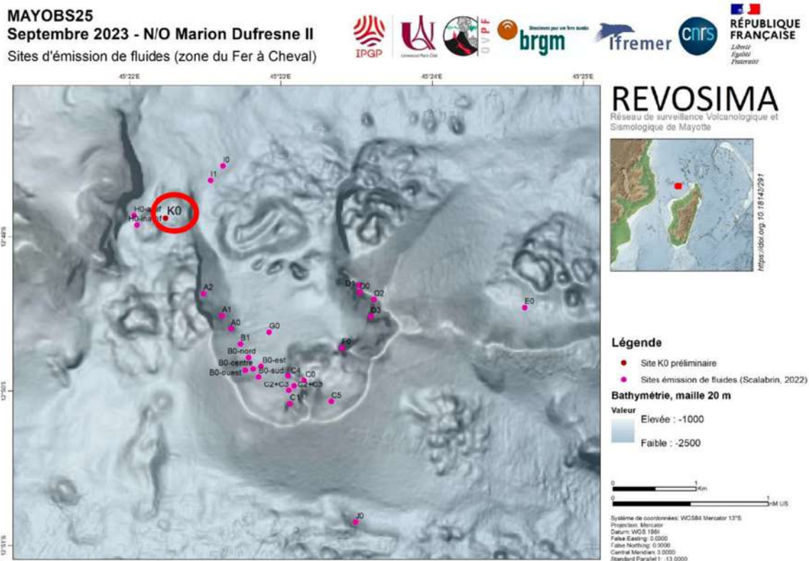
Figure 17 : Localisation des sites actifs d'émission de fluides fond de mer dans le périmètre élargi du Fer à Cheval (@Scalabrin, 2023- https://doi.org/10.12770/070818f6-6520-49e4-bafd-9d4d0609b7fd ). Le nouveau site actif K0 observé (@Scalabrin & A. Potier) pour la première fois pendant la campagne MAYOBS25 y est intégré (entouré en rouge) (©REVOSIMA).
