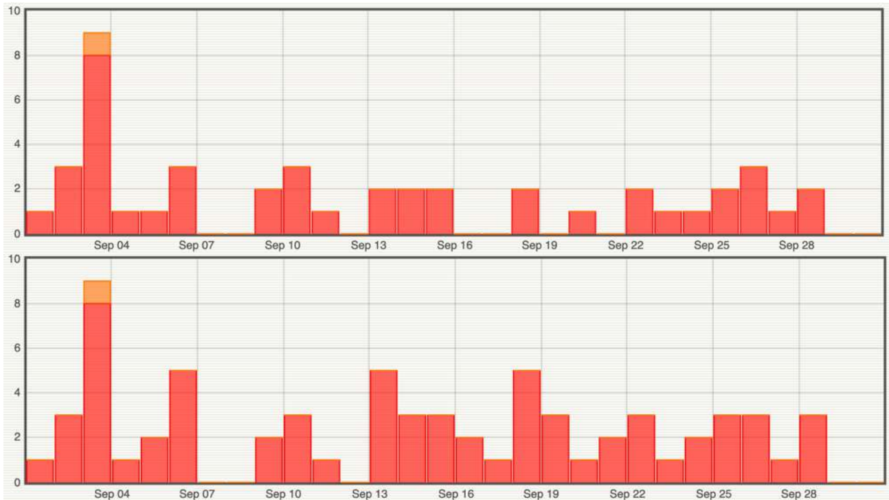
Figure 7 : Histogramme représentant le nombre de séismes par jour détectés (en haut) et localisés (en bas) en septembre 2023 par le réseau sismologique du REVOSIMA. En rouge les séismes volcano-tectoniques, en orange les séismes longues périodes, en jaune les séismes très longues périodes (© OVPF-IPGP et REVOSIMA).
