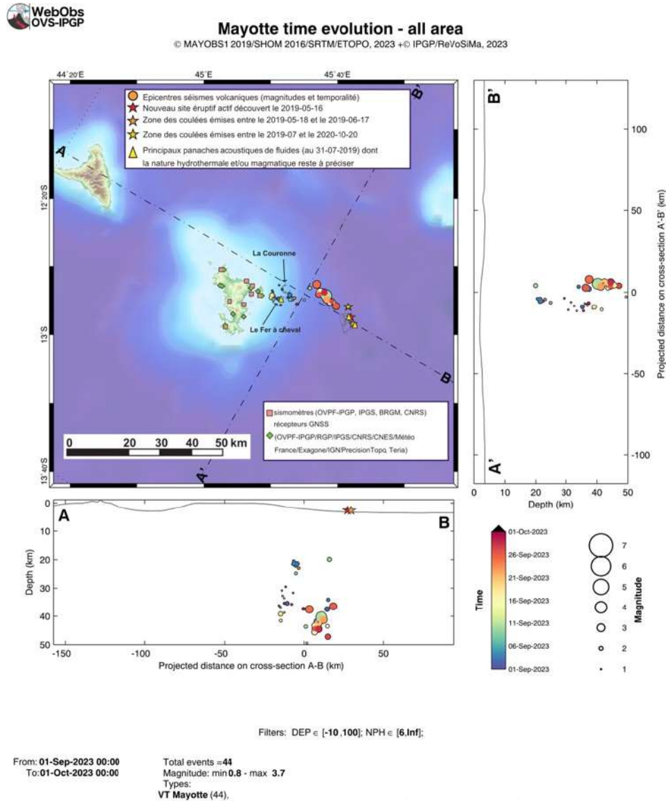
Figure 2 : Carte des épicentres ( \pm 5 km) des séismes volcano-tectoniques (VT) localisés avec les réseaux sismiques à terre (IPGP-CNRS-BRGM-BCSF-RENASS, ITES) entre le 1 er et 30 septembre 2023 (échelle temporelle de couleur). Sont aussi représentées une projection des hypocentres des séismes le long de coupes transverses et axiales le long de la ride montrant la localisation estimée en profondeur (la précision varie entre \pm 5 km et \pm 15 km) des séismes en fonction de la magnitude (taille des symboles et de la date (échelle temporelle de couleur)). La localisation approximative des panaches acoustiques identifiés pendant les campagnes océanographiques (MD220-MAYOBS1, MD221-MAYOBS2, MD222-MAYOBS3, MD223-MAYOBS4, MAYOBS15, MAYOBS17 ; Rinnert et al., 2019) et dont la nature hydrothermale et/ou magmatique reste à préciser, est indiquée par des triangles jaunes, l'étoile rouge indique le site éruptif nouvellement identifié le 16 mai 2019, l'étoile orange la zone des coulées émises entre le 18/05/2019 et le 17/06/2019 et l'étoile jaune la zone des coulées émises entre juillet 2019 et le 18/01/2021. Les structures volcaniques de la zone dite de « La Couronne », du « Fer à cheval » sont indiquées en grisé tout comme les coulées de lave de Fani Maoré. Les stations sismiques du réseau terrestre et les stations de positionnement par satellite GPS sont indiquées par des symboles (voir légende). (©OVVPF-IPGP, BRGM, IFREMER, CNRS, BCSF-RENASS, ITES / REVOSIMA).
