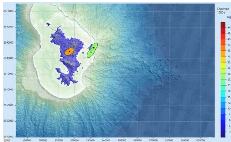
Figure 18 : Carte de tenseurs de phases calculés à 1000 secondes des 3 stations MT du Revosima pour le mois d'août 2023 (©BRGM et REVOSIMA).
