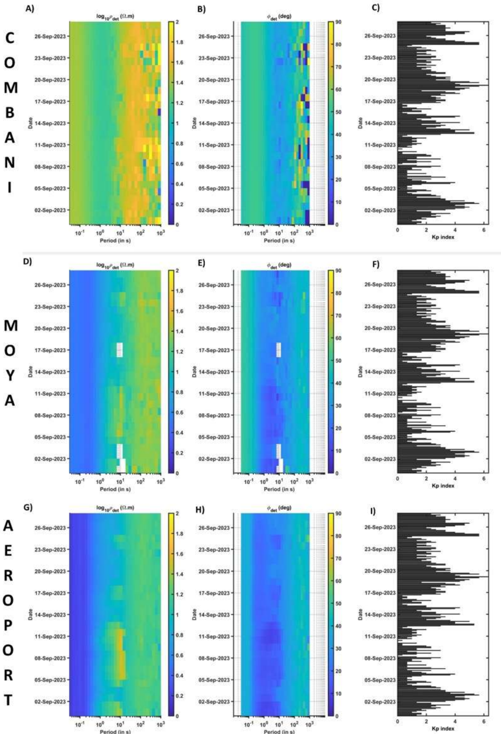
Figure 21 : Période du 01/09/2023 au 28/09/2023 - Chroniques temps-période de résistivité apparente de l'invariant 1D MT en échelle logarithmique (a, d, g), de phases (b, e, h) et index géomagnétiques Kp (c, f, i) du réseau MT Revosima (©BRGM et REVOSIMA) pour le site de Combani (haut), Moya (centre) et Aéroport (bas).
