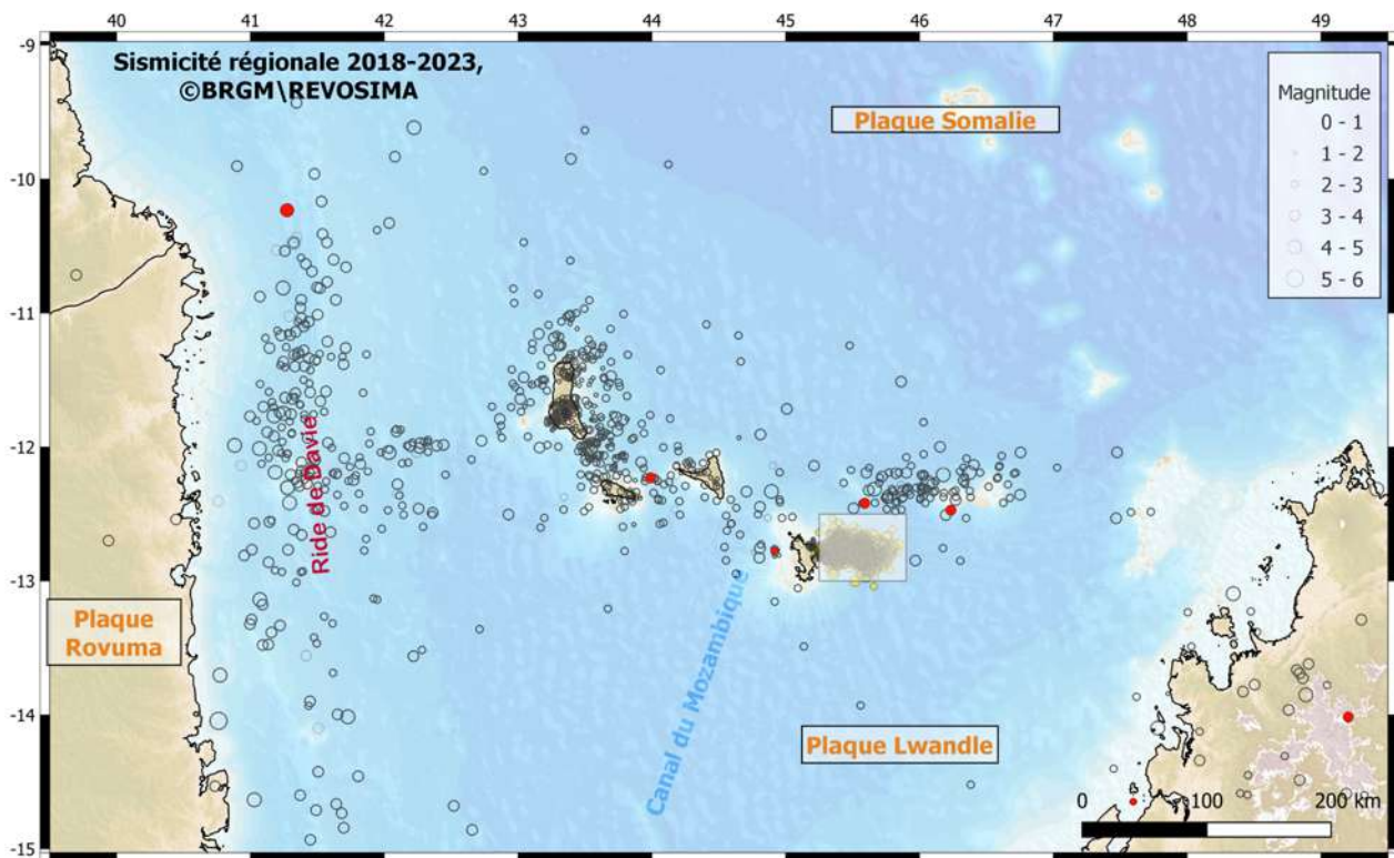
Figure 1: Sismicité régionale enregistrée depuis 2018 (modifié d'après Bertil et al., 2021). Les séismes de septembre 2023 sont représentés en rouge. Le fond de carte est construit à partir des données topographiques et bathymétriques de Gebco 2022 ( www.gebco.net ). Le trait de côte et les frontières administratives sont extraits de https://gadm.org/ . Le carré blanc encadre les essaims sismiques surveillés depuis 2018. Se référer aux Figures 2 et 3 de ce bulletin pour la distribution de cette sismicité.
