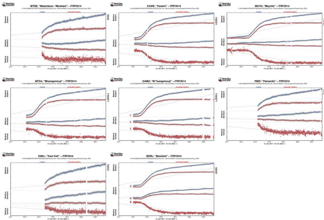
Figure 10 : Déplacements (en cm) enregistrés sur les 8 stations GPS localisés à Mayotte (MTSB, KAWE, MAYG, MTSA, GAMO, PMZI, KNKL, BDRL ; la station PORO a été retirée en 2021 et n'est donc plus affichée ici) entre le 1 er janvier 2017 et le 30 septembre 2023 pour visualiser une longue série temporelle ante crise. En bleu les données brutes, en rouge les données corrigées du mouvement de la plaque. Les stations sont présentées dans un ordre géographique ; du nord au sud (de haut en bas) et d'ouest en est (de gauche à droite). Post-traitement de ces données réalisé par l'IPGP (©OVPF-IPGP / REVOSIMA).
