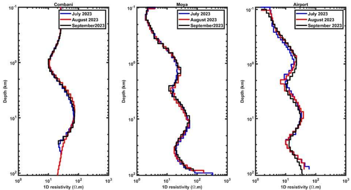
Figure 19 : Modèles 1D de Résistivité du sous-sol de 100 m à 100 km de profondeur sous Combani (gauche), Moya (centre) et Aéroport (droite) pour les mois de juillet (bleu), août 2023 (rouge) et septembre 2023 (noir).
