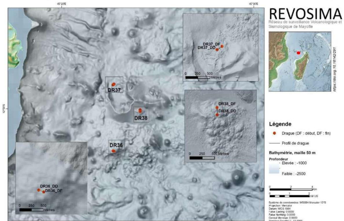
Figure 22 : Localisation des trois dragues obtenues lors de la campagne MD242-MAYOSB25 (© REVOSIMA).
