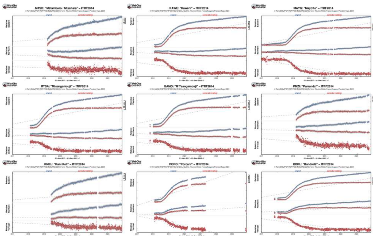
Figure 10 : Déplacements (en cm) enregistrés sur les 9 stations GPS localisés à Mayotte (MTSB, KAWE, MAYG, MTSA, GAMO, PMZI, KNKL, PORO, BDRL ; la station PORO a été remise en service le 10 novembre 2023) entre le 1 er janvier 2017 et le 30 novembre 2023 pour visualiser une longue série temporelle ante crise. En bleu les données brutes, en rouge les données corrigées du mouvement de la plaque. Les stations sont présentées dans un ordre géographique ; du nord au sud (de haut en bas) et d'ouest en est (de gauche à droite). Post-traitement de ces données réalisé par l'IPGP (©OVVPF-IPGP / REVOSIMA).
