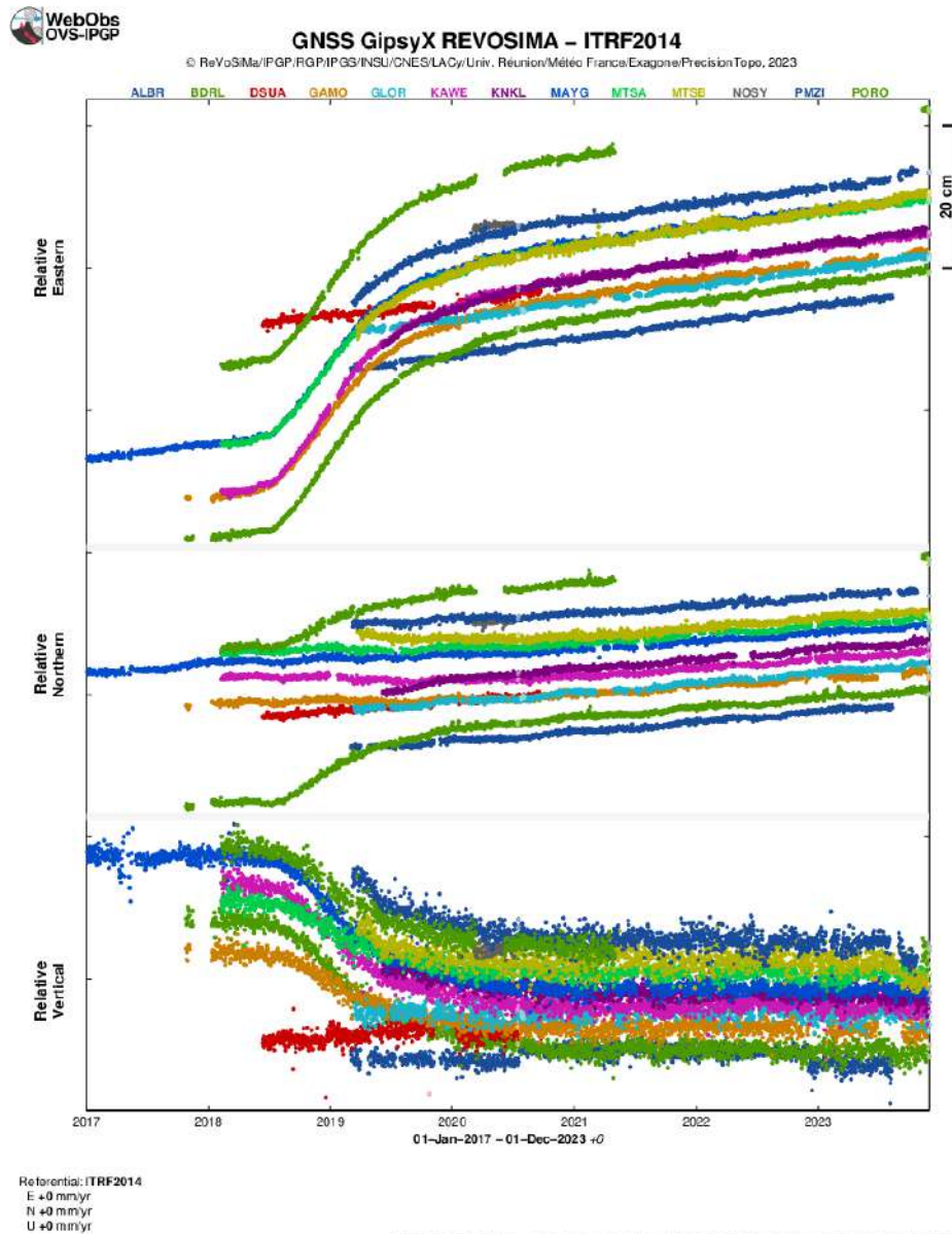
Figure 9 : Déplacements (en cm) enregistrés sur 9 stations GPS localisés à Mayotte (BDRL, GAMO, KAWE, KNKL, MAYG, MTSB, MTSB, PMZI, PORO), 1 station à Grande Glorieuse (GLOR), 1 station à Aldabra (ALBR) et 2 stations au nord de Madagascar à Diego Suarez (DSUA) et Nosy Be (NOSY) sur les composantes est (en haut), nord (au milieu) et vertical (en bas) entre le 1 er janvier 2017 et le 30 novembre 2023 pour visualiser une longue série temporelle ante crise. Post-traitement de ces données réalisé par l'IPGP (©OVPF-IPGP / REVOSIMA).
