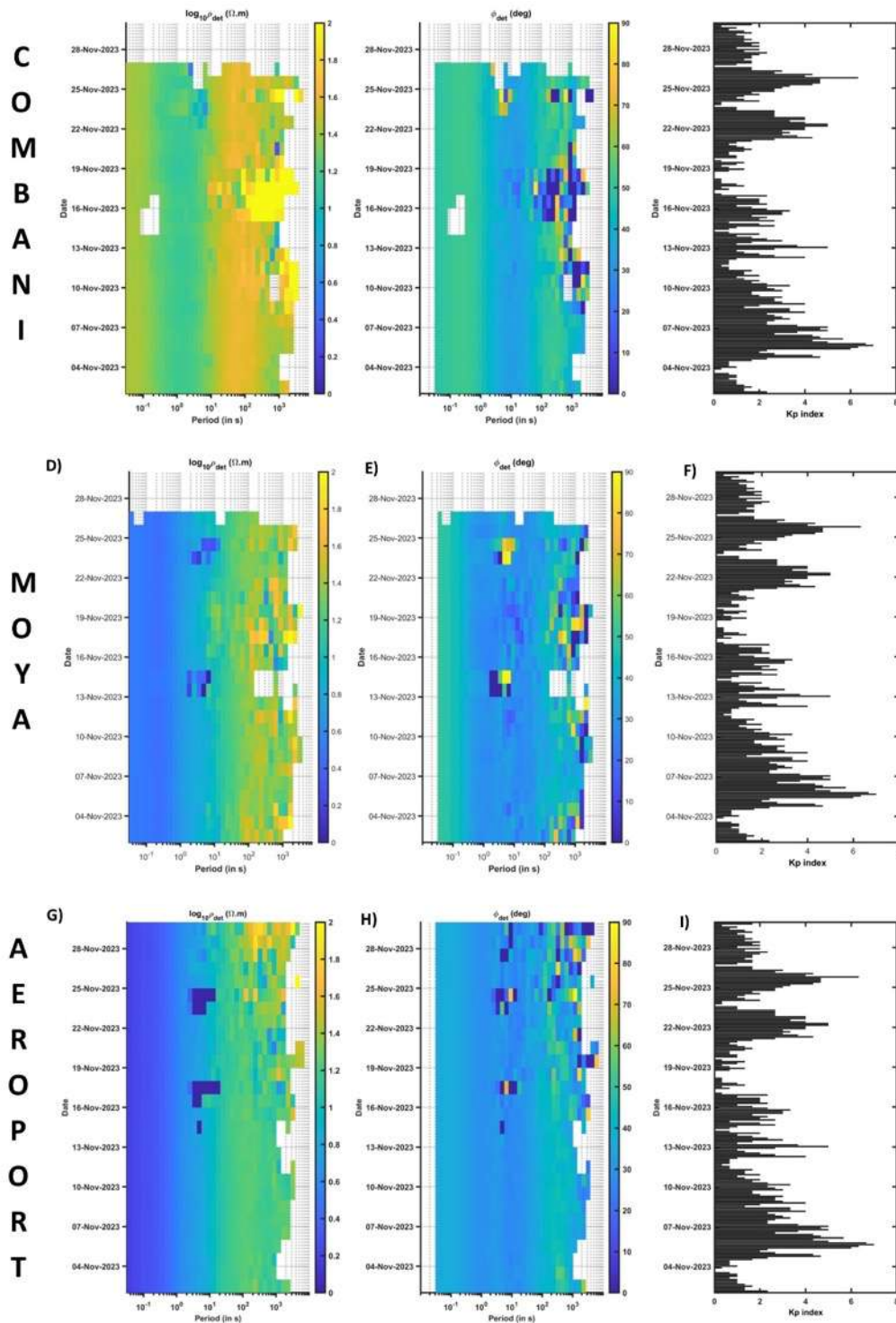
Figure 21 : Période du 01/11/2023 au 30/11/2023 - Chroniques temps-période de résistivité apparente de l'invariant 1D MT en échelle logarithmique (a, d, g), de phases (b, e, h) et index géomagnétiques Kp (c, f, i) du réseau MT Revosima (©BRGM et REVOSIMA) pour le site de Combani (haut), Moya (centre) et Aéroport (bas).
