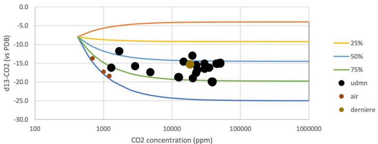
Figure 13 : Variations isotopiques du carbone ( \delta^{13}\text{C} -CO 2 ) du CO 2 dans l'air et dans les gaz du sol à la station UDMN. La composition du pôle magmatique est fixée à -4.0 per mil (signature des bullages du site C1 – estran de l'aéroport).
