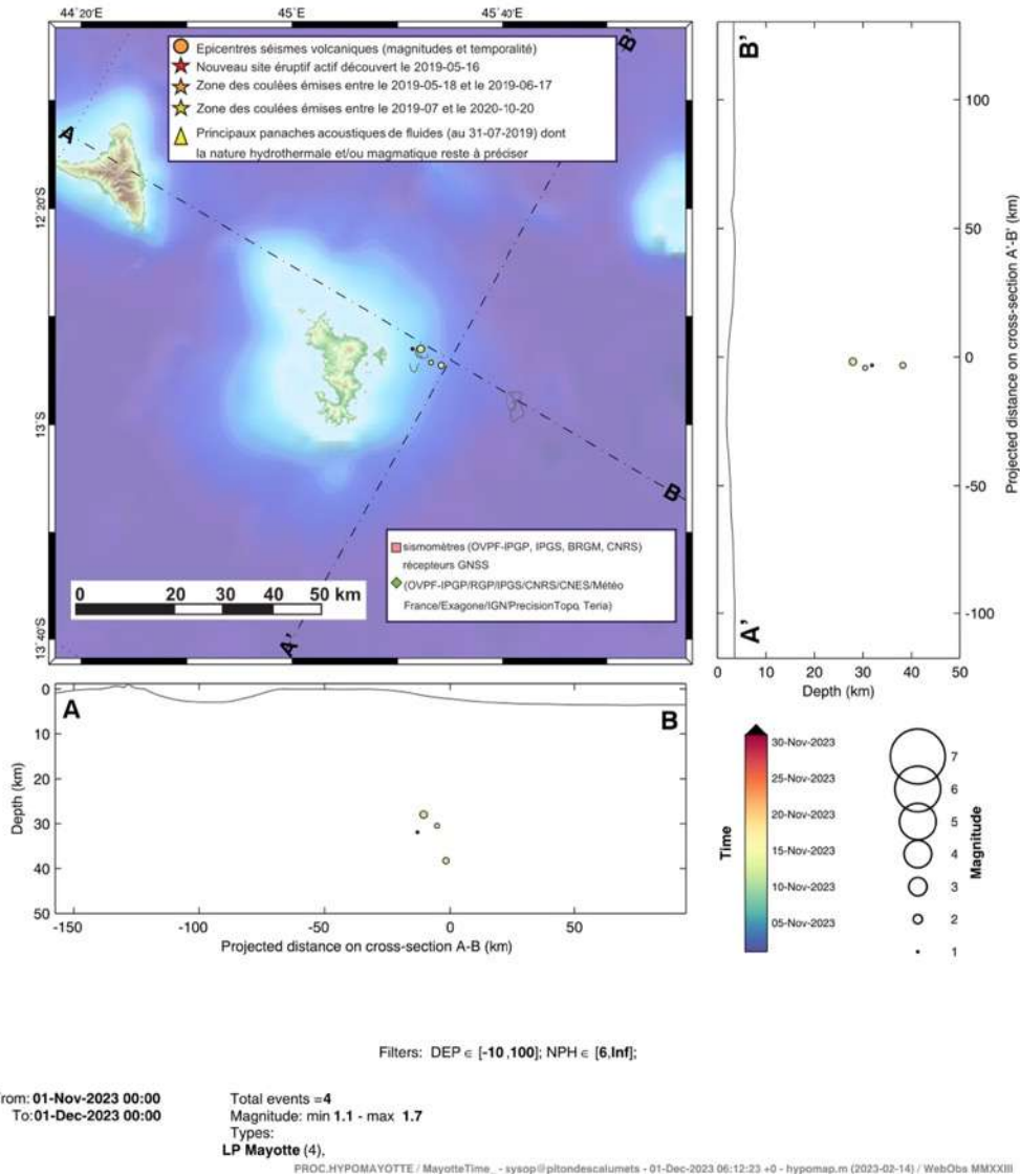
Figure 3 : Carte des épicentres ( \pm 5 km) des séismes longue période (LP) localisés avec les réseaux sismiques à terre (IPGP -CNRS-BRGM-BCSF-RENASS, ITES) entre le 1 er et 30 novembre 2023 (échelle temporelle de couleur). Sont aussi représentées une projection des hypocentres des séismes le long de coupes transversales et axiales le long de la ride montrant la localisation estimée en profondeur (la précision varie entre \pm 5 km et \pm 15 km) des séismes en fonction de la magnitude (taille des symboles) et de la date (échelle temporelle de couleur). La localisation approximative des panaches acoustiques identifiés pendant les campagnes océanographiques (MD220-MAYOBS1, MD221-MAYOBS2, MD222-MAYOBS3, MD223-MAYOBS4, MAYOBS15, MAYOBS17 ; Rinnert et al., 2019) et dont la nature hydrothermale et/ou magmatique reste à préciser, est indiquée par des triangles jaunes, l'étoile rouge indique le site éruptif nouvellement identifié le 16 mai 2019, l'étoile orange la zone des coulées émises entre le 18/05/2019 et le 17/06/2019 et l'étoile jaune la zone des coulées émises entre juillet 2019 et le 18/01/2021. Les structures volcaniques de la zone dite de « La Couronne », du « Fer à Cheval » sont indiquées en grisé tout comme les coulées de lave de Fani Maoré. Les stations sismiques du réseau terrestre) et les stations de positionnement par satellite GPS sont indiquées par des symboles (voir légende). (©OVPF-IPGP, BRGM, IFREMER, CNRS, BCSF-RENASS, ITES / REVOSIMA).
