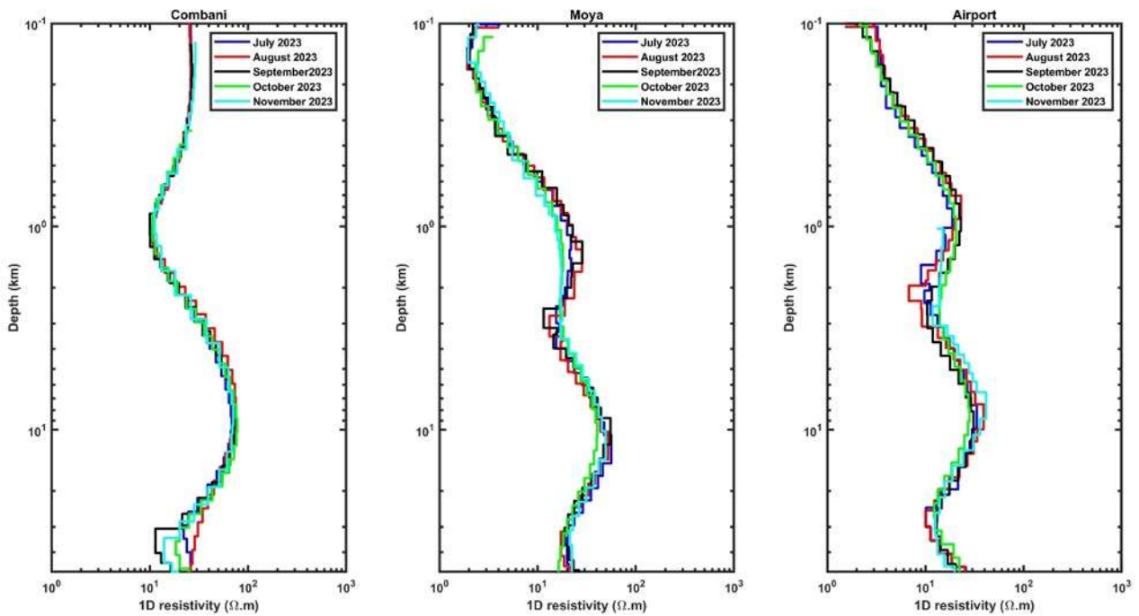
Figure 19 : Modèles 1D de résistivité du sous-sol de 100m à 100km de profondeur sous Combani (gauche), Moya (centre) et Aéroport (droite) pour les mois de juillet (bleu), août 2023 (rouge), septembre 2023 (noir), octobre 2023 (vert) et novembre 2023 (cyan).
