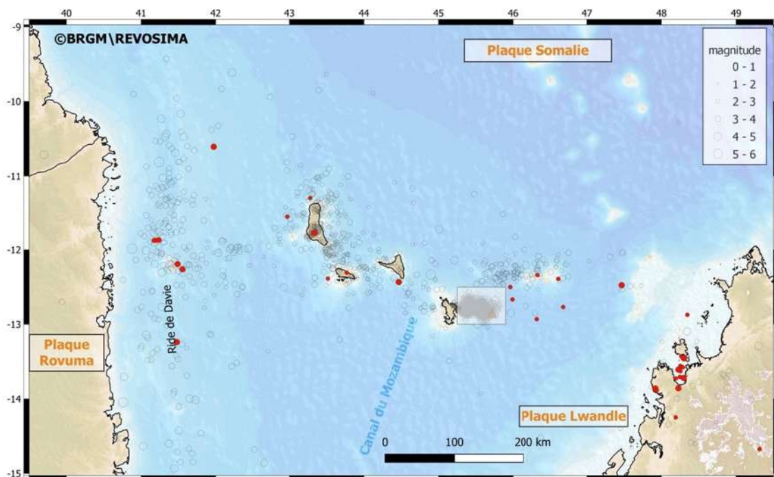
Figure 1: Sismicité régionale enregistrée depuis 2018 (modifié d'après Bertil et al. , 2021). Les séismes de novembre 2023 sont représentés en rouge. Le fond de carte est construit à partir des données topographiques et bathymétriques de Gebco 2022 ( www.gebco.net ). Le trait de côte et les frontières administratives sont extraits de https://gadm.org/ . Le carré blanc encadre les essaims sismiques surveillés depuis 2018. Se référer aux Figures 2 et 3 de ce bulletin pour la distribution de cette sismicité.
