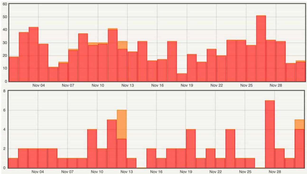
Figure 7 : Histogramme représentant le nombre de séismes par jour détectés (en haut) et localisés (en bas) en novembre 2023 par le réseau sismologique du REVOSIMA. En rouge les séismes volcano-tectoniques, en orange les séismes longues périodes, en jaune les séismes très longues périodes (© OVPF-IPGP et REVOSIMA).
