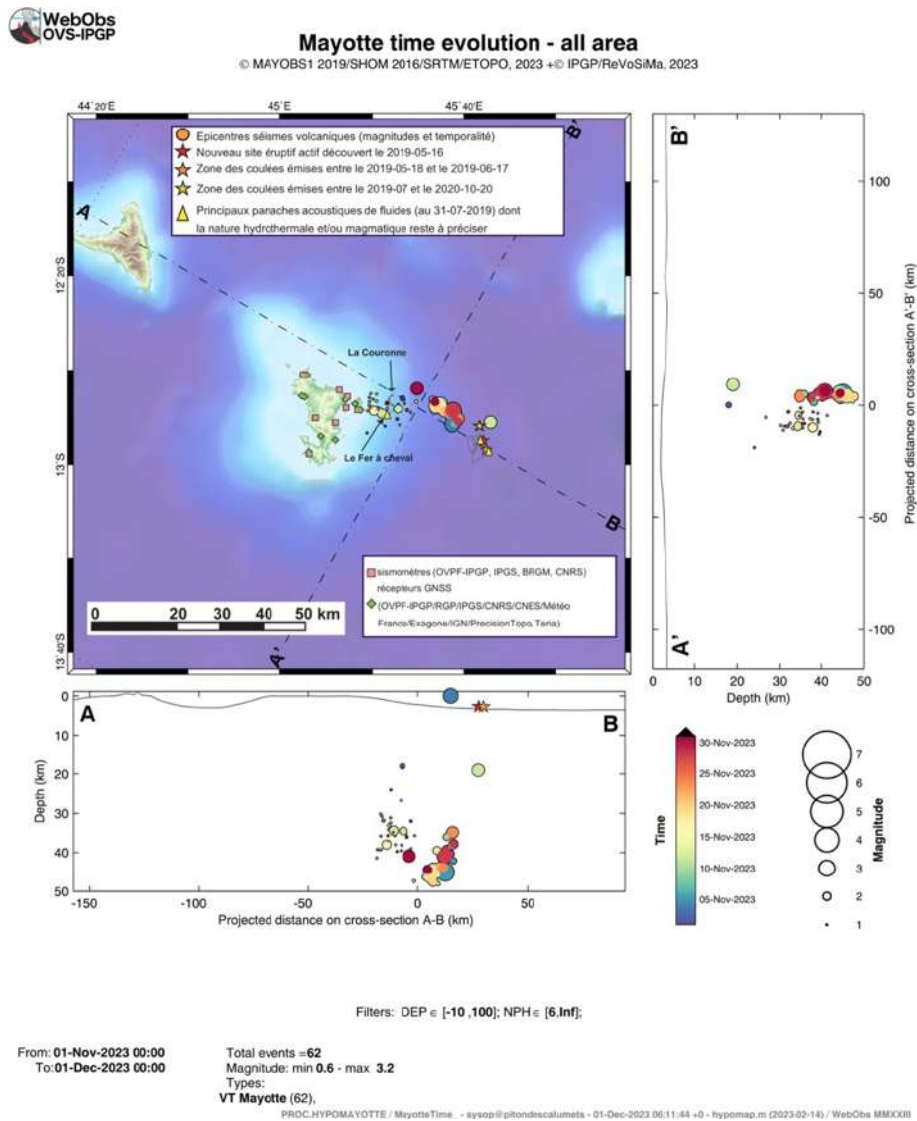
Figure 2 : Carte des épicentres ( \pm 5 km) des séismes volcano-tectoniques (VT) localisés avec les réseaux sismiques à terre (IPGP-CNRS-BRGM-BCSF-RENASS, ITES) entre le 1 er et 30 novembre 2023 (échelle temporelle de couleur). Sont aussi représentées une projection des hypocentres des séismes le long de coupes transverses et axiales le long de la ride montrant la localisation estimée en profondeur (la précision varie entre \pm 5 km et \pm 15 km) des séismes en fonction de la magnitude (taille des symboles et de la date (échelle temporelle de couleur)). La localisation approximative des panaches acoustiques identifiés pendant les campagnes océanographiques (MD220-MAYOBS1, MD221-MAYOBS2, MD222-MAYOBS3, MD223-MAYOBS4, MAYOBS15, MAYOBS17 ; Rinnert et al., 2019) et dont la nature hydrothermale et/ou magmatique reste à préciser, est indiquée par des triangles jaunes, l'étoile rouge indique le site éruptif nouvellement identifié le 16 mai 2019, l'étoile orange la zone des coulées émises entre le 18/05/2019 et le 17/06/2019 et l'étoile jaune la zone des coulées émises entre juillet 2019 et le 18/01/2021. Les structures volcaniques de la zone dite de « La Couronne », du « Fer à Cheval » sont indiquées en grisé tout comme les coulées de lave de Fani Maoré. Les stations sismiques du réseau terrestre et les stations de positionnement par satellite GPS sont indiquées par des symboles (voir légende). (©OVPF-IPGP, BRGM, IFREMER, CNRS, BCSF-RENASS, ITES / REVOSIMA).
