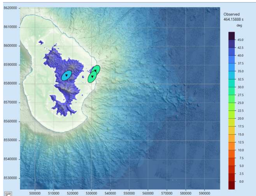
Figure 18 : Carte de tenseurs de phases calculés à 464 secondes des 3 stations MT du Revosima pour le mois de novembre 2023 (©BRGM et REVOSIMA).
