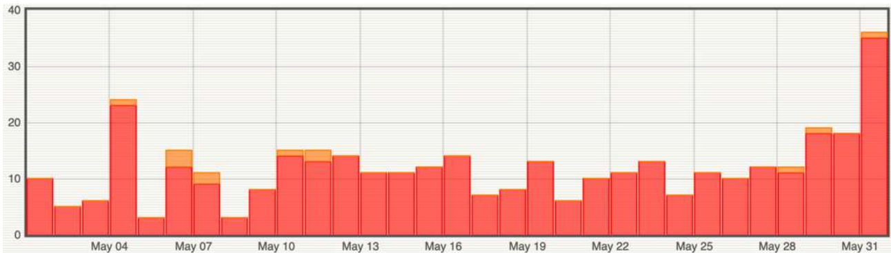
Figure 6 : Histogramme représentant le nombre de séismes par jour détectés en mai 2024 par le réseau sismologique du REVOSIMA. En rouge les séismes volcano-tectoniques, en orange les séismes longues périodes, en jaune les séismes très longues périodes (© OVPF-IPGP et REVOSIMA).
