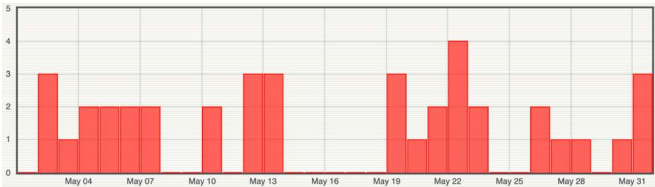
Figure 7 : Histogramme représentant le nombre de séismes par jour localisés en mai 2024 par le réseau sismologique du REVOSIMA. En rouge les séismes volcano-tectoniques, en orange les séismes longues périodes, en jaune les séismes très longues périodes (© OVPF-IPGP et REVOSIMA).
