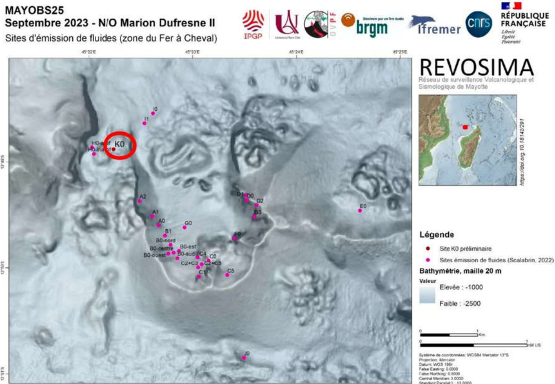
Figure 17 : Localisation des sites actifs d'émission de fluides fond de mer dans le périmètre élargi du Fer à Cheval (@Scalabrin, 2023- https://doi.org/10.12770/070818f6-6520-49e4-bafd-9d4d0609b77d ). Le nouveau site actif K0 observé (@Scalabrin & A. Potier) pour la première fois pendant la campagne MAYOBS25 y est intégré (entouré en rouge) (©REVOSIMA).
