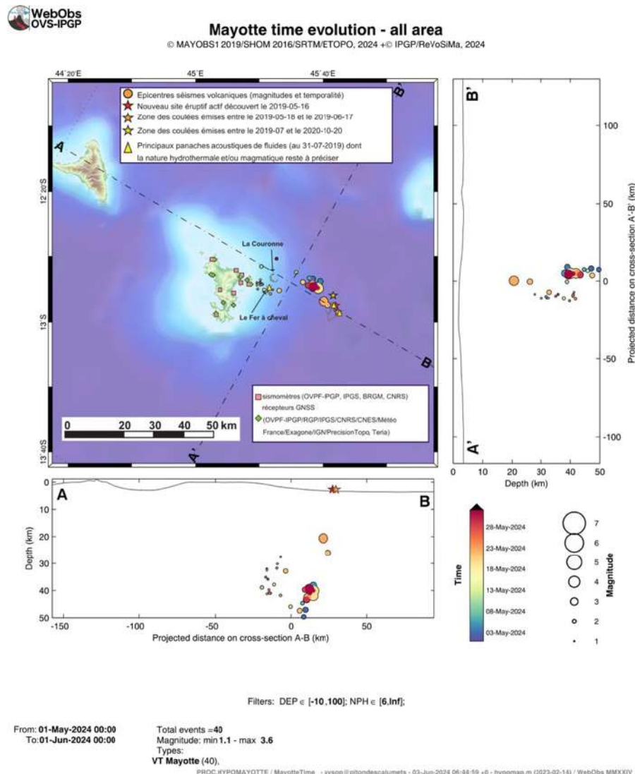
Figure 2 : Carte des épicentres ( \pm 5 km) des séismes volcano-tectoniques (VT) localisés avec les réseaux sismiques à terre (IPGP-CNRS-BRGM-BCSF-RENASS, ITES) entre le 1 er et le 31 mai 2024 (échelle temporelle de couleur). Sont aussi représentées les projections des hypocentres des séismes le long de coupes transverses et axiales le long de la ride montrant la localisation estimée en profondeur (la précision varie entre \pm 5 km et \pm 15 km) des séismes en fonction de la magnitude (taille des symboles) et de la date (échelle temporelle de couleur). La localisation approximative des panaches acoustiques identifiés pendant les campagnes océanographiques (MD220-MAYOBS1, MD221-MAYOBS2, MD222-MAYOBS3, MD223-MAYOBS4, MAYOBS15, MAYOBS17 ; Rinnert et al., 2019) et dont la nature hydrothermale et/ou magmatique reste à préciser, est indiquée par des triangles jaunes, l'étoile rouge indique le site éruptif nouvellement identifié le 16 mai 2019, l'étoile orange la zone des coulées émises entre le 18/05/2019 et le 17/06/2019 et l'étoile jaune la zone des coulées émises entre juillet 2019 et le 18/01/2021. Les structures volcaniques de la zone dite de « La Couronne », du « Fer à Cheval » sont indiquées en grisé tout comme les coulées de lave de Fani Maoré. Les stations sismiques du réseau terrestre et les stations de positionnement par satellite GPS sont indiquées par des symboles (voir légende). (©OVPF-IPGP, BRGM, IFREMER, CNRS, BCSF-RENASS, ITES / REVOSIMA).
