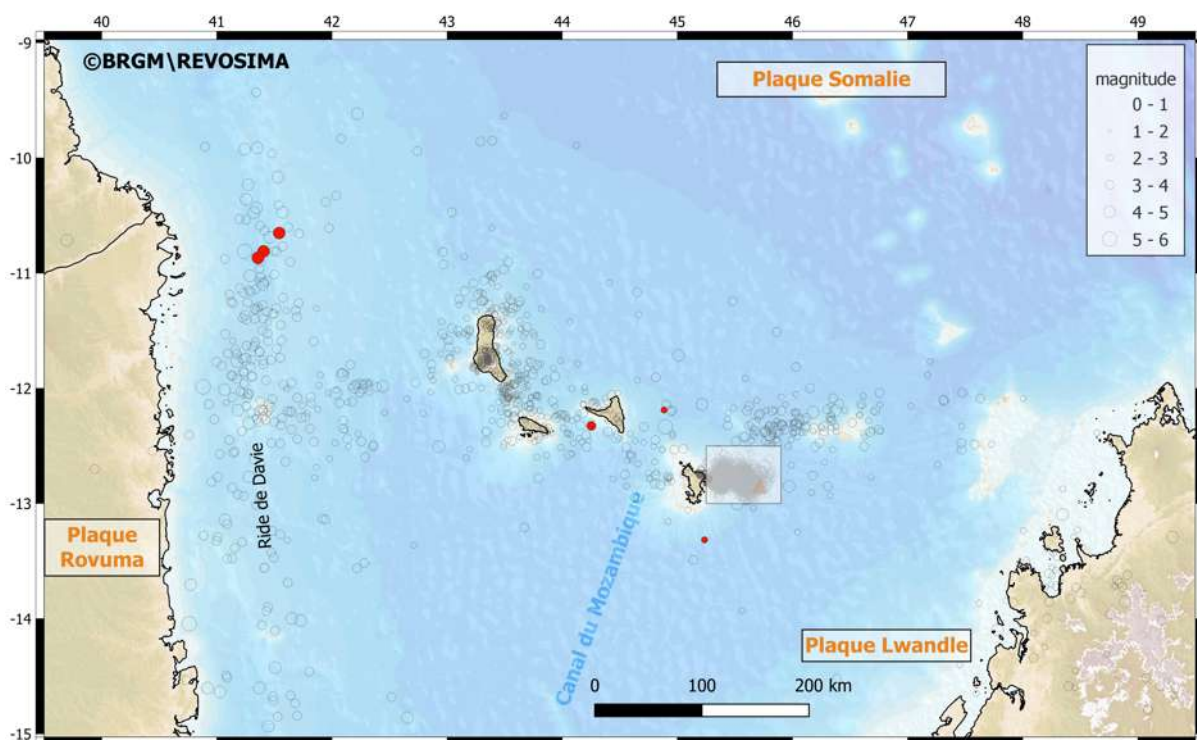
Figure 1: Sismicité régionale enregistrée depuis 2018 (modifié d'après Bertil et al. , 2021). Les séismes de mai 2024 sont représentés en rouge. Le fond de carte est construit à partir des données topographiques et bathymétriques de Gebco 2022 ( www.gebco.net ). Le trait de côte et les frontières administratives sont extraits de https://gadm.org/ . Le carré blanc encadre les essaims sismiques surveillés depuis 2018. Se référer aux Figures 2 et 3 de ce bulletin pour la distribution de cette sismicité.
