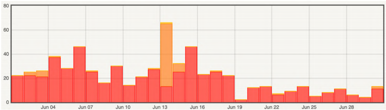
Figure 6 : Histogramme représentant le nombre de séismes par jour détectés en juin 2024 par le réseau sismologique du REVOSIMA. En rouge les séismes volcano-tectoniques, en orange les séismes longues périodes, en jaune les séismes très longues périodes (© OVPF-IPGP et REVOSIMA).
