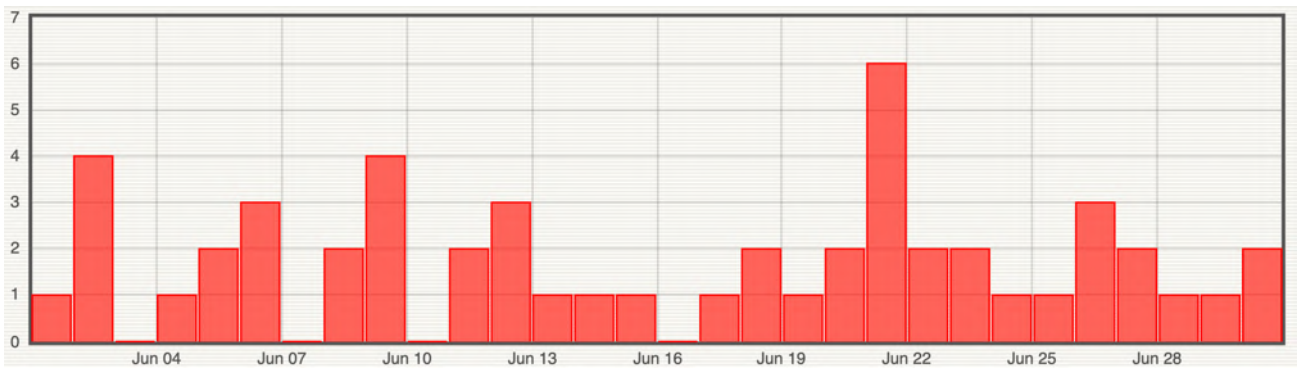
Figure 7 : Histogramme représentant le nombre de séismes par jour localisés en juin 2024 par le réseau sismologique du REVOSIMA. En rouge les séismes volcano-tectoniques, en orange les séismes longues périodes, en jaune les séismes très longues périodes (© OVPF-IPGP et REVOSIMA).
