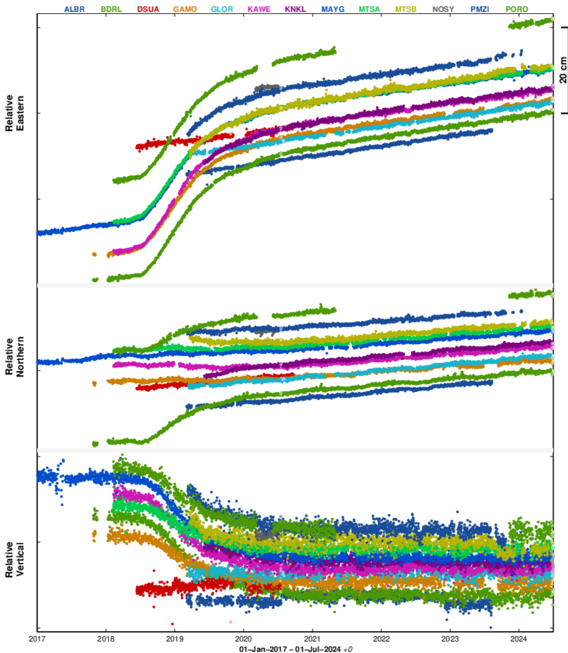
Figure 9 : Déplacements (en cm) enregistrés sur 9 stations GPS localisés à Mayotte (BDRL, GAMO, KAWE, KNKL, MAYG, MTSB, MTSB, PMZI, PORO), 1 station à Grande Glorieuse (GLOR), 1 station à Aldabra (ALBR) et 2 stations au nord de Madagascar à Diego Suarez (DSUA) et Nosy Be (NOSY) sur les composantes est (en haut), nord (au milieu) et vertical (en bas) entre le 1 er janvier 2017 et 30 juin 2024 pour visualiser une longue série temporelle ante crise. Post-traitement de ces données réalisé par l'IPGP (©OVPF-IPGP / REVOSIMA).
