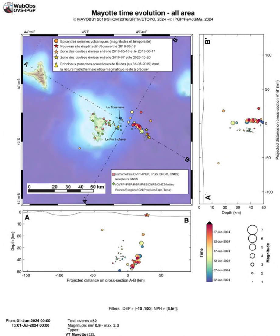
Figure 2 : Carte des épicentres ( \pm 5 km) des séismes volcano-tectoniques (VT) localisés avec les réseaux sismiques à terre (IPGP-CNRS-BRGM-BCSF-RENASS, ITES) entre le 1 er et le 30 juin 2024 (échelle temporelle de couleur). Sont aussi représentées les projections des hypocentres des séismes le long de coupes transversales et axiales le long de la ride montrant la localisation estimée en profondeur (la précision varie entre \pm 5 km et \pm 15 km) des séismes en fonction de la magnitude (taille des symboles) et de la date (échelle temporelle de couleur). La localisation approximative des panaches acoustiques identifiés pendant les campagnes océanographiques (MD220-MAYOBS1, MD221-MAYOBS2, MD222-MAYOBS3, MD223-MAYOBS4, MAYOBS15, MAYOBS17 ; Rinnert et al., 2019) et dont la nature hydrothermale et/ou magmatique reste à préciser, est indiquée par des triangles jaunes, l'étoile rouge indique le site éruptif nouvellement identifié le 16 mai 2019, l'étoile orange la zone des coulées émises entre le 18/05/2019 et le 17/06/2019 et l'étoile jaune la zone des coulées émises entre juillet 2019 et le 18/01/2021. Les structures volcaniques de la zone dite de « La Couronne », du « Fer à Cheval » sont indiquées en grisé tout comme les coulées de lave de Fani Maoré. Les stations sismiques du réseau terrestre et les stations de positionnement par satellite GPS sont indiquées par des symboles (voir légende). (©OVPF-IPGP, BRGM, IFREMER, CNRS, BCSF-RENASS, ITES / REVOSIMA).
