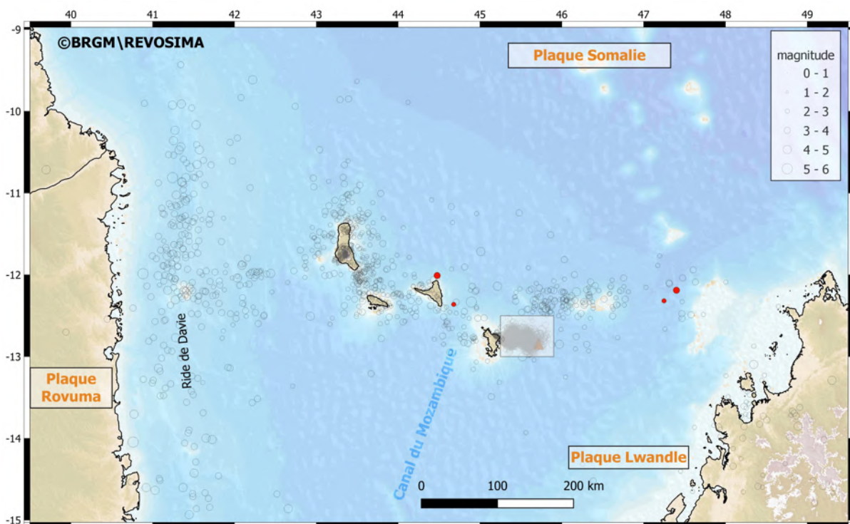
Figure 1: Sismicité régionale enregistrée depuis 2018 (modifié d'après Bertil et al. , 2021). Les séismes d'août 2024 sont représentés en rouge. Le fond de carte est construit à partir des données topographiques et bathymétriques de Gebco 2022 ( www.gebco.net ). Le trait de côte et les frontières administratives sont extraits de https://gadm.org/ . Le carré blanc encadre les essaims sismiques surveillés depuis 2018. Se référer aux Figures 2 et 3 de ce bulletin pour la distribution de cette sismicité.
