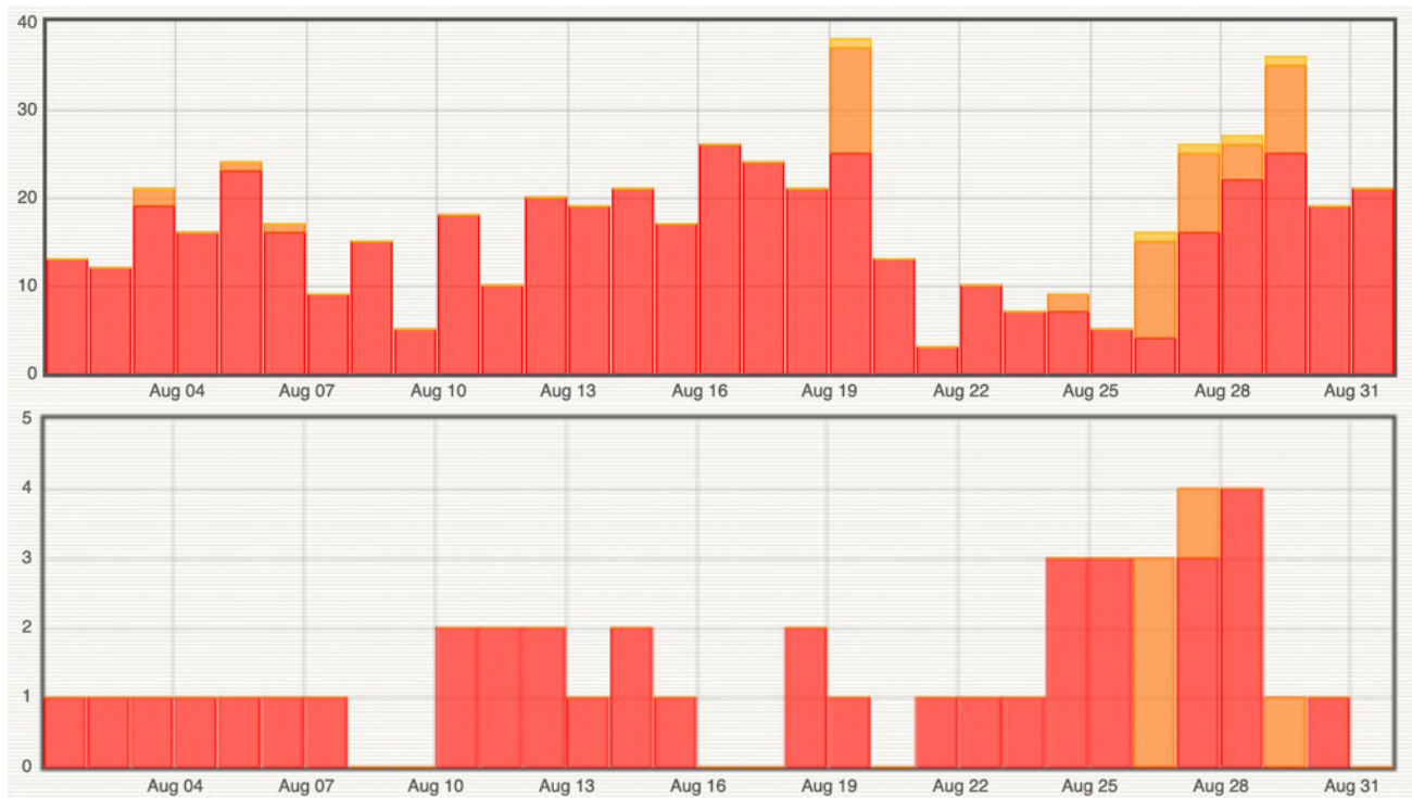
Figure 7 : Histogramme représentant le nombre de séismes par jour détectés (en haut) et localisés (en bas) en août 2024 par le réseau sismologique du REVOSIMA. En rouge les séismes volcano-tectoniques, en orange les séismes longues périodes, en jaune les séismes très longues périodes (© OVPF-IPGP et REVOSIMA).
