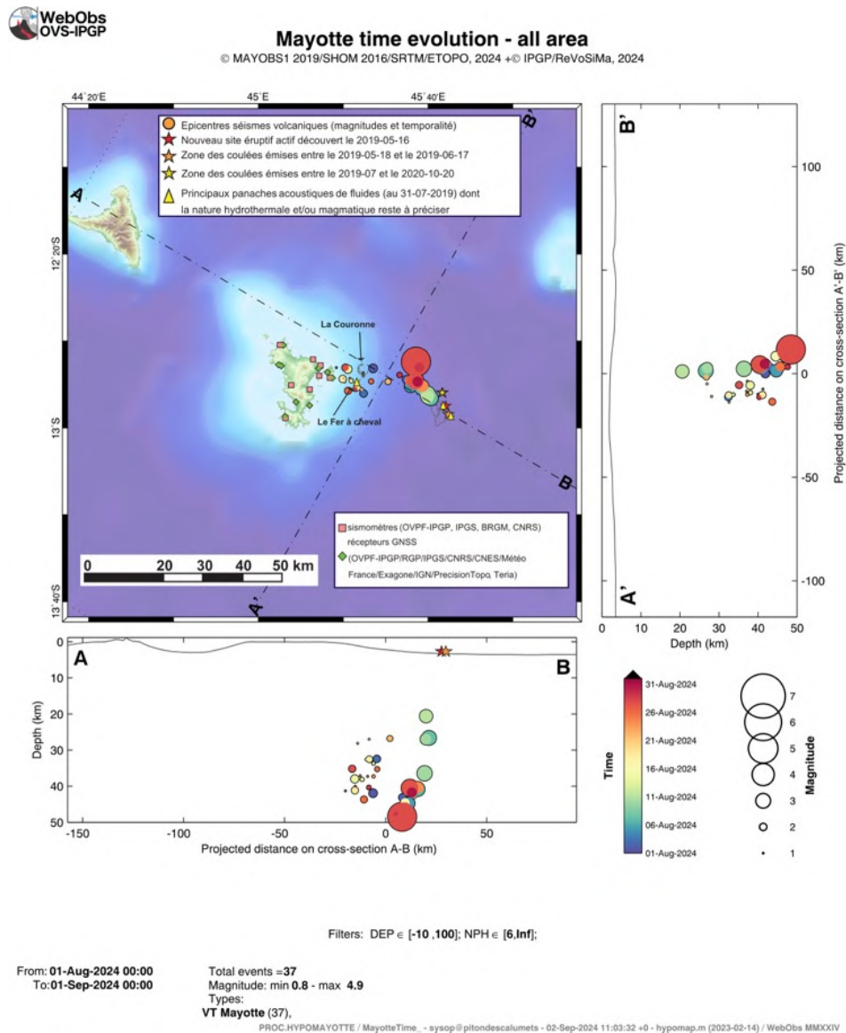
Figure 2 : Carte des épicentres ( \pm 5 km) des séismes volcano-tectoniques (VT) localisés avec les réseaux sismiques à terre (IPGP-CNRS-BRGM-BCSF-RENASS, ITES) entre le 1 er et le 31 août 2024 (échelle temporelle de couleur). Sont aussi représentées les projections des hypocentres des séismes le long de coupes transversales et axiales le long de la ride montrant la localisation estimée en profondeur (la précision varie entre \pm 5 km et \pm 15 km) des séismes en fonction de la magnitude (taille des symboles) et de la date (échelle temporelle de couleur). La localisation approximative des panaches acoustiques identifiés pendant les campagnes océanographiques (MD220-MAYOBS1, MD221-MAYOBS2, MD222-MAYOBS3, MD223-MAYOBS4, MAYOBS15, MAYOBS17 ; Rinnert et al., 2019) est indiquée par des triangles jaunes, l'étoile rouge indique le site éruptif identifié le 16 mai 2019, l'étoile orange la zone des coulées émises entre le 18/05/2019 et le 17/06/2019 et l'étoile jaune la zone des coulées émises entre juillet 2019 et le 18/01/2021. Les structures volcaniques de la zone dite de « La Couronne », du « Fer à Cheval » sont indiquées en grisé tout comme les coulées de lave de Fani Maoré. Les stations sismiques du réseau terrestre et les stations de positionnement par satellite GPS sont indiquées par des symboles (voir légende). (©OVPF-IPGP, BRGM, IFREMER, CNRS, BCSF-RENASS, ITES / REVOSIMA).
