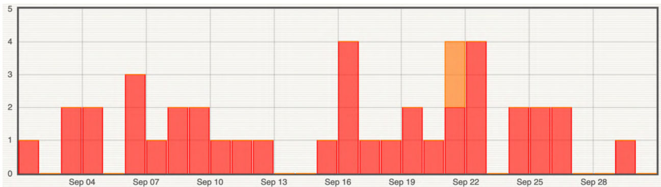
Figure 7 : Histogramme représentant le nombre de séismes par jour localisés en septembre 2024 par le réseau sismologique du REVOSIMA. En rouge les séismes volcano-tectoniques, en orange les séismes longues périodes, en jaune les séismes très longues périodes (© OVPF-IPGP et REVOSIMA).
