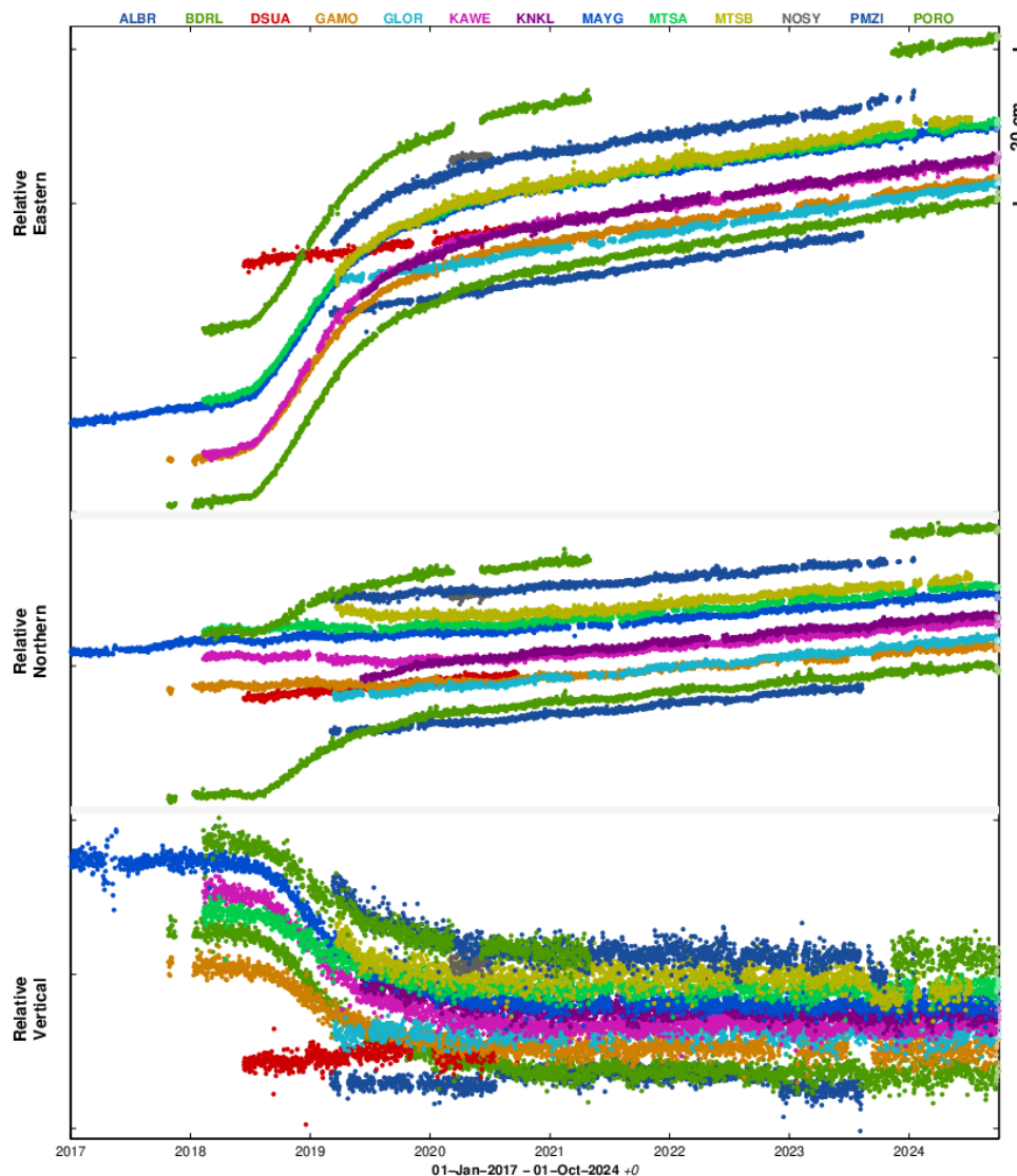
Figure 9 : Déplacements (en cm) enregistrés sur 9 stations GPS localisés à Mayotte (BDRL, GAMO, KAWE, KNKL, MAYG, MTSB, PMZI, PORO), 1 station à Grande Glorieuse (GLOR), 1 station à Aldabra (ALBR) et 2 stations au nord de Madagascar à Diego Suarez (DSUA) et Nosy Be (NOSY) sur les composantes est (en haut), nord (au milieu) et vertical (en bas) entre le 1 er janvier 2017 et 30 septembre 2024 pour visualiser une longue série temporelle ante crise. Post-traitement de ces données réalisé par l'IPGP (©OVPF-IPGP / REVOSIMA).
