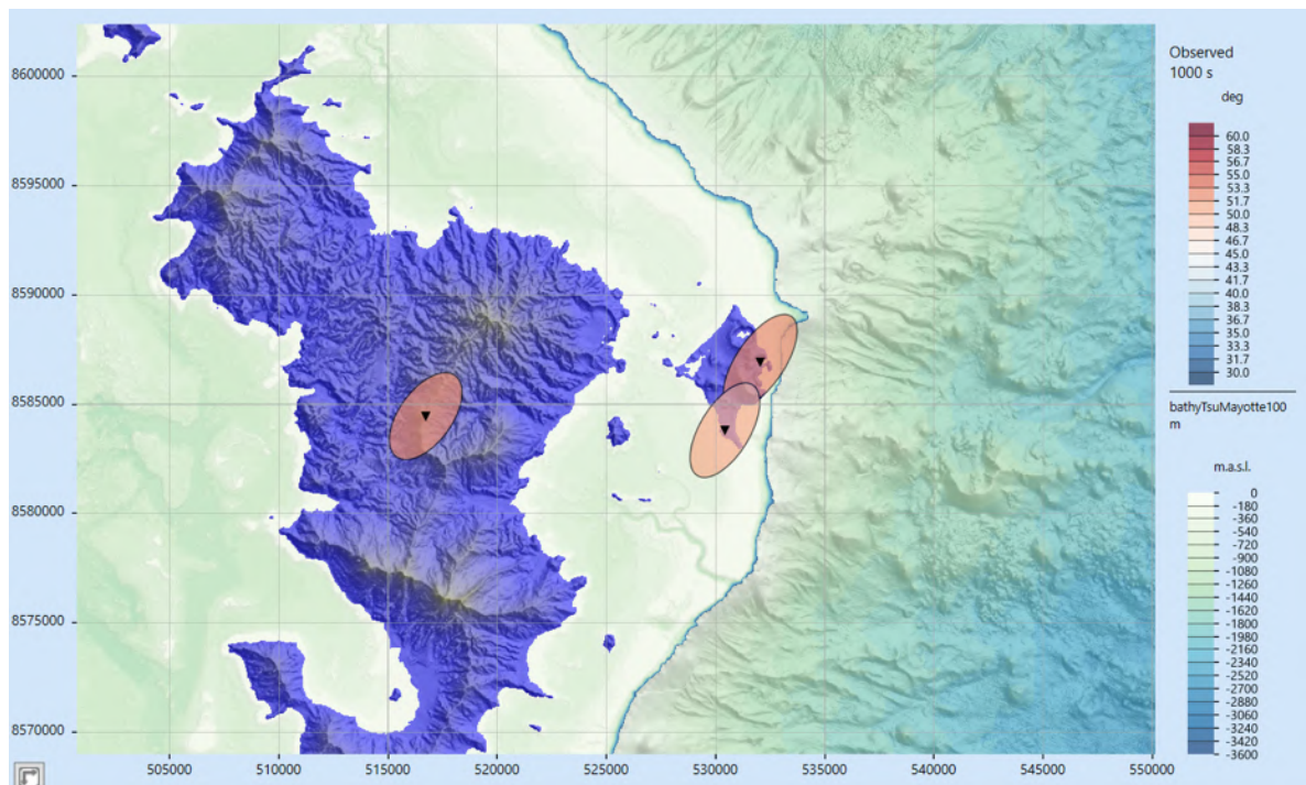
Figure 18 : Carte de tenseurs de phases calculés à 1000 secondes des 3 stations MT du Revosima pour le mois de septembre 2024 (©BRGM et REVOSIMA). Les ellipses de tenseurs de phases sont colorées avec les valeurs de phase maximum \varphi_{max} (en degrés) qui sont supérieures à 45°, traduisant ainsi une décroissance de résistivité en profondeur.
