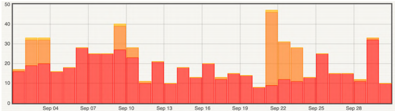
Figure 6 : Histogramme représentant le nombre de séismes par jour détectés en septembre 2024 par le réseau sismologique du REVOSIMA. En rouge les séismes volcano-tectoniques, en orange les séismes longues périodes, en jaune les séismes très longues périodes (© OVPF-IPGP et REVOSIMA).
