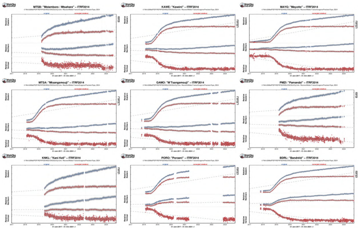
Figure 10 : Déplacements (en cm) enregistrés sur les 9 stations GPS localisés à Mayotte (MTSB, KAWÉ, MAYG, M TSA, GAMO, PMZI, KNKL, PORO, BDRL) entre le 1 er janvier 2017 et le 30 septembre 2024 pour visualiser une longue série temporelle ante crise. En bleu les données brutes, en rouge les données corrigées du mouvement de la plaque. Les stations sont présentées dans un ordre géographique ; du nord au sud (de haut en bas) et d'ouest en est (de gauche à droite). Post-traitement de ces données réalisé par l'IPGP (©OVPF-IPGP / REVOSIMA).
