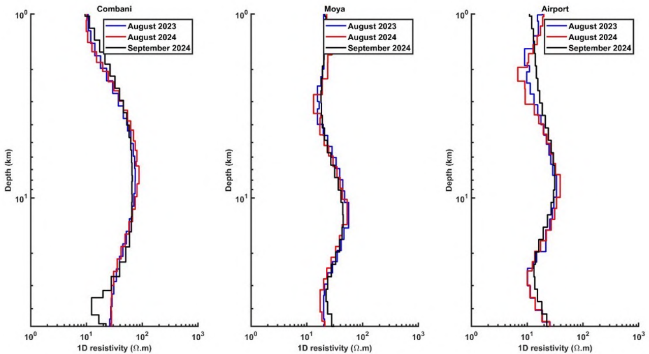
Figure 19 : Modèles 1D de Résistivité du sous-sol de 1 km à 50 km de profondeur sous Combani (gauche), Moya (centre) et Aéroport (droite) pour les mois d'août 2023 (bleu), août 2024 (rouge) et septembre 2024 (noir).
