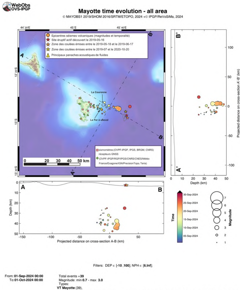
Figure 2 : Carte des épicentres ( \pm 5 km) des séismes volcano-tectoniques (VT) localisés avec les réseaux sismiques à terre (IPGP-CNRS-BRGM-BCSF-RENAISS, ITES) entre le 1 er et le 30 septembre 2024 (échelle temporelle de couleur). Sont aussi représentées les projections des hypocentres des séismes le long de coupes transversales et axiales le long de la ride montrant la localisation estimée en profondeur (la précision varie entre \pm 5 km et \pm 15 km) des séismes en fonction de la magnitude (taille des symboles) et de la date (échelle temporelle de couleur). La localisation approximative des panaches acoustiques identifiés pendant les campagnes océanographiques (MD220-MAYOBS1, MD221-MAYOBS2, MD222-MAYOBS3, MD223-MAYOBS4, MAYOBS15, MAYOBS17 ; Rinnert et al., 2019) est indiquée par des triangles jaunes, l'étoile rouge indique le site éruptif identifié le 16 mai 2019, l'étoile orange la zone des coulées émises entre le 18/05/2019 et le 17/06/2019 et l'étoile jaune la zone des coulées émises entre juillet 2019 et le 18/01/2021. Les structures volcaniques de la zone dite de « La Couronne », du « Fer à Cheval » sont indiquées en gris tout comme les coulées de lave de Fani Maoré. Les stations sismiques du réseau terrestre et les stations de positionnement par satellite GPS sont indiquées par des symboles (voir légende). (©OVPF-IPGP, BRGM, IFREMER, CNRS, BCSF-RENAISS, ITES / REVOSIMA).
