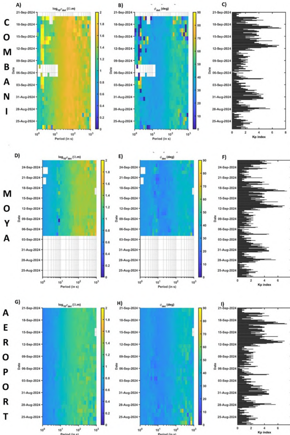
Figure 21 : Période du 23/08/2024 au 26/09/2024 - Chroniques temps-période de résistivité apparente de l'invariant 1D MT en échelle logarithmique (a, d, g), de phases (b, e, h) et l'index géomagnétique Kp (c, f, i) du réseau MT Revosima (©BRGM et REVOSIMA) pour le site de Combani (haut), Moya (centre) et Aéroport (bas). Des conditions particulières de bruits anthropiques empêchent épisodiquement l'algorithme de converger lors du calcul des chroniques de Combani et l'Aéroport entre le 22 et le 26 septembre, ce qui explique que les chroniques sont plus courtes. On peut également observer que les orages géomagnétiques du 12 et 18 septembre permettent d'obtenir des courbes plus lisses en fréquences.
