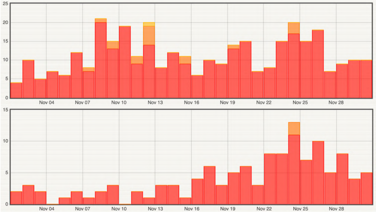
Figure 7 : Histogramme représentant le nombre de séismes par jour détectés (en haut) et localisés (en bas) en novembre 2024 par le réseau sismologique du REVOSIMA. En rouge les séismes volcano-tectoniques, en orange les séismes longues périodes, en jaune les séismes très longues périodes (© OVPF-IPGP et REVOSIMA).
