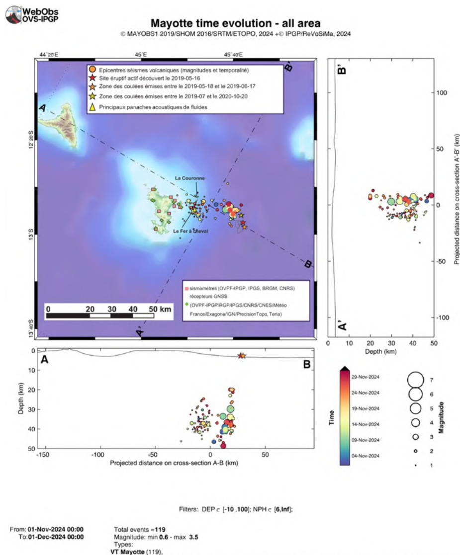
Figure 2 : Carte des épencentres ( \pm 5 km) des séismes volcano-tectoniques (VT) localisés avec les réseaux sismiques à terre (IPGP-CNRS-BRGM-BCSF-RENASS, ITES) entre le 1 er et le 30 novembre 2024 (échelle temporelle de couleur). Sont aussi représentées les projections des hypocentres des séismes le long de coupes transverses et axiales le long de la ride montrant la localisation estimée en profondeur (la précision varie entre \pm 5 km et \pm 15 km) des séismes en fonction de la magnitude (taille des symboles) et de la date (échelle temporelle de couleur). La localisation approximative des panaches acoustiques identifiés pendant les campagnes océanographiques est indiquée par des triangles jaunes, l'étoile rouge indique le site éruptif identifié le 16 mai 2019, l'étoile orange la zone des coulées émises entre le 18/05/2019 et le 17/06/2019 et l'étoile jaune la zone des coulées émises entre juillet 2019 et le 18/01/2021. Les structures volcaniques de la zone dite de « La Couronne », du « Fer à Cheval » sont indiquées en grisé tout comme les coulées de lave de Fani Maoré. Les stations sismiques du réseau terrestre et les stations de positionnement par satellite GPS sont indiquées par des symboles (voir légende). (©OVPF-IPGP, BRGM, IFREMER, CNRS, BCSF-RENASS, ITES / REVOSIMA).
