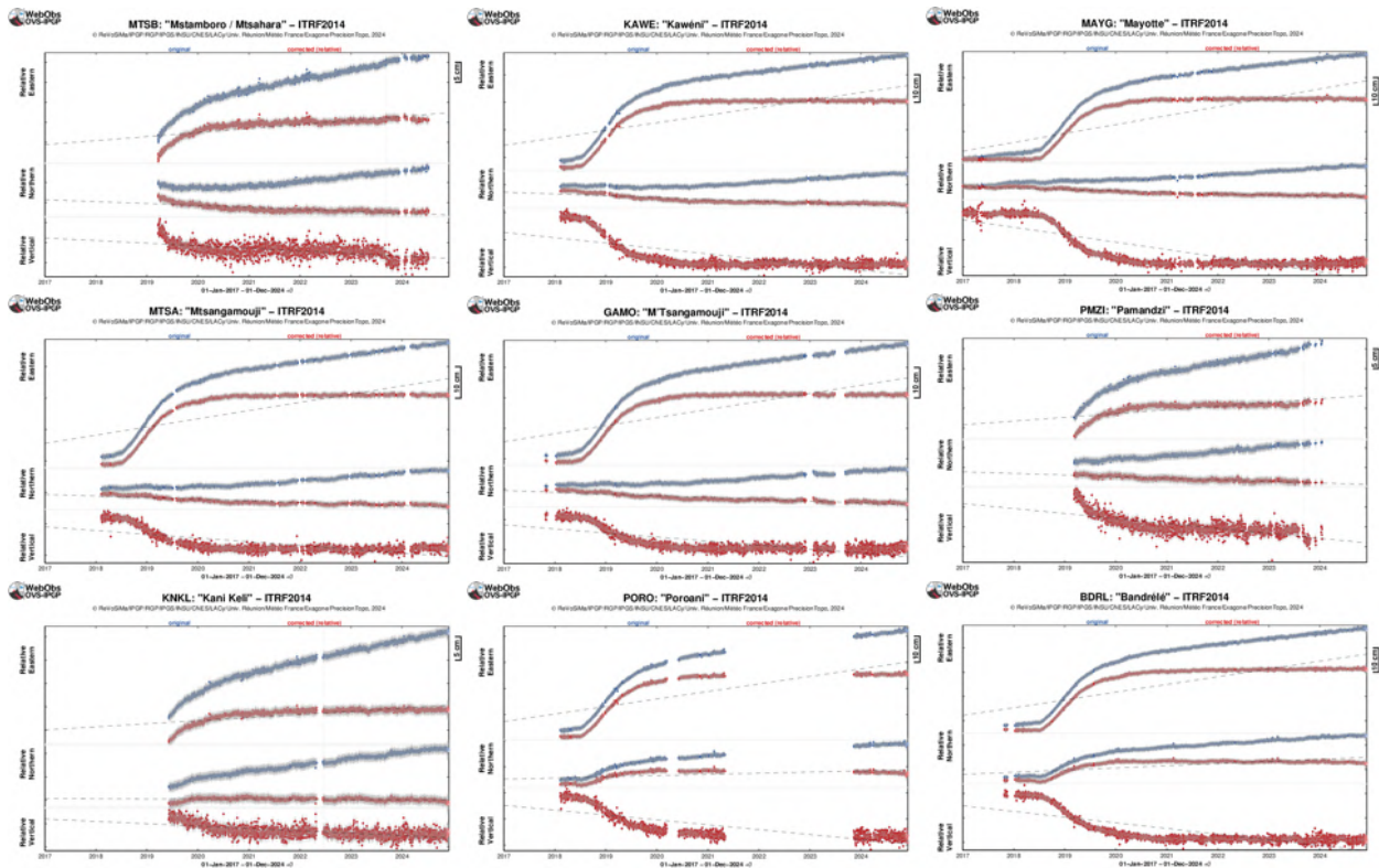
Figure 10 : Déplacements (en cm) enregistrés sur les 9 stations GPS localisés à Mayotte (MTSB, KAWE, MAYG, M TSA, GAMO, PMZI, KNKL, PORO, BDRL) entre le 1 er janvier 2017 et le 30 novembre 2024 pour visualiser une longue série temporelle ante crise. En bleu les données brutes, en rouge les données corrigées du mouvement de la plaque. Les stations sont présentées dans un ordre géographique ; du nord au sud (de haut en base à et d'ouest en est (de gauche à droite). Post-traitement de ces données réalisé par l'IPGP (©OVPF-IPGP / REVOSIMA).
