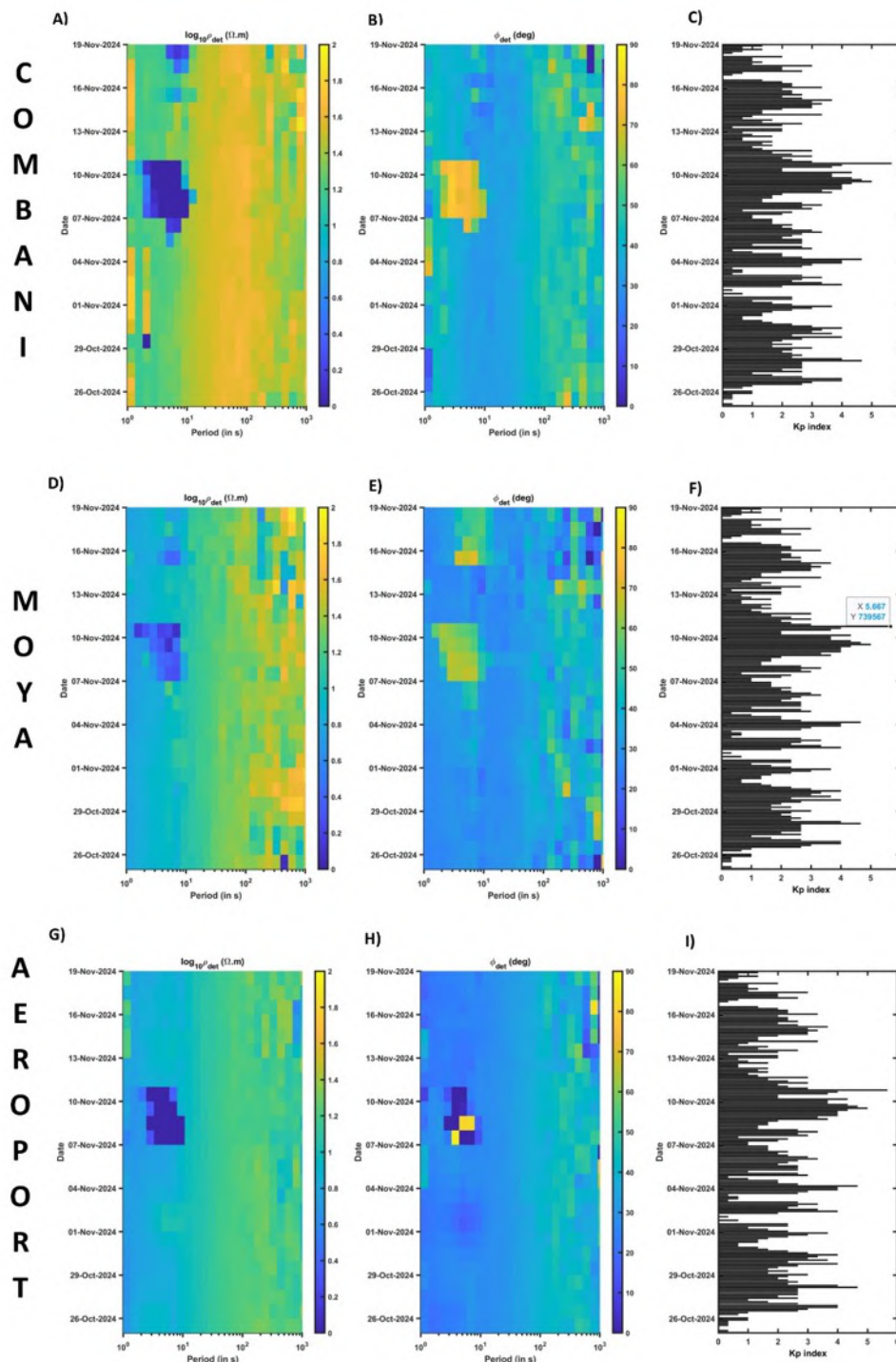
Figure 21 : Période du 23/10/2024 au 19/11/2024 - Chroniques temps-période de résistivité apparente de l'invariant 1D MT en échelle logarithmique (a, d, g), de phases (b, e, h) et l'index géomagnétique Kp (c, f, i) du réseau MT Revosima (©BRGM et REVOSIMA) pour le site de Combani (haut), Moya (centre) et Aéroport (bas). Les 3 stations présentent des périodes de bruits synchrones centrées sur la bande de fréquences entre [0.1 Hz - 1 Hz] entre le 7 et le 10 Novembre, provoquant des variations sur les chroniques temporelles MT non attribuables à des variations de la structure géo-électrique du sous-sol sous les stations.
