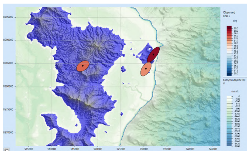
Figure 18 : Carte de tenseurs de phases calculés à 800 secondes des 3 stations MT du Revosima pour le mois de novembre 2024 (©BRGM et REVOSIMA). Les ellipses de tenseurs de phases sont colorées avec les valeurs de phase maximum \varphi_{max} (en degrés) qui sont supérieures à 45°, traduisant ainsi une décroissance de résistivité en profondeur.
