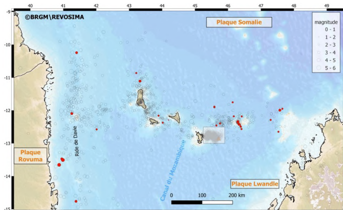
Figure 1: Sismicité régionale enregistrée depuis 2018 (modifié d'après Bertil et al., 2021). Les séismes de novembre 2024 sont représentés en rouge. Le fond de carte est construit à partir des données topographiques et bathymétriques de Gebco 2022 ( www.gebco.net ). Le trait de côte et les frontières administratives sont extraits de https://gadm.org/ . Le carré blanc encadre les essaims sismiques surveillés depuis 2018. Se référer aux Figures 2 et 3 de ce bulletin pour la distribution de cette sismicité.
