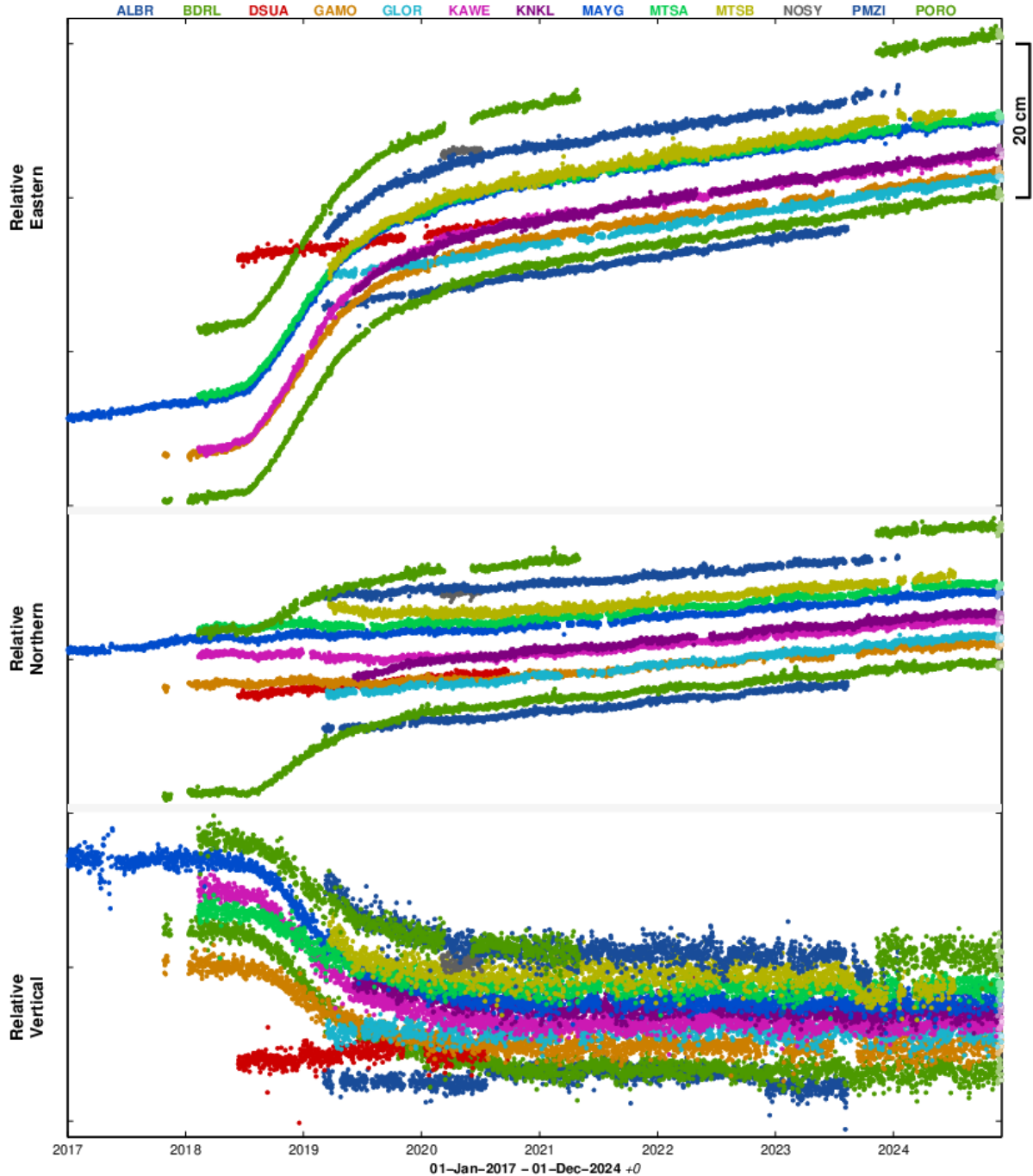
Figure 9 : Déplacements (en cm) enregistrés sur 9 stations GPS localisés à Mayotte (BDRL, GAMO, KAWE, KNKL, MAYG, MTSA, MTSB, PMZI, PORO), 1 station à Grande Glorieuse (GLOR), 1 station à Aldabra (ALBR) et 2 stations au nord de Madagascar à Diego Suarez (DSUA) et Nosy Be (NOSY) sur les composantes est (en haut), nord (au milieu) et vertical (en bas) entre le 1 er janvier 2017 et 30 novembre 2024 pour visualiser une longue série temporelle ante crise. Post-traitement de ces données réalisé par l'IPGP (©OVPF-IPGP / REVOSIMA).
