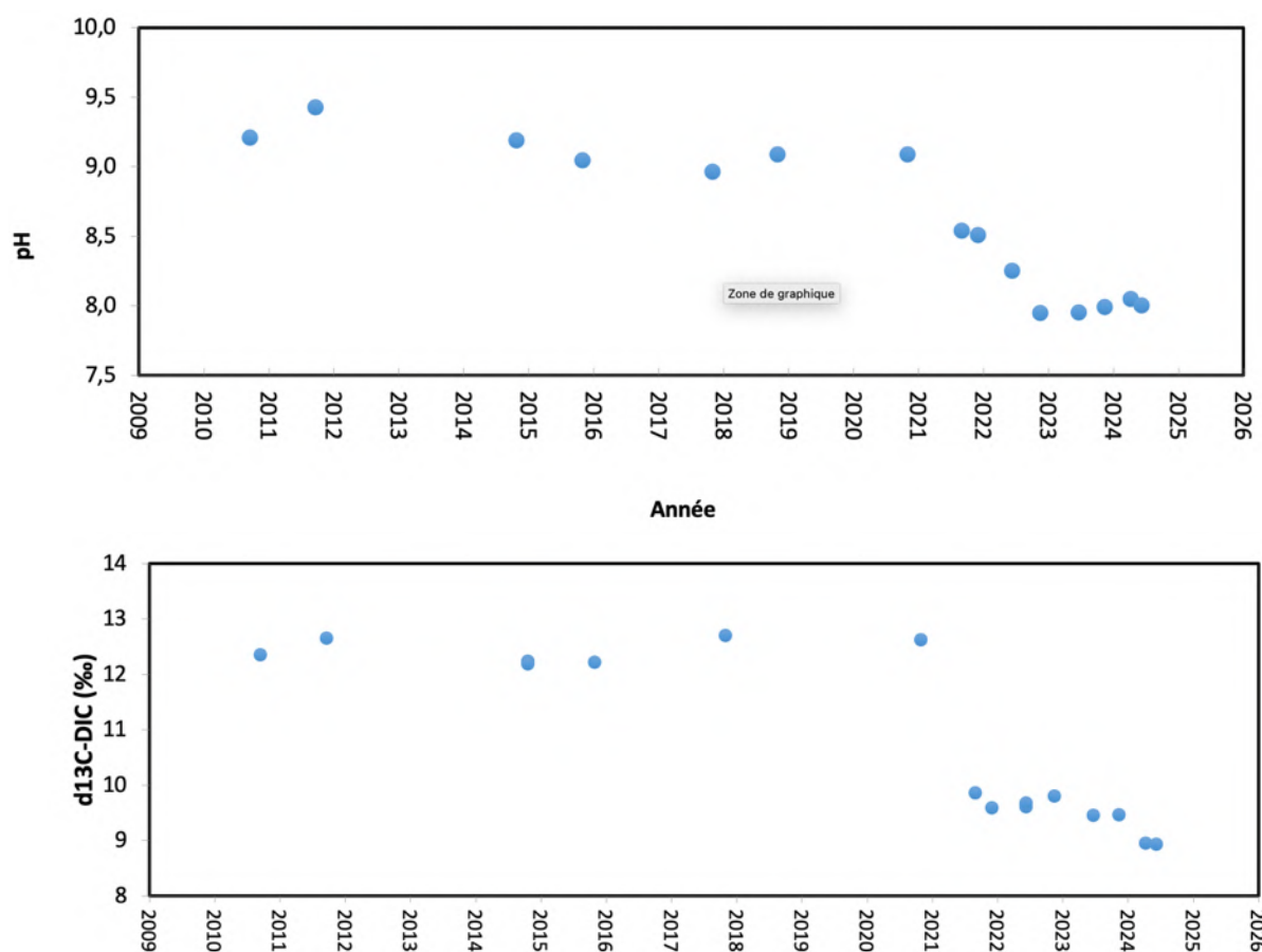
Figure 16 : Évolution temporelle du pH et du \delta^{13}C_{DIC} des eaux du Dziani Dzaha. Données antérieures à 2015 issues de Sarazin et al., (2021) et Cadeau et al., (2020). Données de 2016 à 2021 issues de Cadeau et al., (2022). Données de 2022 et 2024 non publiées.
