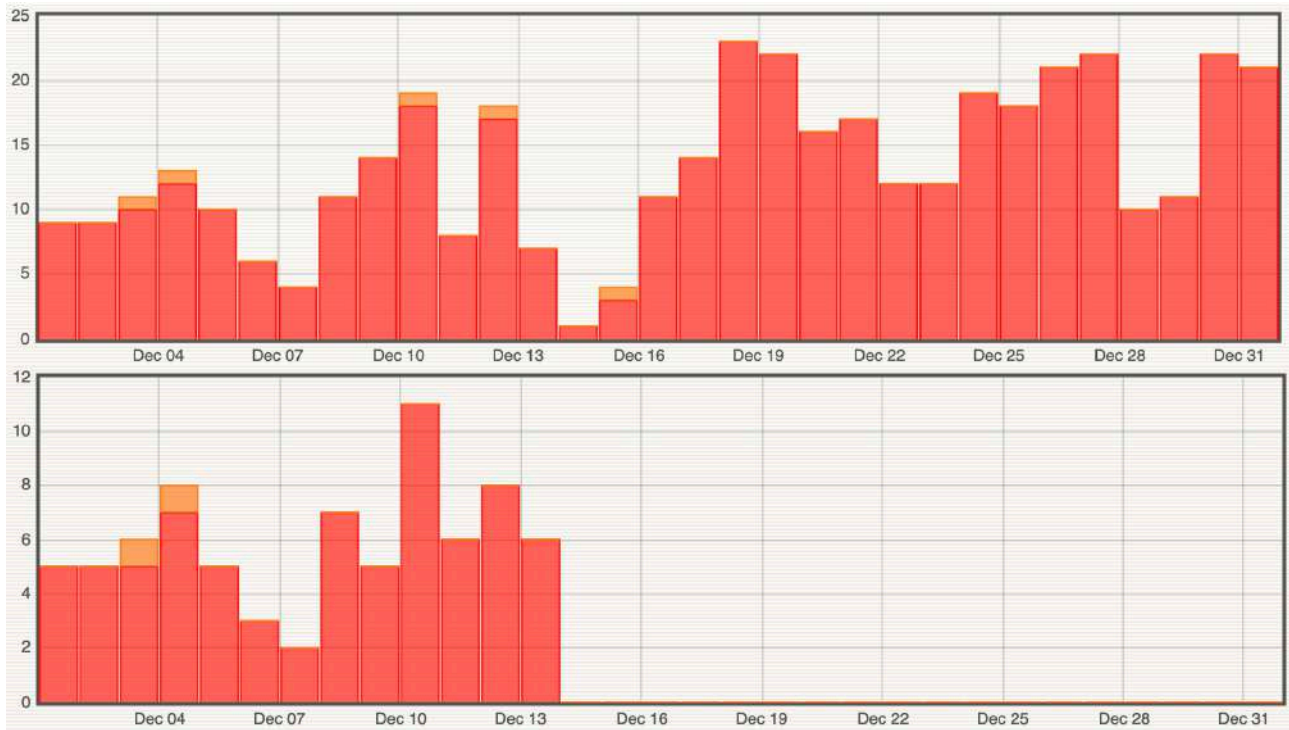
Figure 7 : Histogramme représentant le nombre de séismes par jour détectés (en haut) et localisés (en bas) en décembre 2024 par le réseau sismologique du REVOSIMA. En rouge les séismes volcano-tectoniques, en orange les séismes longues périodes, en jaune les séismes très longues périodes (© OVPF-IPGP et REVOSIMA). Suite au passage du cyclone Chido sur Mayotte et à la perte de données de la majorité des stations sismologiques, il n'a pas été possible de localiser les séismes entre le 14 et le 31 décembre.
