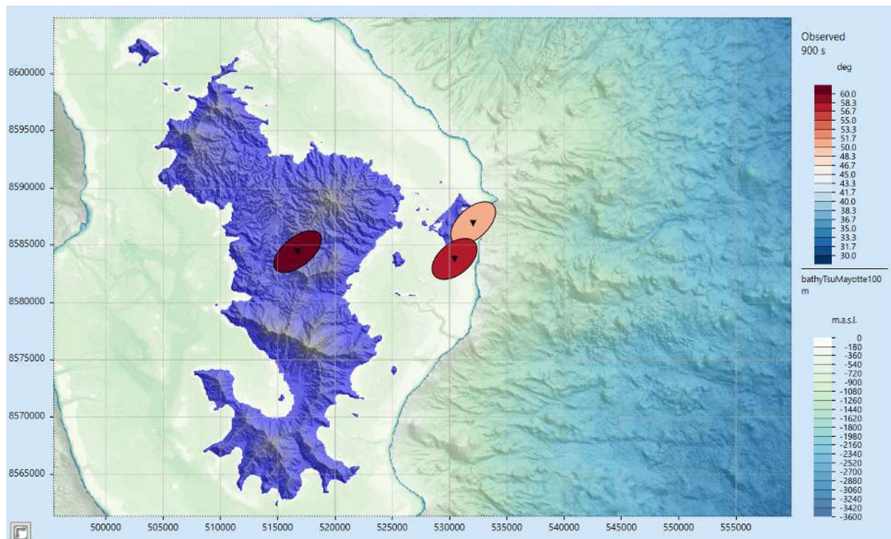
Figure 18 : Carte de tenseurs de phases calculés à une période de 900 secondes des 3 stations MT du Revosima pour le mois de Décembre 2024 (©BRGM et REVOSIMA). Les ellipses de tenseurs de phases sont colorées avec les valeurs de phase maximum \varphi_{max} (en degrés) qui sont supérieures à 45^\circ , traduisant ainsi une décroissance de résistivité en profondeur.
