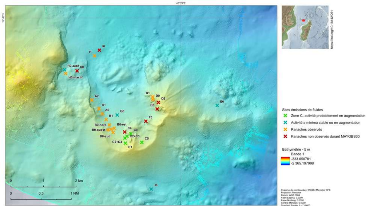
Figure 17 : Localisation des sites actifs d'émission de fluides fond de mer dans le périmètre élargi du Fer à Cheval identifiés pendant la campagne MAYOBS30 sur la base d'une analyse préliminaire à bord (@Scalabrin, 2023- https://doi.org/10.12770/070818f6-6520-49e4-bafd-9d4d0609bf7d ). (©REVOSIMA).
