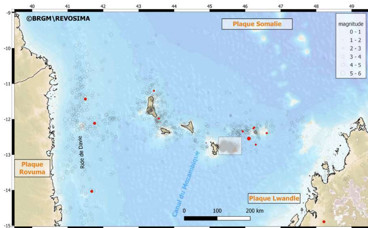
Figure 1: Sismicité régionale enregistrée depuis 2018 (modifié d'après Bertil et al., 2021). Les séismes de décembre 2024 sont représentés en rouge. Le fond de carte est construit à partir des données topographiques et bathymétriques de Gebco 2022 ( www.gebco.net ). Le trait de côte et les frontières administratives sont extraits de https://gadm.org/ . Le carré blanc encadre les essaims sismiques surveillés depuis 2018. Se référer aux Figures 2 et 3 de ce bulletin pour la distribution de cette sismicité.
