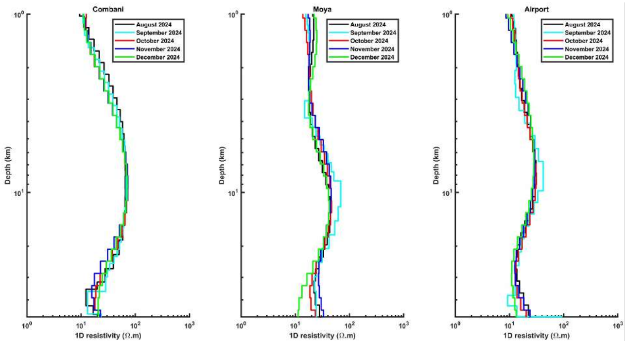
Figure 19 : Modèles 1D de résistivité du sous-sol de 1km à 50 km de profondeur sous Combani (gauche), Moya (centre) et Aéroport (droite) pour les mois d'août 2024 (noir), septembre 2024 (cyan), octobre 2024 (rouge), novembre 2024 (bleu) et décembre 2024 (vert).
