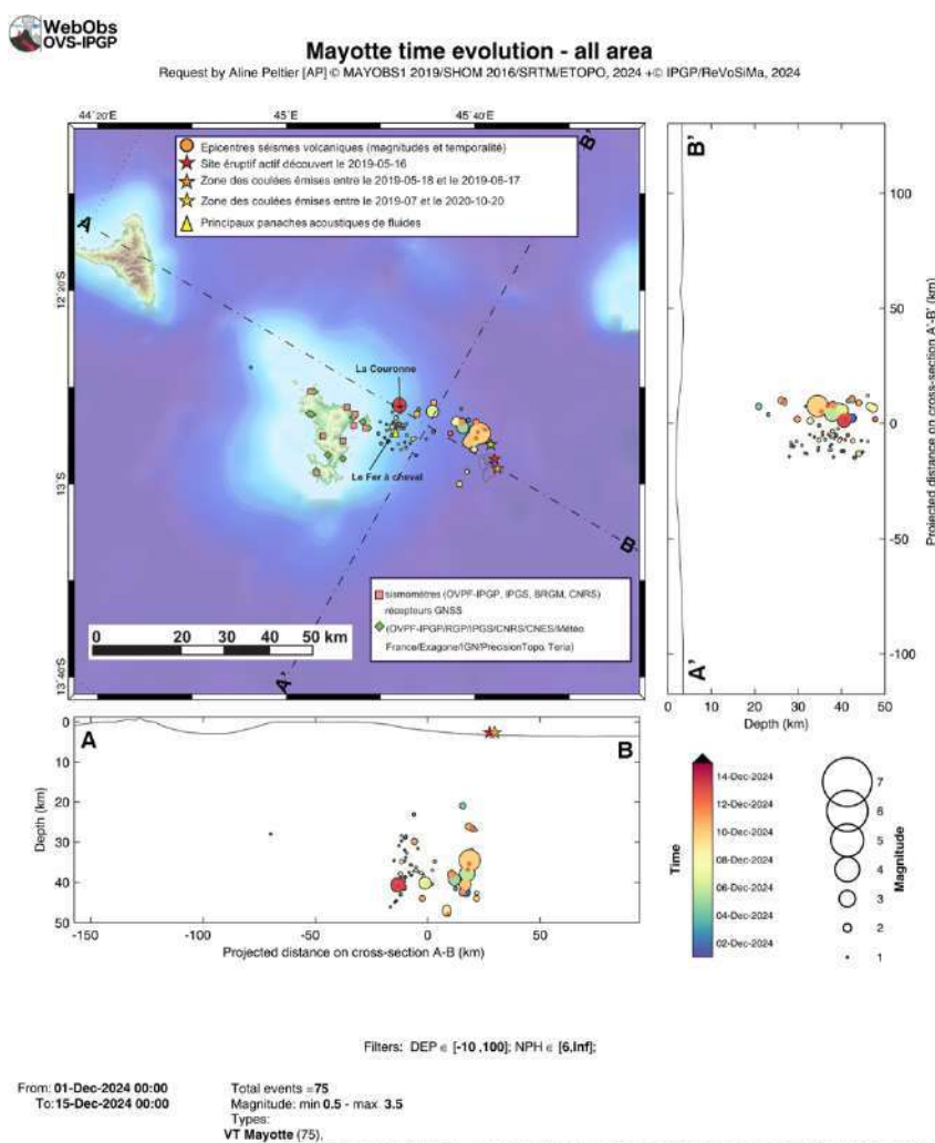
Figure 2 : Carte des épicentres ( \pm 5 km) des séismes volcano-tectoniques (VT) localisés avec les réseaux sismiques à terre (IPGP-CNRS-BRGM-BCSF-RENASS, ITES) entre le 1 er et le 14 décembre 2024 (échelle temporelle de couleur). Sont aussi représentées les projections des hypocentres des séismes le long de coupes transverses et axiales le long de la ride montrant la localisation estimée en profondeur (la précision varie entre \pm 5 km et \pm 15 km) des séismes en fonction de la magnitude (taille des symboles) et de la date (échelle temporelle de couleur). La localisation approximative des panaches acoustiques identifiés pendant les campagnes océanographiques est indiquée par des triangles jaunes, l'étoile rouge indique le site éruptif identifié le 16 mai 2019, l'étoile orange la zone des coulées émises entre le 18/05/2019 et le 17/06/2019 et l'étoile jaune la zone des coulées émises entre juillet 2019 et le 18/01/2021. Les structures volcaniques de la zone dite de « La Couronne », du « Fer à Cheval » sont indiquées en grisé tout comme les coulées de lave de Fani Maoré. Les stations sismiques du réseau terrestre et les stations de positionnement par satellite GPS sont indiquées par des symboles (voir légende). (©OVPF-IPGP, BRGM, IFREMER, CNRS, BCSF-RENASS, ITES / REVOSIMA).
