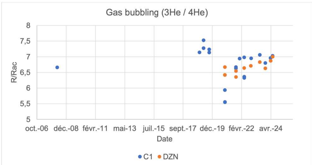
Figure 14 : Analyses isotopiques (gaz rares) des bullages aux points de contrôle C1 (estran de l'aéroport) et DZN (Lac Dziiani). Une augmentation du R/Rac (rapport isotopique de l'He normalisé à celui de l'atmosphère) est liée à une augmentation de la contribution des fluides profonds remontant du manteau. Erreur moyenne sur chaque analyse : 0.05 unité.
