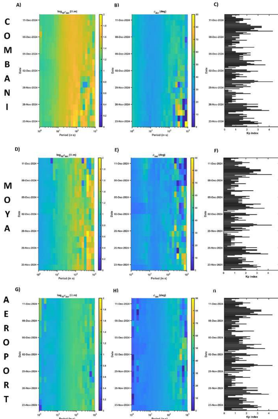
Figure 21 : Période du 20/11/2024 au 13/12/2024 - Chroniques temps-période de résistivité apparente de l'invariant 1D MT en échelle logarithmique (a, d, g), de phases (b, e, h) et l'index géomagnétique Kp (c, f, i) du réseau MTRevosima (©BRGM et REVOSIMA) pour le site de Combani (haut), Moya (centre) et Aéroport (bas). Les stations de Moya et de Combani présentent des variations aux périodes >100 secondes attribuables à une dégradation progressive de la qualité du contact de leurs électrodes, provoquant des variations sur les chroniques temporelles MT non attribuables à des variations de la structure géo-électrique du sous-sol sous les stations.
