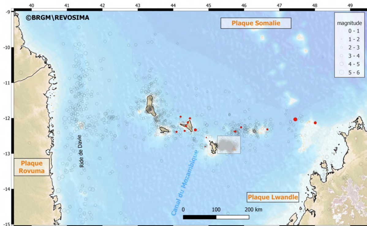
Figure 1: Sismicité régionale enregistrée depuis 2018 (modifié d'après Bertil et al. , 2021). Les séismes de janvier 2025 sont représentés en rouge. Le fond de carte est construit à partir des données topographiques et bathymétriques de Gebco 2022 ( www.gebco.net ). Le trait de côte et les frontières administratives sont extraits de https://gadm.org/ . Le carré blanc encadre les essaims sismiques surveillés depuis 2018. Se référer aux Figures 2 et 3 de ce bulletin pour la distribution de cette sismicité.
