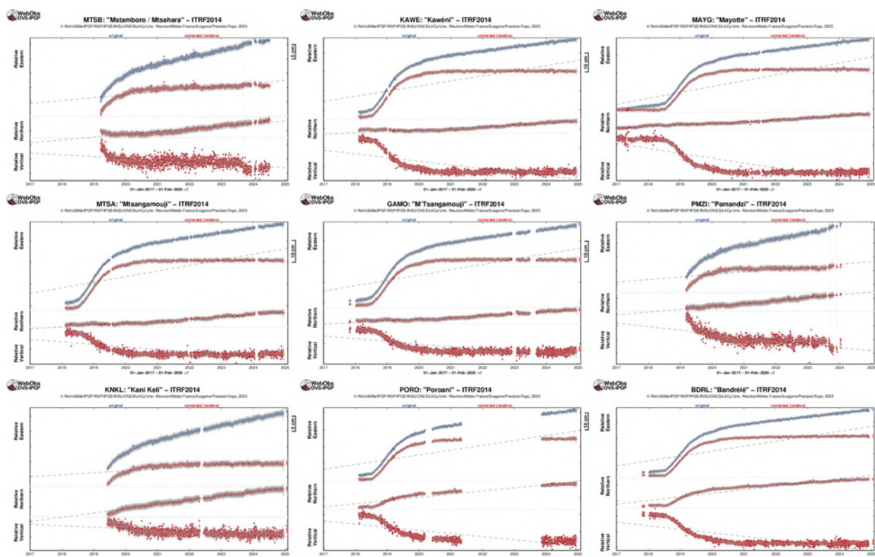
Figure 10 : Déplacements (en cm) enregistrés sur les 9 stations GPS localisés à Mayotte (MTSB, KAWE, MAYG, MTSA, GAMO, PMZI, KNKL, PORO, BDRL) entre le 1 er janvier 2017 et le 31 janvier 2025 pour visualiser une longue série temporelle ante crise. En bleu les données brutes, en rouge les données corrigées du mouvement de la plaque. Les stations sont présentées dans un ordre géographique ; du nord au sud (de haut en base à et d'ouest en est (de gauche à droite)). Post-traitement de ces données réalisé par l'IPGP (©OVPF-IPGP / REVOSIMA). Suite au passage du cyclone Chido sur Mayotte le 14 décembre 2024, deux stations (MAYG et MTSA) ont été détruites, alors que les stations KNKL, KAWE, PORO, GAMO et BDRL ont subi des coupures électriques et/ou de transmission. Au retour des données, aucun changement de tendance n'a été observé.
