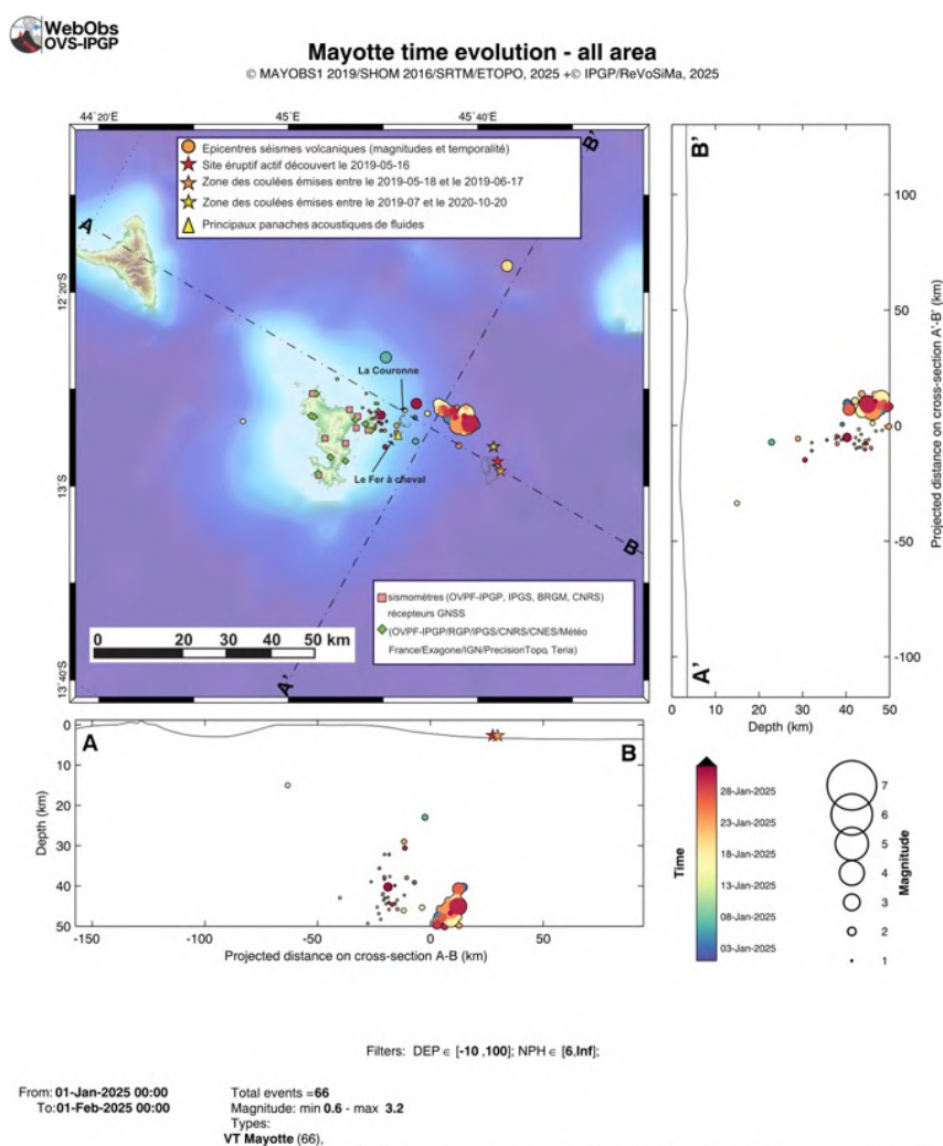
Figure 2 : Carte des épicentres ( \pm 5 km) des séismes volcano-tectoniques (VT) localisés avec les réseaux sismiques à terre (IPGP-CNRS-BRGM-BCSF-RENASS, ITES) en janvier 2025 (échelle temporelle de couleur). Sont aussi représentées les projections des hypocentres des séismes le long de coupes transverses et axiales le long de la ride montrant la localisation estimée en profondeur (la précision varie entre \pm 5 km et \pm 15 km) des séismes en fonction de la magnitude (taille des symboles) et de la date (échelle temporelle de couleur). La localisation approximative des panaches acoustiques identifiés pendant les campagnes océanographiques est indiquée par des triangles jaunes, l'étoile rouge indique le site éruptif identifié le 16 mai 2019, l'étoile orange la zone des coulées émises entre le 18/05/2019 et le 17/06/2019 et l'étoile jaune la zone des coulées émises entre juillet 2019 et le 04/12/2020. Les structures volcaniques de la zone dite de « La Couronne », du « Fer à Cheval » sont indiquées en grisé tout comme les coulées de lave de Fani Maoré. Les stations sismiques du réseau terrestre et les stations de positionnement par satellite GPS sont indiquées par des symboles (voir légende). (©OVPF-IPGP, BRGM, IFREMER, CNRS, BCSF-RENASS, ITES / REVOSIMA).
