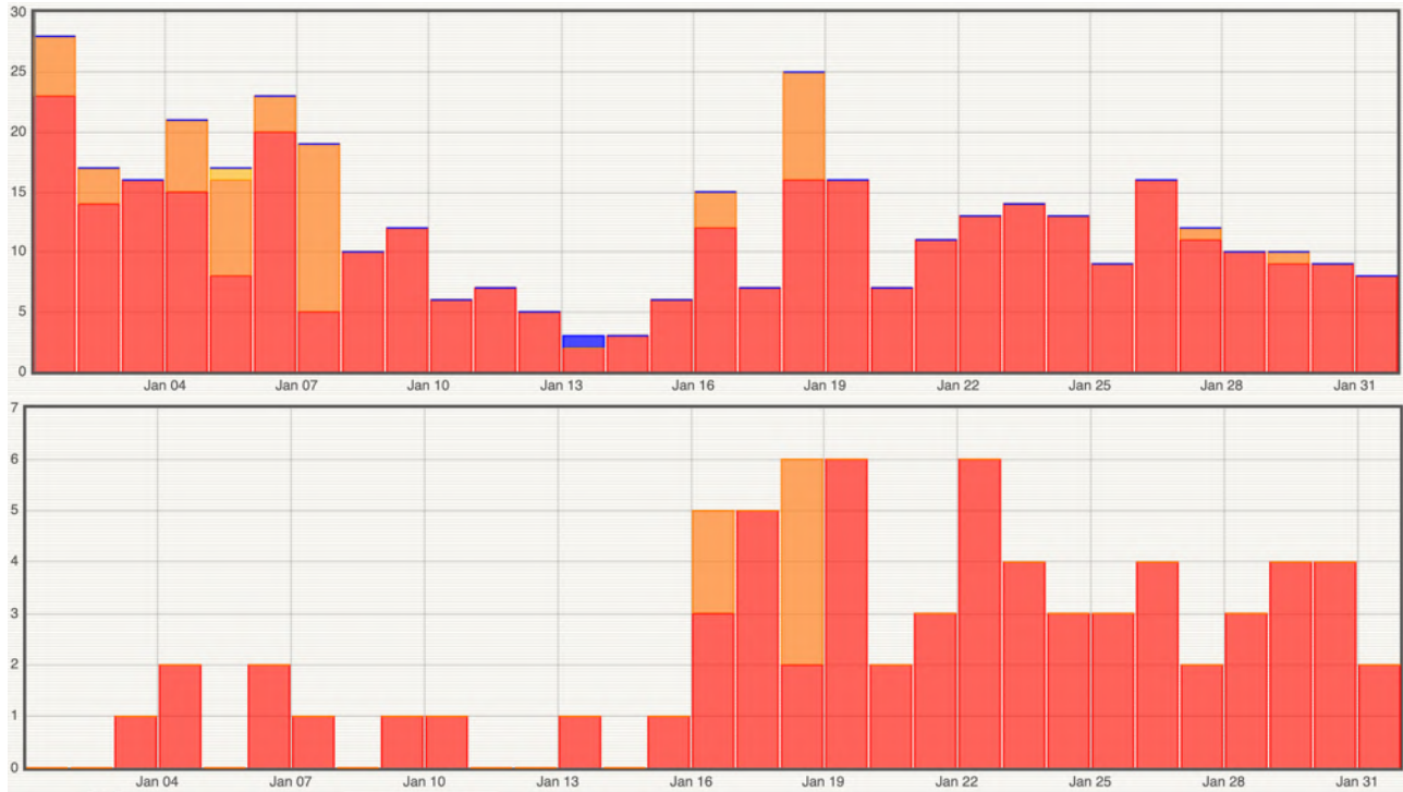
Figure 7 : Histogramme représentant le nombre de séismes par jour détectés (en haut) et localisés (en bas) en janvier 2025 par le réseau sismologique du REVOSIMA. En rouge les séismes volcano-tectoniques, en orange les séismes longues périodes, en jaune les séismes très longues périodes, en bleu les éboulements (© OVPF-IPGP et REVOSIMA). Suite au passage du cyclone Chido sur Mayotte le 14 décembre 2024 et à la perte de données de la majorité des stations sismologiques, il n'a pas été possible de localiser les séismes jusqu'au 3 janvier 2025. La localisation n'a pu reprendre de manière habituelle qu'à partir du 16 janvier.
