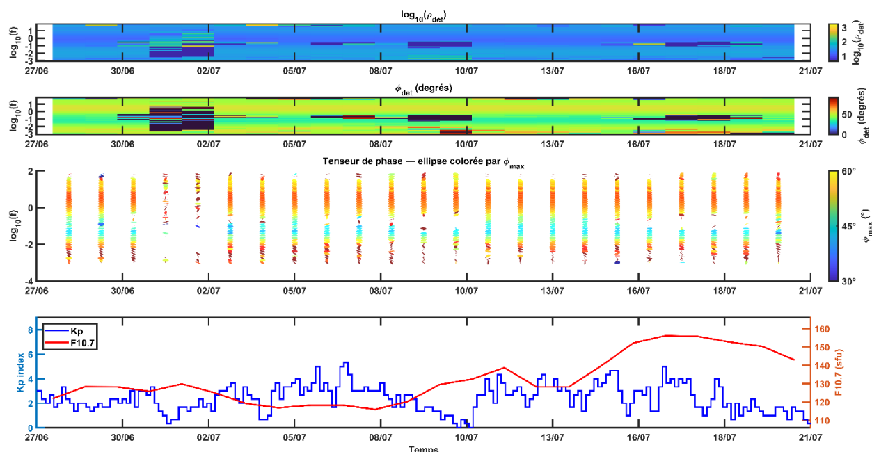
Figure 24 : Station Combani. Période du 27/06/2025 au 21/07/2025 – De haut en bas, chroniques temps-période de résistivité apparente de l’invariant 1D MT en échelle logarithmique, de phases, de tenseurs de phases journaliers et des index géomagnétiques Kp et F10.7 du réseau MT Revosima (©BRGM et REVOSIMA). Autour du 2 juillet, la présence d’activités anthropiques à côté de la station perturbe le signal.
