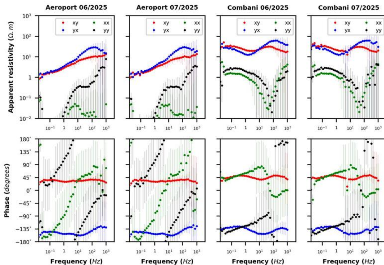
Figure 23 : Comparaison des sondages médians MT de juin 2025 et juillet 2025 pour Combani et Aéroport. Résistivités apparentes (en haut) et phases (en bas) en fonction de la période (secondes) de 64Hz à 1000s du réseau MT Revosima (©BRGM et REVOSIMA). On peut constater de légères différences de variations de résistivités apparentes et phases en fonction de la fréquence mais les tendances et magnitudes sont similaires pour les composantes majoritaires (xy et yx). Les données de juin 2025 sont de meilleure qualité que celles de juillet 2025 en raison d'une forte activité géomagnétique. En l'état de nos connaissances, les variations entre les sondages de juin 2025 et juillet 2025 sont imputables aux variations de ratio signal sur bruit et non à des variations de la structure géoelectrique de Mayotte.
