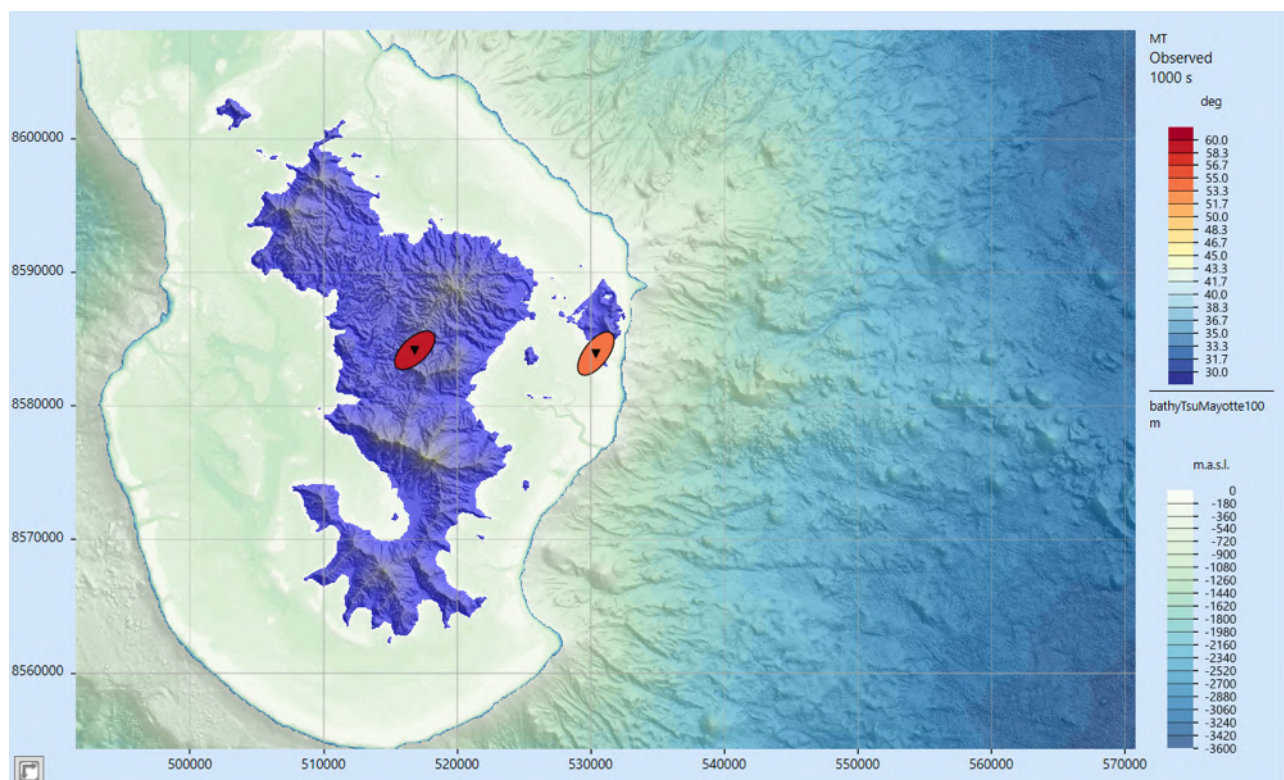
Figure 22 : Carte de tenseurs de phases calculés à 1000 secondes des 2 stations MT actives du Revosima pour le mois de juillet 2025 (©BRGM et REVOSIMA). Les ellipses de tenseurs de phases sont colorées avec les valeurs de phase maximum \varphi_{max} (en degrés) qui sont supérieures à 45^\circ , traduisant ainsi une décroissance de résistivité en profondeur.
