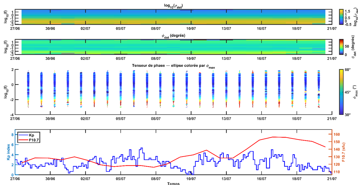
Figure 25 : Station Aéroport. Période du 27/06/2025 au 21/07/2025 – De haut en bas, chroniques temps-période de résistivité apparente de l’invariant 1D MT en échelle logarithmique, de phases, de tenseurs de phases journaliers et des index géomagnétiques Kp et F10.7 du réseau MT Revosima (©BRGM et REVOSIMA).
