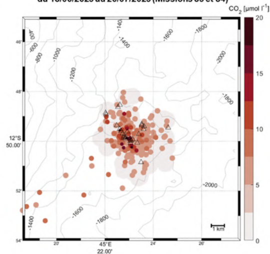
Figure 21 : Cartes centrées sur le Fer à Cheval représentant la distribution spatiale des maxima, pour chaque yo du planeur, des anomalies de concentration en \text{CO}_2 entre 800 et 1250 m de profondeur. A gauche, depuis le début de la surveillance par planeur du 17/09/2021 au 26/07/2025 ; à droite, pour la période du 18/06/2025 au 26/07/2025 (missions 83 et 84). Les valeurs des anomalies sont classées par couleur correspondant à des intervalles de concentrations et sont représentées par des cercles de taille décroissante avec l'intensité de la concentration. La bathymétrie est indiquée par des isobathes tous les 200 m. Les triangles gris correspondent à la position du barycentre des sites actifs d'émissions de fluides déjà répertoriés (Scalabrin, C. (2023), https://doi.org/10.12770/070818f6-6520-49e4-bafd-9d4d0609bf7d ).
