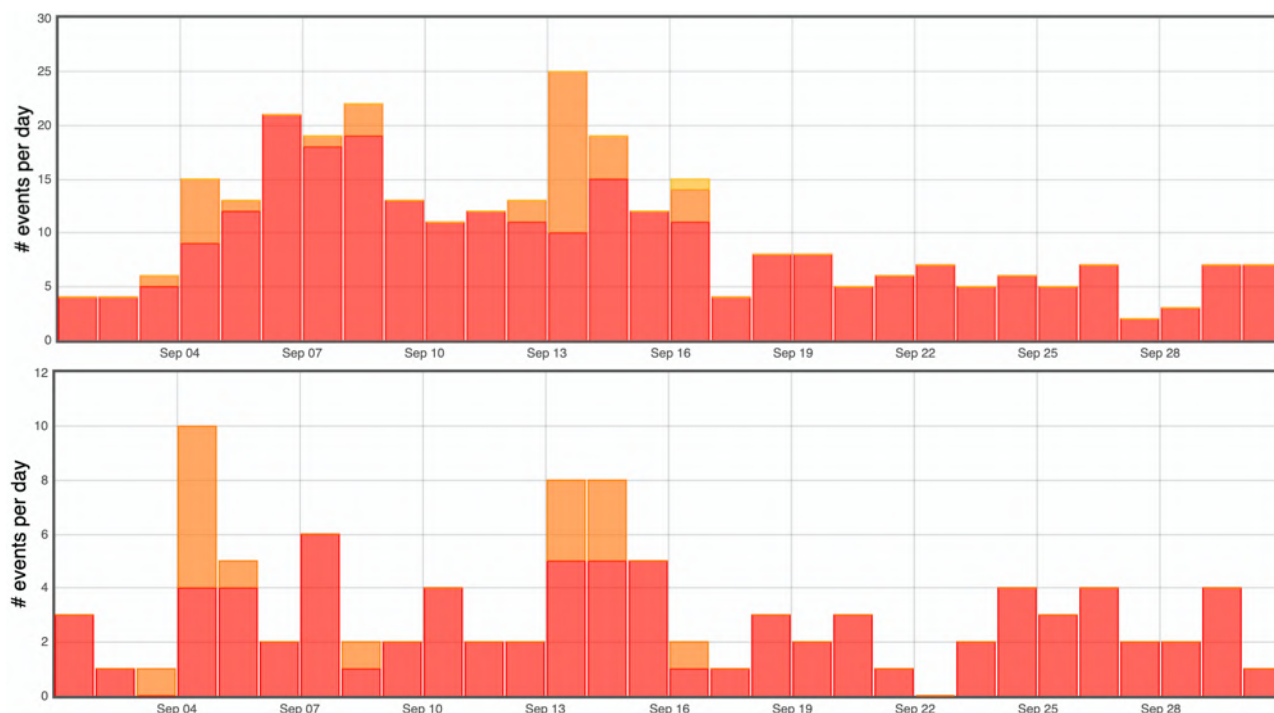
Figure 7 : Histogramme représentant le nombre de séismes par jour détectés (en haut) et localisés (en bas) en septembre 2025 par le réseau sismologique du REVOSIMA. En rouge les séismes volcano-tectoniques, en orange les séismes longues périodes, en jaune les séismes très longues périodes, en bleu les éboulements (© OVPF-IPGP et REVOSIMA).
