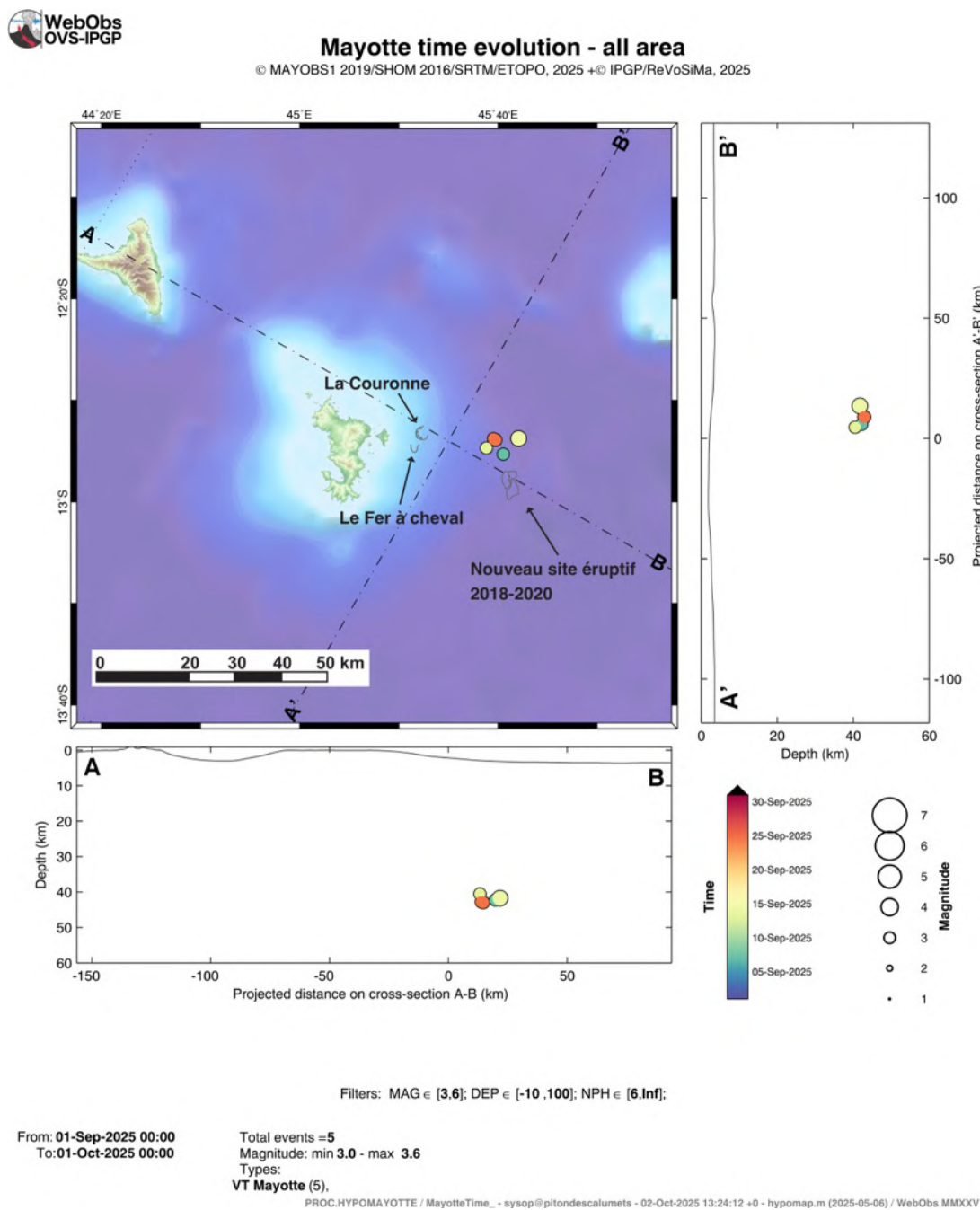
Figure 4 : Carte de localisation des épacentres ( \pm 5 km) des séismes de magnitude M \geq 3 en septembre 2025 enregistrés avec les réseaux sismiques à terre (IPGP-IFREMER-CNRS-BRGM-BCSF-RENASS-ITES). Sont aussi représentées les projections des hypocentres des séismes le long de coupes transverses et axiales le long de la ride montrant la localisation estimée en profondeur (la précision varie entre \pm 5 km et \pm 15 km) des séismes en fonction de la magnitude (taille des symboles) et de la date (échelle temporelle de couleur). La localisation approximative des panaches acoustiques identifiés pendant les campagnes océanographiques est indiquée par des triangles jaunes, l'étoile rouge indique le site éruptif identifié le 16 mai 2019, l'étoile orange la zone des coulées émises entre le 18/05/2019 et le 17/06/2019 et l'étoile jaune la zone des coulées émises entre juillet 2019 et le 04/12/2020. Les structures volcaniques de la zone dites de « La Couronne » et du « Fer à Cheval » sont indiquées en grisé tout comme les coulées de lave de Fani Maoré (©OVPF-IPGP, BRGM, IFREMER, CNRS, BCSF-RENASS, ITES / REVOSIMA).
