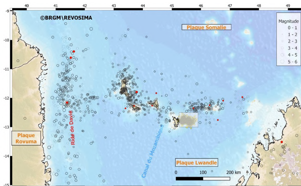
Figure 1: Sismicité régionale enregistrée depuis 2018 (modifié d'après Bertil et al. , 2021). Les séismes de septembre 2025 sont représentés en rouge. Le fond de carte est construit à partir des données topographiques et bathymétriques de Gebco 2022 ( www.gebco.net ). Le trait de côte et les frontières administratives sont extraits de https://gadm.org/ . Le carré blanc encadre les essaims sismiques surveillés depuis 2018. Se référer aux Figures 2 et 3 de ce bulletin pour la distribution de cette sismicité.
