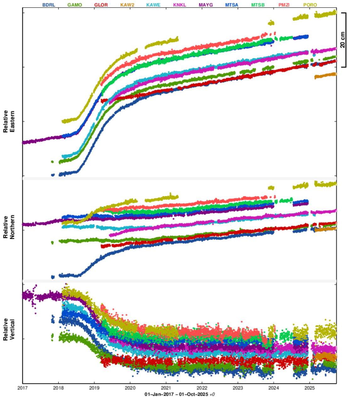
Figure 9 : Déplacements (en cm) enregistrés sur les stations GPS localisées à Mayotte (BDRL, GAMO, KAW, remplacée en 2025 par KAW2, KNKL, MAYG, MTSA, MTSB, PMZI, PORO) et la station GLOR localisée à Grande Glorieuse sur les composantes est (en haut), nord (au milieu) et vertical (en bas) entre le 1 er janvier 2017 et 30 septembre 2025 pour visualiser une longue série temporelle ante crise. Post-traitement de ces données réalisé par l'IPGP (©OVPF-IPGP / REVOSIMA). Suite au passage du cyclone Chido sur Mayotte le 14 décembre 2024, deux stations (MAYG et MTSA) ont été détruites. En février 2025, une maintenance de la monumentation ainsi qu'un changement d'antenne à la station KAW ont conduit à la création d'une nouvelle station, KAW2 en remplacement de KAW.
