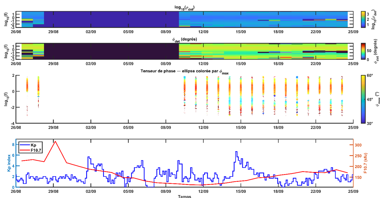
Figure 24 : Station Combani. Période du 26/08/2025 au 24/09/2025 – De haut en bas, chroniques temps-période de résistivité apparente de l'invariant 1D MT en échelle logarithmique, de phases, de tenseurs de phases journaliers et des index géomagnétiques Kp et F10.7 du réseau MT Revosima (©BRGM et REVOSIMA).
