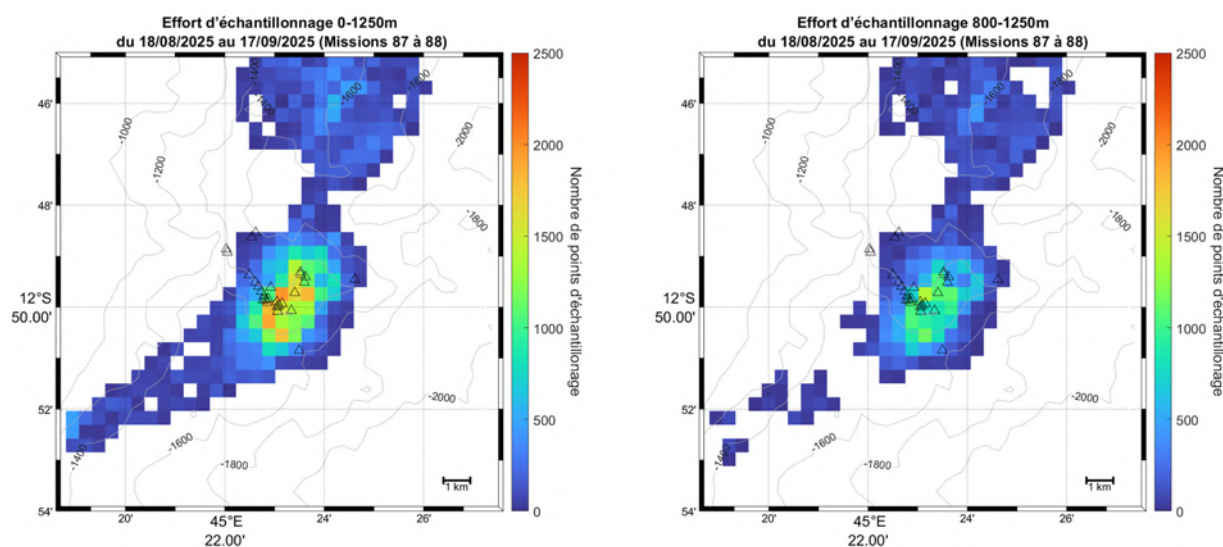
Figure 18 : Cartes centrées sur le Fer à Cheval représentant l'effort d'échantillonnage du planeur pour la période du 18/08/2025 au 17/09/2025 (missions 87 et 88) entre 0 et 1250 m de profondeur (à gauche), et entre 800 et 1250 m de profondeur (à droite). Le maillage est illustré par des cellules carrées mesurant 500 m de côté (0,25 km 2 ). La couleur représente le nombre de points d'échantillonnage réalisés dans chaque cellule. La bathymétrie est indiquée par des isobathes tous les 200 m. Les triangles noirs correspondent à la position du barycentre des sites actifs d'émissions de fluides déjà répertoriés (Scalabrin, C. (2023), https://doi.org/10.12770/070818f6-6520-49e4-bafd-9d4d0609bf7d ).
