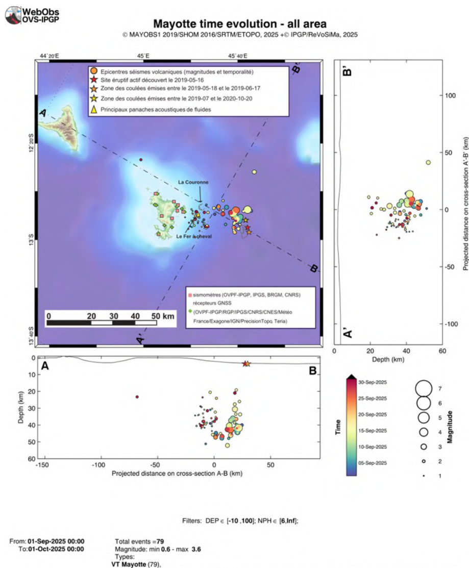
Figure 2 : Carte des épicentres ( \pm 5 km) des séismes volcano-tectoniques (VT) localisés avec les réseaux sismiques à terre (IPGP-CNRS-BRGM-BCSF-RENASS-ITES) en septembre 2025 (échelle temporelle de couleur). Sont aussi représentées les projections des hypocentres des séismes le long de coupes transverses et axiales le long de la ride montrant la localisation estimée en profondeur (la précision varie entre \pm 5 km et \pm 15 km) des séismes en fonction de la magnitude (taille des symboles) et de la date (échelle temporelle de couleur). La localisation approximative des panaches acoustiques identifiés pendant les campagnes océanographiques est indiquée par des triangles jaunes, l'étoile rouge indique le site éruptif identifié le 16 mai 2019, l'étoile orange la zone des coulées émises entre le 18/05/2019 et le 17/06/2019 et l'étoile jaune la zone des coulées émises entre juillet 2019 et le 04/12/2020. Les structures volcaniques de la zone dites de « La Couronne » et du « Fer à Cheval » sont indiquées en grisé tout comme les coulées de lave de Fani Maoré. Les stations sismiques du réseau terrestre et les stations de positionnement par satellite GPS sont indiquées par des symboles (voir légende) (©OVFP-IPGP, BRGM, IFREMER, CNRS, BCSF-RENASS, ITES / REVOSIMA).
