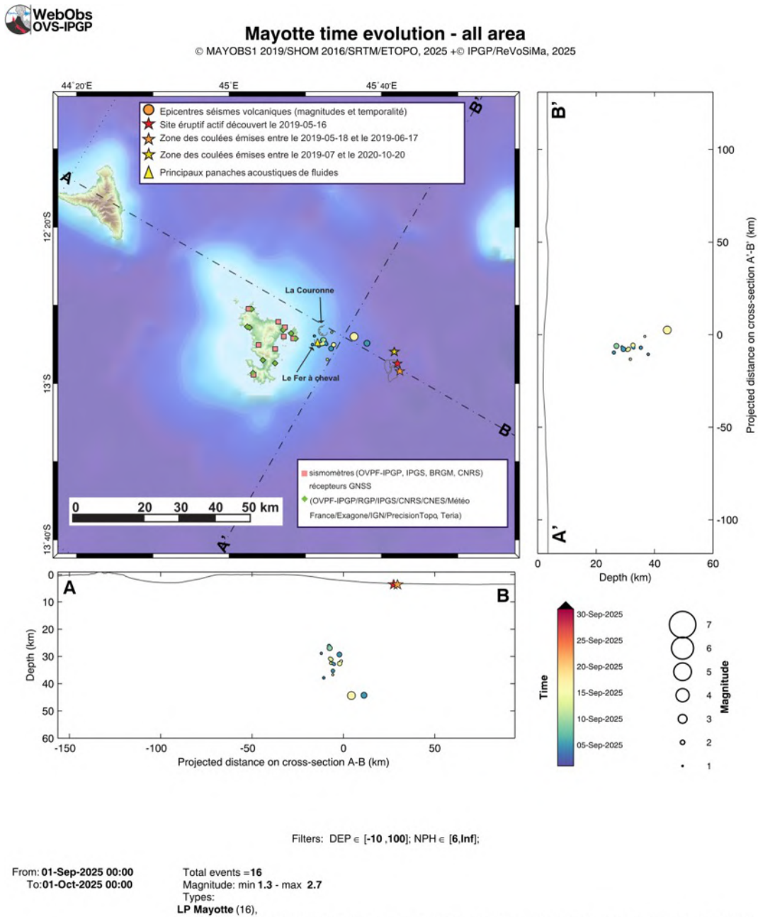
Figure 3 : Carte des épicentres ( \pm 5 km) des séismes longue période (LP) localisés avec les réseaux sismiques à terre (IPGP-CNRS-BRGM-BCSF-RENASS-ITES) en septembre 2025 (échelle temporelle de couleur). Sont aussi représentées les projections des hypocentres des séismes le long de coupes transverses et axiales le long de la ride montrant la localisation estimée en profondeur (la précision varie entre \pm 5 km et \pm 15 km) des séismes en fonction de la magnitude (taille des symboles) et de la date (échelle temporelle de couleur). La localisation approximative des panaches acoustiques identifiés pendant les campagnes océanographiques est indiquée par des triangles jaunes, l'étoile rouge indique le site éruptif identifié le 16 mai 2019, l'étoile orange la zone des coulées émises entre le 18/05/2019 et le 17/06/2019 et l'étoile jaune la zone des coulées émises entre juillet 2019 et le 04/12/2020. Les structures volcaniques de la zone dites de « La Couronne » et du « Fer à Cheval » sont indiquées en grisé tout comme les coulées de lave de Fani Maoré. Les stations sismiques du réseau terrestre et les stations de positionnement par satellite GPS sont indiquées par des symboles (voir légende) (©OVPF-IPGP, BRGM, IFREMER, CNRS, BCSF-RENASS, ITES / REVOSIMA).
