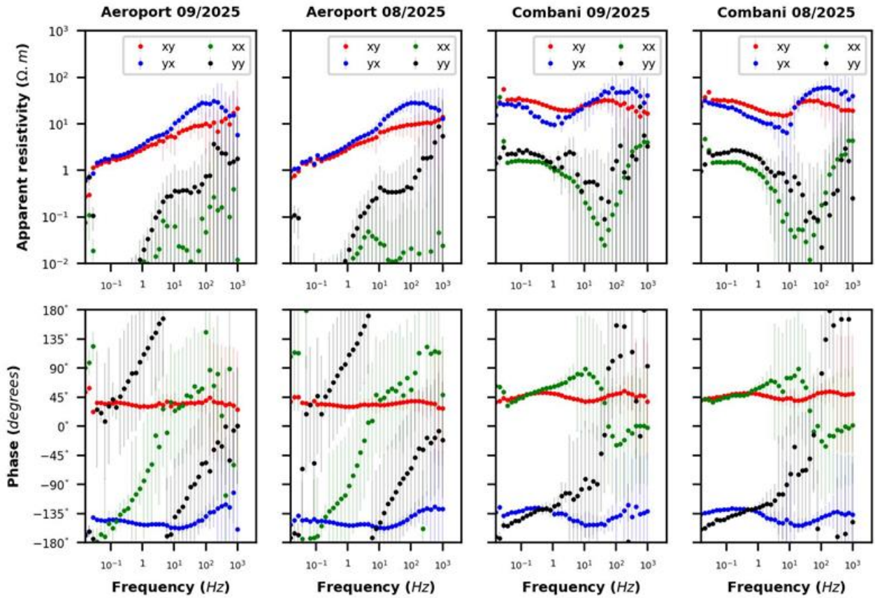
Figure 23 : Comparaison des sondages médians MT d'août 2025 et septembre 2025 pour Combani et Aéroport. Résistivités apparentes (en haut) et phases (en bas) en fonction de la période (secondes) de 64Hz à 1000s du réseau MT Revosima (©BRGM et REVOSIMA). On peut constater de légères différences de variations de résistivités apparentes et phases en fonction de la fréquence mais les tendances et magnitudes sont similaires pour les composantes majoritaires (xy et yx). Les données d'août 2025 sont de meilleure qualité que celles de septembre 2025 en raison d'une dégradation des électrodes marquées sur les données en septembre. Sur la station Combani, la présence d'une forte variabilité autour de la fréquence 1 Hz est liée aux variations de condition de bruits au niveau de la station. En l'état de nos connaissances, les variations entre les sondages d'août 2025 et septembre 2025 sont imputables aux variations de ratio signal sur bruit et non à des variations de la structure géoelectrique de Mayotte.
