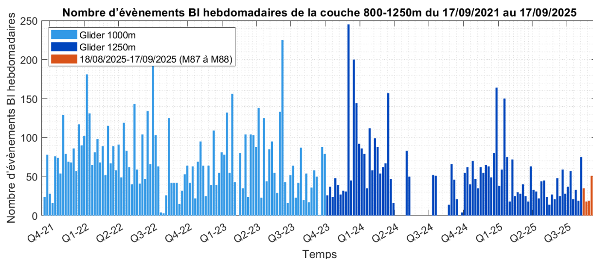
Figure 19 : Histogramme du nombre hebdomadaire de détections d'évènement BI (Backscatter Index) depuis le début de la surveillance par planeur (17/09/2021) et jusqu'au 17/09/2025 (fin de la mission 88). Résultats obtenus avec les planeurs limités à 1000 m d'immersion en bleu clair et à 1250 m d'immersion en bleu foncé. En orange, résultats pour la période entre le 18/08/2025 et le 17/09/2025 (Missions 87 et 88) avec le planeur limité à 1250 m d'immersion. L'échelle de temps est représentée par quartiles des années 2021 à 2025. Les périodes où le planeur n'a pas été utilisé sont symbolisées par un nombre d'évènements BI hebdomadaire égal à zéro.
