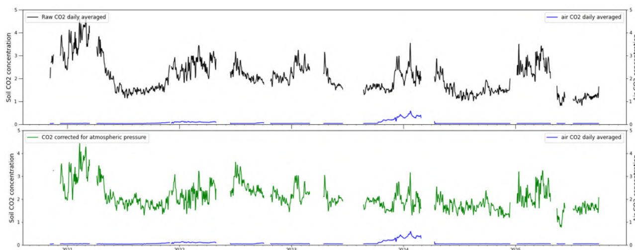
Figure 12 : Concentration en \text{CO}_2 dans le sol à la station permanente UDMN. Comparaison entre les données brutes (noir) et les données corrigées de l'influence de la pression atmosphérique (vert). Bleu : concentration du \text{CO}_2 dans l'air (1 m au-dessus du sol). Les variations de concentrations dans l'air sont liées à l'activité biogénique (©OVPF-IPGP / REVOSIMA).
