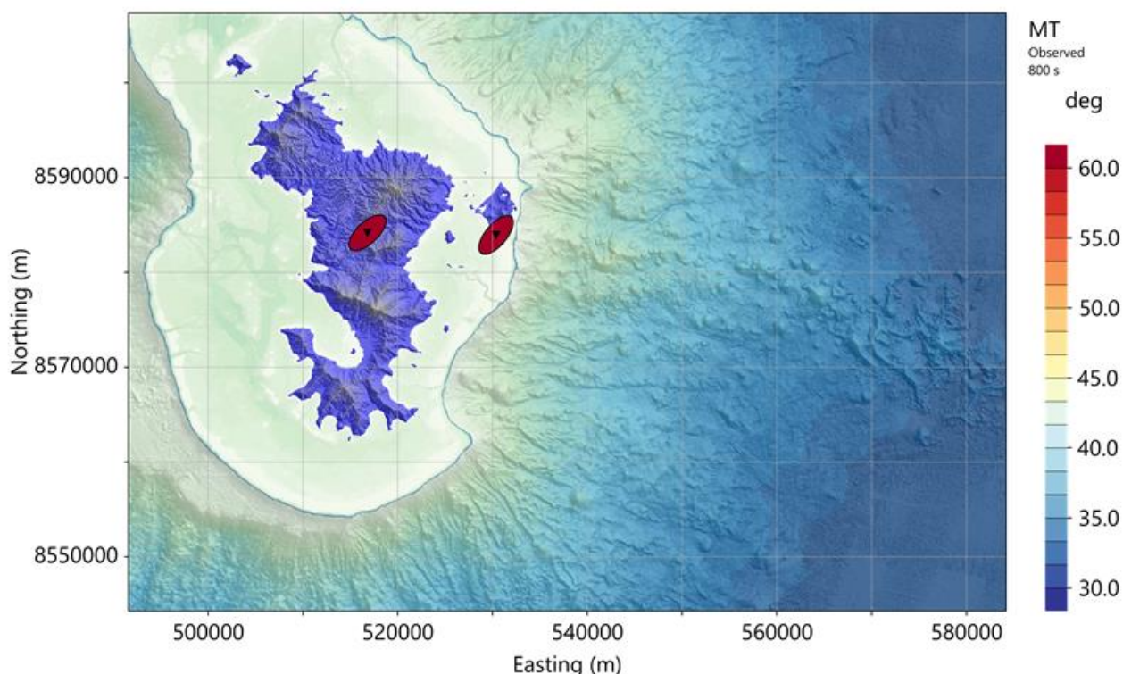
Figure 22 : Carte de tenseurs de phases calculés à 800 secondes des 2 stations MT actives du Revosima pour le mois de septembre 2025 (©BRGM et REVOSIMA). Les ellipses de tenseurs de phases sont colorées avec les valeurs de phase maximum \varphi_{\max} (en degrés) qui sont supérieures à 45^\circ , traduisant ainsi une décroissance de résistivité en profondeur.
