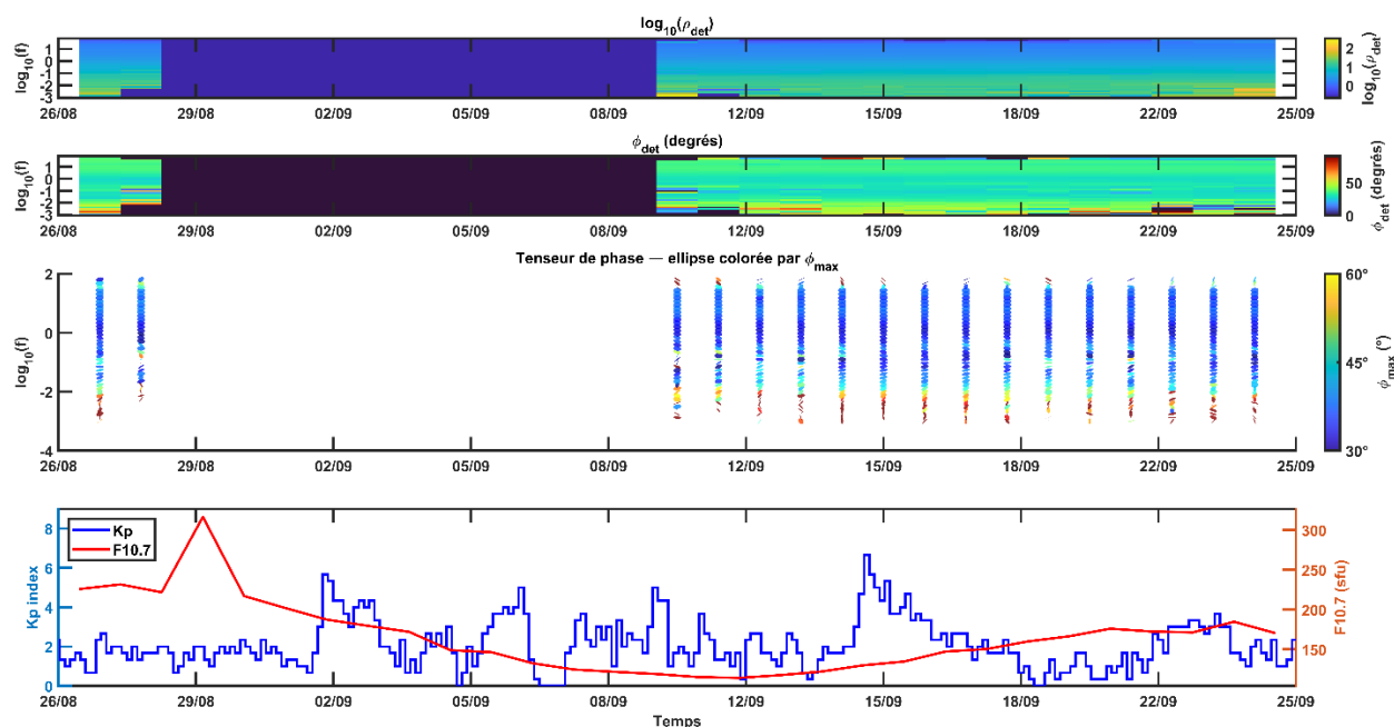
Figure 25 : Station Aéroport. Période du 26/08/2025 au 24/09/2025 – De haut en bas, chroniques temps-période de résistivité apparente de l'invariant 1D MT en échelle logarithmique, de phases, de tenseurs de phases journaliers et des index géomagnétiques Kp et F10.7 du réseau MT Revosima (©BRGM et REVOSIMA).
