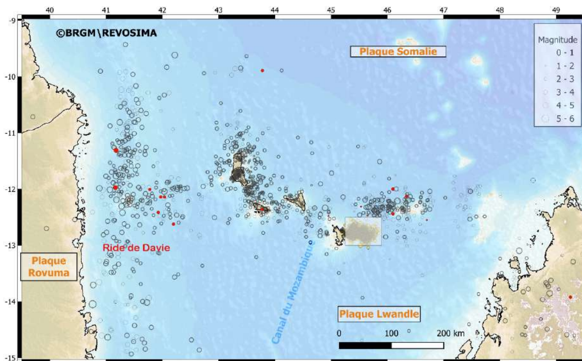
Figure 1: En rouge : séismes localisés au nord du Canal du Mozambique au mois de mai 2026. Les cercles gris représentent la sismicité localisée depuis 2018. Bathymétrie et topographie : Gebco 2022, GEBCO Compilation Group (2022) GEBCO_2022 Grid (doi:10.5285/e0f0bb80-ab44-2739-e053-6c86abc0289c). Le cadre blanc à l'est de Mayotte délimite l'emprise de la sismicité associée au phénomène tellurique surveillé par le REVOSIMA dont le descriptif est présent dans une autre section de ce bulletin.
