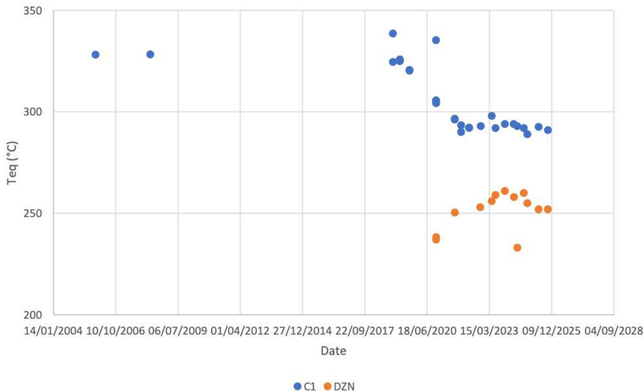
Figure 15 : Température d'équilibre des fluides au sein du système hydrothermal. La température d'équilibre entre le CO 2 et le CH 4 dans le système hydrothermal est estimée à l'aide de l'équation de Giggenbach 1992.
