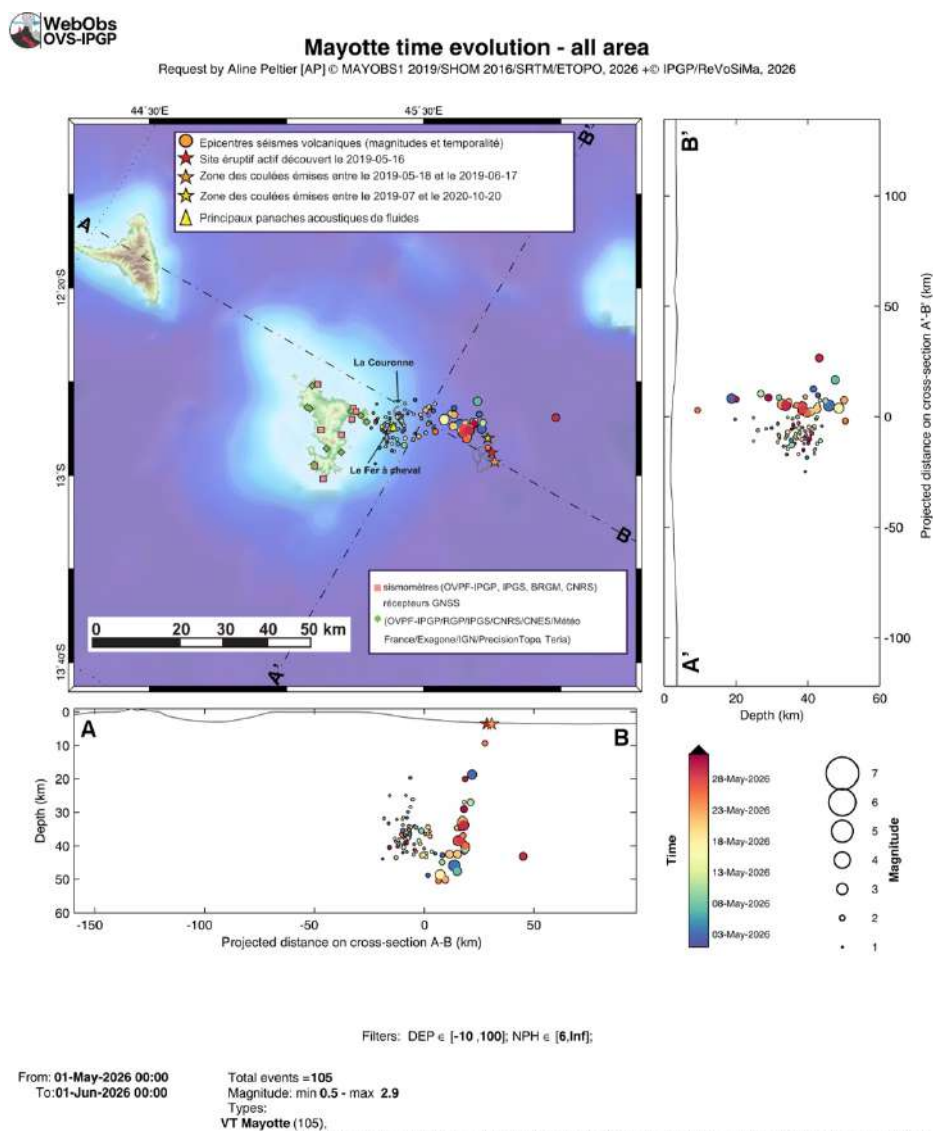
Figure 2 : Carte des épicentres ( \pm 5 km) des séismes volcano-tectoniques (VT) localisés avec les réseaux sismiques à terre (IPGP-CNRS-BRGM-BCSF-RENASS-ITES) en mai 2026 (échelle temporelle de couleur). Sont aussi représentées les projections des hypocentres des séismes le long de coupes transverses et axiales le long de la ride montrant la localisation estimée en profondeur (la précision varie entre \pm 5 km et \pm 15 km) des séismes en fonction de la magnitude (taille des symboles) et de la date (échelle temporelle de couleur). La localisation approximative des panaches acoustiques identifiés pendant les campagnes océanographiques est indiquée par des triangles jaunes, l'étoile rouge indique le site éruptif identifié le 16 mai 2019, l'étoile orange la zone des coulées émises entre le 18/05/2019 et le 17/06/2019 et l'étoile jaune la zone des coulées émises entre juillet 2019 et le 04/12/2020. Les structures volcaniques de la zone dites de « La Couronne » et du « Fer à Cheval » sont indiquées en grisé tout comme les coulées de lave de Fani Maoré. Les stations sismiques du réseau terrestre et les stations de positionnement par satellite GNSS sont indiquées par des symboles (voir légende) ©OVPP-IPGP, BRGM, IFREMER, CNRS, BCSF-RENASS, ITES / REVOSIMA).
