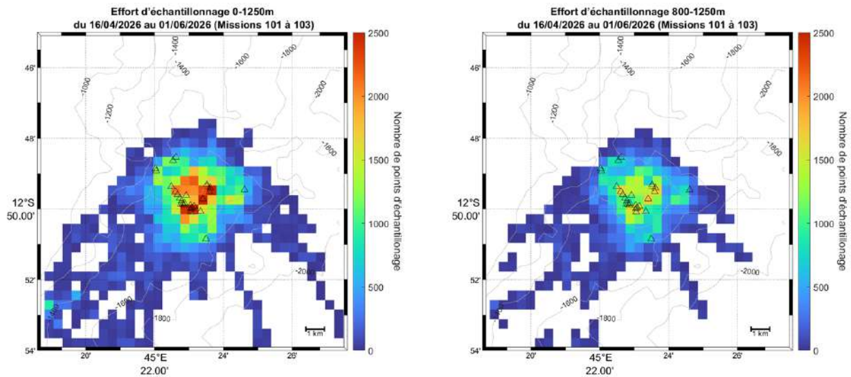
Figure 18 : Cartes centrées sur le Fer à Cheval représentant l'effort d'échantillonnage du planeur pour la période du 16/04/2026 au 01/06/2026 (missions 101, 102 et 103) entre 0 et 1250 m de profondeur (à gauche), et entre 800 et 1250 m de profondeur (à droite). Le maillage est illustré par des cellules carrées mesurant 500 m de côté (0,25 km 2 ). La couleur représente le nombre de points d'échantillonnage réalisés dans chaque cellule. La bathymétrie est indiquée par des isobathes tous les 200 m. Les triangles noirs correspondent à la position du barycentre des sites actifs d'émissions de fluides déjà répertoriés (Scalabrin, C. (2023), https://doi.org/10.12770/070818f6-6520-49e4-bafd-9d4d0609bf7d ).
