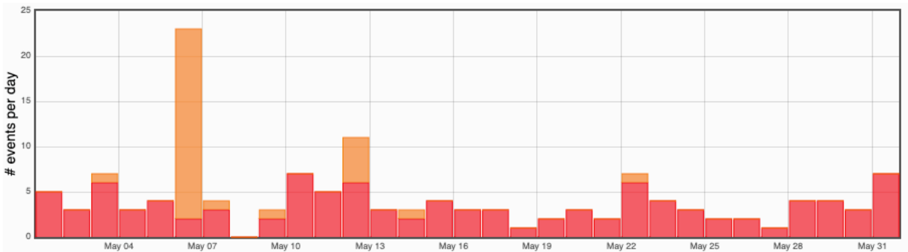
Figure 7 : Histogramme représentant le nombre de séismes par jour localisés en mai 2026 par le réseau sismologique du REVOSIMA. En rouge les séismes volcano-tectoniques, en orange les séismes longues périodes, en jaune les séismes très longues périodes, en bleu les éboulements (©WebObs/ OVPF-IPGP/REVOSIMA).
