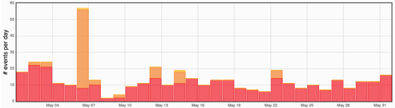
Figure 6 : Histogramme représentant le nombre de séismes par jour détectés en mai 2026 par le réseau sismologique du REVOSIMA. En rouge les séismes volcano-tectoniques, en orange les séismes longues périodes, en jaune les séismes très longues périodes, en bleu les éboulements (©WebObs/ OVPF-IPGP/REVOSIMA).
