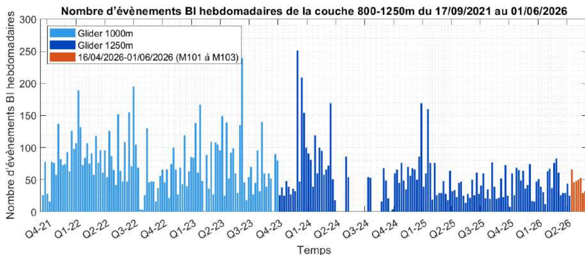
Figure 19 : Histogramme du nombre hebdomadaire de détections d'évènement BI (Backscatter Index) depuis le début de la surveillance par planeur (17/09/2021) et jusqu'au 01/06/2026 (fin de la mission 103). Résultats obtenus avec les planeurs limités à 1000 m d'immersion en bleu clair et à 1250 m d'immersion en bleu foncé. En orange, résultats pour la période entre le 16/04/2026 et le 01/06/2026 (Missions 101, 102 et 103) avec le planeur limité à 1250 m d'immersion. L'échelle de temps est représentée par quartiles des années 2021 à 2026. Les périodes où le planeur n'a pas été utilisé sont symbolisées par un nombre d'évènements BI hebdomadaire égal à zéro.
