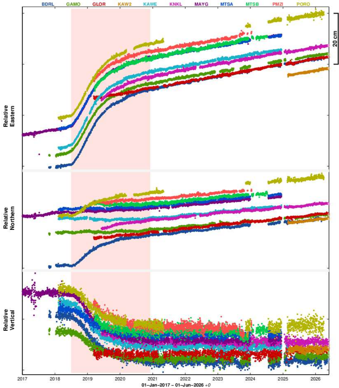
Figure 9 : Déplacements (en cm) enregistrés sur les stations GNSS localisées à Mayotte (BDRL, GAMO, KAWL remplacée en 2025 par KAW2, KNKL, MAYG, MTSB, PMZI, PORO) et la station GLOL localisée à Grande Glorieuse sur les composantes est (en haut), nord (au milieu) et vertical (en bas) entre le 1 er janvier 2017 et 31 mai 2026 pour visualiser une longue série temporelle ante crise. Post-traitement de ces données réalisé par l'IPGP. La durée de l'éruption du Fani Maoré est indiquée en rouge (©Webobs/OVPF-IPGP/REVOSIMA). Suite au passage du cyclone Chido sur Mayotte le 14 décembre 2024, deux stations (MAYG et MTSB) ont été détruites. En février 2025, une maintenance de la monumentation ainsi qu'un changement d'antenne à la station KAWL ont conduit à la création d'une nouvelle station, KAW2 en remplacement de KAWL.
