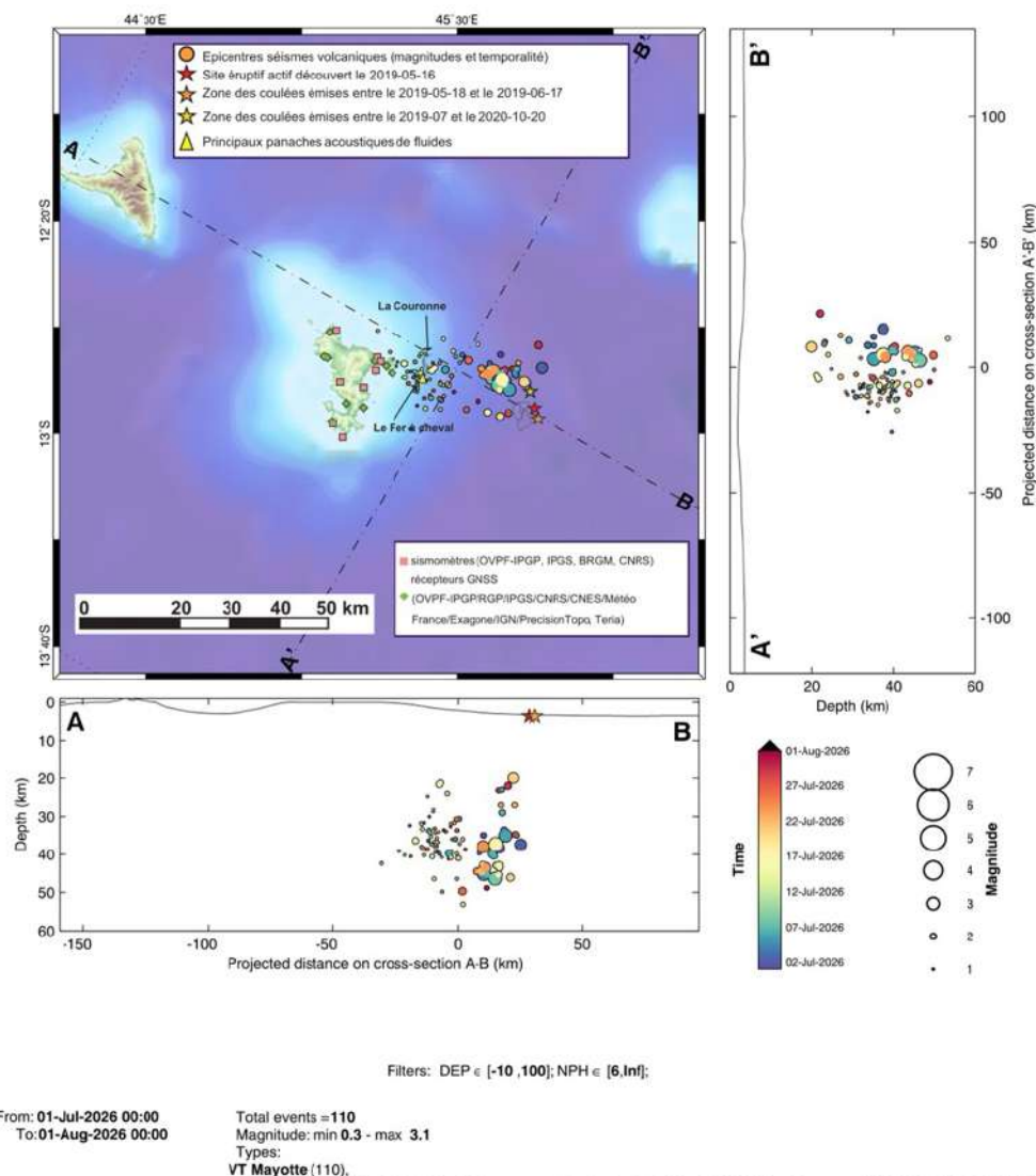
Figure 2 : Carte des épicentres ( \pm 5 km) des séismes volcano-tectoniques (VT) localisés avec les réseaux sismiques à terre (IPGP-CNRS-BRGM-BCSF-RENASS-ITES) en juillet 2026 (échelle temporelle de couleur). Sont aussi représentées les projections des hypocentres des séismes le long de coupes transverses et axiales le long de la ride montrant la localisation estimée en profondeur (la précision varie entre \pm 5 km et \pm 15 km) des séismes en fonction de la magnitude (taille des symboles) et de la date (échelle temporelle de couleur). La localisation approximative des panaches acoustiques identifiés pendant les campagnes océanographiques est indiquée par des triangles jaunes, l'étoile rouge indique le site éruptif identifié le 16 mai 2019, l'étoile orange la zone des coulées émises entre le 18/05/2019 et le 17/06/2019 et l'étoile jaune la zone des coulées émises entre juillet 2019 et le 04/12/2020. Les structures volcaniques de la zone dites de « La Couronne » et du « Fer à Cheval » sont indiquées en grisé tout comme les coulées de lave de Fani Maoré. Les stations sismiques du réseau terrestre et les stations de positionnement par satellite GNSS sont indiquées par des symboles (voir légende) (©OVPF-IPGP, BRGM, IFREMER, CNRS, BCSF-RENASS, ITES / REVOSIMA).
