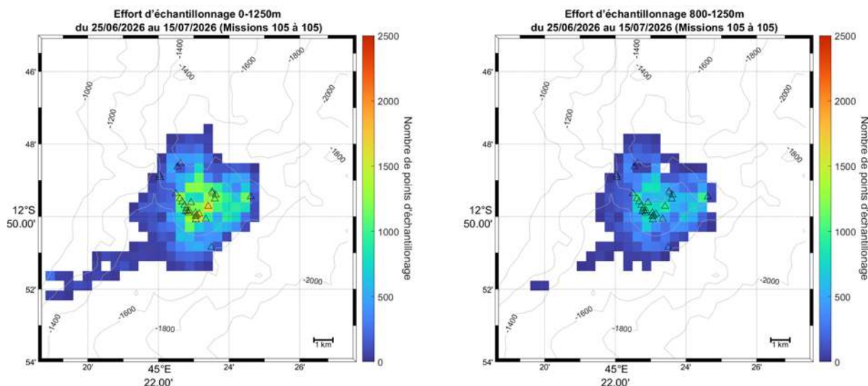
Figure 18 : Cartes centrées sur le Fer à Cheval représentant l'effort d'échantillonnage du planeur pour la période du 25/06/2026 au 15/07/2026 (mission 105) entre 0 et 1250 m de profondeur (à gauche), et entre 800 et 1250 m de profondeur (à droite). Le maillage est illustré par des cellules carrées mesurant 500 m de côté (0,25 km 2 ). La couleur représente le nombre de points d'échantillonnage réalisés dans chaque cellule. La bathymétrie est indiquée par des isobathes tous les 200 m. Les triangles noirs correspondent à la position du barycentre des sites actifs d'émissions de fluides déjà répertoriés (Scalabrin, C. (2023), https://doi.org/10.12770/070818f6-6520-49e4-bafd-9d4d0609bf7d ).
