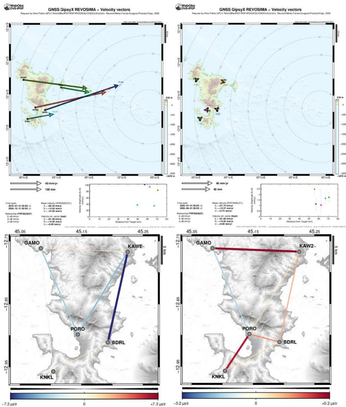
Figure 8 : Illustration de la déformation En haut : Déplacements du sol enregistrés sur les stations GNSS de Mayotte entre le 1 er juillet 2018 et fin 2020 (à gauche) et sur les derniers douze mois (à droite). Les déplacements horizontaux sont représentés sous forme vectorielle et les déplacements verticaux sont indiqués par les valeurs chiffrées en couleur. Les données sont corrigées du mouvement de la plaque. En bas : Cartes de contraintes linéaires 3D (en microstrain) entre le 1 er juillet 2018 et fin 2020 (à gauche) et sur les derniers douze mois (à droite). L'épaisseur et la couleur des lignes de base indiquent l'intensité de la contrainte soit en compression (bleu), soit en extension (rouge). Les échelles sont différentes pour les deux cartes de contraintes. Post-traitement de ces données réalisé par l'IPGP (©Webobs/OVPF-IPGP/REVOSIMA).
