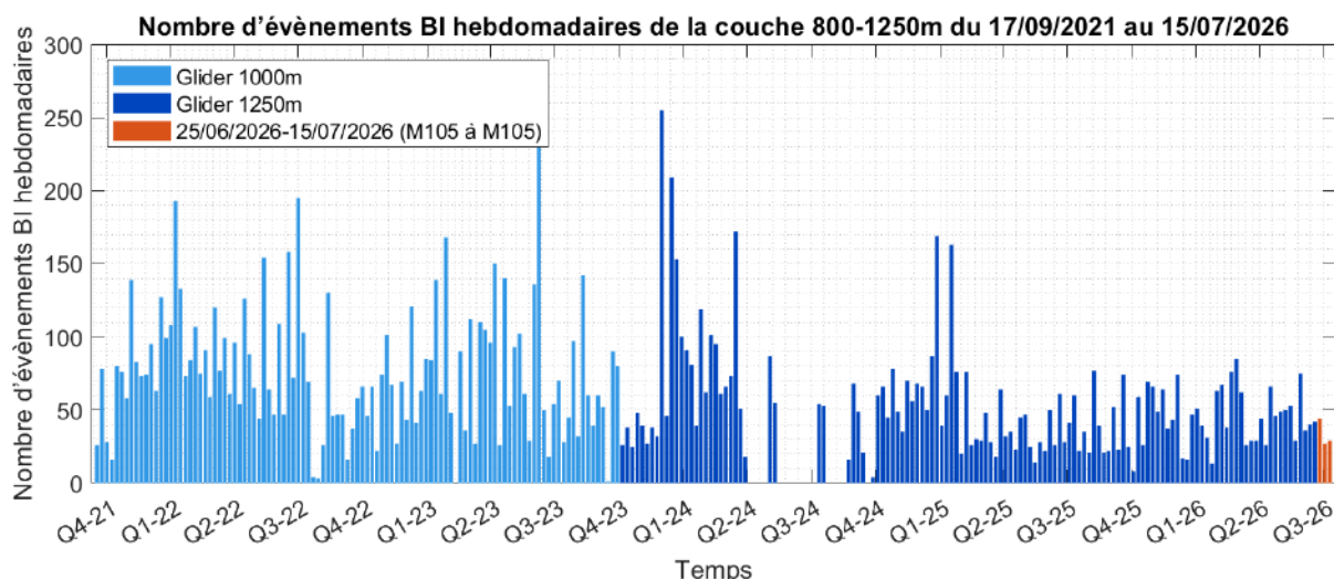
Figure 19 : Histogramme du nombre hebdomadaire de détections d'évènement BI (Backscatter Index) depuis le début de la surveillance par planeur (17/09/2021) et jusqu'au 15/07/2026 (fin de la mission 105). Résultats obtenus avec les planeurs limités à 1000 m d'immersion en bleu clair et à 1250 m d'immersion en bleu foncé. En orange, résultats pour la période entre le 25/06/2026 et le 15/07/2026 (Mission 105) avec le planeur limité à 1250 m d'immersion. L'échelle de temps est représentée par quartiles des années 2021 à 2026. Les périodes où le planeur n'a pas été utilisé sont symbolisées par un nombre d'évènements BI hebdomadaire égal à zéro.
