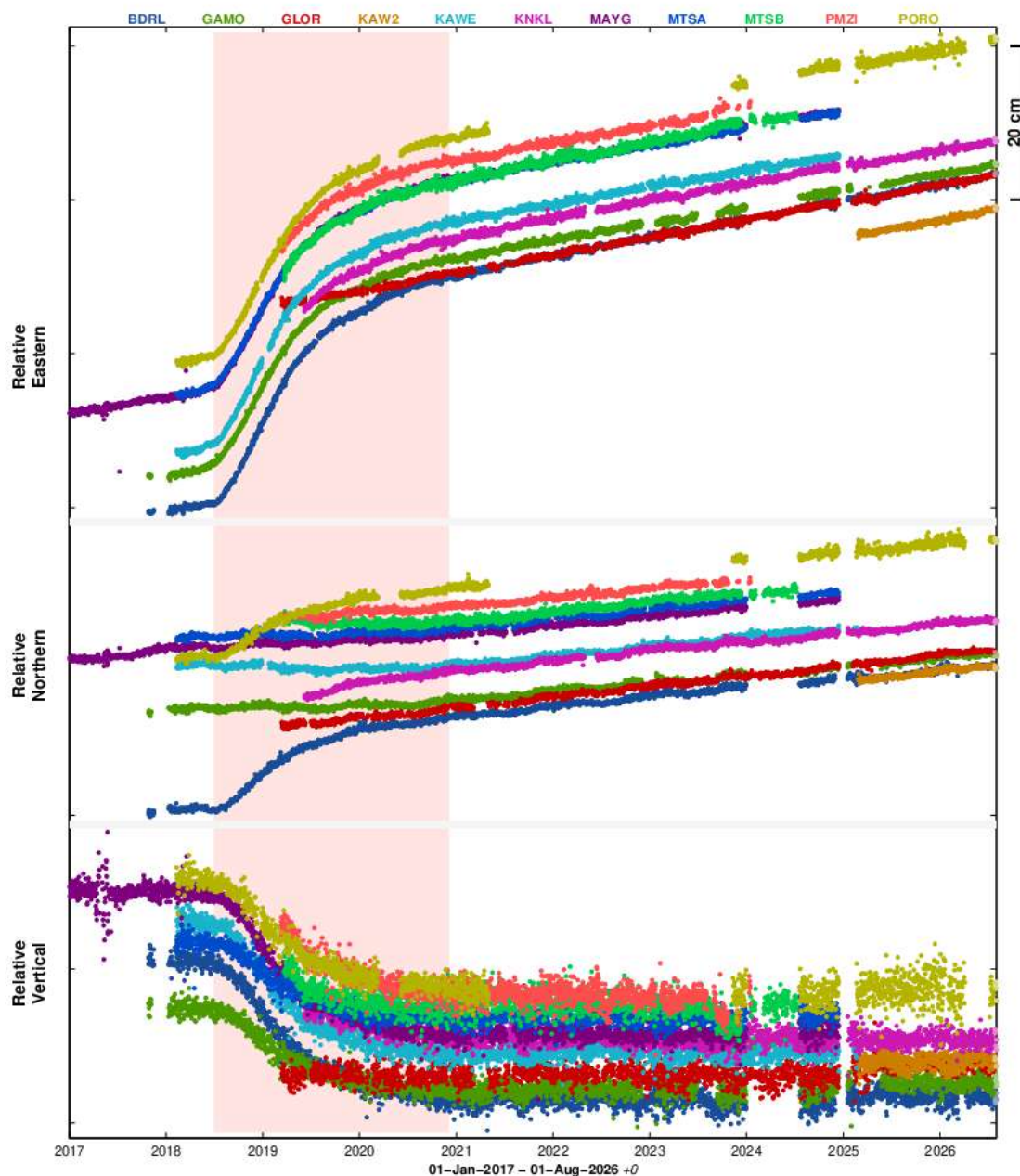
Figure 9 : Déplacements (en cm) enregistrés sur les stations GNSS localisées à Mayotte (BDRL, GAMO, KAW2 remplacée en 2025 par KAW2, KNKL, MAYG, MTSA, MTSB, PMZI, PORO) et la station GLOR localisée à Grande Glorieuse sur les composantes est (en haut), nord (au milieu) et vertical (en bas) entre le 1 er janvier 2017 et 31 juillet 2026 pour visualiser une longue série temporelle ante crise. Post-traitement de ces données réalisé par l'IPGP. La durée de l'éruption du Fani Maoré est indiquée en rouge (©WebObs/OVPF-IPGP/REVOSIMA). Suite au passage du cyclone Chido sur Mayotte le 14 décembre 2024, deux stations (MAYG et MTSA) ont été détruites. En février 2025, une maintenance de la monumentation ainsi qu'un changement d'antenne à la station KAW2 ont conduit à la création d'une nouvelle station, KAW2 en remplacement de KAW2.
