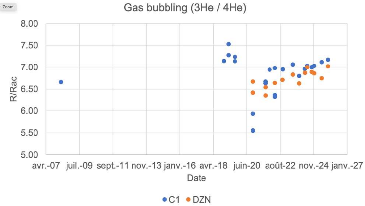
Figure 14 : Analyses isotopiques (gaz rares) des bullages aux points de contrôle C1 (estran de l'aéroport) et DZN (Lac Dziani). Une augmentation du R/Rac (rapport isotopique de l'He normalisé à celui de l'atmosphère) est liée à une augmentation de la contribution des fluides profonds remontant du manteau. Erreur moyenne sur chaque analyse : 0.05 unité.
