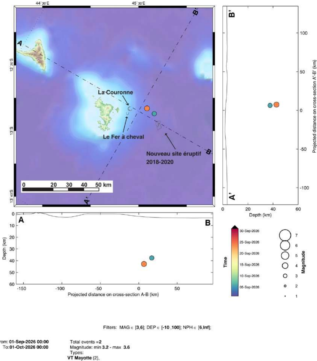
Figure 4 : Carte de localisation des épicentres ( \pm 5 km) des séismes de magnitude M \geq 3 en septembre 2026 enregistrés avec les réseaux sismiques à terre (IPGP-IFREMER-CNRS-BRGM-BCSF-RENASS-ITES). Sont aussi représentées les projections des hypocentres des séismes le long de coupes transverses et axiales le long de la ride montrant la localisation estimée en profondeur (la précision varie entre \pm 5 km et \pm 15 km) des séismes en fonction de la magnitude (taille des symboles) et de la date (échelle temporelle de couleur). La localisation approximative des panaches acoustiques identifiés pendant les campagnes océanographiques est indiquée par des triangles jaunes, l'étoile rouge indique le site éruptif identifié le 16 mai 2019, l'étoile orange la zone des coulées émises entre le 18/05/2019 et le 17/06/2019 et l'étoile jaune la zone des coulées émises entre juillet 2019 et le 04/12/2020. Les structures volcaniques de la zone dites de « La Couronne » et du « Fer à Cheval » sont indiquées en grisé tout comme les coulées de lave de Fani Maoré (©OVPF-IPGP, BRGM, IFREMER, CNRS, BCSF-RENASS, ITES / REVOSIMA).
