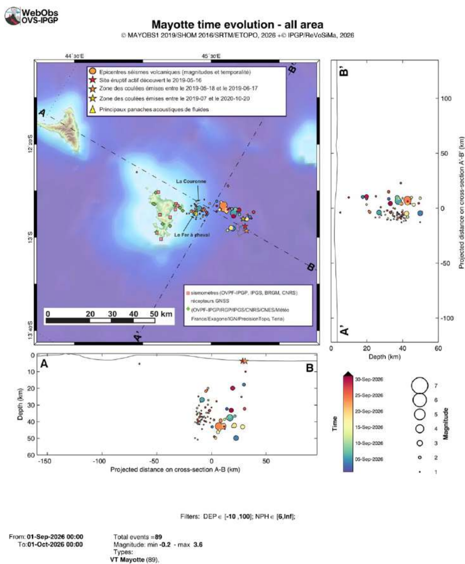
Figure 2 : Carte des épicentres ( \pm 5 km) des séismes volcano-tectoniques (VT) localisés avec les réseaux sismiques à terre (IPGP-CNRS-BRGM-BCSF-RENASS-ITES) en septembre 2026 (échelle temporelle de couleur). Sont aussi représentées les projections des hypocentres des séismes le long de coupes transverses et axiales le long de la ride montrant la localisation estimée en profondeur (la précision varie entre \pm 5 km et \pm 15 km) des séismes en fonction de la magnitude (taille des symboles) et de la date (échelle temporelle de couleur). La localisation approximative des panaches acoustiques identifiés pendant les campagnes océanographiques est indiquée par des triangles jaunes, l'étoile rouge indique le site éruptif identifié le 16 mai 2019, l'étoile orange la zone des coulées émises entre le 18/05/2019 et le 17/06/2019 et l'étoile jaune la zone des coulées émises entre juillet 2019 et le 04/12/2020. Les structures volcaniques de la zone dites de « La Couronne » et du « Fer à Cheval » sont indiquées en grisé tout comme les coulées de lave de Fani Maoré. Les stations sismiques du réseau terrestre et les stations de positionnement par satellite GNSS sont indiquées par des symboles (voir légende) (©OVPF-IPGP, BRGM, IFREMER, CNRS, BCSF-RENASS, ITES / REVOSIMA).
