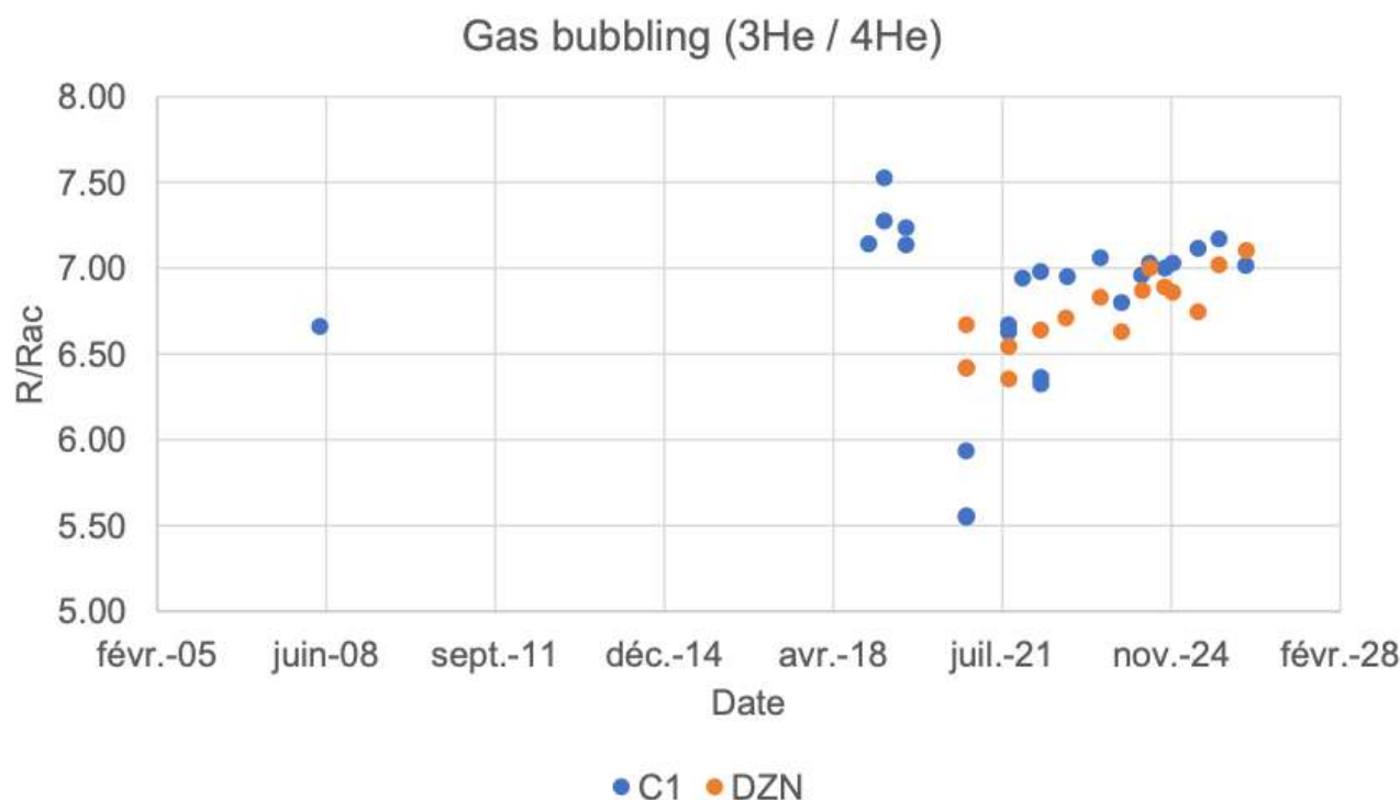
Figure 14 : Analyses isotopiques (gaz rares) des bullages aux points de contrôle C1 (estran de l'aéroport) et DZN (Lac Dziani). Une augmentation du R/R_{ac} (rapport isotopique de l'He normalisé à celui de l'atmosphère) est liée à une augmentation de la contribution des fluides profonds remontant du manteau. Après la fin de l'éruption du Fani Maoré, on observe une évolution de la composition des fluides dans le Dziani, qui convergent vers la composition de ceux de l'estran. Erreur moyenne sur chaque analyse : 0.05 unité.
