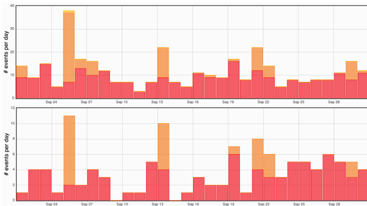
Figure 7 : Histogramme représentant le nombre de séismes par jour détectés (en haut) et localisés (en bas) en septembre 2026 par le réseau sismologique du REVOSIMA. En rouge les séismes volcano-tectoniques, en orange les séismes longues périodes, en jaune les séismes très longues périodes, en bleu les éboulements (© OVPF-IPGP et REVOSIMA).
