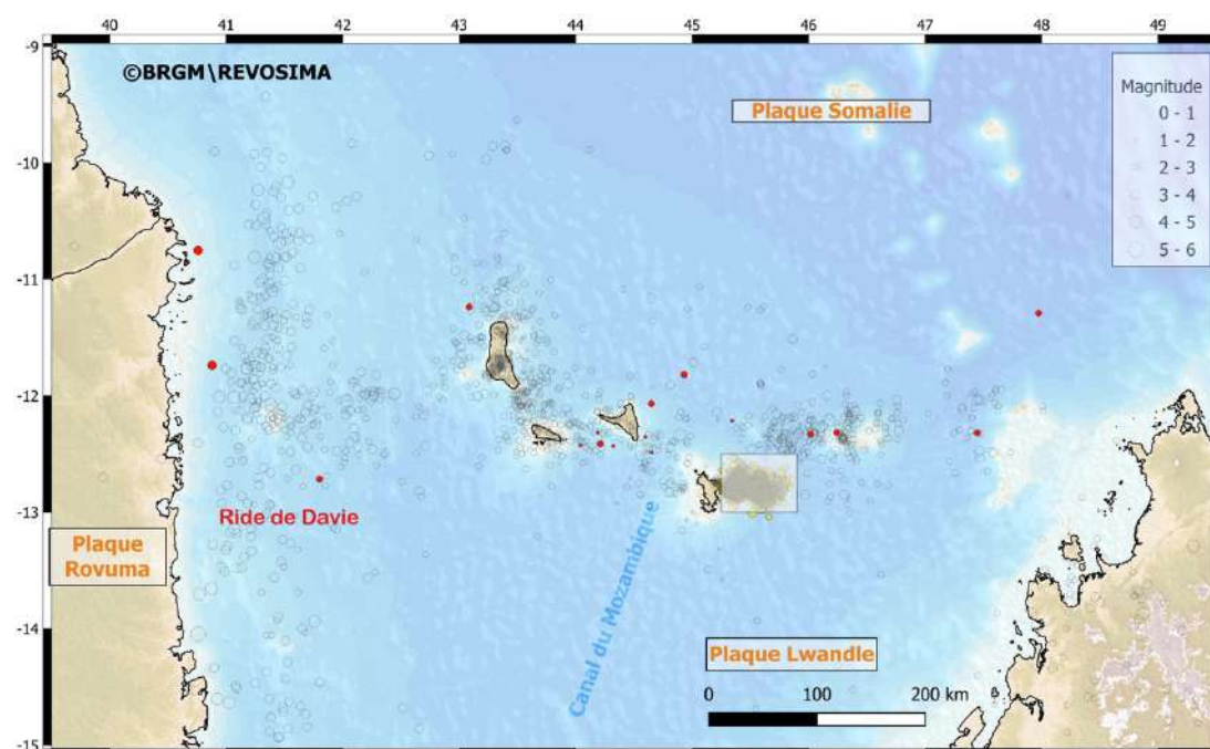
Figure 1: En rouge : séismes localisés au nord du Canal du Mozambique au mois de septembre 2026. Les cercles gris représentent la sismicité localisée depuis 2018. Bathymétrie et topographie : Gebco 2022, GEBCO Compilation Group (2022) GEBCO_2022 Grid (doi:10.5285/e0f0bb80-ab44-2739-e053-6c86abc0289c. Le cadre blanc à l'est de Mayotte délimite l'emprise de la sismicité associée au phénomène tellurique surveillé par le REVOSIMA dont le descriptif est présent dans une autre section de ce bulletin.
