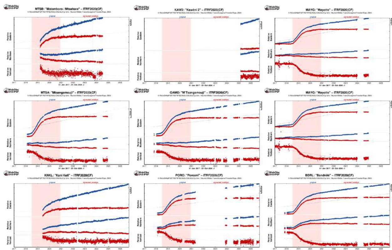
Figure 10 : Déplacements (en cm) enregistrés sur les stations GNSS localisées à Mayotte (MTSB, KAW2, MAYG, MTSA, GAMO, PMZI, KNKL, PORO, BDRL) entre le 1 er janvier 2017 et le 30 septembre 2026 pour visualiser une longue série temporelle ante crise. En bleu les données brutes, en rouge les données corrigées du mouvement de la plaque. Les stations sont présentées dans un ordre géographique ; du nord au sud (de haut en bas) et d'ouest en est (de gauche à droite). Post-traitement de ces données réalisé par l'IPGP. La durée de l'éruption du Fani Maoré est indiquée en rouge (©WebObs/OVPF-IPGP/REVOSIMA). Suite au passage du cyclone Chido sur Mayotte le 14 décembre 2024, deux stations (MAYG et MTSA) ont été détruites. En février 2025, une maintenance de la monumentation ainsi qu'un changement d'antenne à la station KAW2 ont conduit à la création d'une nouvelle station, KAW2 en remplacement de KAW1.
