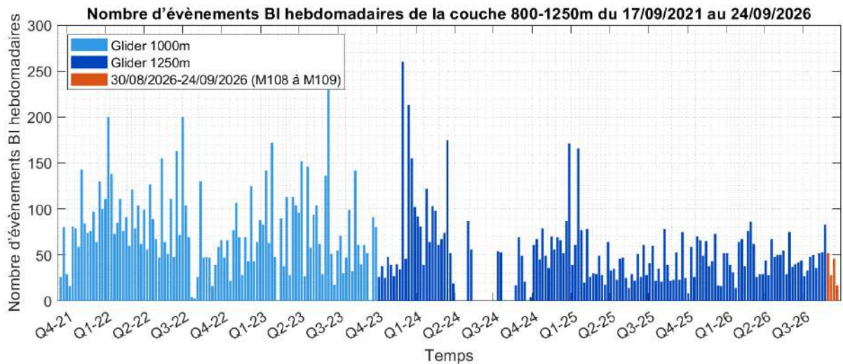
Figure 19 : Histogramme du nombre hebdomadaire de détections d'évènement BI (Backscatter Index) depuis le début de la surveillance par planeur (17/09/2021) et jusqu'au 24/09/2026 (fin de la mission 108). Résultats obtenus avec les planeurs limités à 1000 m d'immersion en bleu clair et à 1250 m d'immersion en bleu foncé. En orange, résultats pour la période entre le 30/08/2026 et le 24/09/2026 (missions 108 et 109) avec le planeur limité à 1250 m d'immersion. L'échelle de temps est représentée par quartiles des années 2021 à 2026. Les périodes où le planeur n'a pas été utilisé sont symbolisées par un nombre d'évènements BI hebdomadaire égal à zéro.
