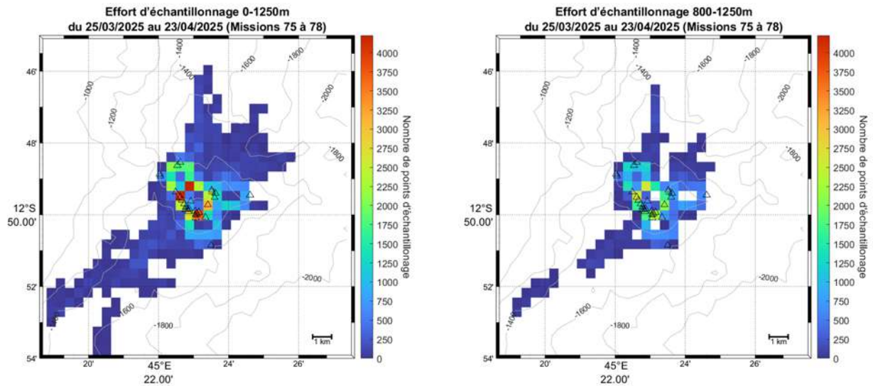
Figure 18 : Cartes centrées sur le Fer à Cheval représentant l'effort d'échantillonnage du planeur pour la période du 25/03/2025 au 23/04/2025 (missions 75 à 78) entre 0 et 1250 m de profondeur (à gauche), et entre 800 et 1250 m de profondeur (à droite). Le maillage est illustré par des cellules carrées mesurant 500 m de côté (0,5 km 2 ). La couleur représente le nombre de points d'échantillonnage réalisés dans chaque cellule. La bathymétrie est indiquée par des isobathes tous les 200 m. Les triangles noirs correspondent à la position du barycentre des sites actifs d'émissions de fluides déjà répertoriés (Scalabrin, C. (2023), https://doi.org/10.12770/070818f6-6520-49e4-bafd-9d4d0609bf7d ).
