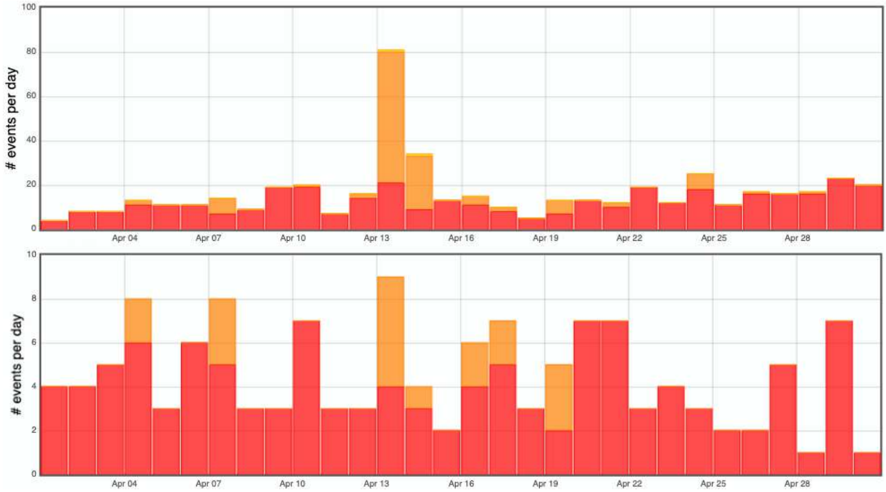
Figure 7 : Histogramme représentant le nombre de séismes par jour détectés (en haut) et localisés (en bas) en avril 2025 par le réseau sismologique du REVOSIMA. En rouge les séismes volcano-tectoniques, en orange les séismes longues périodes, en jaune les séismes très longues périodes, en bleu les ondes sonores liées aux orages (© OVPF-IPGP et REVOSIMA).
