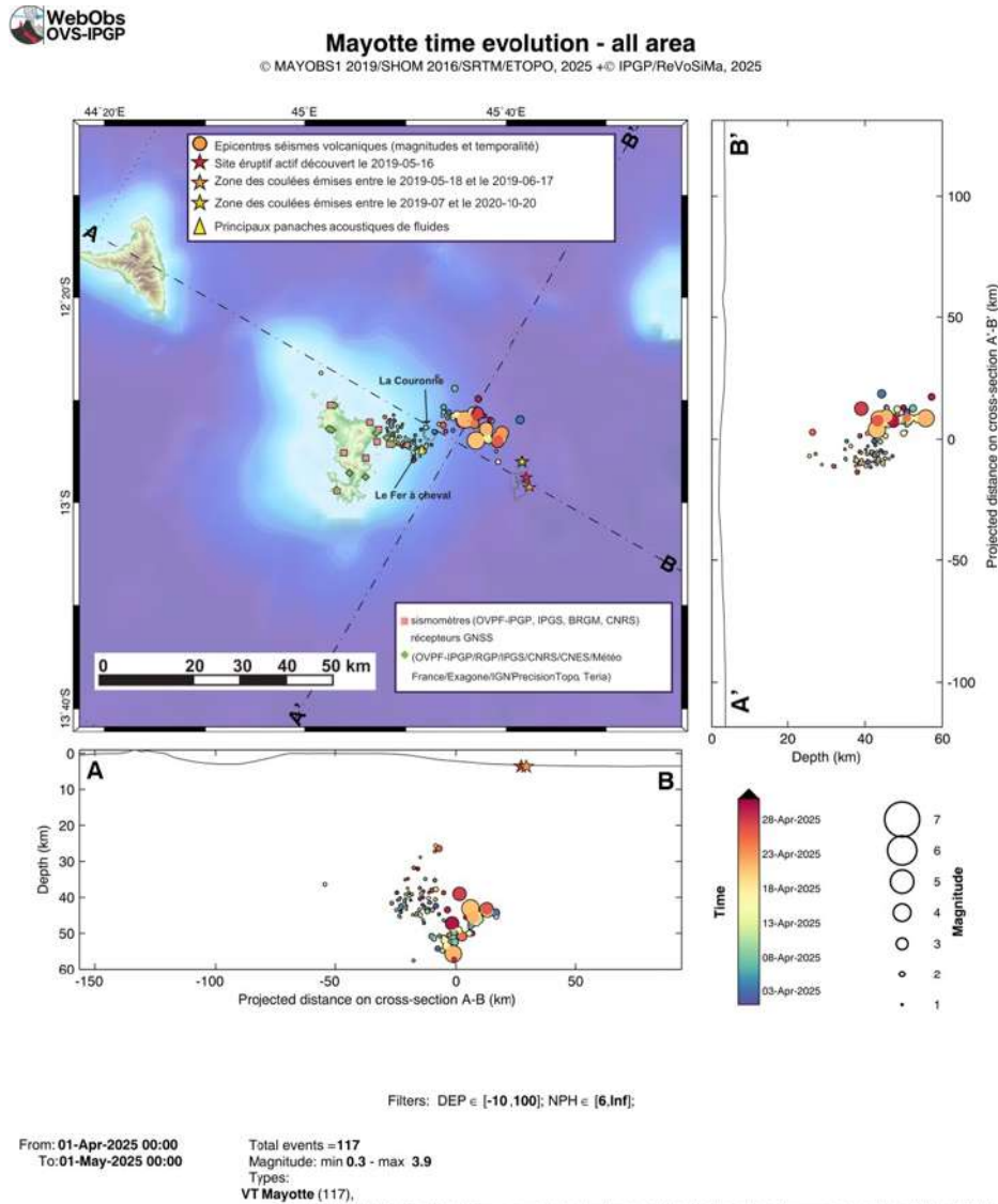
Figure 2 : Carte des épicentres ( \pm 5 km) des séismes volcano-tectoniques (VT) localisés avec les réseaux sismiques à terre (IPGP-CNRS-BRGM-BCSF-RENASS-ITES) en avril 2025 (échelle temporelle de couleur). Sont aussi représentées les projections des hypocentres des séismes le long de coupes transverses et axiales le long de la ride montrant la localisation estimée en profondeur (la précision varie entre \pm 5 km et \pm 15 km) des séismes en fonction de la magnitude (taille des symboles) et de la date (échelle temporelle de couleur). La localisation approximative des panaches acoustiques identifiés pendant les campagnes océanographiques est indiquée par des triangles jaunes, l'étoile rouge indique le site éruptif identifié le 16 mai 2019, l'étoile orange la zone des coulées émises entre le 18/05/2019 et le 17/06/2019 et l'étoile jaune la zone des coulées émises entre juillet 2019 et le 04/12/2020. Les structures volcaniques de la zone dites de « La Couronne » et du « Fer à Cheval » sont indiquées en gris tout comme les coulées de lave de Fani Maoré. Les stations sismiques du réseau terrestre et les stations de positionnement par satellite GPS sont indiquées par des symboles (voir légende) (©OVPF-IPGP, BRGM, IFREMER, CNRS, BCSF-RENASS, ITES / REVOSIMA).
