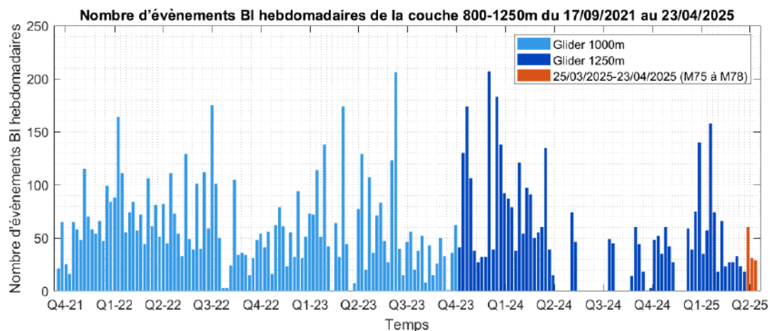
Figure 19 : Histogramme du nombre hebdomadaire de détections d'évènement BI (Backscatter Index) depuis le début de la surveillance par planeur (17/09/2021) et jusqu'au 23/04/2025 (fin de la mission 78). Résultats obtenus avec les planeurs limités à 1000 m d'immersion en bleu clair et à 1250 m d'immersion en bleu foncé. En orange, résultats pour la période entre le 25/03/2025 et le 23/04/2025 (Missions 75 à 78) avec le planeur limité à 1250 m d'immersion. L'échelle de temps est représentée par quartiles des années 2021 à 2025. Les périodes où le planeur n'a pas été utilisé sont symbolisées par un nombre d'évènements BI hebdomadaire égal à zéro.
