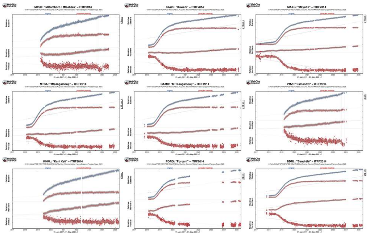
Figure 10 : Déplacements (en cm) enregistrés sur les stations GPS localisées à Mayotte (MTSB, KAWE, MAYG, MTSA, GAMO, PMZI, KNKL, PORO, BDRL) entre le 1 er janvier 2017 et le 30 avril 2025 pour visualiser une longue série temporelle ante crise. En bleu les données brutes, en rouge les données corrigées du mouvement de la plaque. Les stations sont présentées dans un ordre géographique ; du nord au sud (de haut en base à et d'ouest en est (de gauche à droite)). Post-traitement de ces données réalisé par l'IPGP / REVOSIMA. Suite au passage du cyclone Chido sur Mayotte le 14 décembre 2024, deux stations (MAYG et MTSA) ont été détruites, alors que les stations KNKL, KAWE, PORO, GAMO et BRDL ont subi des coupures électriques et/ou de transmission. En février 2025, une maintenance de la monumentation ainsi qu'un changement d'antenne à la station KAWE ont conduit à la création d'une nouvelle station, KAW2 en remplacement de KAWE.
