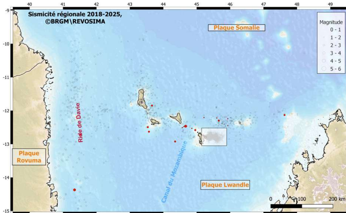
Figure 1: Sismicité régionale enregistrée depuis 2018 (modifié d'après Bertil et al. , 2021). Les séismes d'avril 2025 sont représentés en rouge. Le fond de carte est construit à partir des données topographiques et bathymétriques de Gebco 2022 ( www.gebco.net ). Le trait de côte et les frontières administratives sont extraits de https://gadm.org/ . Le carré blanc encadre les essaims sismiques surveillés depuis 2018. Se référer aux Figures 2 et 3 de ce bulletin pour la distribution de cette sismicité.
