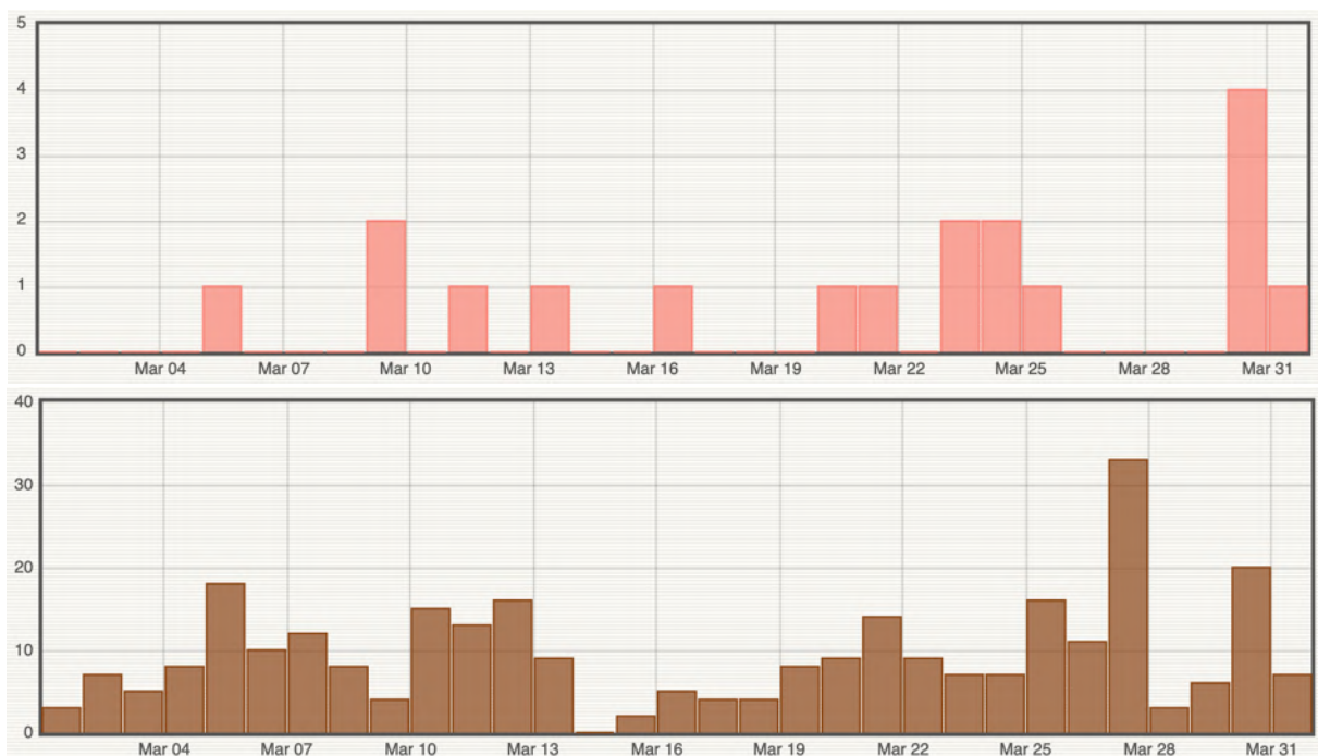
Figure 1 : Histogramme représentant le nombre de séismes volcano-tectoniques superficiels (en haut) et d'éboulements (en bas) par jour enregistrés en mars 2023 (© OVPF-IPGP).
