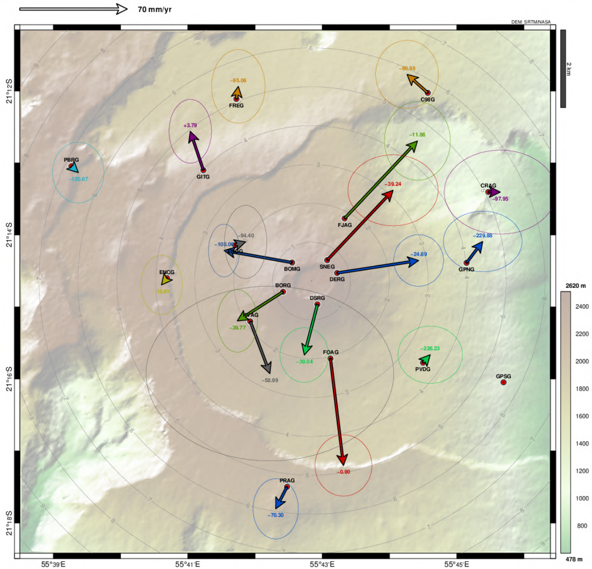
Figure 5 : Carte des déplacements du sol (exprimés en vitesse) enregistrés en mars 2023 à partir du réseau GPS permanent de l'OVPF-IPGP. Les déplacements horizontaux sont représentés sous forme vectorielle et les déplacements verticaux sont indiqués par les valeurs chiffrées en couleur (© OVPF-IPGP).
