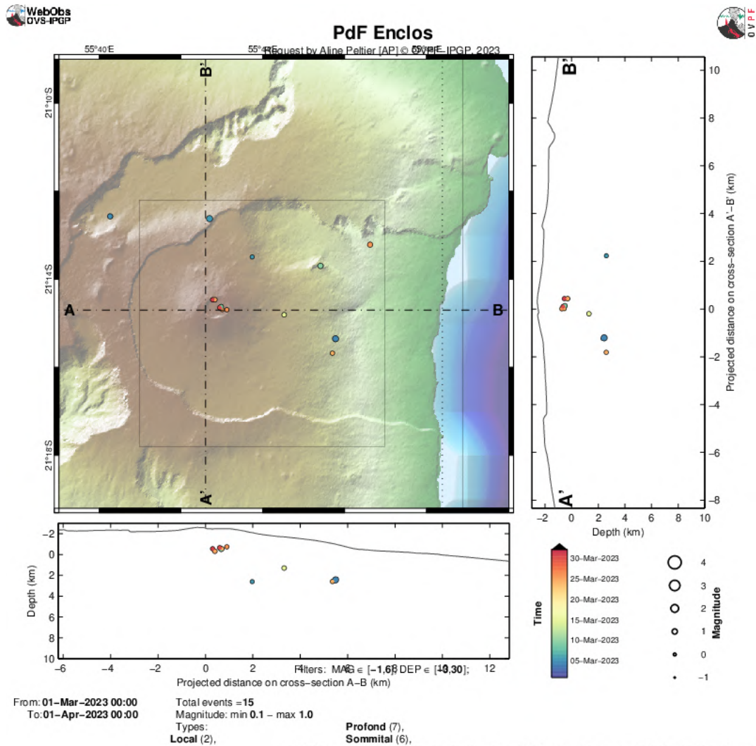
Figure 2 : Sismicité sous le Piton de la Fournaise au mois de mars 2023. Carte de localisation (épicentres) et coupes nord-sud et est-ouest (montrant la localisation en profondeur, hypocentres) des séismes enregistrés et localisés manuellement par l'OVPF-IPGP. Seuls les séismes localisables sont représentés sur la carte (© OVPF-IPGP).
