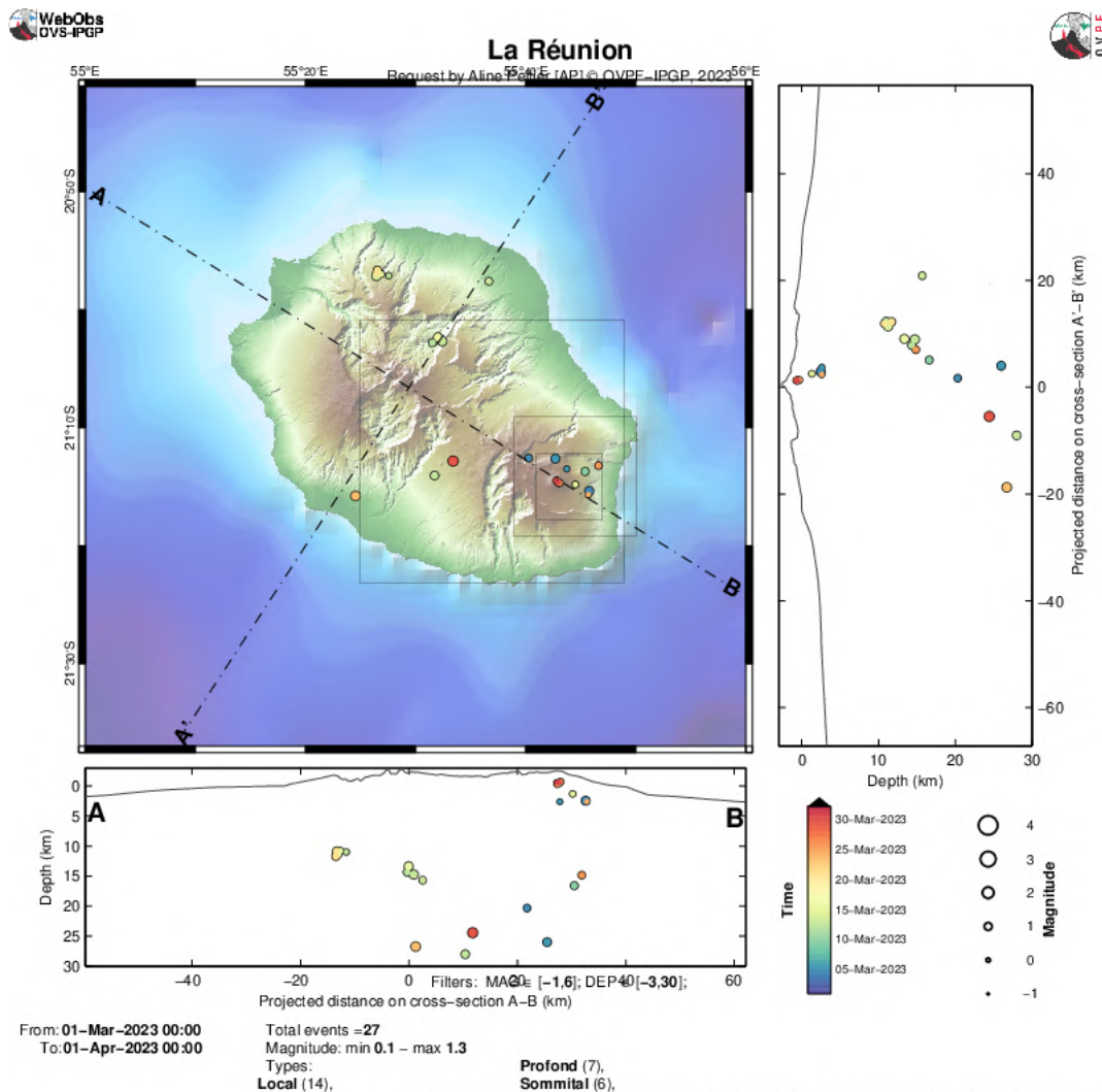
Figure 11 : Sismicité sous La Réunion au mois de mars 2023. Carte de localisation (épicentres) et coupes nord-ouest - sud-est et sud-ouest – nord-est (montrant la localisation en profondeur, hypocentres) des séismes enregistrés et localisés par l'OVPF-IPGP. Seuls les séismes localisables ont été représentés sur la carte (© OVPF-IPGP).
