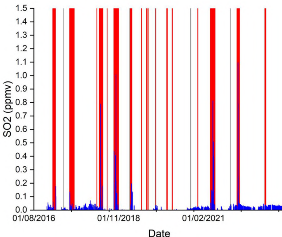
Figure 9 : Concentrations brutes (en bleu) de \text{SO}_2 dans l'atmosphère au sommet du Piton de la Fournaise (station MultiGaS) Barres rouges : éruptions ; Barres grises : intrusions (© OVPF-IPGP)
