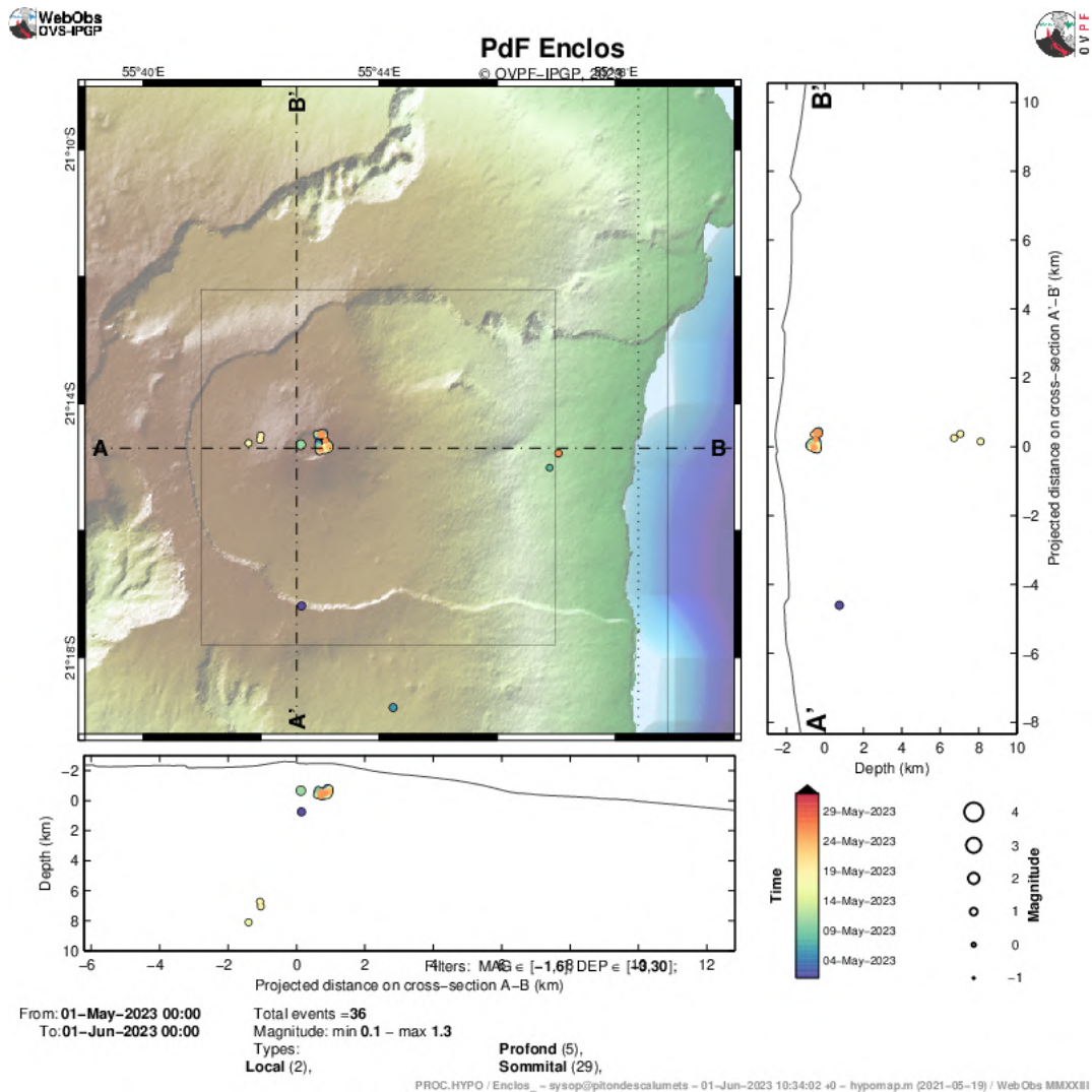
Figure 2 : Sismicité sous le Piton de la Fournaise au mois de mai 2023. Carte de localisation (épices) et coupes nord-sud et est-ouest (montrant la localisation en profondeur, hypocentres) des séismes enregistrés et localisés manuellement par l'OVPF-IPGP. Seuls les séismes localisables sont représentés sur la carte (© OVPF-IPGP).
