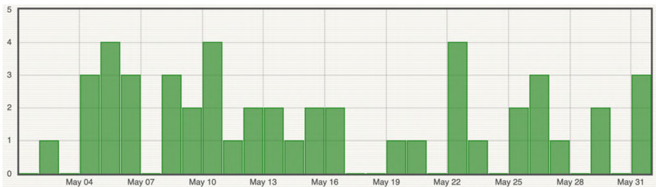
Figure 9 : Histogramme représentant le nombre de séismes locaux (Ile de La Réunion) par jour enregistrés en mai 2023 (© OVPF-IPGP).
