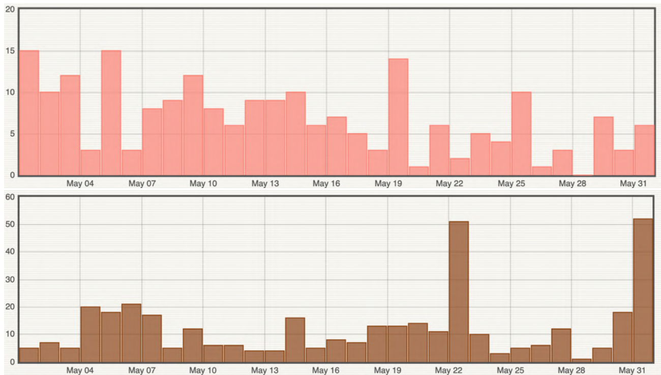
Figure 1 : Histogramme représentant le nombre de séismes volcano-tectoniques superficiels (en haut) et d'éboulements (en bas) par jour enregistrés en mai 2023 (© OVPF-IPGP).
