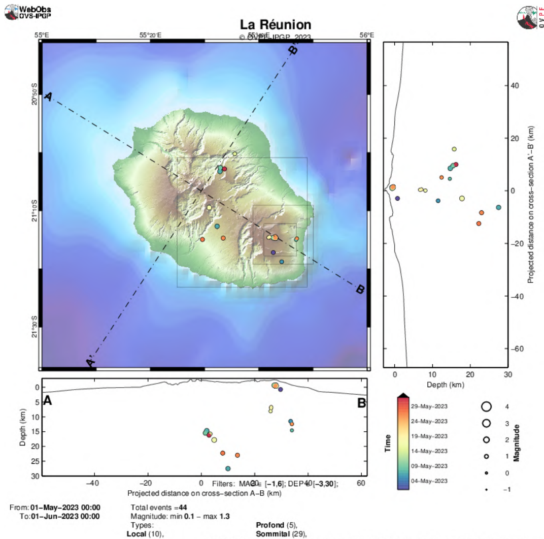
Figure 10 : Sismicité sous La Réunion au mois de mai 2023. Carte de localisation (épencentres) et coupes nord-ouest - sud-est et sud-ouest – nord-est (montrant la localisation en profondeur, hypocentres) des séismes enregistrés et localisés par l'OVPF-IPGP. Seuls les séismes localisables ont été représentés sur la carte (© OVPF-IPGP).
