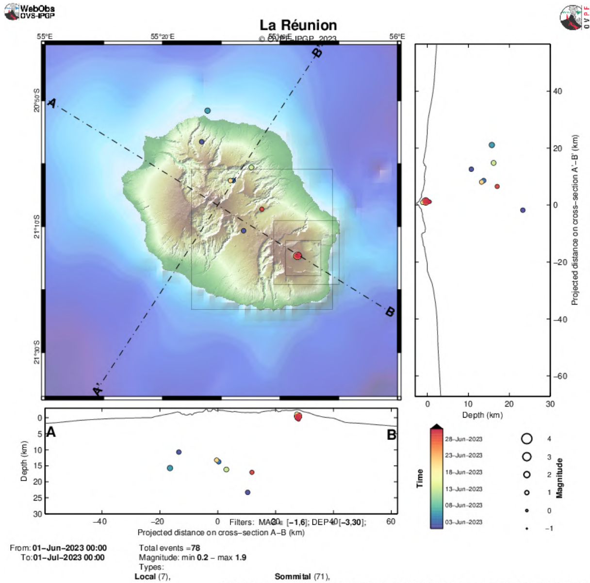
Figure 10 : Sismicité sous La Réunion au mois de juin 2023. Carte de localisation (épicentres) et coupes nord-ouest - sud-est et sud-ouest - nord-est (montrant la localisation en profondeur, hypocentres) des séismes enregistrés et localisés par l'OVPF-IPGP. Seuls les séismes localisables ont été représentés sur la carte (© OVPF-IPGP).
