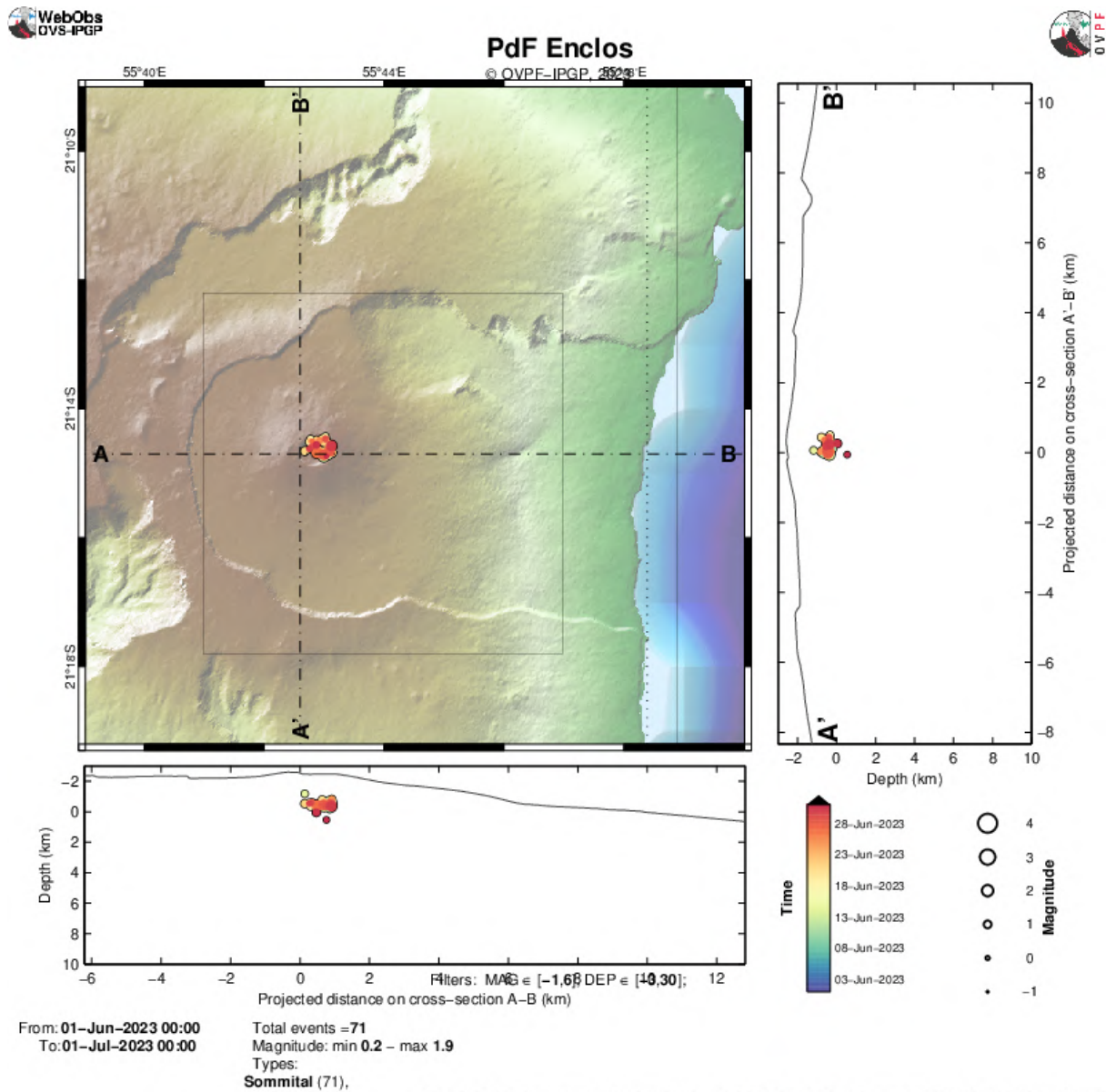
Figure 2 : Sismicité sous le Piton de la Fournaise au mois de juin 2023. Carte de localisation (épicentres) et coupes nord-sud et est-ouest (montrant la localisation en profondeur, hypocentres) des séismes enregistrés et localisés manuellement par l'OVPF-IPGP. Seuls les séismes localisables sont représentés sur la carte (© OVPF-IPGP).
