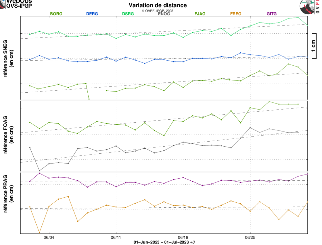
Figure 4 : Illustration de la déformation en juin 2023 (les éventuelles périodes éruptives et intrusives sont respectivement représentées par un fond rouge et vert). Sont ici représentées les variations de distance entre deux récepteurs GPS traversant l'édifice du Piton de la Fournaise, au sommet (référence SNEG ; en haut), à la base du cône terminal (référence FOAG ; au milieu) et en champ lointain (référence PRAG ; en bas) (cf. localisation sur la Figure 6). Une hausse est synonyme d'élongation et donc de gonflement du volcan ; inversement une diminution indique une contraction et donc un dégonflement du volcan (© OVPF-IPGP).
