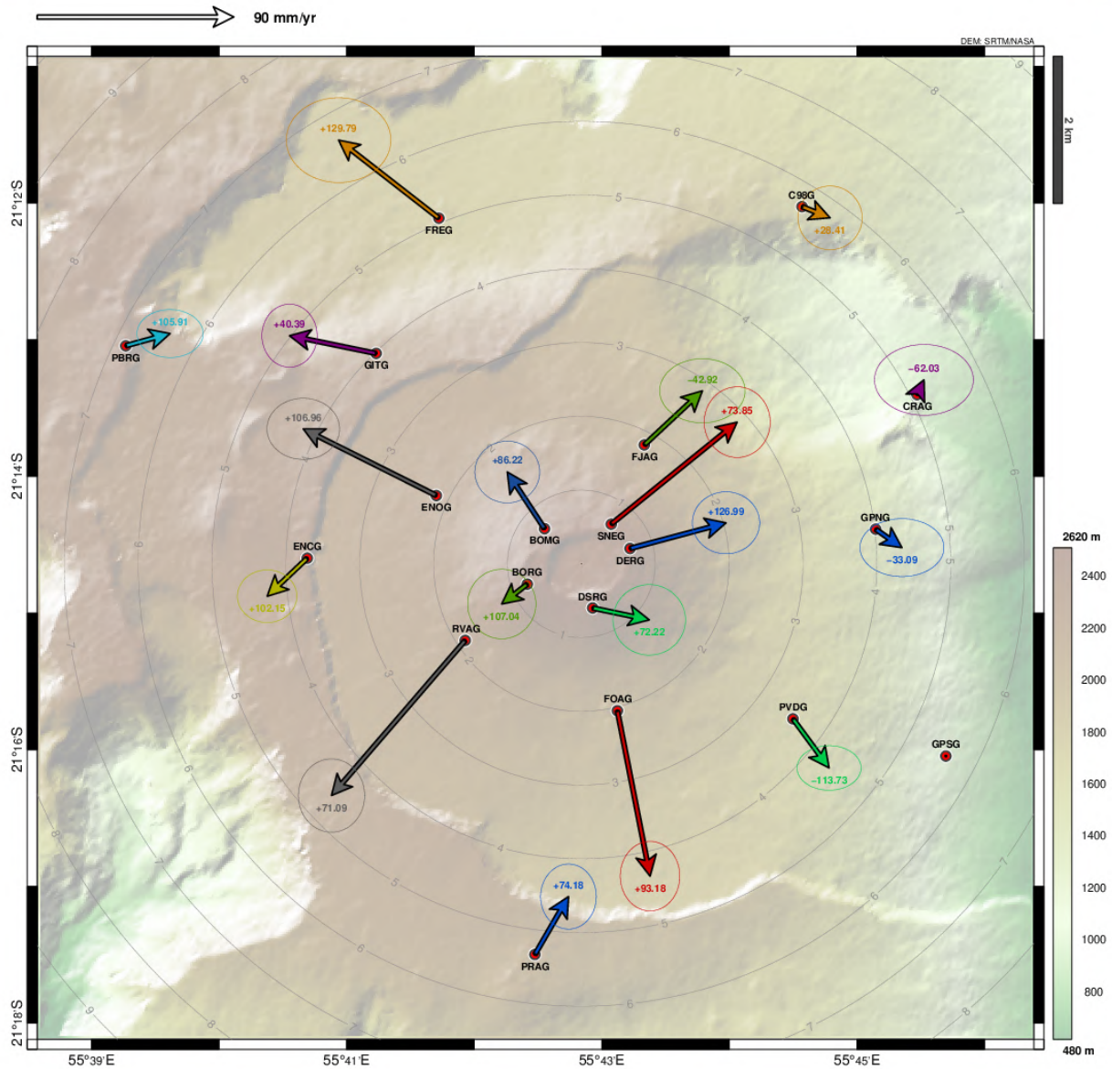
Figure 5 : Carte des déplacements du sol (exprimés en vitesse) enregistrés en juin 2023 à partir du réseau GPS permanent de l'OVPF-IPGP. Les déplacements horizontaux sont représentés sous forme vectorielle et les déplacements verticaux sont indiqués par les valeurs chiffrées en couleur (© OVPF-IPGP).
