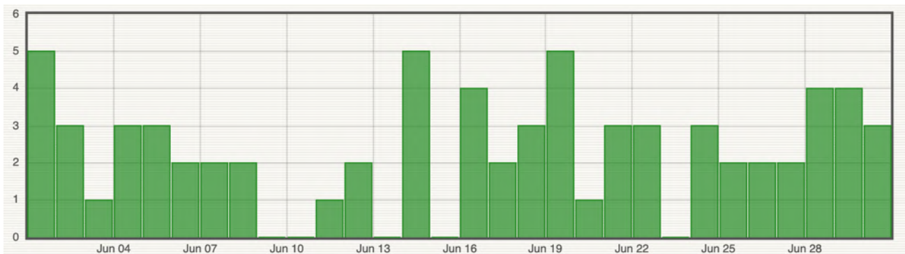
Figure 9 : Histogramme représentant le nombre de séismes locaux (Ile de La Réunion) par jour enregistrés en juin 2023 (© OVPF-IPGP).
