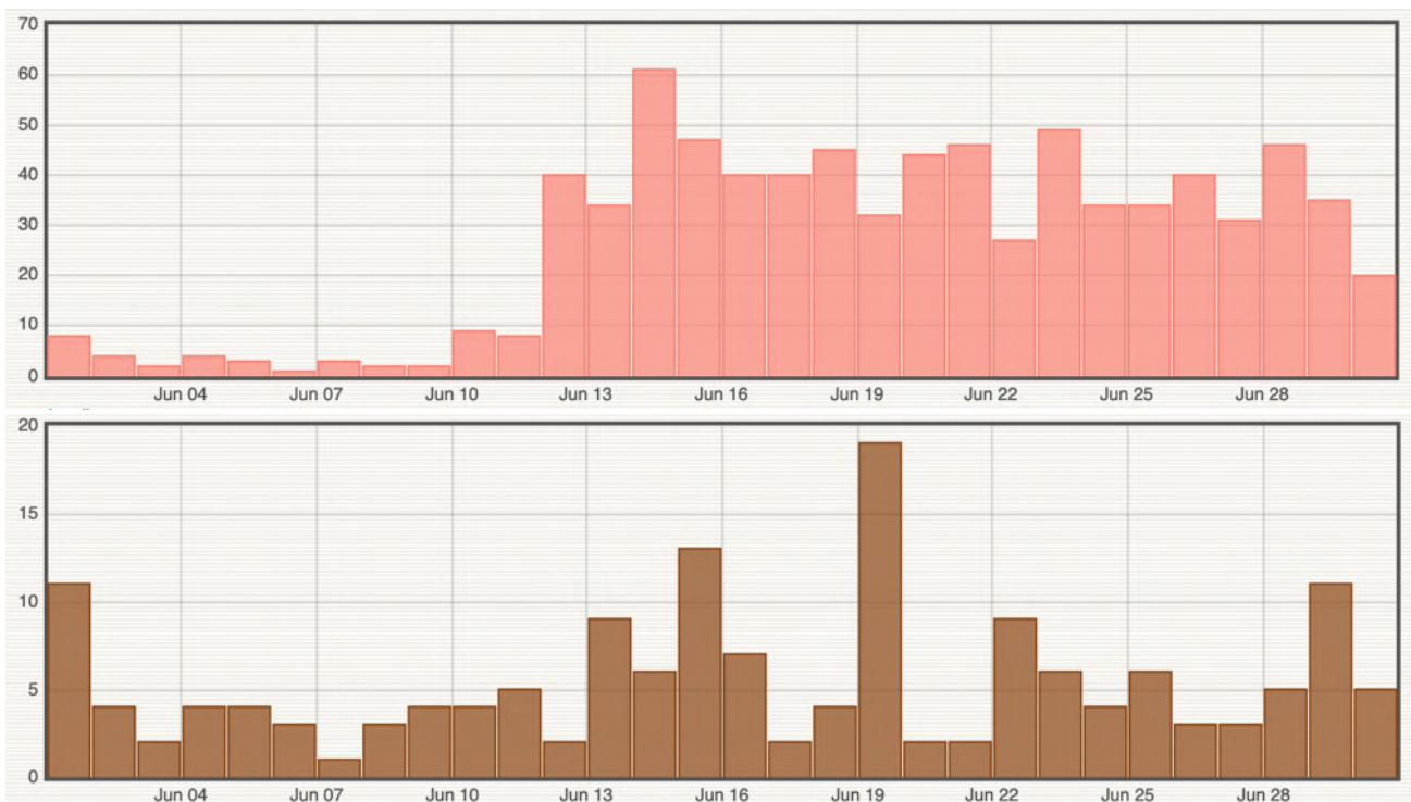
Figure 1 : Histogramme représentant le nombre de séismes volcano-tectoniques superficiels (en haut) et d'éboulements (en bas) par jour enregistrés en juin 2023 (© OVPF-IPGP).
