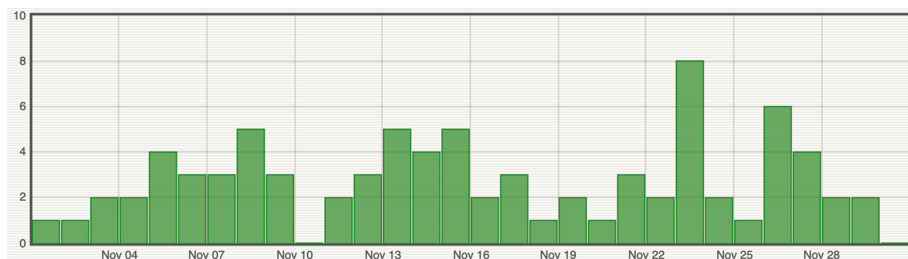
Figure 9 : Histogramme représentant le nombre de séismes locaux (Île de La Réunion) par jour enregistrés en novembre 2023 (© OVPF-IPGP).
