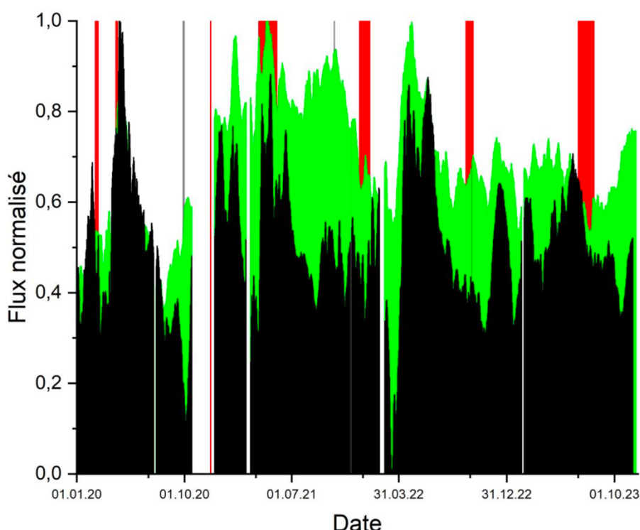
Figure 7 : Comparaison entre les moyennes normalisées des données de flux de CO 2 dans le sol, corrigées de l'influence à court terme (modèle OVPF ; moyennées sur une fenêtre glissante de 15 jours, en vert) et corrigées de l'influence à long terme des paramètres environnementaux (modèle INGV MALFIT ; en noir), enregistrées sur les stations localisées en champ lointain depuis octobre 2016 (date d'installation de la dernière station). Les périodes éruptives sont représentées en rouge et les périodes intrusives en gris (© OVPF-IPGP).
