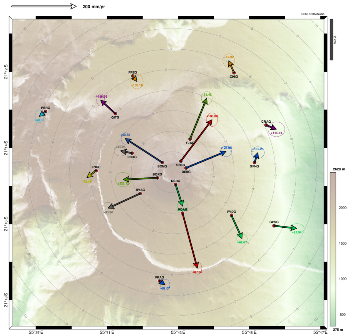
Figure 6 : Carte des déplacements du sol (exprimés en vitesse, mm/an) enregistrés entre le 1 er et le 30 novembre 2023 à partir du réseau GPS permanent de l'OVPF-IPGP. Les déplacements horizontaux sont représentés sous forme vectorielle et les déplacements verticaux sont indiqués par les valeurs chiffrées en couleur (© OVPF-IPGP).
