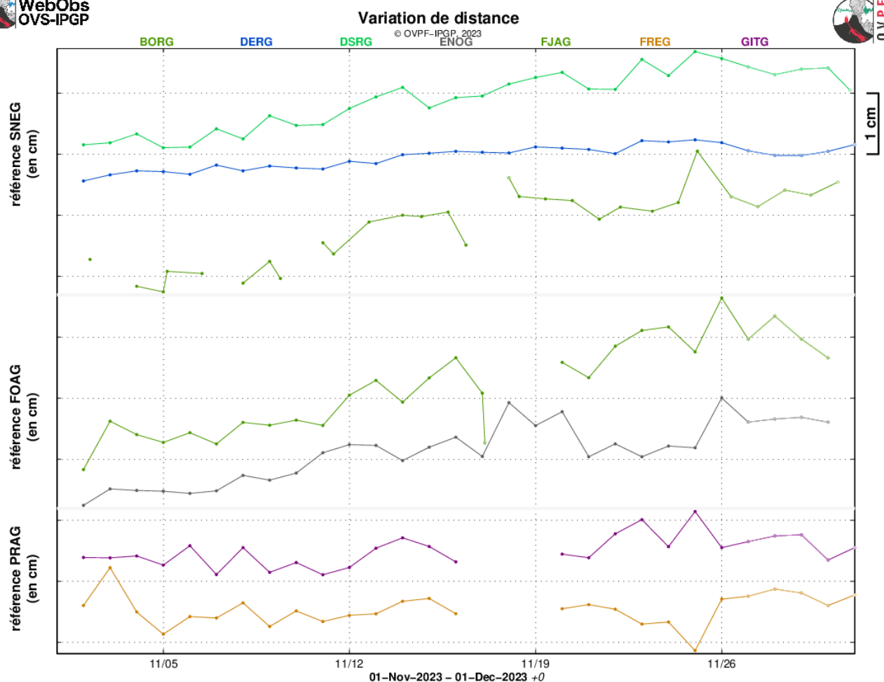
Figure 4 : Illustration de la déformation en novembre 2023 (les éventuelles périodes éruptives et intrusives sont respectivement représentées par un fond rouge et vert). Sont ici représentées les variations de distance entre deux récepteurs GPS traversant l'édifice du Piton de la Fournaise, au sommet (référence SNEG ; en haut), à la base du cône terminal (référence FOAG ; au milieu) et en champ lointain (référence PRAG ; en bas). La localisation des stations GPS est indiquée sur la Figure 5. Une hausse est synonyme d'élongation et donc de gonflement du volcan ; inversement une diminution indique une contraction et donc un dégonflement du volcan (© OVPF-IPGP).
