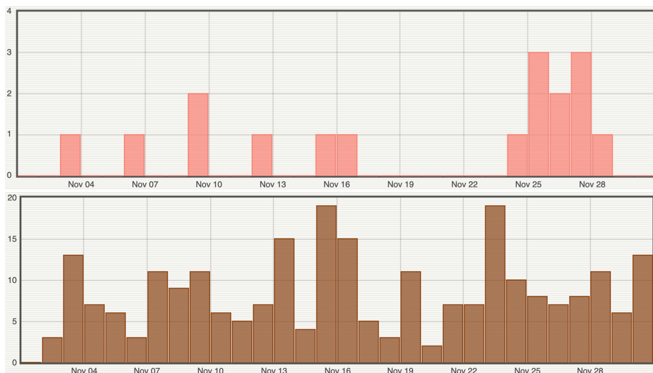
Figure 1 : Histogramme représentant le nombre de séismes volcano-tectoniques superficiels (en haut) et d'éboulements (en bas) par jour enregistrés en novembre 2023 (© OVPF-IPGP).
