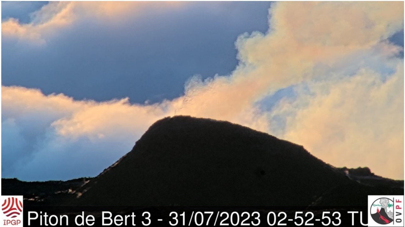
Figure 2 : Prise de vue du point d'émission actif situé au sud-est de l'Enclos Fouqué le 31/07/2023 à 06h52 heure locale (02h52 UTC). Image zoomée depuis la webcam IRT-OVPF-IPGP située au Piton de Bert (©IRT et OVPF-IPGP)
