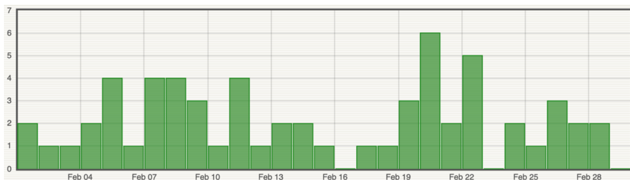
Figure 8 : Histogramme représentant le nombre de séismes locaux (Ile de La Réunion) par jour enregistrés en février 2024 (© OVPF-IPGP).
