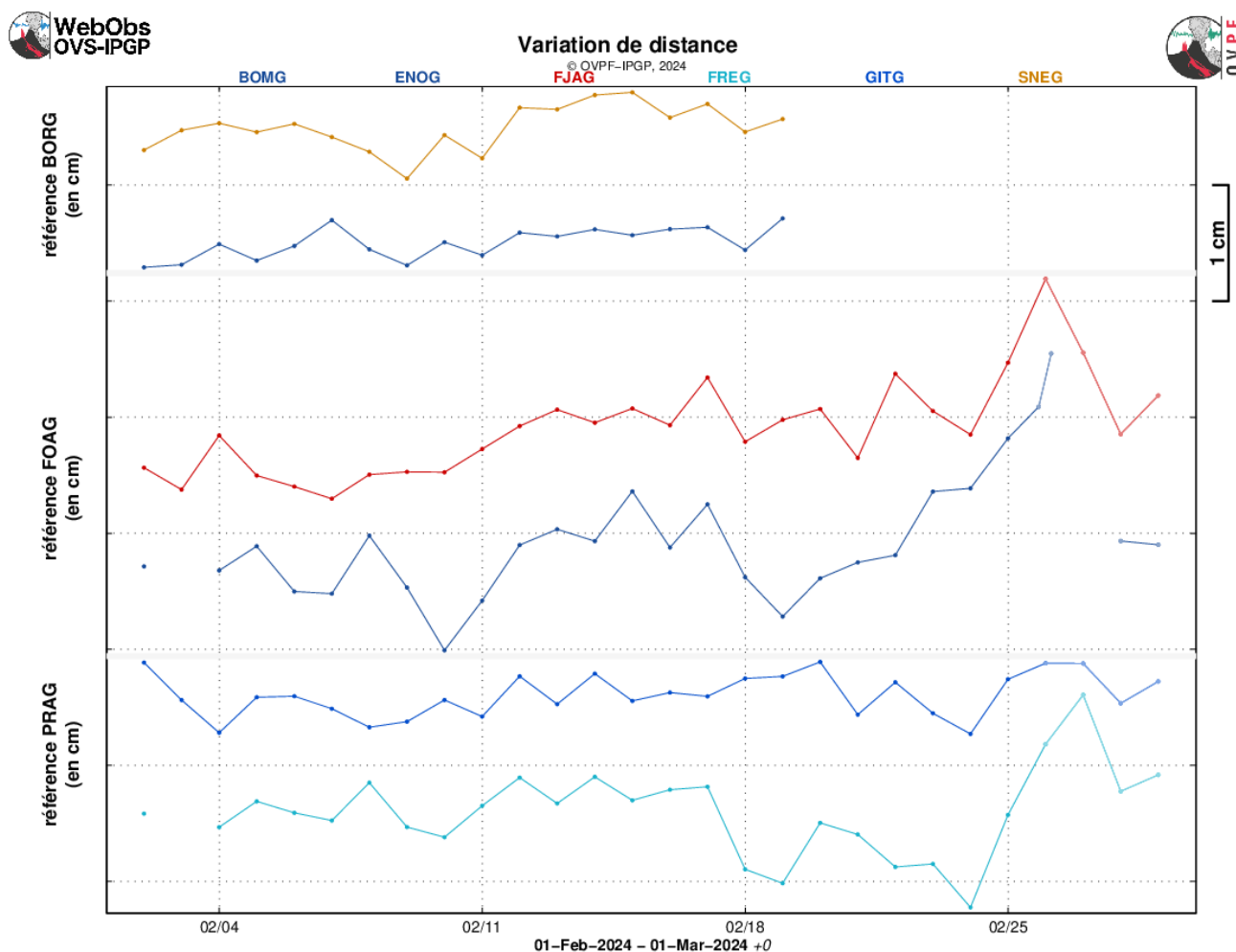
Figure 4 : Illustration de la déformation en février 2024 (les éventuelles périodes éruptives et intrusives sont respectivement représentées par un fond rouge et vert). Sont ici représentées les variations de distance entre deux récepteurs GPS traversant l'édifice du Piton de la Fournaise, au sommet (référence BORG ; en haut), à la base du cône terminal (référence FOAG ; au milieu) et en champ lointain (référence PRAG ; en bas). La localisation des stations GPS est indiquée sur la Figure 5. Une hausse est synonyme d'élongation et donc de gonflement du volcan ; inversement une diminution indique une contraction et donc un dégonflement du volcan. A noter que suite au passage du cyclone Belal 3 des 5 stations GNSS situées au sommet du volcan sont actuellement HS, et une 4 ème (BORG) présente des soucis d'énergie (© OVPF-IPGP).
