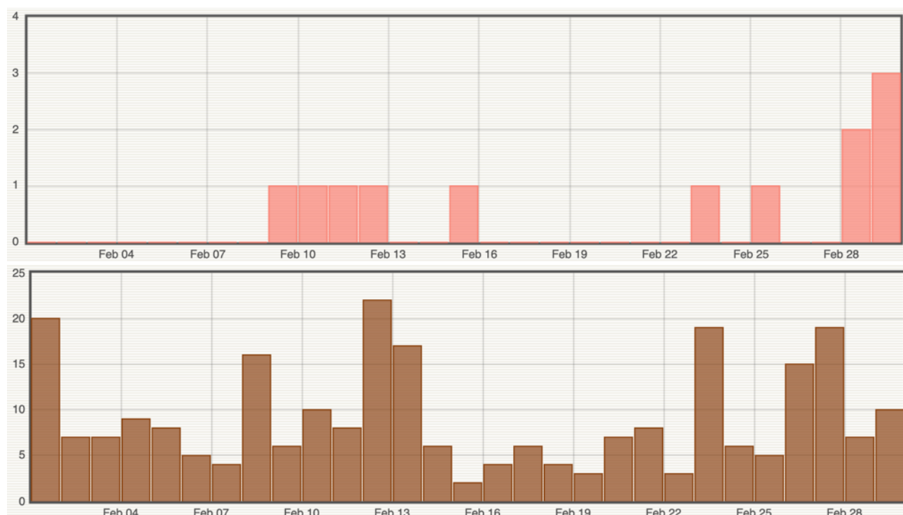
Figure 1 : Histogramme représentant le nombre de séismes volcano-tectoniques superficiels (en haut) et d'éboulements (en bas) par jour enregistrés en février 2024 (© OVPF-IPGP).
