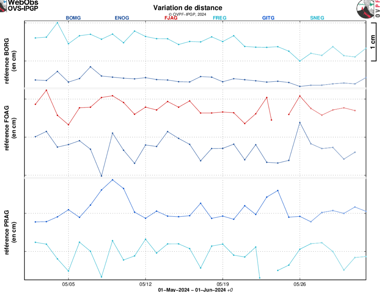
Figure 4 : Illustration de la déformation en mai 2024 (les éventuelles périodes éruptives et intrusives sont respectivement représentées par un fond rouge et vert). Sont ici représentées les variations de distance entre deux récepteurs GPS traversant l'édifice du Piton de la Fournaise, au sommet (référence BORG ; en haut), à la base du cône terminal (référence FOAG ; au milieu) et en champ lointain (référence PRAG ; en bas). La localisation des stations GPS est indiquée sur la Figure 5. Une hausse est synonyme d'élongation et donc de gonflement du volcan ; inversement une diminution indique une contraction et donc un dégonflement du volcan (© OVPF-IPGP).
