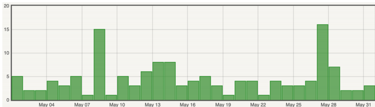
Figure 8 : Histogramme représentant le nombre de séismes locaux (Île de La Réunion) par jour enregistrés en mai 2024 (© OVPF-IPGP).
