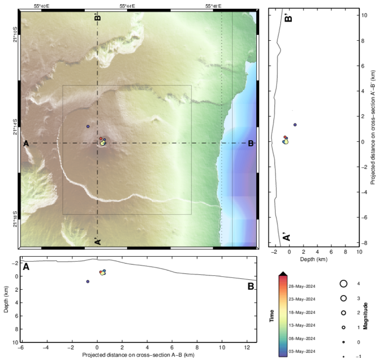
Figure 2 : Sismicité sous le Piton de la Fournaise au mois de mai 2024. Carte de localisation (épices) et coupes nord-sud et est-ouest (montrant la localisation en profondeur, hypocentres) des séismes enregistrés et localisés manuellement par l'OVPF-IPGP. Seuls les séismes localisables sont représentés sur la carte (© OVPF-IPGP).
