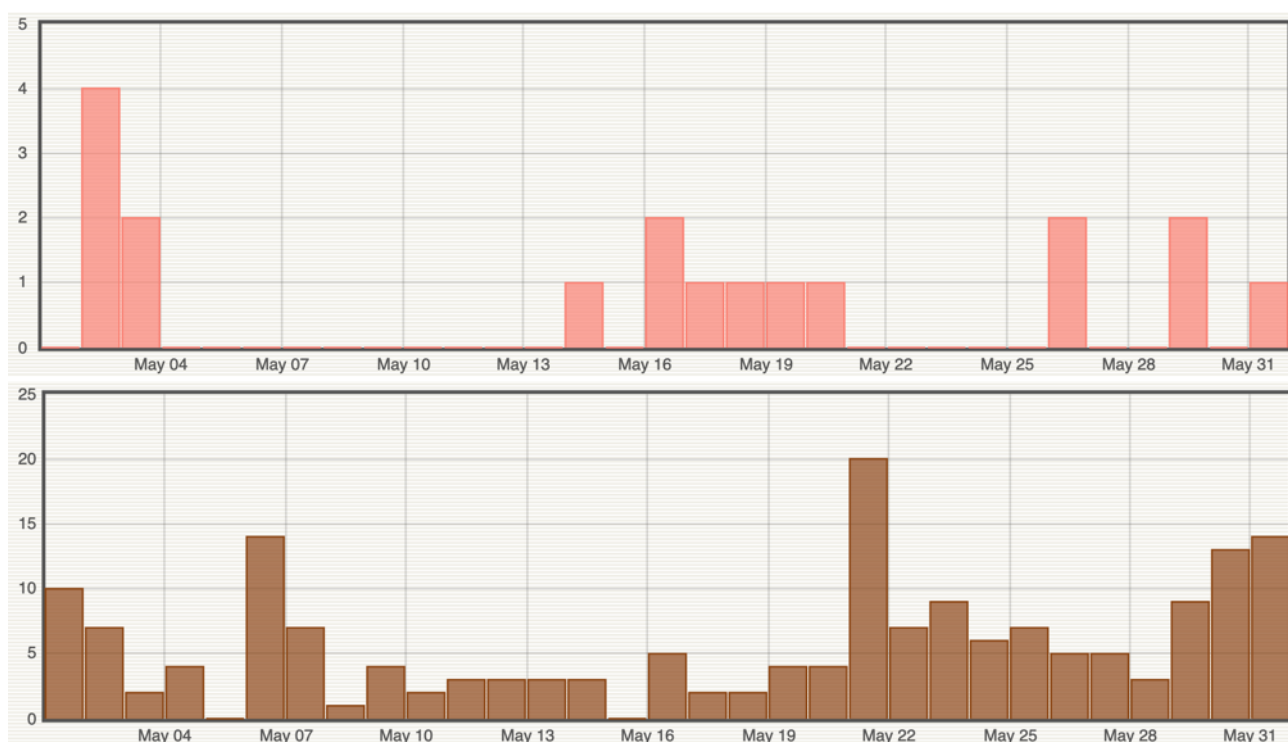
Figure 1 : Histogramme représentant le nombre de séismes volcano-tectoniques superficiels (en haut) et d'éboulements (en bas) par jour enregistrés en mai 2024 (© OVPF-IPGP).
