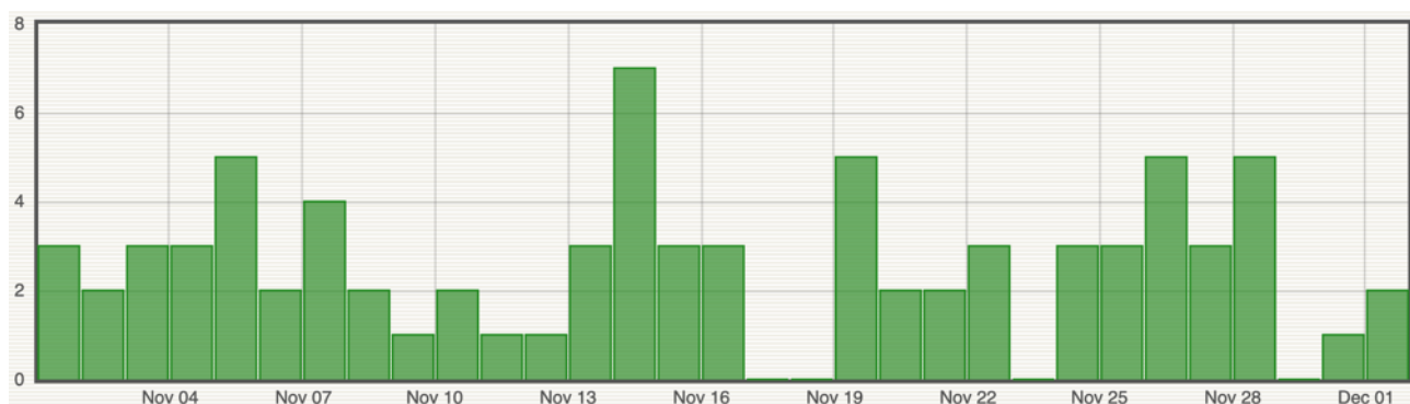
Figure 8 : Histogramme représentant le nombre de séismes locaux (Ile de La Réunion) par jour enregistrés en novembre 2024 (© OVPF-IPGP).
