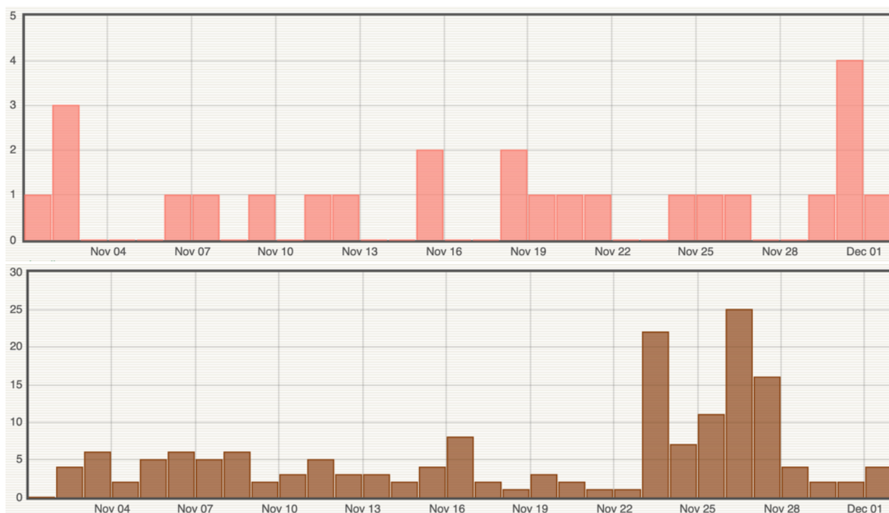
Figure 1 : Histogramme représentant le nombre de séismes volcano-tectoniques superficiels (en haut) et d'éboulements (en bas) par jour enregistrés en novembre 2024 (© OVPF-IPGP).
