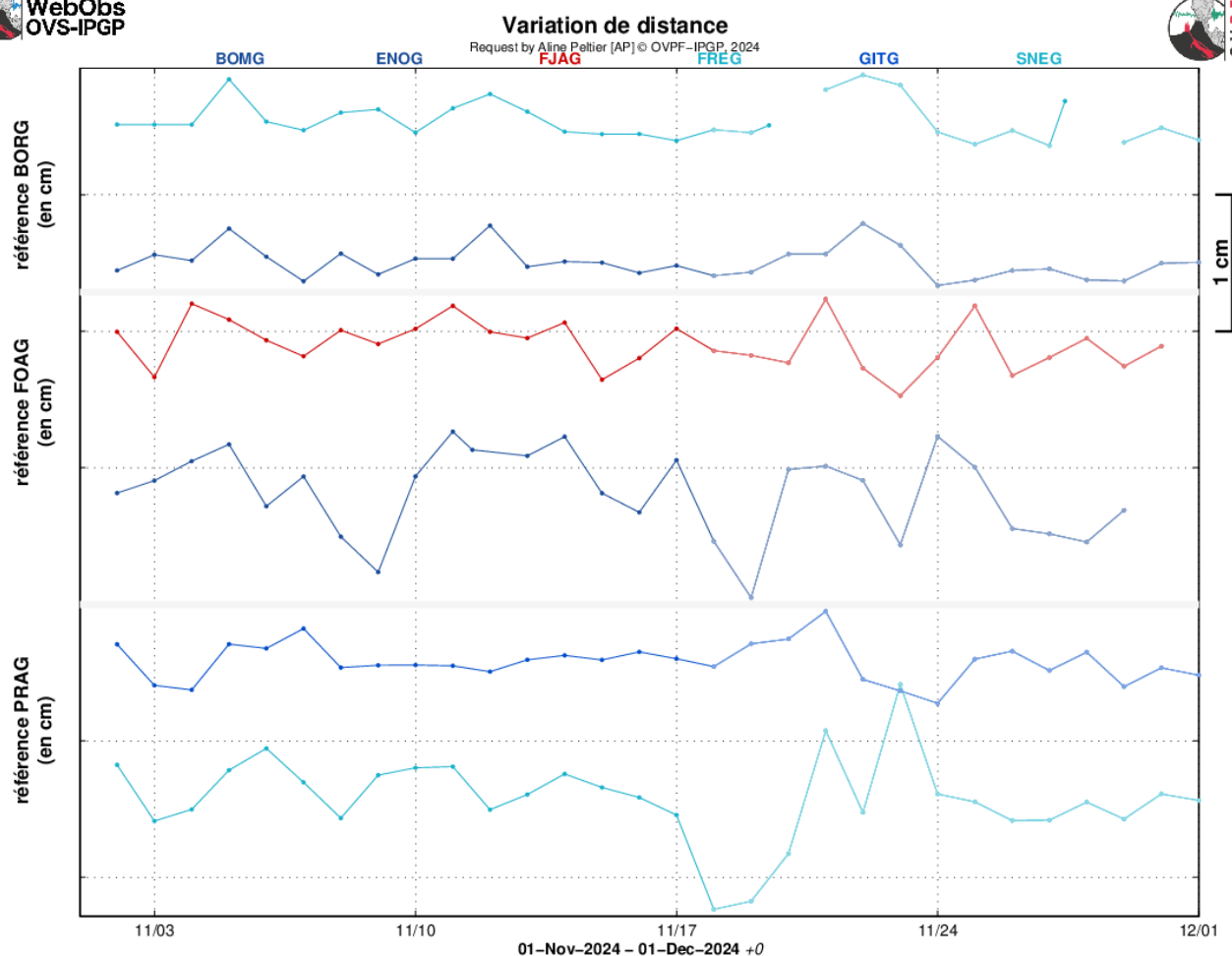
Figure 4 : Illustration de la déformation en novembre 2024 (les éventuelles périodes éruptives et intrusives sont respectivement représentées par un fond rouge et vert). Sont ici représentées les variations de distance entre deux récepteurs GPS traversant l'édifice du Piton de la Fournaise, au sommet (référence BORG ; en haut), à la base du cône terminal (référence FOAG ; au milieu) et en champ lointain (référence PRAG ; en bas). La localisation des stations GPS est indiquée sur la Figure 5. Une hausse est synonyme d'élongation et donc de gonflement du volcan ; inversement une diminution indique une contraction et donc un dégonflement du volcan (© OVPF-IPGP).
