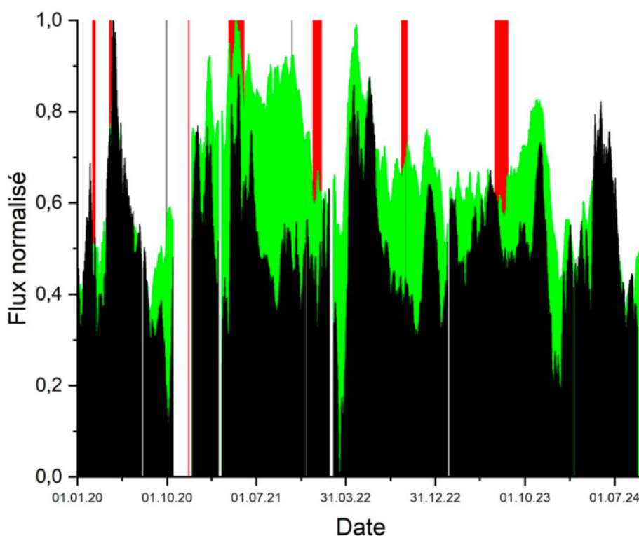
Figure 6 : Comparaison entre les moyennes normalisées des données de flux de CO 2 dans le sol, corrigées de l'influence à court terme (modèle OVPF ; moyennées sur une fenêtre glissante de 15 jours, en vert) et corrigées de l'influence à long terme des paramètres environnementaux (modèle INGV Malfit ; en noir), enregistrées sur les stations localisées en champ lointain depuis octobre 2016 (date d'installation de la dernière station). Les périodes éruptives sont représentées en rouge et les périodes intrusives en gris (© OVPF-IPGP).
