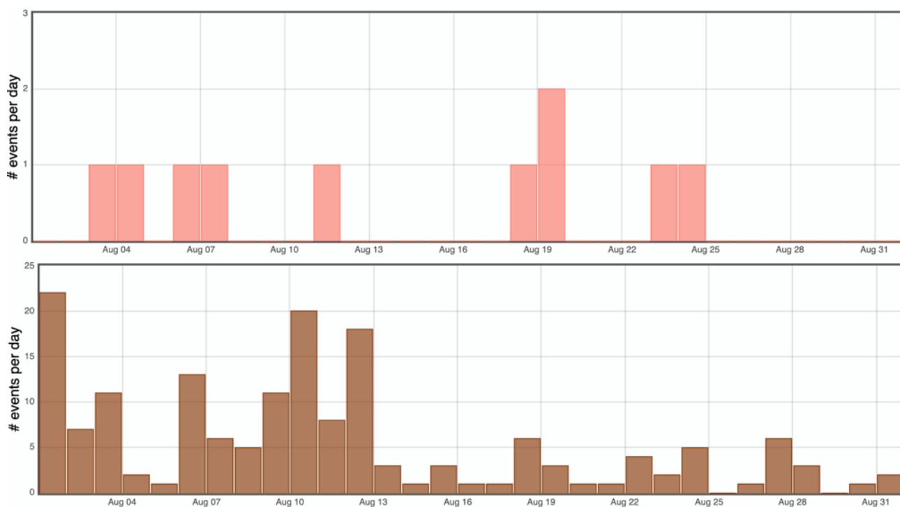
Figure 1 : Histogramme représentant le nombre de séismes volcano-tectoniques superficiels (en haut) et d'éboulements (en bas) par jour enregistrés en août 2025 (© OVPF-IPGP).
