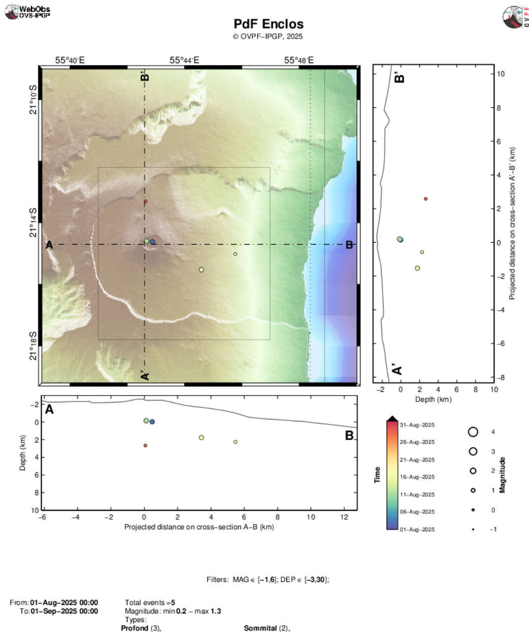
Figure 2 : Sismicité sous le Piton de la Fournaise au mois d'août 2025. Carte de localisation (épices) et coupes nord-sud et est-ouest (montrant la localisation en profondeur, hypocentres) des séismes enregistrés et localisés manuellement par l'OVPF-IPGP. Seuls les séismes localisables sont représentés sur la carte (© OVPF-IPGP).
