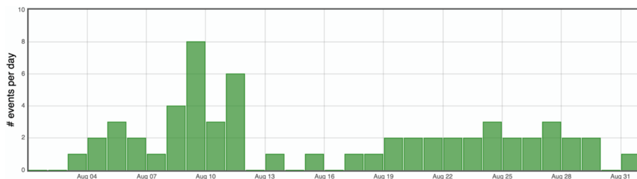
Figure 9 : Histogramme représentant le nombre de séismes locaux (Ile de La Réunion) par jour enregistrés en août 2025 (© OVPF-IPGP).
