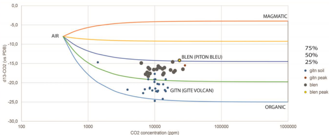
Figure 7 : Variations des isotopes du carbone ( \delta^{13}C ) dans le CO 2 des gaz du sol émis par la station proximale GITN et distale BLEN. Les mesures effectuées au début (mars 2024) de la phase de pic des émissions de CO 2 ne montrent pas de forte augmentation du pourcentage de la contribution magmatique.
