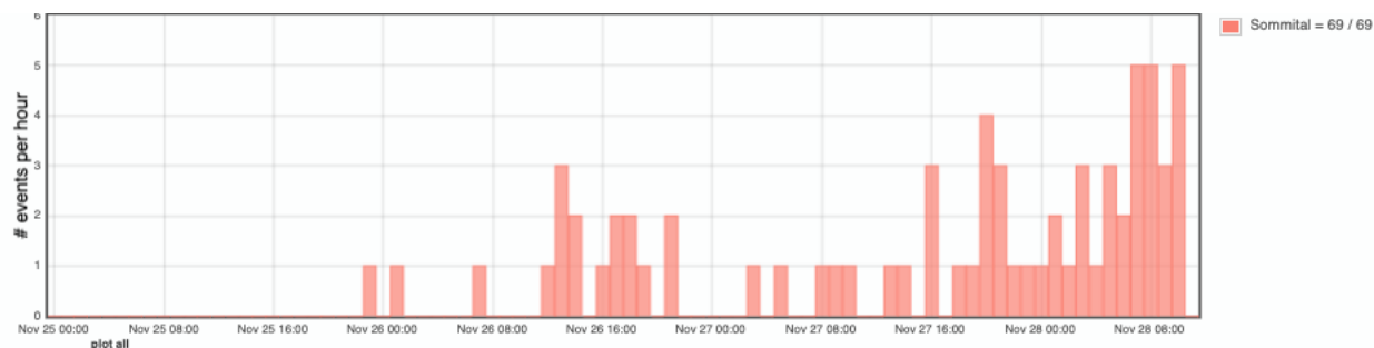
Figure 1 : Histogramme représentant le nombre de séismes volcano-tectoniques superficiels par heure depuis le 25 novembre (© OVPF-IPGP).
