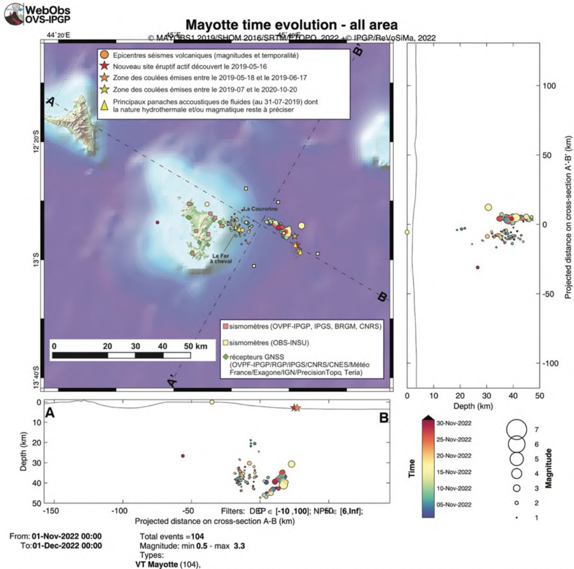
Figure 1a : Carte des épicentres ( \pm 5 km) des séismes volcano-tectoniques (VT) localisés avec les réseaux sismiques à terre (IPGP-CNRS-BRGM-BCSF-RENASS, ITES) entre le 1 er et 30 novembre 2022 (échelle temporelle de couleur). Sont aussi représentées une projection des hypocentres des séismes le long de coupes transversales et axiales le long de la ride montrant la localisation estimée en profondeur (la précision varie entre \pm 5 km et \pm 15 km) des séismes en fonction de la magnitude (taille des symboles et de la date (échelle temporelle de couleur)). La localisation approximative des panaches acoustiques identifiés pendant les campagnes océanographiques (MD220-MAYOBS1, MD221-MAYOBS2, MD222-MAYOBS3, MD223-MAYOBS4, MAYOBS15, MAYOBS17) et dont la nature hydrothermale et/ou magmatique reste à préciser, est indiquée par des triangles jaunes, l'étoile rouge indique le site éruptif nouvellement identifié le 16 mai 2019, l'étoile orange la zone des coulées émises entre le 18/05/2019 et le 17/06/2019 et l'étoile jaune la zone des coulées émises entre juillet 2019 et le 18/01/2021. Les structures volcaniques de la zone dite de « La Couronne », du « Fer à cheval » sont indiquées en grisé tout comme les coulées de lave de Fani Maoré. Les stations sismiques du réseau terrestre, les sismomètres fond de mer (OBS) et les stations de positionnement par satellite GPS sont indiquées par des symboles (voir légende). (©OVPF-IPGP, BRGM, IFREMER, CNRS, BCSF-RENASS, ITES / REVOSIMA).
