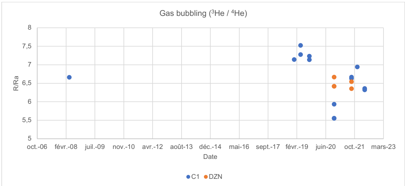
Figure 13 : Analyses isotopiques (gaz rares) des bullages au points de contrôle C1 (estran de l'aéroport) et DZN (Lac Dziani). Une augmentation du R/Ra (rapport isotopique de l'He normalisé à celui de l'atmosphère) est liée à une augmentation de la contribution des fluides profonds remontant du manteau. Erreur moyenne sur chaque analyse : 0.05 unité.
