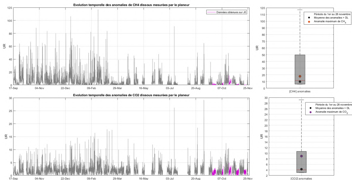
Figure 18 : Évolution temporelle des anomalies en CH 4 (haut) et CO 2 (bas) dissous mesurées entre 900 et 1000 m de profondeur par le planeur sous-marin entre le 17 septembre 2021 et le 28 novembre 2022. Chaque point de mesure correspond à la valeur maximale en gaz dissous enregistré sur un profil. Les données en violet correspondent aux données échantillonnées autour du site J0. Les diagrammes en boîte de la distribution des anomalies en CH 4 (haut) et CO 2 (bas) dissous enregistrées depuis le 17 septembre 2021. Le cercle noir représente la valeur moyenne en unités relatives des anomalies mesurées sur la période du 1 er au 28 novembre 2022.
