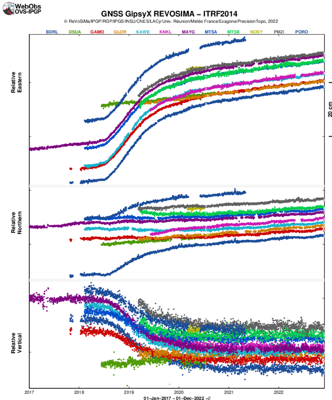
Figure 8 : Déplacements (en cm) enregistrés sur 9 stations GPS localisés à Mayotte (BDRL, GAMO, KAWE, KNKL, MAYG, MTSA, MTSB, PMZI, PORO), 1 station à Grande Glorieuse (GLOB) et 2 stations au nord de Madagascar à Diego Suarez (DSUA) et Nosy Be (NOSY) sur les composantes est (en haut), nord (au milieu) et vertical (en bas) entre le 1 er janvier 2017 et le 30 novembre 2022 pour visualiser une longue série temporelle ante crise. Post-traitement de ces données réalisé par l'IPGP (©OVPF-IPGP / REVOSIMA).
