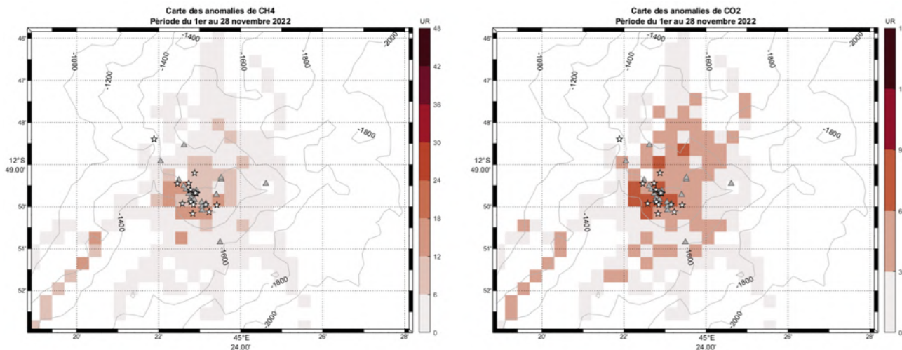
Figure 17 : Carte des anomalies en CH 4 (gauche) et CO 2 (droite) dissous mesurées entre 900 et 1000 m de profondeur par le planeur sous-marin entre le 1 er et le 28 novembre 2022. L'échelle de couleur correspond à l'anomalie maximale en gaz dissous exprimée en unité relative dans des rectangles de 0,5 km 2 . Sont aussi représentées par des étoiles les localisations des panaches acoustiques observés entre 900 et 1000 m de profondeur par le planeur sous-marin entre le 1 er et 28 novembre 2022. Les triangles sont les sites actifs d'émission de fluides identifiés avec le sondeur multifaisceaux coque et des observations visuelles sur site avec un ROV lors des campagnes MAYOBS du REVOSIMA.
