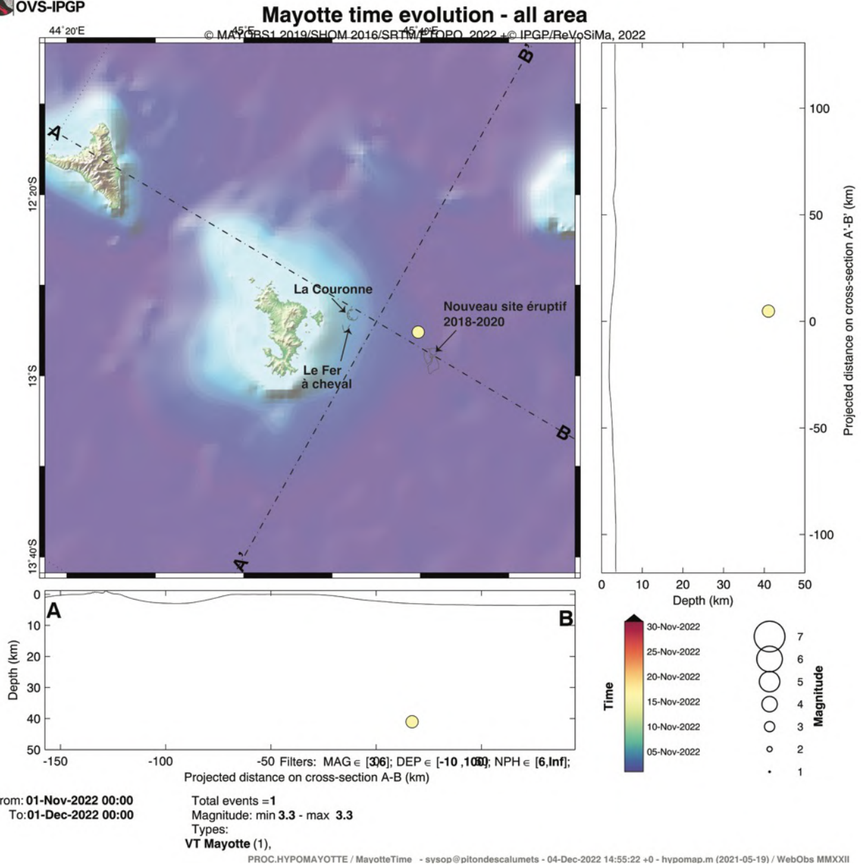
Figure 1c : Carte de localisation des épicentres ( \pm 5 km) des séismes volcano-tectoniques (VT) de magnitude M \geq 3 entre le 1 er et le 30 novembre 2022 enregistrés avec les réseaux sismiques à terre (IPGP-IFREMER-CNRS-BRGM-BCSF-RENAISS, ITES). Sont aussi représentées une projection des hypocentres des séismes le long de coupes transverses et axiales le long de la ride montrant la localisation estimée en profondeur (la précision varie entre \pm 5 km et \pm 15 km) des séismes en fonction de la magnitude (taille des symboles) et de la date (échelle temporelle de couleur). Les structures volcaniques de la zone dite de « La Couronne », du « Fer à cheval » sont indiquées en grisé tout comme les coulées de lave de Fani Maoré. De nombreux points de sortie de panaches de fluides dans la colonne d'eau ont été identifiés dans la structure du Fer à Cheval avec une signature géochimique magmatique (voir section Géochimie des fluides). © OVPF-IPGP, BRGM, IFREMER, CNRS, BCSF-RENAISS, ITES / REVOSIMA).
