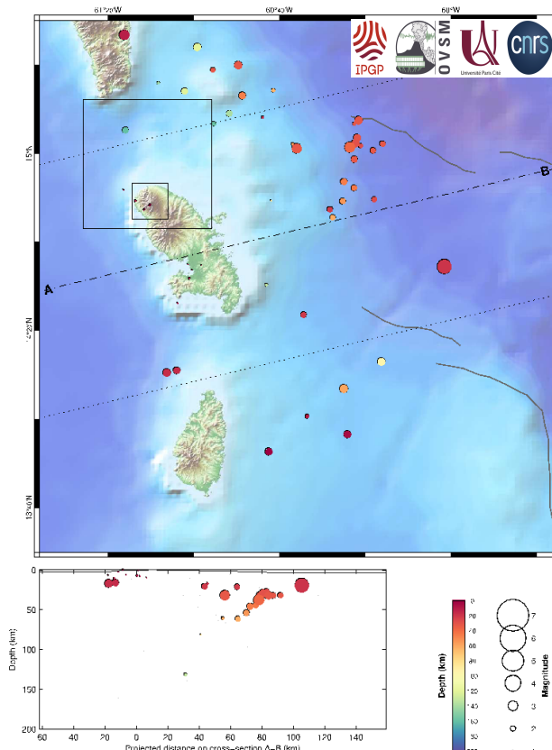
Figure 4. Partie supérieure : carte des hypocentres des séismes enregistrés et localisés par l'OVSM-IPGP au cours du mois de septembre 2022 autour de la Martinique. Partie inférieure : représentation des séismes en profondeur le long du profil A-B.
