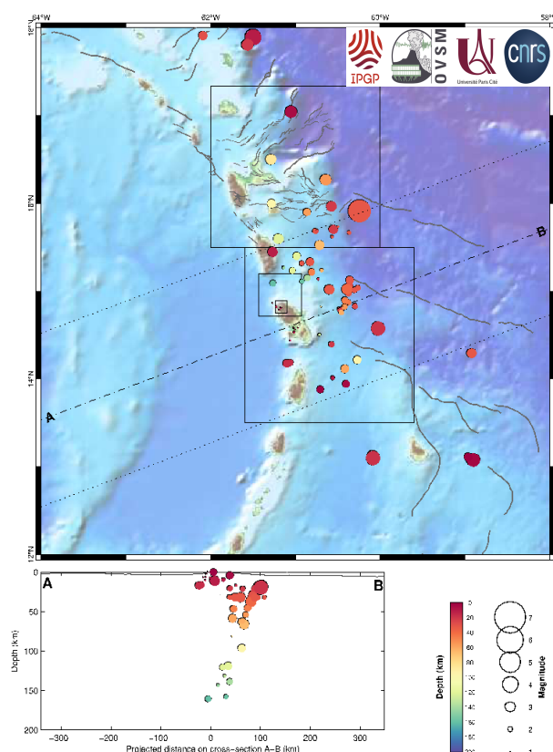
Figure 3. Partie supérieure : carte des hypocentres des séismes enregistrés et localisés par l'OVSM-IPGP au cours du mois de septembre 2022 sur l'arc antillais. Partie inférieure : représentation des séismes en profondeur le long du profil A-B.
