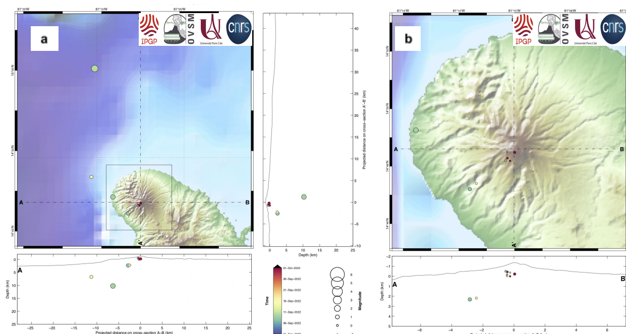
Figure 2. a) Carte de localisation manuelle de la sismicité de la Montagne Pelée au mois de septembre 2022 et coupes est-ouest indiquant la localisation en profondeur des hypocentres. Le séisme représenté en vert au nord de la Martinique est d'origine tectonique et situé à environ 160 km de profondeur. b) zoom sur la Montagne Pelée.
