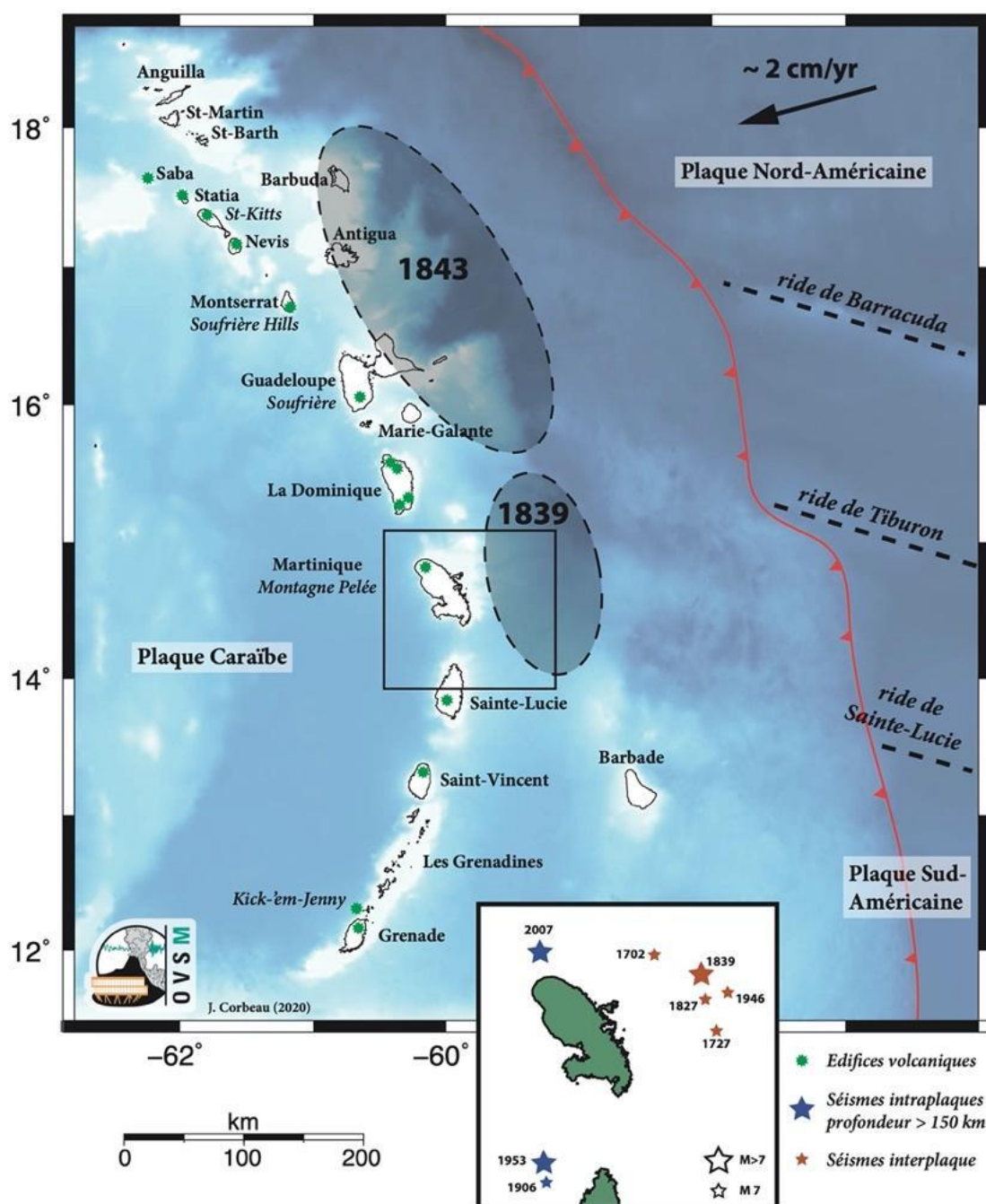
Figure 5. Localisation des séismes historiques de magnitude estimée supérieure à 7. Cette figure illustre aussi la relation entre l'activité tectonique associée à la subduction oblique des plaques Nord-Américaine et Sud-Américaine sous la plaque Caraïbe et l'activité volcanique dans les Petites Antilles. Figure simplifiée d'après Feuillet et al. (2011). Les étoiles vertes correspondent à la localisation des volcans.
