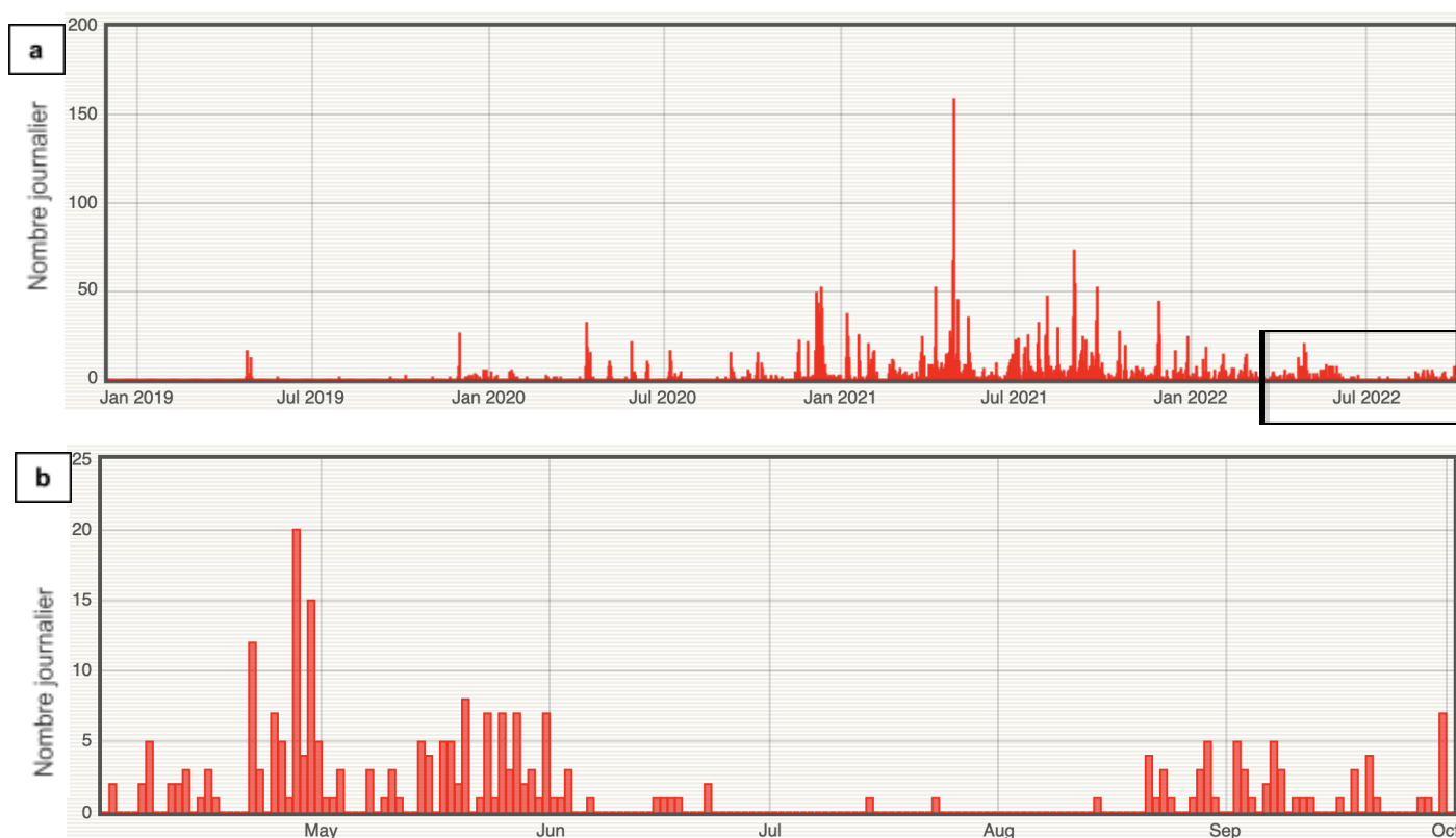
Figure 1. Nombre journalier de séismes de type volcano-tectoniques détectés par l'OVSM : a) Période du 1 er décembre 2018 au 1 er octobre 2022. b) Période des 6 derniers mois (du 1 er avril 2022 au 1 er octobre 2022, zoom sur la figure 1a). Noter que les 5 séismes hybrides et le séisme longue-période enregistrés lors de cette période (Tableau 1) ne sont pas représentés dans la Figure 1b.
