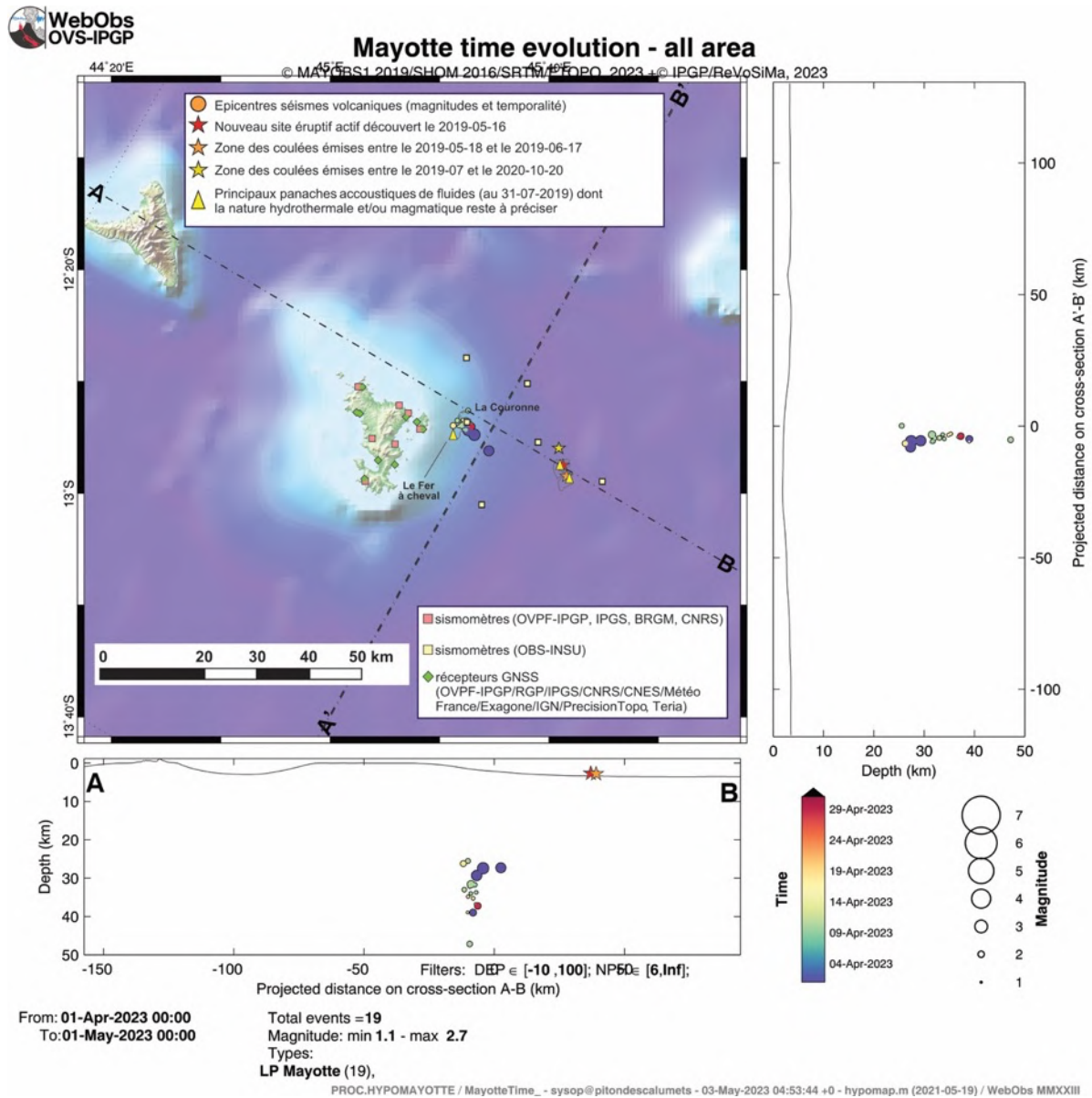
Figure 1b : Carte des épicentres ( \pm 5 km) des séismes longue période (LP) localisés avec les réseaux sismiques à terre (IPGP -CNRS-BRGM-BCSF-RENAISS, ITES) entre le 1 er et 30 avril 2023 (échelle temporelle de couleur). Sont aussi représentées une projection des hypocentres des séismes le long de coupes transverses et axiales le long de la ride montrant la localisation estimée en profondeur (la précision varie entre \pm 5 km et \pm 15 km) des séismes en fonction de la magnitude (taille des symboles et de la date (échelle temporelle de couleur)). La localisation approximative des panaches acoustiques identifiés pendant les campagnes océanographiques (MD220-MAYOBS1, MD221-MAYOBS2, MD222-MAYOBS3, MD223-MAYOBS4, MAYOBS15, MAYOBS17 ; Rinnert et al., 2019) et dont la nature hydrothermale et/ou magmatique reste à préciser, est indiquée par des triangles jaunes, l'étoile rouge indique le site éruptif nouvellement identifié le 16 mai 2019, l'étoile orange la zone des coulées émises entre le 18/05/2019 et le 17/06/2019 et l'étoile jaune la zone des coulées émises entre juillet 2019 et le 18/01/2021. Les structures volcaniques de la zone dite de « La Couronne », du « Fer à cheval » sont indiquées en grisé tout comme les coulées de lave de Fani Maoré. Les stations sismiques du réseau terrestre, les sismomètres fond de mer (OBS) et les stations de positionnement par satellite GPS sont indiquées par des symboles (voir légende). (©OVPF-IPGP, BRGM, IFREMER, CNRS, BCSF-RENAISS, ITES / REVOSIMA).
