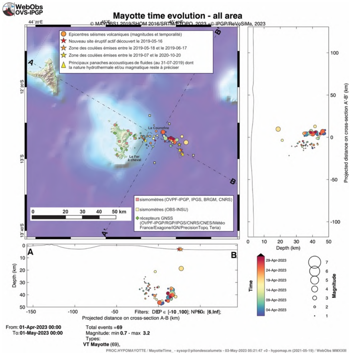
Figure 1a : Carte des épicentres ( \pm 5 km) des séismes volcano-tectoniques (VT) localisés avec les réseaux sismiques à terre (IPGP-CNRS-BRGM-BCSF-RENAISS, ITES) entre le 1 er et 30 avril 2023 (échelle temporelle de couleur). Sont aussi représentées une projection des hypocentres des séismes le long de coupes transversales et axiales le long de la ride montrant la localisation estimée en profondeur (la précision varie entre \pm 5 km et \pm 15 km) des séismes en fonction de la magnitude (taille des symboles et de la date (échelle temporelle de couleur)). La localisation approximative des panaches acoustiques identifiés pendant les campagnes océanographiques (MD220-MAYOBS1, MD221-MAYOBS2, MD222-MAYOBS3, MD223-MAYOBS4, MAYOBS15, MAYOBS17 ; Rinnert et al., 2019) et dont la nature hydrothermale et/ou magmatique reste à préciser, est indiquée par des triangles jaunes, l'étoile rouge indique le site éruptif nouvellement identifié le 16 mai 2019, l'étoile orange la zone des coulées émises entre le 18/05/2019 et le 17/06/2019 et l'étoile jaune la zone des coulées émises entre juillet 2019 et le 18/01/2021. Les structures volcaniques de la zone dite de « La Couronne », du « Fer à cheval » sont indiquées en grisé tout comme les coulées de lave de Fani Maoré. Les stations sismiques du réseau terrestre, les sismomètres fond de mer (OBS) et les stations de positionnement par satellite GPS sont indiquées par des symboles (voir légende). (©OVPF-IPGP, BRGM, IFREMER, CNRS, BCSF-RENAISS, ITES / REVOSIMA).
