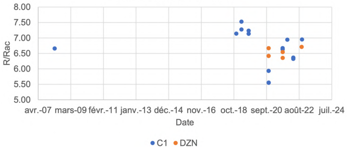
Figure 13 : Analyses isotopiques (gaz rares) des bullages aux points de contrôle C1 (estran de l'aéroport) et DZN (Lac Dziani). Une augmentation du R/Ra (rapport isotopique de l'He normalisé à celui de l'atmosphère) est liée à une augmentation de la contribution des fluides profonds remontant du manteau. Erreur moyenne sur chaque analyse : 0.05 unité.
