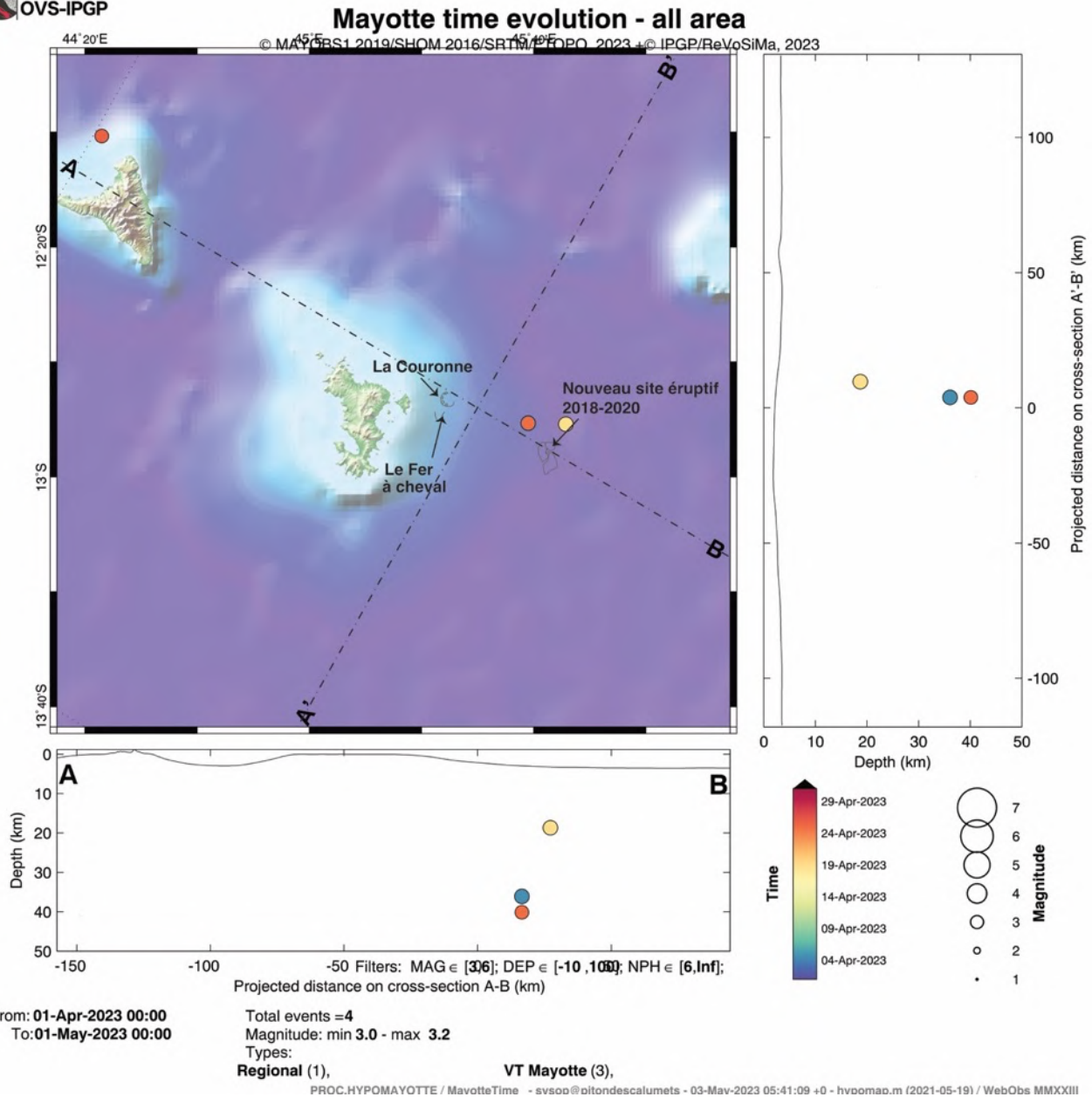
Figure 1c : Carte de localisation des épicentres ( \pm 5 km) des séismes volcano-tectoniques (VT) de magnitude M \geq 3 entre le 1 er et le 30 avril 2023 enregistrés avec les réseaux sismiques à terre (IPGP-IFREMER-CNRS-BRGM-BCSF-RENAISS, ITES). Sont aussi représentées une projection des hypocentres des séismes le long de coupes transverses et axiales le long de la ride montrant la localisation estimée en profondeur (la précision varie entre \pm 5 km et \pm 15 km) des séismes en fonction de la magnitude (taille des symboles) et de la date (échelle temporelle de couleur). Les structures volcaniques de la zone dite de « La Couronne », du « Fer à cheval » sont indiquées en grisé tout comme les coulées de lave de Fani Maoré. De nombreux points de sortie de panaches de fluides dans la colonne d'eau ont été identifiés dans la structure du Fer à Cheval avec une signature géochimique magmatique (voir section Géochimie des fluides). © OVPF-IPGP, BRGM, IFREMER, CNRS, BCSF-RENAISS, ITES / REVOSIMA).
