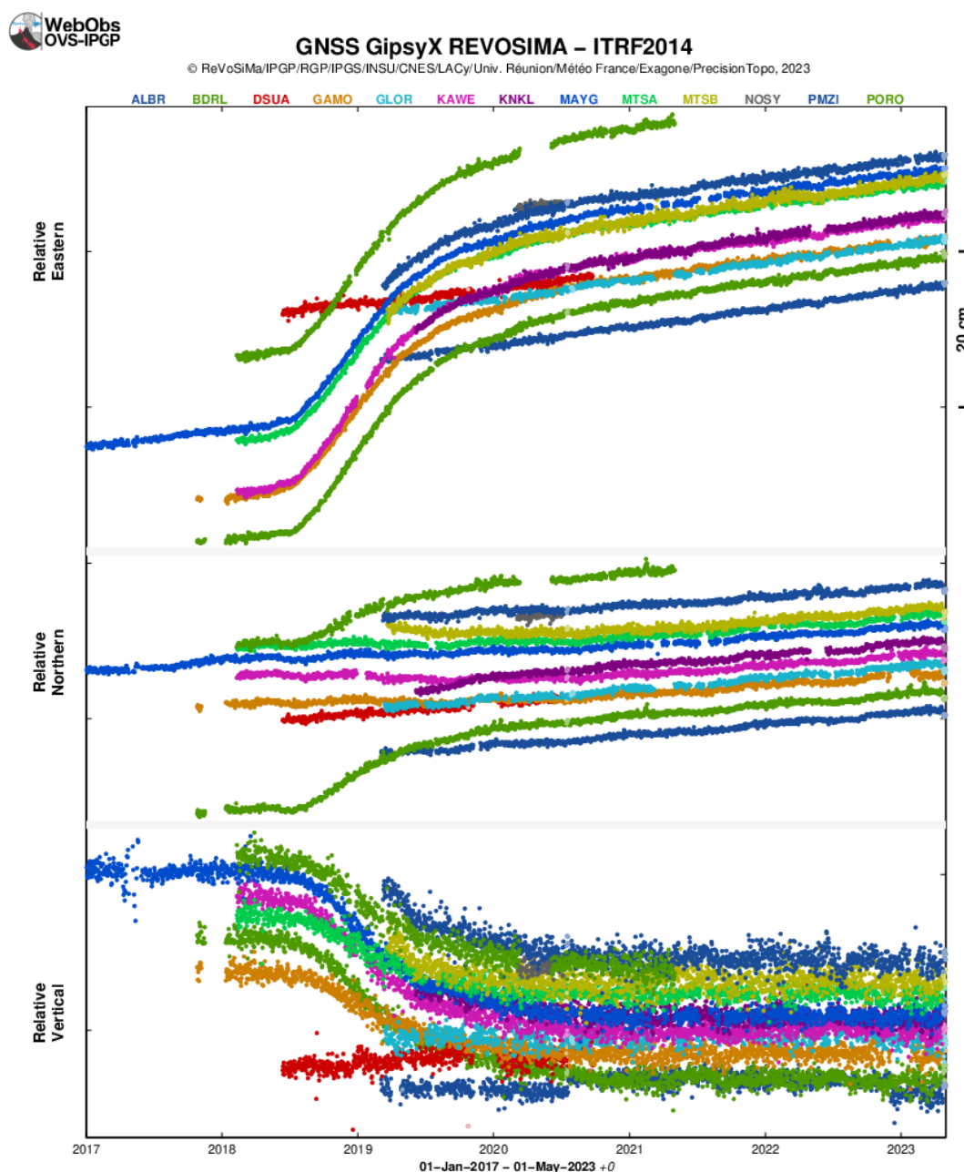
Figure 8 : Déplacements (en cm) enregistrés sur 9 stations GPS localisés à Mayotte (BDRL, GAMO, KAWE, KNKL, MAYG, MTSB, PMZI, PORO), 1 station à Grande Glorieuse (GLOR), 1 station à Aldabra (ALBR) et 2 stations au nord de Madagascar à Diego Suarez (DSUA) et Nosy Be (NOSY) sur les composantes est (en haut), nord (au milieu) et vertical (en bas) entre le 1 er janvier 2017 et le 30 avril 2023 pour visualiser une longue série temporelle ante crise. Post-traitement de ces données réalisé par l'IPGP (©OVPF-IPGP / REVOSIMA).
