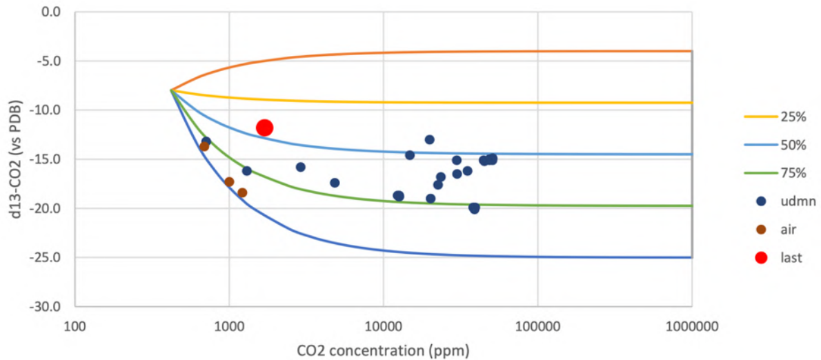
Figure 12 : Variations isotopiques du carbone ( \delta^{13}\text{C}\text{-CO}_2 ) du \text{CO}_2 dans l'air et dans les gaz du sol à la station UDMN. La composition du pôle magmatique est fixée à -4.0 per mil (signature des bullages du site C1 – estran de l'aéroport).
