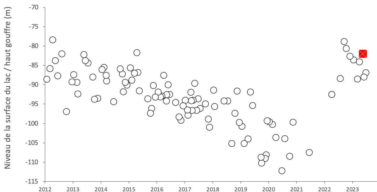
Figure 9. Niveau du lac, ou fond du gouffre Tarissan. Carré rouge : prélèvement de mai 2023 ayant ramené de l'argile uniquement
