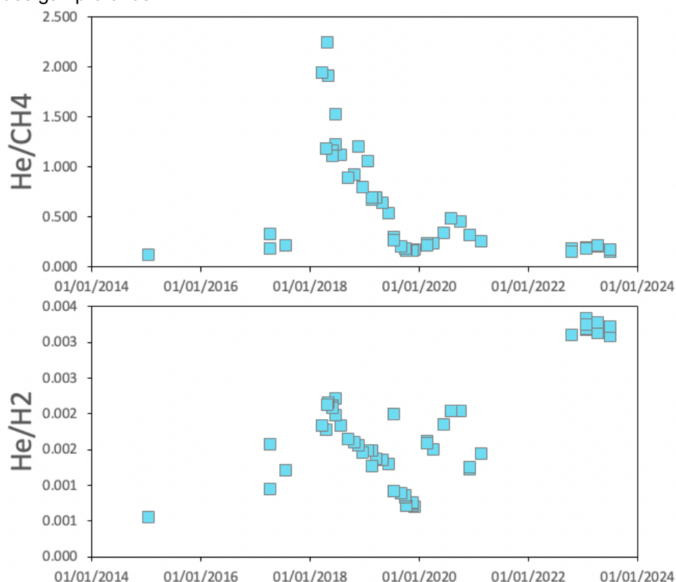
Figure 6. Abondances relatives des gaz non condensables He, H 2 et CH 4 dans les gaz prélevés (ampoule de Giggenbach) à l'évent Napoléon Nord (NAPN).
