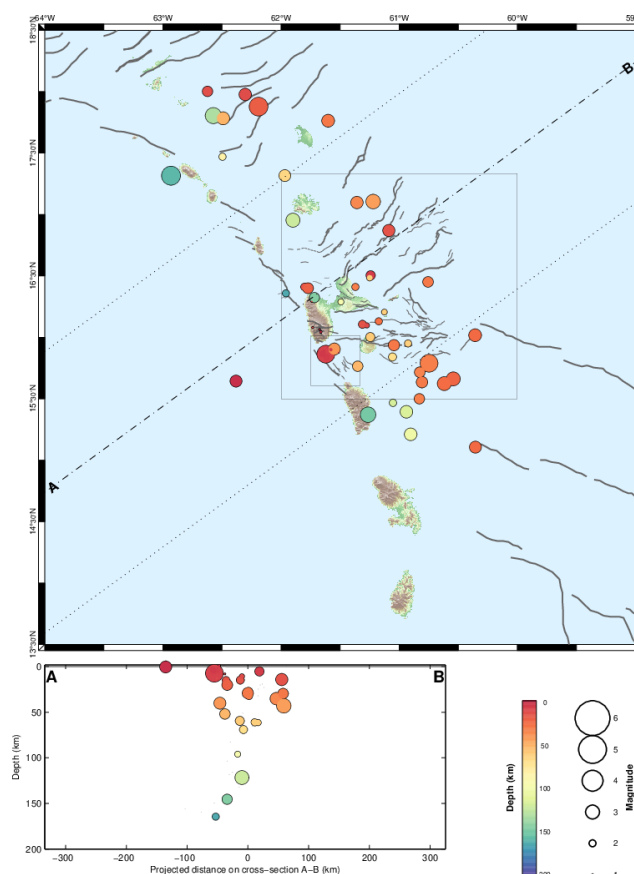
Figure 10. Localisation des épicentres des séismes tectoniques enregistrés au mois de juillet 2023 par l'OVSG-IPGP
