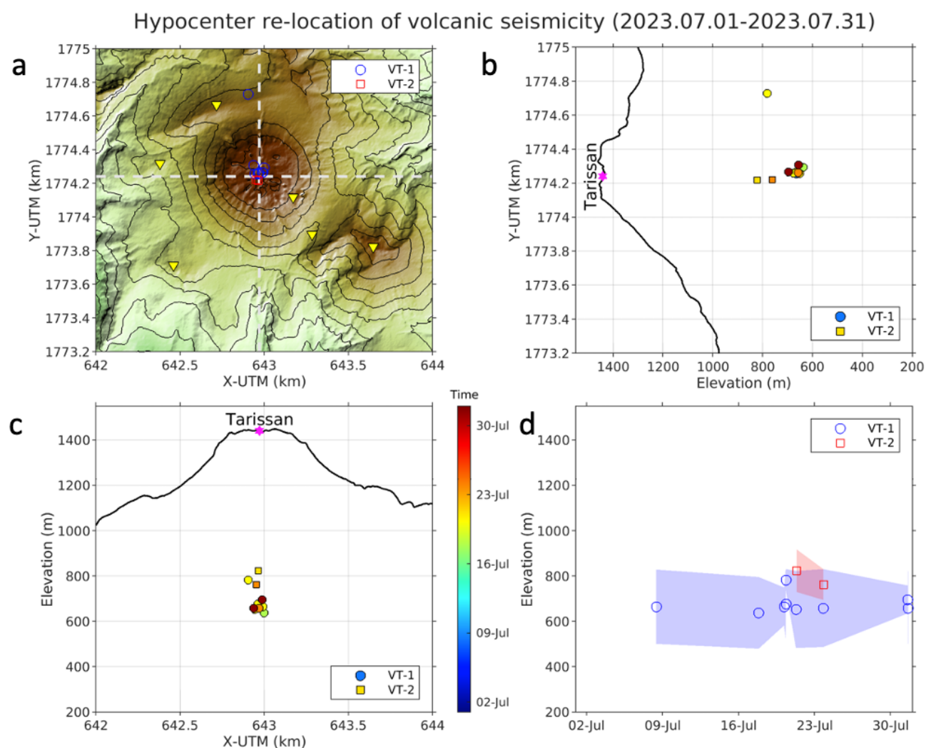
Figure 3. (a) Carte de localisation (épices), (b et c) coupes NS et EO, et (d) évolution temporelle montrant la localisation en profondeur (hypocentres) des séismes VT localisables au mois de juillet 2023 sous le dôme de la Soufrière et le complexe volcanique autour du dôme. (a) Triangles jaunes : localisation des stations sismiques.
