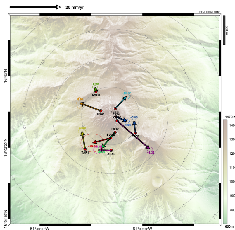
Figure 4. Déformation du dôme de la Soufrière enregistrée par le réseau GNSS permanent entre le 1er août 2022 et le 1er août 2023. La taille de la flèche est proportionnelle au taux de déformation horizontale (en mm par an, selon l'échelle indiquée en haut à gauche). Le chiffre au bout de chaque flèche indique la valeur de la déformation verticale, positif pour une élévation, négatif pour un affaissement. Les ellipses représentent l'incertitude sur la position horizontale de l'extrémité du vecteur horizontal de déformation.
