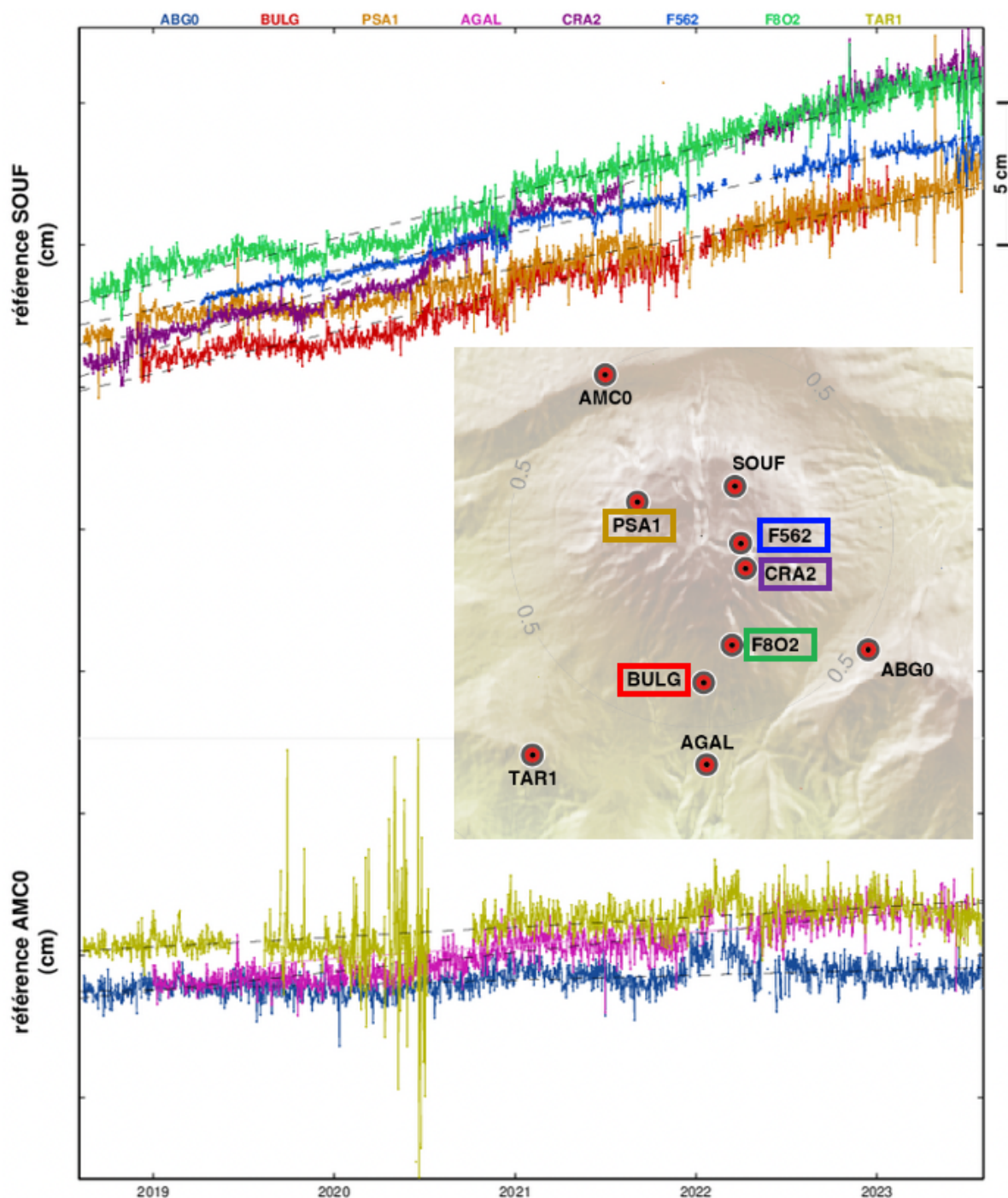
Figure 5. Evolution sur 5 ans des distances séparant les stations GNSS de deux stations de référence. Haut : déplacement des stations localisées au sommet de la Soufrière, relativement à la station SOUF localisée au nord du dôme. Bas : déplacement des stations localisées en périphérie immédiate de la Soufrière, relativement à la station AMC localisée au Nord-Ouest de l'édifice. Centre : localisation des stations GNSS. Les rectangles indiquent les cinq stations dont les distances à SOUF sont rapportées.
