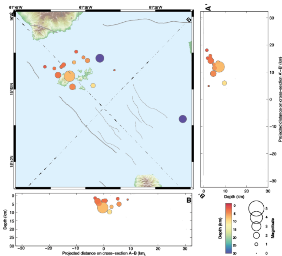
Figure 11. Epicentres des séismes tectoniques localisables, enregistrés au mois de juillet 2023 par l'OVSG-IPGP dans la zone des Saintes.
