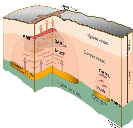
Illustration schématique du système magmatique à l'aplomb de la dorsale Est-Pacifique. © Marjanovic - CNRS-IPGP
