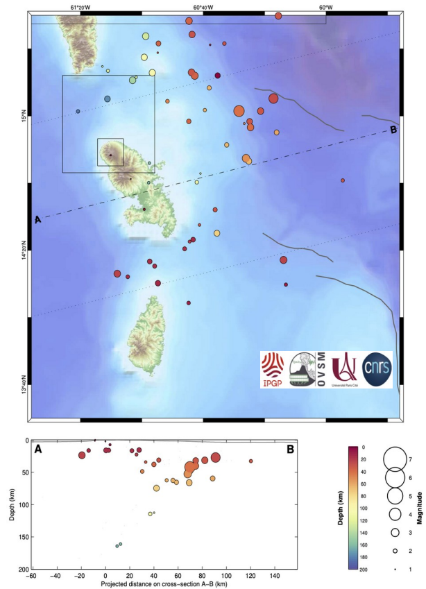
Figure B2. Partie supérieure : carte des hypocentres des séismes enregistrés et localisés par l'OVSM-IPGP au cours du mois d'octobre 2023 autour de la Martinique. Partie inférieure : représentation des séismes en profondeur le long du profil A-B (source WebObs/OVSM).
