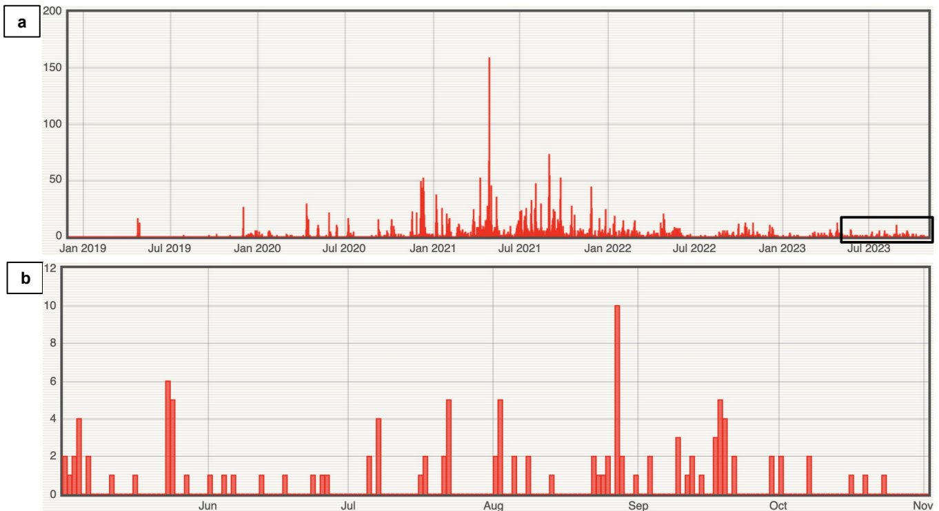
Figure A2. Nombre journalier de séismes de type volcano-tectonique (VT) détectés par l'OVSM-IPGP : a) Période du 1 er décembre 2018 au 31 octobre 2023. b) Période des 6 derniers mois (du 1 er avril 2023 au 31 octobre 2023, zoom sur la sous-figure a). Source WebObs/OVSM.
