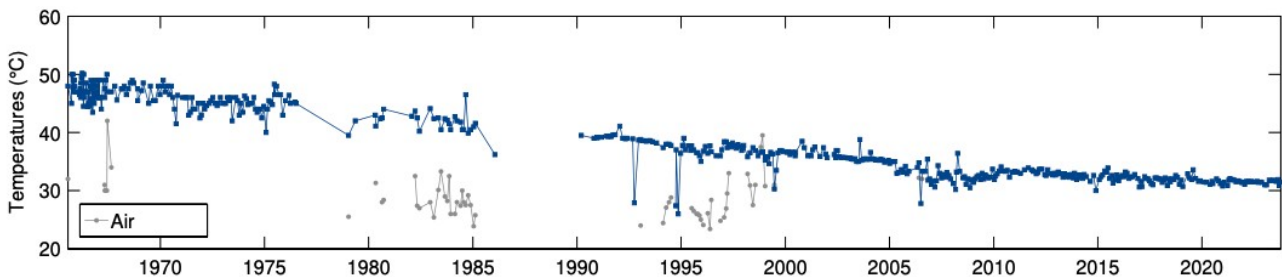
Figure A6. Évolution de la température du forage Puits Chaud (points bleus foncés) de 1965 à octobre 2023 (source WebObs/OVSM).
