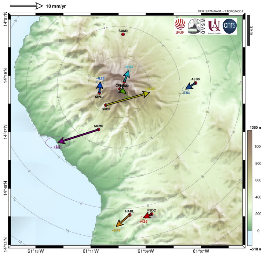
Figure A4. Vecteurs des vitesses moyennes de déformations horizontales mesurées entre le 1er novembre 2022 et le 31 octobre 2023 (un an) sur la Montagne Pelée (échelle donnée par la flèche en haut à gauche en mm par an). Chaque vecteur est associé à une ellipse d'erreur ainsi qu'à une indication de la vitesse verticale (non significative). Les cercles concentriques gris indiquent les distances en km depuis le sommet. Ces vitesses sont calculées de façon relative par rapport à un référentiel local (source WebObs / OVSM).
