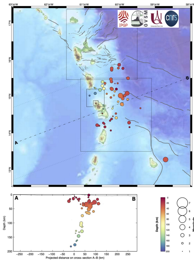
Figure B1. Partie supérieure : carte des hypocentres des séismes enregistrés et localisés par l'OVSM-IPGP au cours du mois d'octobre 2023 sur l'arc antillais. Partie inférieure : représentation des séismes en profondeur le long du profil A-B (source WebObs/OVSM).
