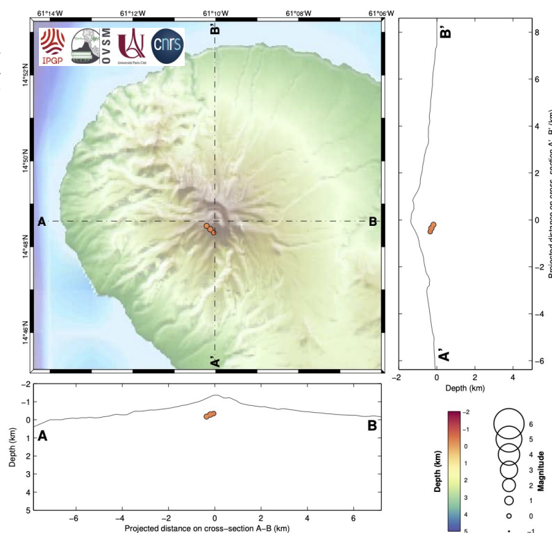
Figure A1. Carte de localisation manuelle de la sismicité d'origine volcanique du mois d'octobre 2023, et coupes est-ouest et nord-sud indiquant la localisation en profondeur des hypocentres (source WebObs/OVSM).
