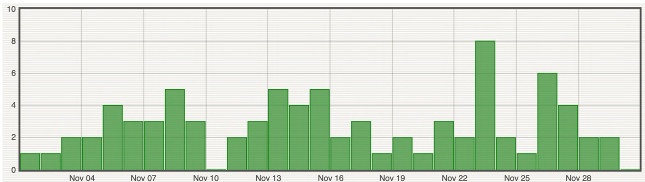
Figure 9 : Histogramme représentant le nombre de séismes locaux (Ile de La Réunion) par jour enregistrés en novembre 2023 (© OVPF-IPGP).
