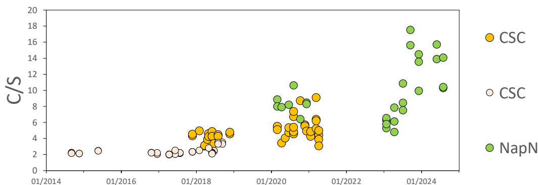
Figure 8: Évolution du rapport molaire Carbon / Soufre dans le gaz total prélevé à l'aide d'ampoules à soude. CSC : Cratère Sud Centre. NapN : Napoléon Nord.
