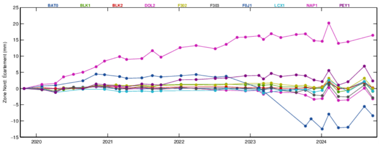
Figure 6. Évolution de l'écartement des failles entre 2020 et septembre 2024.
