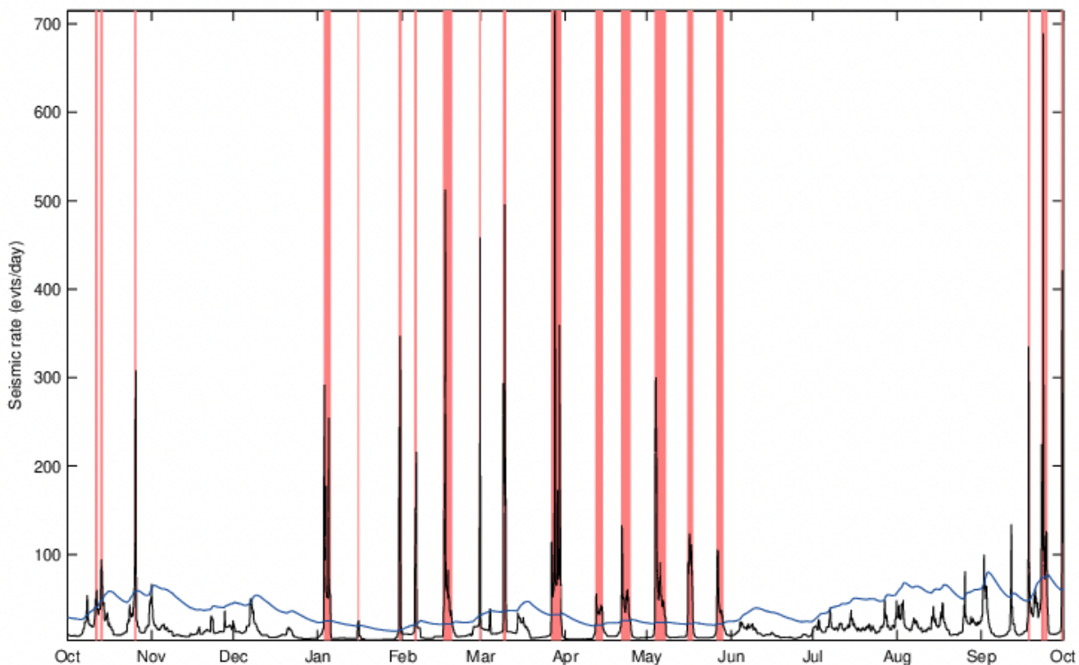
Figure 2. Taux instantané de sismicité volcano-tectonique (VT) entre le 1 er octobre 2023 et le 1 er octobre 2024. Les bandes rouges caractérisent les essaims sismiques (voir les définitions de ces paramètres en annexe).
