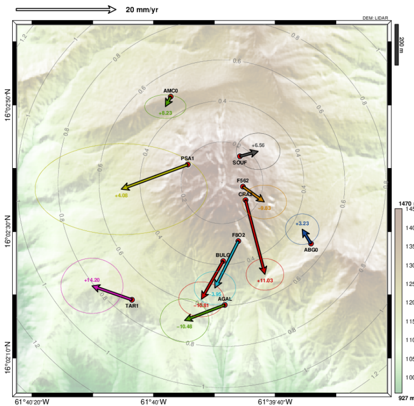
Figure 4. Déformation du dôme de la Soufrière enregistrée par le réseau GNSS permanent entre le 1er octobre 2023 et le 1er octobre 2024. La taille de la flèche et la valeur indiquée en haut à gauche indiquent le taux de déformation horizontale en mm par an. Le chiffre au bout de chaque flèche indique la valeur de la déformation verticale, positif pour une élévation, négatif pour un affaissement. Les ellipses représentent l'incertitude sur la position horizontale de l'extrémité du vecteur de déformation.
