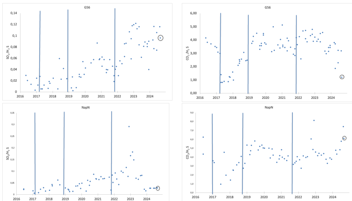
Figure 9: Évolution des rapports SO_2/H_2S et CO_2/H_2S dans les panaches de gaz émis par les événements CS (Cratère Sud), G56 (Gouffre 56) et Napoléon Nord (NAPN). Le site CS comprend un événement nord (CSN) et plusieurs événements sud (CSS). La bouche principale de CSS (flèches), la plus au nord et donc la plus proche de CSN, a la même composition que CSN. Les lignes bleues marquent des changements de compositions chimiques observées sur la plupart des sites (Mars 2017; Décembre 2018; Octobre 2021). Les cercles noirs indiquent les dernières mesures effectuées le 5/09/2024.
