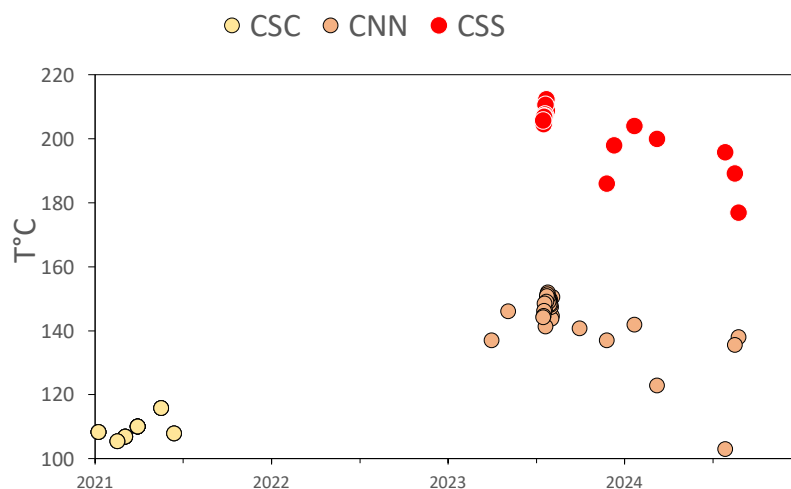
Figure 7 : Evolution 2021-2024 de la température des fumerolles de la fissure Cratère Sud (CSC : Cratère Sud Centre, inactif depuis 2021 ; CSN : Cratère Sud Nord ; CSS : Cratère Sud Sud)
