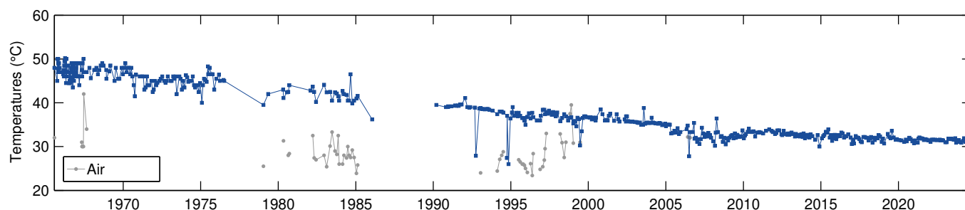
Figure 6 – Évolution de la température du forage Puits Chaud (points bleus foncés) de 1965 à septembre 2024 (mesures manuelles mensuelles, source WebObs/OVSM).
