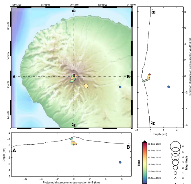
Figure 2 – Sismicité d'origine volcanique du mois de septembre 2024 ayant pu être localisée au niveau de la partie superficielle de la Montagne Pelée, et coupes est-ouest et nord-sud indiquant la localisation en profondeur des hypocentres (source WebObs/OVSM).
