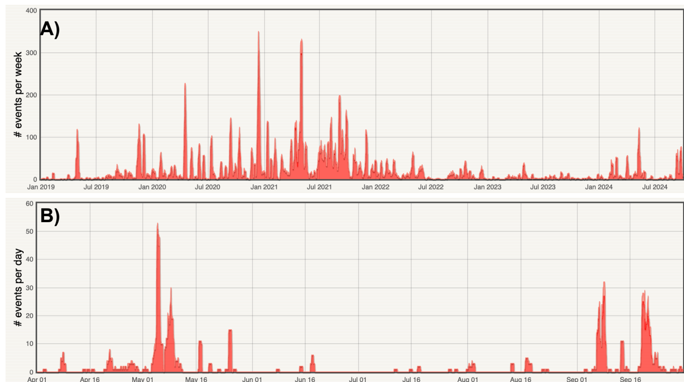
Figure 3 – Taux de sismicité pour les événements de type volcano-tectonique (rouge) et volcano-tectonique emboîtés (rose) détectés par l'OVSM-IPGP : A) Nombre par semaine du 1 er janvier 2019 au 30 septembre 2024. B) Nombre par jour durant les 6 derniers mois (du 1 er Avril 2024 au 30 septembre 2024). Source WebObs/OVSM.
