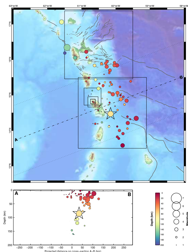
Figure 8 – Partie supérieure : carte des hypocentres des séismes enregistrés et localisés par l'OVSM-IPGP au cours du mois de septembre 2024 sur l'arc antillais. La présence d'une étoile indique un séisme ressenti. Partie inférieure : représentation des séismes en profondeur le long du profil A-B (source WebObs/OVSM).
