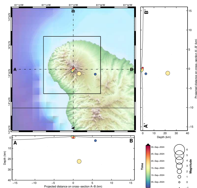
Figure 1 – Carte de localisation manuelle de la sismicité d'origine volcanique du mois de septembre 2024, et coupes est-ouest et nord-sud indiquant la localisation en profondeur des hypocentres (source WebObs/OVSM).
