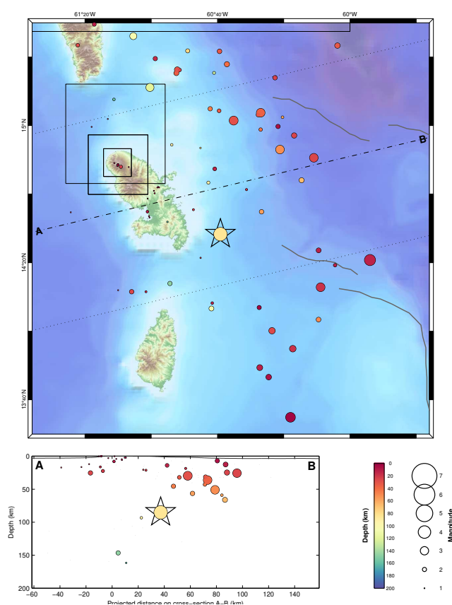
Figure 9 – Partie supérieure : carte des hypocentres des séismes enregistrés et localisés par l'OVSM-IPGP au cours du mois de septembre 2024 autour de la Martinique. La présence d'une étoile indique un séisme ressenti. Partie inférieure : représentation des séismes en profondeur le long du profil A-B (source WebObs/OVSM).
