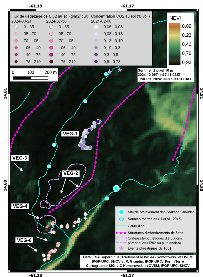
Figure 6 – Suivi du dépérissement de la végétation sur le flanc sud-ouest de la Montagne Pelée par la cartographie de l'indice NDVI à partir d'imagerie satellitale. Cette image du 09 octobre 2024 (Sentinel-2) a été traitée pour montrer l'indice NDVI qui varie entre 0 (absence de végétation) et 1. La végétation saine se caractérise par un indice NDVI > 0,6. Le dépérissement de la végétation peut être un traceur du dégazage passif de CO 2 dans le sol. Les mesures du flux de dégazage diffus de CO 2 (en g/m 2 /jour) au sol réalisées avec la chambre d'accumulation West Systems le 21 mars 2024 et le 30 juillet 2024 sont indiquées, respectivement, par des diamants et des cercles dans la gamme de couleur blanc-rose-magenta. Les zones dont le flux est > 25 g/m 2 /jour indiquent des flux de CO 2 qui comportent nécessairement une composante non-biogénique qui est d'origine volcanique et donc magmatique. Les cercles dans la gamme de couleur du blanc au violet foncé montrent les mesures de la concentration (en ppm) du dégazage diffus du CO 2 mesurées avec un détecteur Dräger le 8 février 2021. Ces premières mesures avaient atteint une valeur maximale de 7800 ppm très largement supérieure à la concentration du CO 2 dans l'atmosphère. Traitement imagerie NDVI : J-C Komorowski et OVSM-IPGP, UPC, SNOV (INSU-CNRS) et R. Grandin, IPGP-UPC, FormaTerre (INSU-CNRS). Cartographie SIG : J-C Komorowski et OVSM-IPGP, UPC, SNOV (INSU-CNRS). Données CO 2 : A. Andrieu, F. Jadelus, D. Melezan, J-G Gabriel, J-C Komorowski, OVSM-IPGP.
