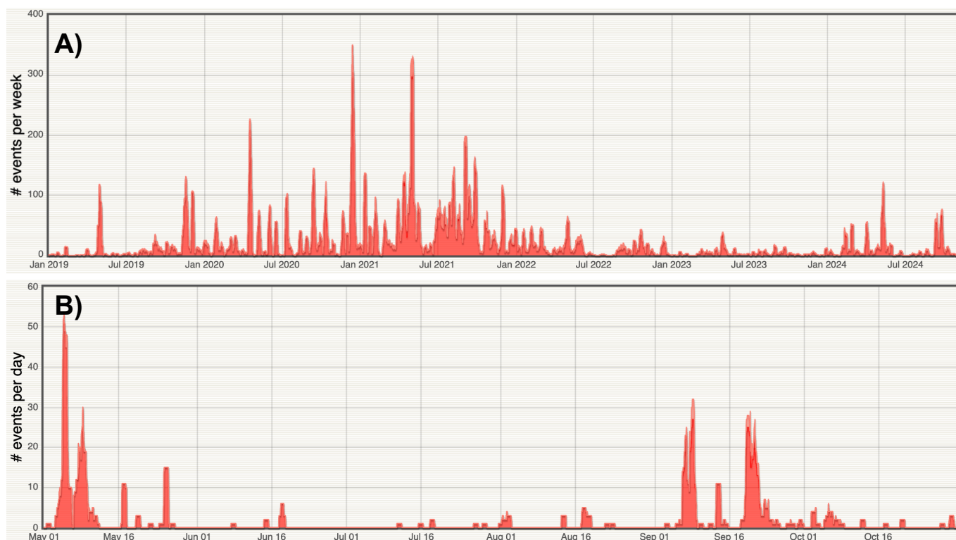
Figure 2 – Taux de sismicité pour les événements de type volcano-tectonique (rouge) et volcano-tectonique emboîtés (rose) détectés par l'OVSM-IPGP : A) Nombre par semaine du 1 er janvier 2019 au 31 octobre 2024. B) Nombre par jour durant les 6 derniers mois (du 1 er mai 2024 au 31 octobre 2024). Source WebObs/OVSM.
