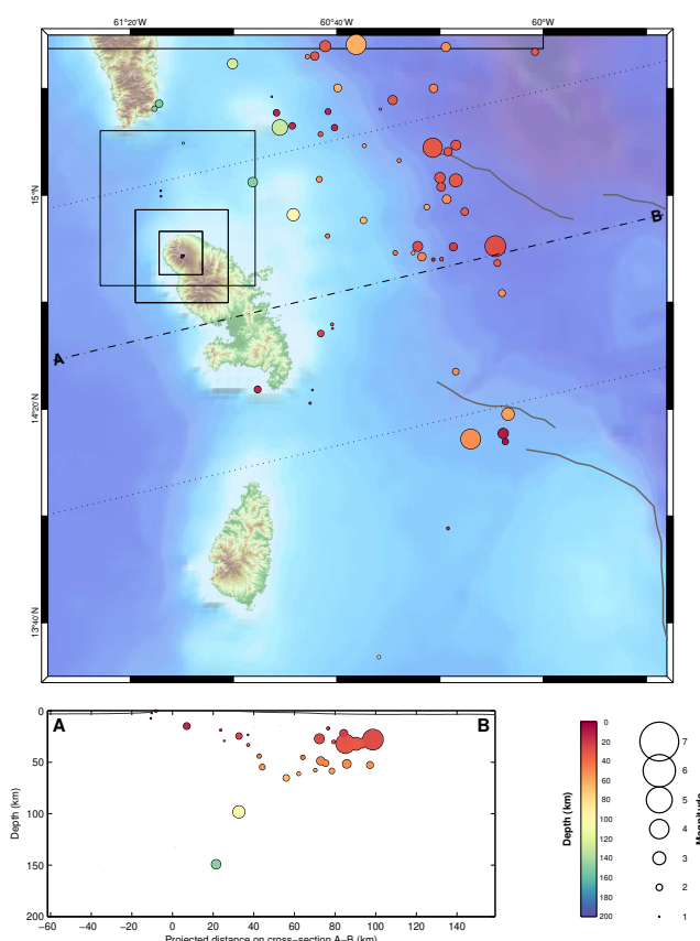
Figure 8 – Partie supérieure : carte des hypocentres des séismes enregistrés et localisés par l'OVSM-IPGP au cours du mois d'octobre 2024 autour de la Martinique. La présence d'une étoile indique un séisme ressenti. Partie inférieure : représentation des séismes en profondeur le long du profil A-B (source WebObs/OVSM).
