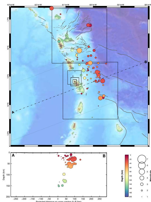
Figure 7 – Partie supérieure : carte des hypocentres des séismes enregistrés et localisés par l'OVSM-IPGP au cours du mois d'octobre 2024 sur l'arc antillais. La présence d'une étoile indique un séisme ressenti. Partie inférieure : représentation des séismes en profondeur le long du profil A-B (source WebObs/OVSM).
