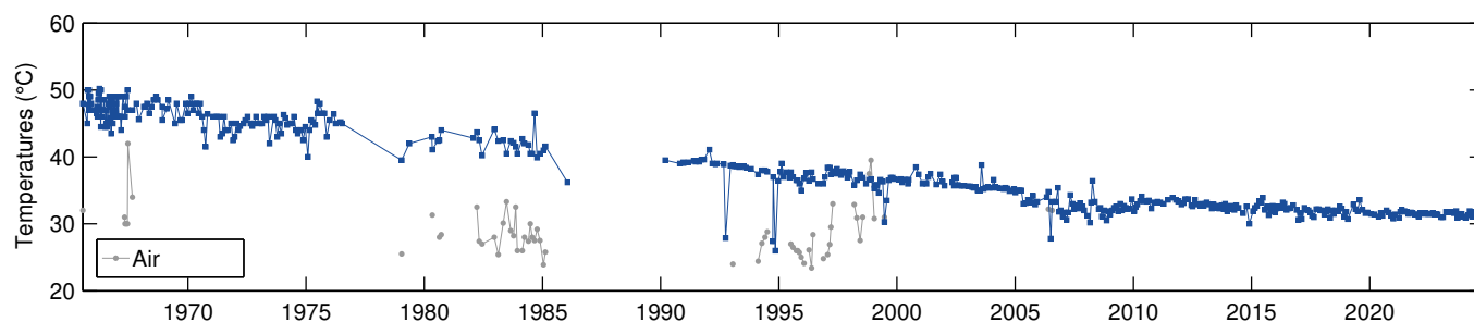
Figure 5 – Évolution de la température du forage Puits Chaud (points bleus foncés) de 1965 à octobre 2024 (mesures manuelles mensuelles, source WebObs/OVSM).
