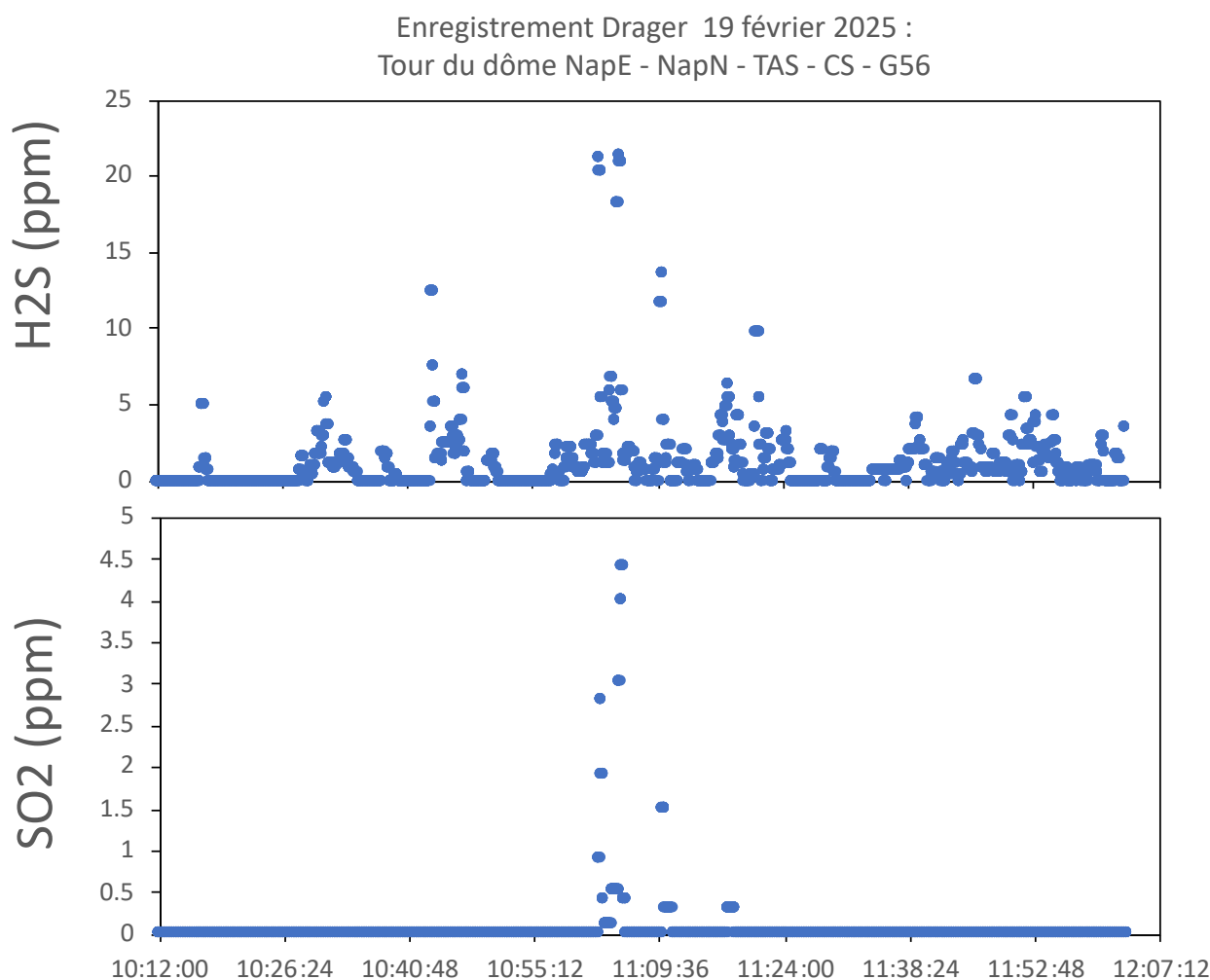
Figure 6 : Concentrations des gaz dans l'air du sommet, enregistré par microanalyseur Dräger lors d'une visite au sommet le 19 février 2025.
