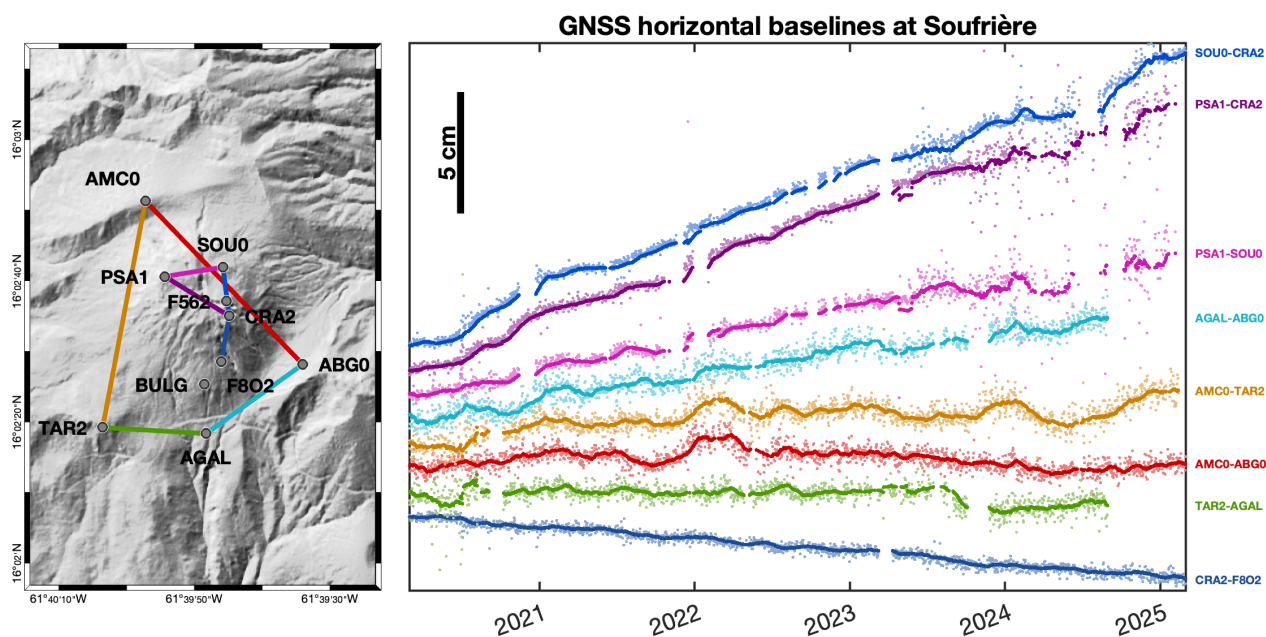
Figure 5. Evolution sur 5 an (1er mars 2020 - 1er mars 2025) des distances séparant les stations GNSS permanentes localisées sur le volcan de la Soufrière.
