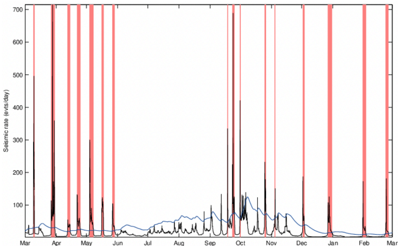
Figure 2. Taux instantané de sismicité volcano-tectonique (VT) entre le 1 er Mars 2024 et le 1 er Mars 2025 (courbe noire). Les bandes rouges caractérisent les essaims sismiques (voir les définitions de ces paramètres en annexe). Taux moyen de sismicité sur les 60 jours précédents (courbe bleue, figée pendant les essaims).
