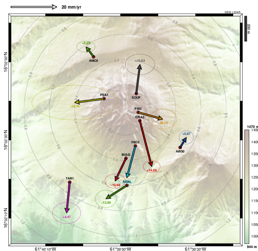
Figure 4. Déformation du dôme de la Soufrière enregistrée par le réseau GNSS permanent entre le 1er mars 2024 et le 1er mars 2025. La taille de la flèche et la valeur indiquée en haut à gauche indiquent le taux de déformation horizontale en mm par an. Le chiffre au bout de chaque flèche indique la valeur de la déformation verticale, positif pour une élévation, négatif pour un affaissement. Les ellipses représentent l'incertitude sur la position horizontale de l'extrémité du vecteur de déformation.
