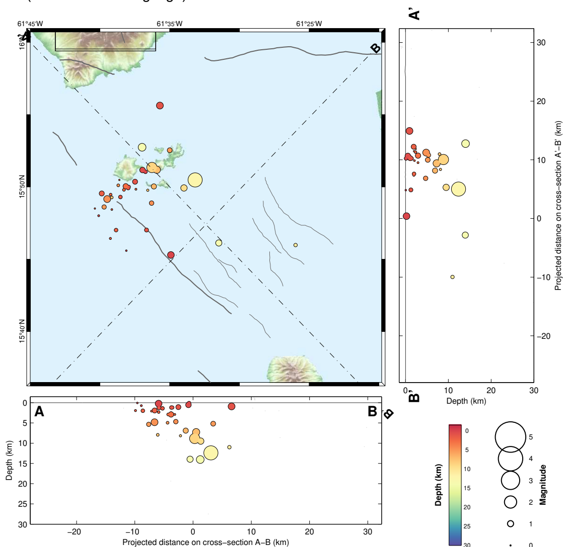
Figure 8. Épicentres des séismes tectoniques localisables, enregistrés au mois de février 2025 par l'OVSG-IPGP dans la zone des Saintes.
