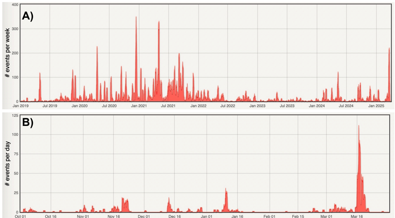
Figure 3 – Taux de sismicité pour les événements de type volcano-tectonique (rouge) et volcano-tectonique emboîtés (rose) détectés par l'OVSM-IPGP : A) Nombre par semaine du 1 er janvier 2019 au 31 mars 2025. B) Nombre par jour durant les 6 derniers mois (du 1 er octobre 2024 au 31 mars 2025). Source WebObs/OVSM.
