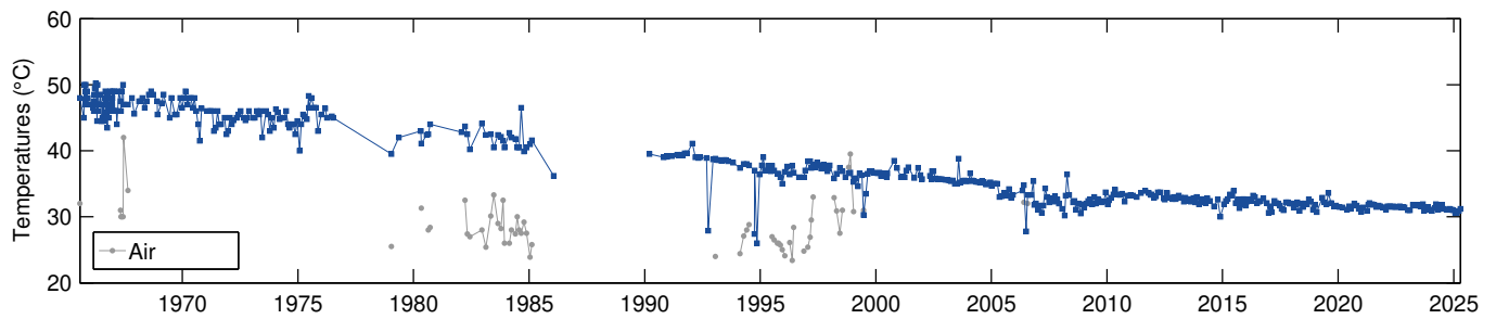
Figure 6 – Évolution de la température du forage Puits Chaud (points bleus foncés) de 1965 à mars 2025 (mesures manuelles mensuelles, source WebObs/OVSM).
