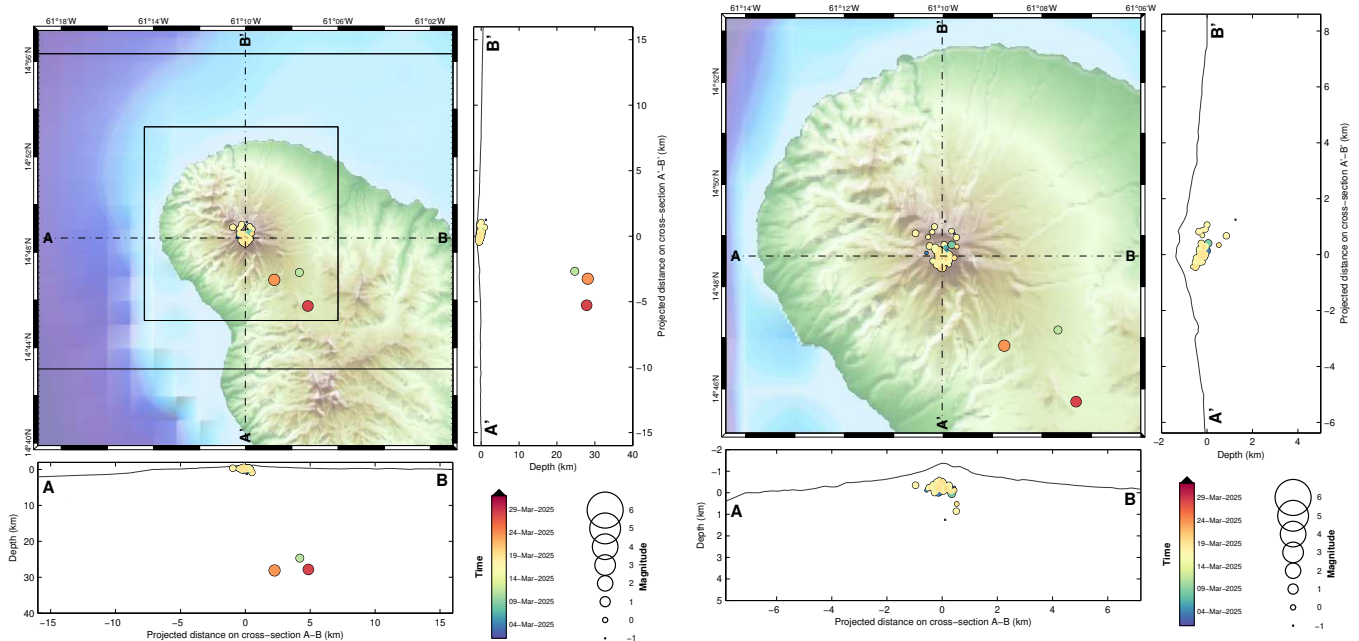
Figure 2 – Sismicité d'origine volcanique du mois de mars 2025 ayant pu être localisée au niveau de la partie superficielle de la Montagne Pelée, et coupes est-ouest et nord-sud indiquant la localisation en profondeur des hypocentres (source WebObs/OVSM).
