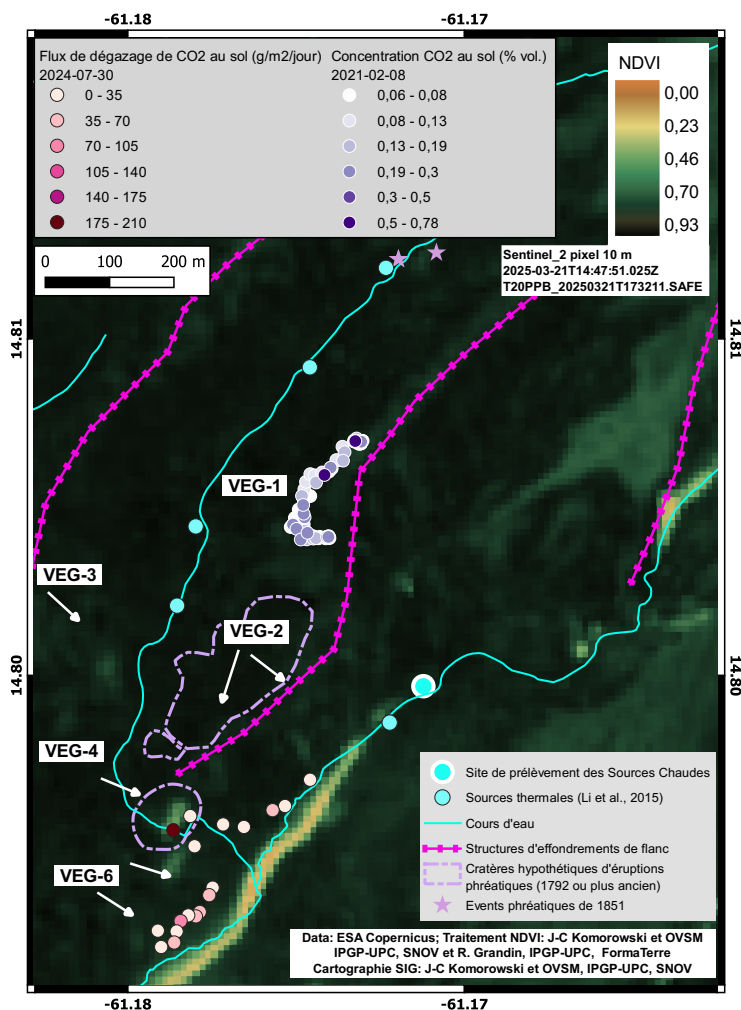
Figure 7 – Suivi du dépérissement de la végétation sur le flanc sud-ouest de la Montagne Pelée par la cartographie de l'indice NDVI à partir d'imagerie satellitale. Cette image du 21 mars 2025 (Sentinel-2) a été traitée pour montrer l'indice NDVI qui varie entre 0 (absence de végétation) et 1 (végétation saine). Les mesures du flux de dégazage diffus de CO 2 (en g/m 2 /jour) au sol réalisées avec la chambre d'accumulation West Systems le 30 juillet 2024 sont indiquées par des cercles dans la gamme de couleur blanc-rose-magenta. Les zones dont le flux est > 25 g/m 2 /jour indiquent des flux de CO 2 qui comportent nécessairement une composante non-biogénique qui est d'origine volcanique et donc magmatique. Les cercles dans la gamme de couleur du blanc au violet foncé montrent les mesures de la concentration (en ppm) du dégazage diffus du CO 2 mesurées avec un détecteur Dräger le 8 février 2021. Ces premières mesures avaient atteint une valeur maximale de 7800 ppm très largement supérieure à la concentration du CO 2 dans l'atmosphère. Traitement imagerie NDVI : J Corbeau et J-C Komorowski, OVSM-IPGP, UPC, SNOV (INSU-CNRS) et R. Grandin, IPGP-UPC, FormaTerre (INSU-CNRS). Cartographie SIG : J. Corbeau et J-C Komorowski, OVSM-IPGP, UPC, SNOV (INSU-CNRS). Données CO 2 : A. Andrieu, F. Jadelus, D. Melezan, J-G Gabriel, J-C Komorowski, OVSM-IPGP.
