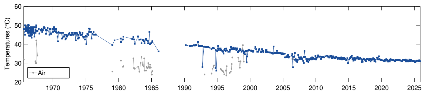
Figure 8 – Évolution de la température du forage Puits Chaud (points bleus foncés) de 1965 à novembre 2025 (mesures manuelles mensuelles, source WebObs/OVSM).
