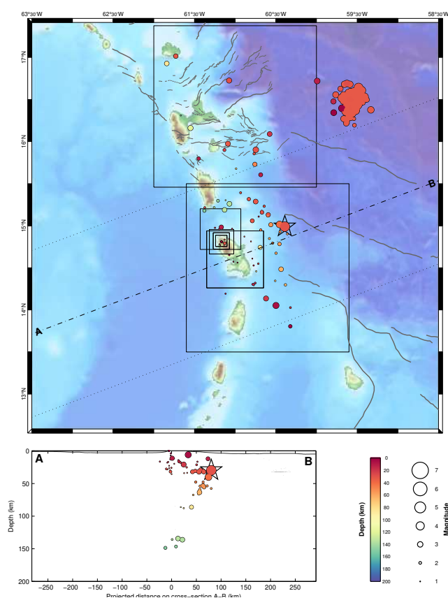
Figure 10 – Partie supérieure : carte des hypocentres des séismes enregistrés et localisés par l'OVSM-IPGP au cours du mois de novembre 2025 sur l'arc antillais. La présence d'une étoile indique un séisme ressenti. Partie inférieure : représentation des séismes en profondeur le long du profil A-B et situés dans la zone comprises entre les deux lignes en pointillé (source WebObs/OVSM).
