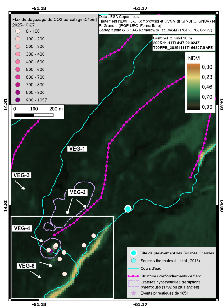
Figure 9 – Suivi du dépérissement de la végétation sur le flanc sud-ouest de la Montagne Pelée par la cartographie de l'indice NDVI à partir d'imagerie satellitaire. (Gauche) Cette image du 11 novembre 2025 (Sentinel-2) a été traitée pour montrer l'indice NDVI qui varie entre 0 (absence de végétation) et 1 (végétation saine). Les mesures du flux de dégazage diffus de CO 2 (en g/m 2 /jour) au sol réalisées avec la chambre d'accumulation West Systems le 14 octobre 2025 sont indiquées par des cercles dans la gamme de couleur blanc-rose-magenta. Les zones dont le flux est > 25 g/m 2 /jour indiquent des flux de CO 2 qui comportent nécessairement une composante non-biogénique qui est d'origine volcanique et donc magmatique. (Droite) Agrandissement des zones VEG-4 et VEG-6 encadrées en blanc sur la carte principale. Traitement imagerie NDVI : J Corbeau et J-C Komorowski, OVSM-IPGP, UPC, SNOV (INSU-CNRS) et R. Grandin, IPGP-UPC, FormaTerre (INSU-CNRS). Cartographie SIG : J. Corbeau et J-C Komorowski, OVSM-IPGP, UPC, SNOV (INSU-CNRS). Données CO 2 : T. Abauzit, F. Jadelus, D. Melezan, OVSM-IPGP.
