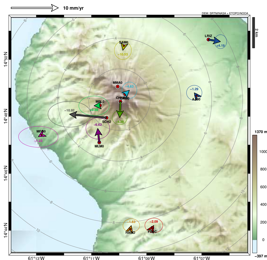
Figure 6 – Vecteurs des vitesses moyennes de déformations horizontales mesurées entre le 1 er décembre 2023 et le 30 novembre 2025 (deux ans) sur la Montagne Pelée (échelle donnée par la flèche en haut à gauche en mm par an). Chaque vecteur est associé à une ellipse d'erreur ainsi qu'à une indication de la vitesse verticale (non significative). Ces vitesses sont calculées de façon relative par rapport à un référentiel local et les ellipses d'erreur sont évaluées par rapport à l'écart-type des données relatifs à une tendance linéaire. Les cercles concentriques gris indiquent les distances en km depuis le sommet (calculs préliminaires. Source WebObs / OVSM).
