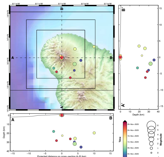
Figure 1 – Carte de localisation manuelle de la sismicité d'origine volcanique du mois de novembre 2025, et coupes est-ouest et nord-sud indiquant la localisation en profondeur des hypocentres (source WebObs/OVSM).
