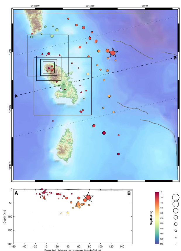
Figure 11 – Partie supérieure : carte des hypocentres des séismes enregistrés et localisés par l'OVSM-IPGP au cours du mois de novembre 2025 autour de la Martinique. La présence d'une étoile indique un séisme ressenti. Partie inférieure : représentation des séismes en profondeur le long du profil A-B et situés dans la zone comprises entre les deux lignes en pointillé (source WebObs/OVSM).
