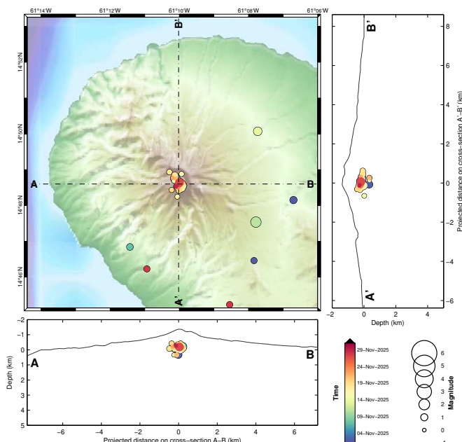
Figure 2 – Sismicité d'origine volcanique du mois de novembre 2025 ayant pu être localisée au niveau de la partie superficielle de la Montagne Pelée, et coupes est-ouest et nord-sud indiquant la localisation en profondeur des hypocentres (source WebObs/OVSM).
