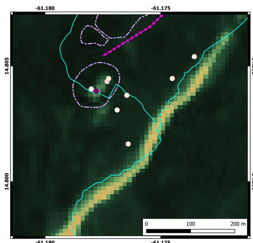
Figure 9 – Suivi du dépérissement de la végétation sur le flanc sud-ouest de la Montagne Pelée par la cartographie de l'indice NDVI à partir d'imagerie satellitaire. (Gauche) Cette image du 11 novembre 2025 (Sentinel-2) a été traitée pour montrer l'indice NDVI qui varie entre 0 (absence de végétation) et 1 (végétation saine). Les mesures du flux de dégazage diffus de CO 2 (en g/m 2 /jour) au sol réalisées avec la chambre d'accumulation West Systems le 14 octobre 2025 sont indiquées par des cercles dans la gamme de couleur blanc-rose-magenta. Les zones dont le flux est > 25 g/m 2 /jour indiquent des flux de CO 2 qui comportent nécessairement une composante non-biogénique qui est d'origine volcanique et donc magmatique. (Droite) Agrandissement des zones VEG-4 et VEG-6 encadrées en blanc sur la carte principale. Traitement imagerie NDVI : J Corbeau et J-C Komorowski, OVSM-IPGP, UPC, SNOV (INSU-CNRS) et R. Grandin, IPGP-UPC, FormaTerre (INSU-CNRS). Cartographie SIG : J. Corbeau et J-C Komorowski, OVSM-IPGP, UPC, SNOV (INSU-CNRS). Données CO 2 : T. Abauzit, F. Jadelus, D. Melezan, OVSM-IPGP.
