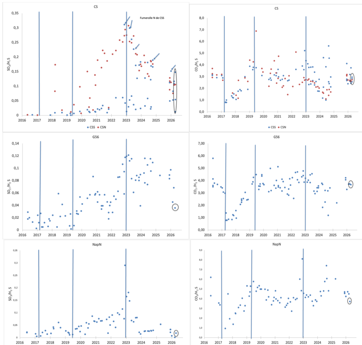
Figure 6 : Évolution des rapports SO_2/H_2S et CO_2/H_2S dans les panaches de gaz émis par les événements CS (Cratère Sud), G56 (Gouffre 56) et Napoléon Nord (NAPN). Le site CS comprend un événement nord (CSN) et plusieurs événements sud (CSS). La bouche principale de CSS (flèches), la plus au nord et donc la plus proche de CSN, a la même composition que CSN. Les lignes bleues marquent des changements de compositions chimiques observées sur la plupart des sites (Mars 2017; Mai 2019; Jan 2023). Les cercles noirs indiquent les dernières mesures effectuées le 22/04/2026.
