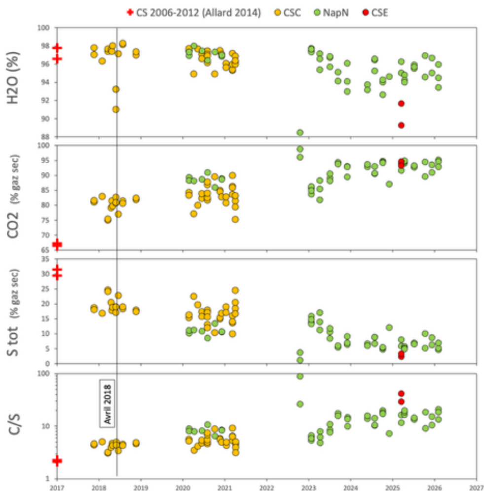
Figure 7. Évolution de la composition du gaz total prélevé à l'aide d'ampoules à soude. Les derniers échantillons de gaz total analysés datent du 5 février 2026.
