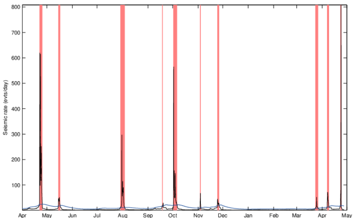
Figure 2. Taux instantané de sismicité volcano-tectonique (VT) entre le 1 er avril 2025 et le 1 er mai 2026 (courbe noire). Les bandes rouges caractérisent les essaims sismiques (voir les définitions de ces paramètres en annexe). Taux moyen de sismicité sur les 60 jours précédents (courbe bleue, figée pendant les essaims).
