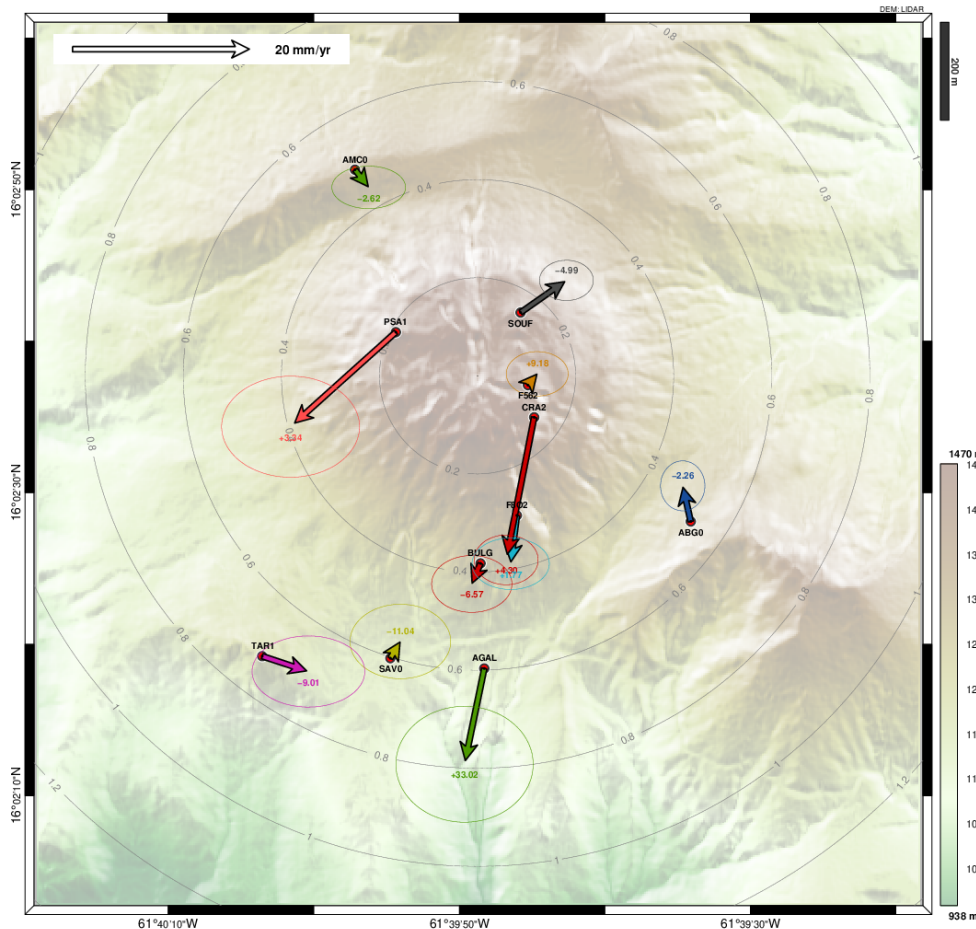
Figure 4. Déformation du dôme de la Soufrière enregistrée par le réseau GNSS permanent entre le 1er mai 2025 et le 1er mai 2026. La taille des flèches indique le taux de déformation horizontale en mm par an (échelle en haut à gauche). Le chiffre au bout de chaque flèche indique la valeur de la déformation verticale, positif pour une élévation, négatif pour un affaissement. Les ellipses représentent l'incertitude sur la position horizontale de l'extrémité du vecteur horizontal de déformation.
