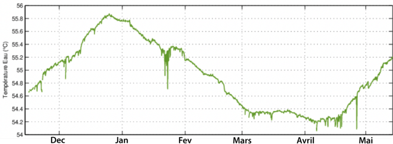
Figure 8 : Température de la source Galion, située en altitude sur le flanc sud de la Soufrière.
