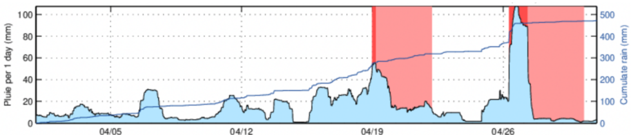
Figure 9. Précipitations instantanées et cumulées enregistrées au sommet de la Soufrière (station Piton Sanner) au cours du mois d'avril 2026 par l'OVSG-IPGP.
