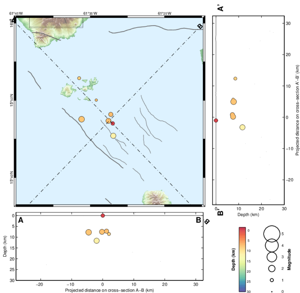
Figure 11. Épicentres et hypocentres des séismes tectoniques localisables, enregistrés au mois d'avril 2026 par l'OVSG-IPGP dans la zone des Saintes.
