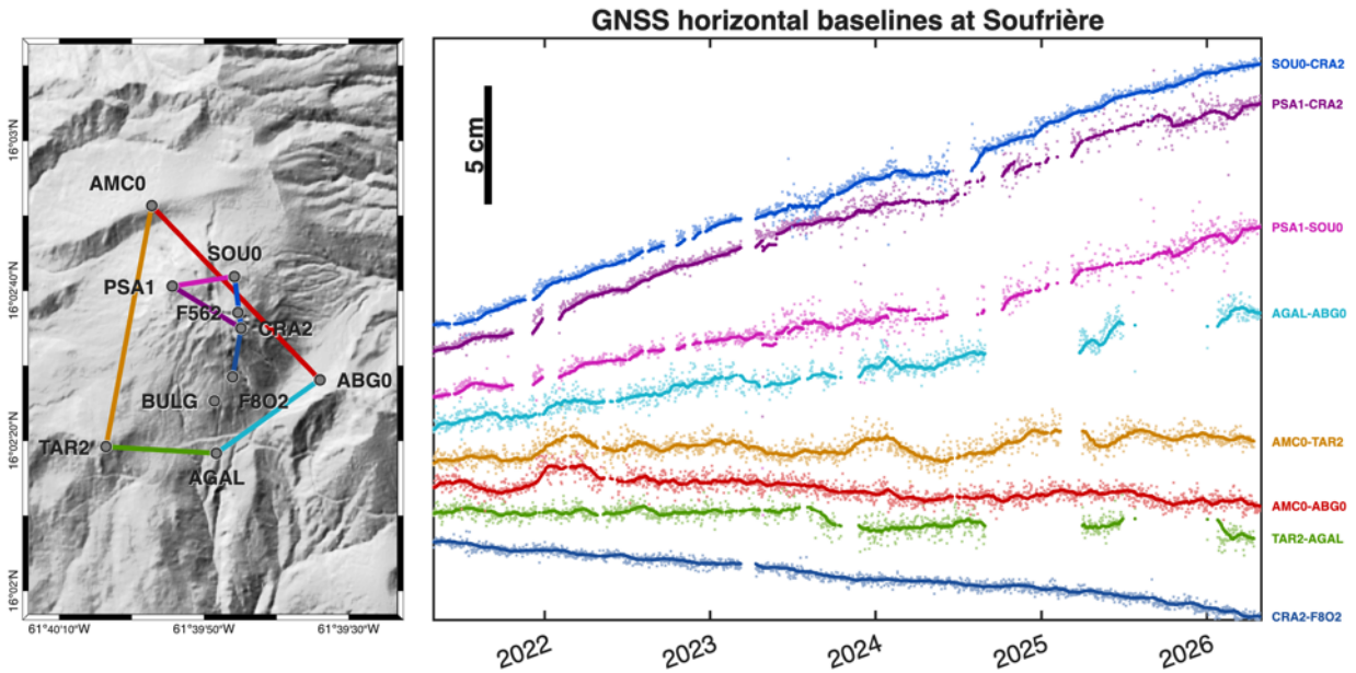
Figure 5. Évolution sur 5 ans (1er avril 2021 - 1er mai 2026) des distances séparant les stations GNSS permanentes localisées sur le volcan de la Soufrière.
