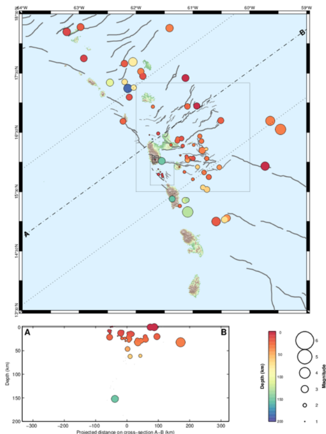
Figure 10. Epicentres (haut) et hypocentres (bas) des séismes tectoniques localisables enregistrés au mois d'avril 2026 par l'OVSG-IPGP.
