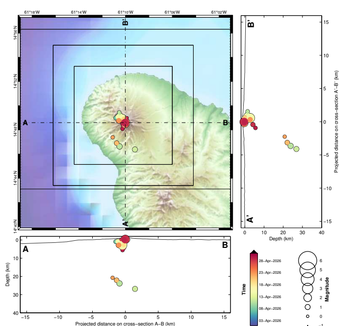
Figure 1 – Carte de localisation manuelle de la sismicité d'origine volcanique du mois d'avril 2026, et coupes est-ouest et nord-sud indiquant la localisation en profondeur des hypocentres (source WebObs/OVSM).
