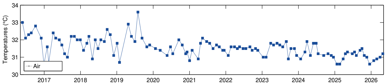
Figure 10 – Évolution de la température du forage Puits Chaud (points bleus foncés) de mai 2016 à avril 2026 inclus (mesures manuelles mensuelles, source WebObs/OVSM).
