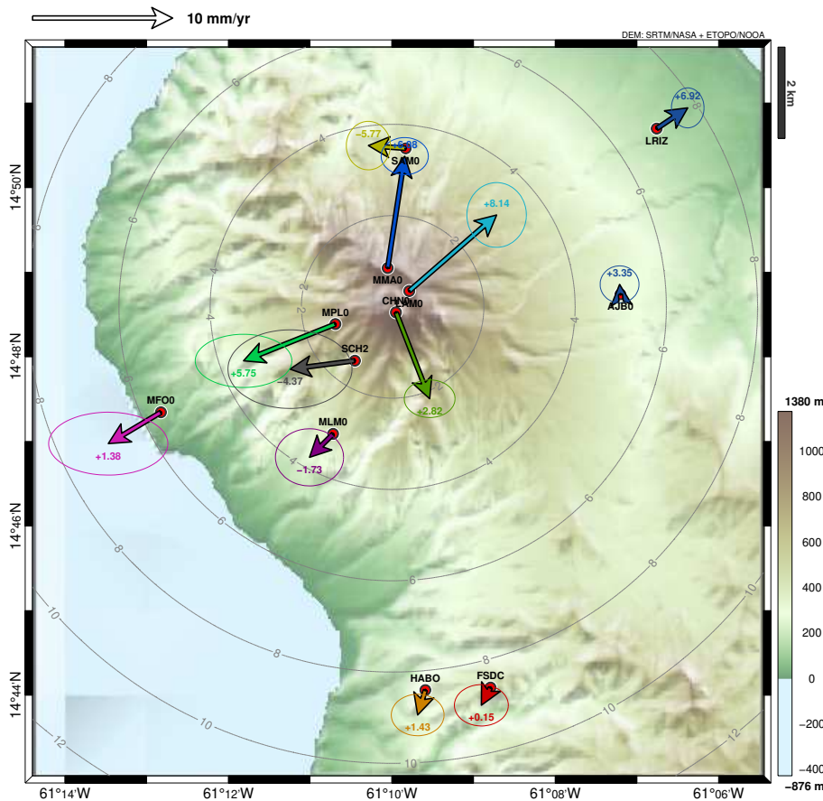
Figure 8 – Vecteurs des vitesses moyennes de déformations horizontales mesurées entre le 1 er mai 2024 et le 30 avril 2026 (deux ans) sur la Montagne Pelée (échelle donnée par la flèche en haut à gauche en mm par an). Chaque vecteur est associé à une ellipse d'erreur ainsi qu'à une indication de la vitesse verticale (non significative). Ces vitesses sont calculées de façon relative par rapport à un référentiel local et les ellipses d'erreur sont évaluées par rapport à l'écart-type des données relatifs à une tendance linéaire. Les cercles concentriques gris indiquent les distances en km depuis le sommet (calculs préliminaires). Source WebObs / OVSM).
