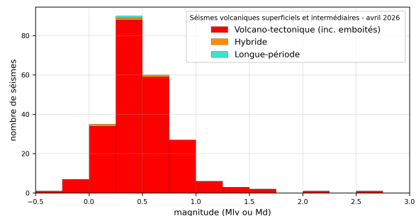
Figure 7 – Répartition en magnitude (magnitude locale M_{lv} ou magnitude de durée M_d ) des séismes superficiels de type volcano-tectonique, hybride et longue-période localisés au niveau de la Montagne Pelée en avril 2026 par gamme de 0,25 point de magnitude.
