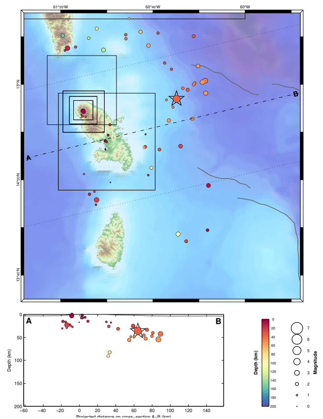
Figure 14 – Partie supérieure : carte des hypocentres des séismes enregistrés et localisés par l'OVSM-IPGP au cours du mois d'avril 2026 autour de la Martinique. La présence d'une étoile indique un séisme ressenti. Partie inférieure : représentation des séismes en profondeur le long du profil A-B et situés dans la zone comprises entre les deux lignes en pointillé (source WebObs/OVSM).
