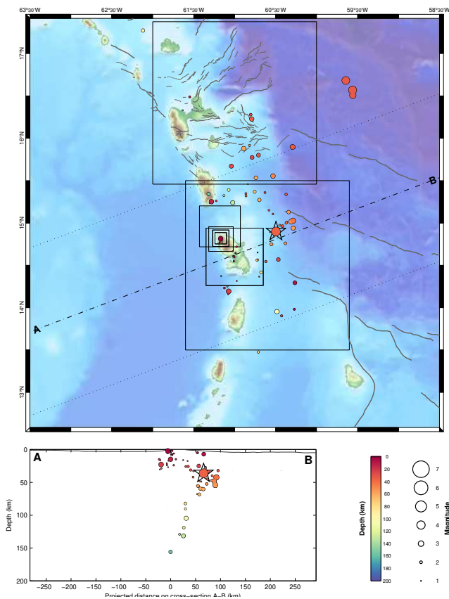
Figure 13 – Partie supérieure : carte des hypocentres des séismes enregistrés et localisés par l'OVSM-IPGP au cours du mois d'avril 2026 sur l'arc antillais. La présence d'une étoile indique un séisme ressenti. Partie inférieure : représentation des séismes en profondeur le long du profil A-B et situés dans la zone comprises entre les deux lignes en pointillé (source WebObs/OVSM).
