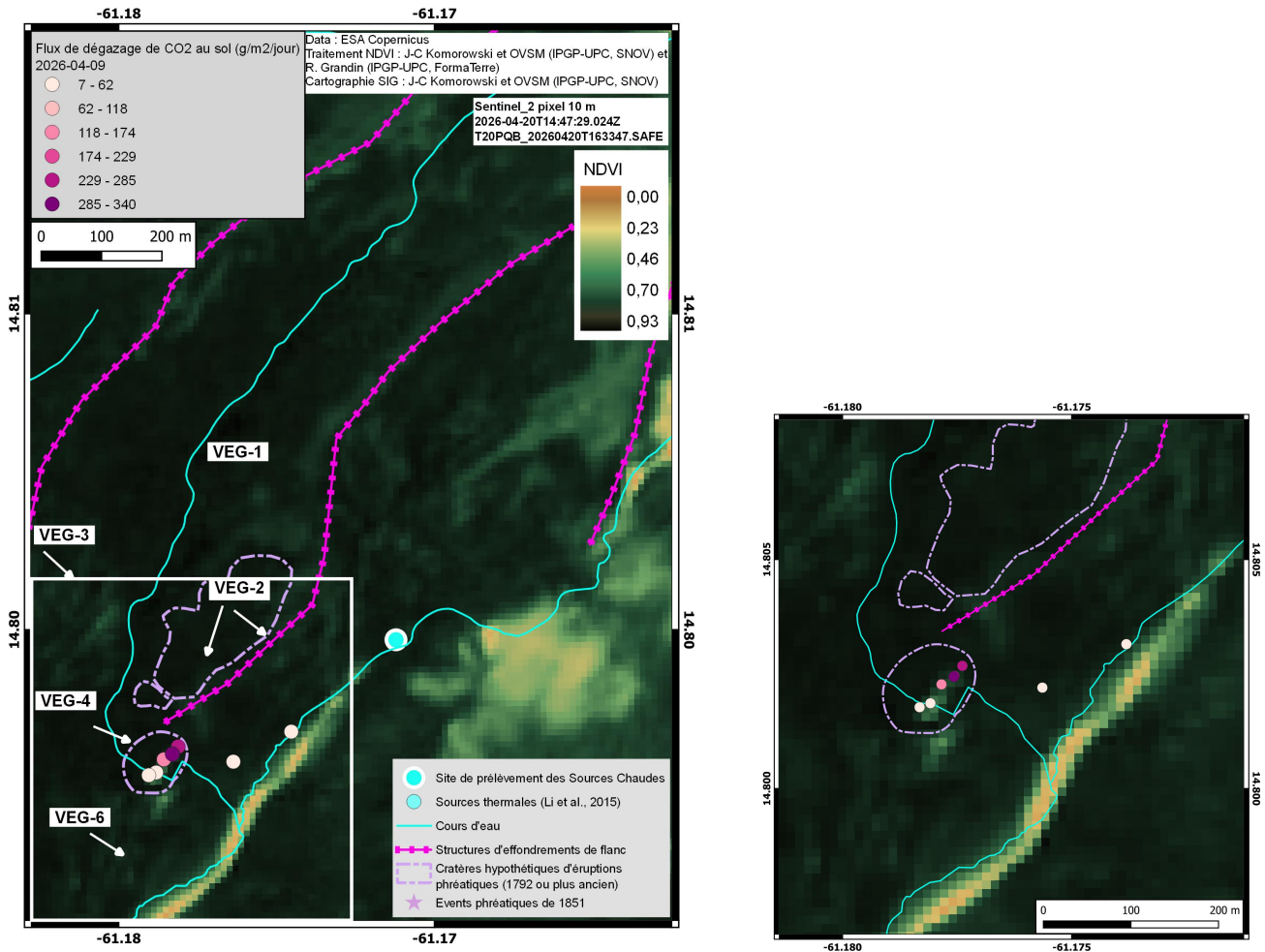
Figure 12 – Suivi du dépérissement de la végétation sur le flanc sud-ouest de la Montagne Pelée par la cartographie de l'indice NDVI à partir d'imagerie satellitale. (Gauche) Cette image du 20 avril 2026 (Sentinel-2) a été traitée pour montrer l'indice NDVI qui varie entre 0 (absence de végétation) et 1 (végétation saine). Les mesures du flux de dégazage diffus de CO 2 (en g/m 2 /jour) au sol réalisées avec la chambre d'accumulation West Systems le 9 avril 2026 sont indiquées par des cercles dans la gamme de couleur blanc-rose-magenta. Les zones dont le flux est > 25 g/m 2 /jour indiquent des flux de CO 2 qui comportent nécessairement une composante non-biogénique qui est d'origine volcanique et donc magmatique. (Droite) Agrandissement des zones VEG-3 à VEG-6 encadrées en blanc sur la carte principale. Traitement imagerie NDVI : J Corbeau et J-C Komorowski, OVSM-IPGP, UPC, SNOV (INSU-CNRS) et R. Grandin, IPGP-UPC, FormaTerre (INSU-CNRS). Cartographie SIG : J. Corbeau et J-C Komorowski, OVSM-IPGP, UPC, SNOV (INSU-CNRS). Données CO 2 : T. Abauzit, F. Jadelus, D. Melezan, OVSM-IPGP.
