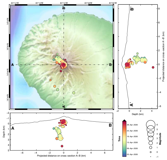
Figure 2 – Sismicité d'origine volcanique du mois d'avril 2026 ayant pu être localisée au niveau de la partie superficielle de la Montagne Pelée, et coupes est-ouest et nord-sud indiquant la localisation en profondeur des hypocentres (source WebObs/OVSM).
