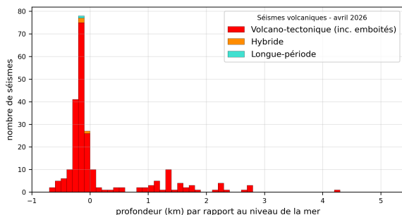
Figure 6 – Répartition en profondeur des séismes superficiels et intermédiaires de type volcano-tectonique, hybride et longue-période localisés au niveau de la Montagne Pelée en avril 2026 par gamme de 0,2 km.
