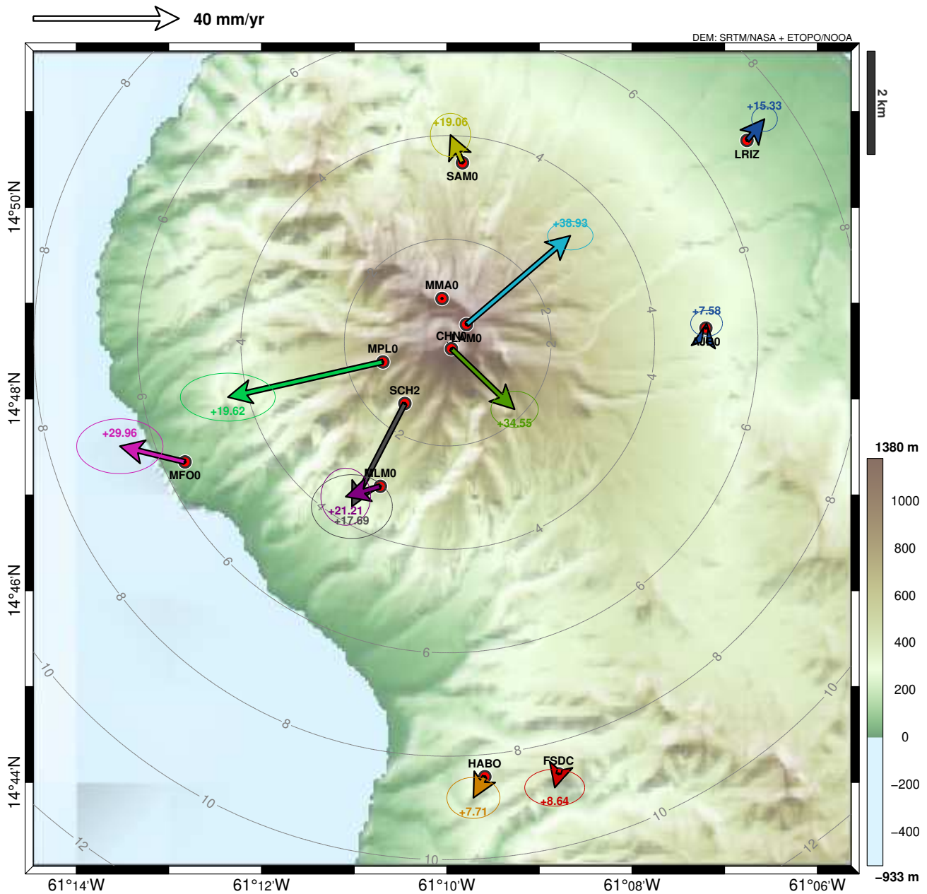
Figure 6 – Vecteurs des vitesses moyennes de déformations horizontales mesurées entre le 1 er décembre 2025 et le 31 mai 2026 (six mois) sur la Montagne Pelée (échelle donnée par la flèche en haut à gauche en mm par an). Chaque vecteur est associé à une ellipse d'erreur ainsi qu'à une indication de la vitesse verticale (non significative). Ces vitesses sont calculées de façon relative par rapport à un référentiel local et les ellipses d'erreur sont évaluées par rapport à l'écart-type des données relatifs à une tendance linéaire. Les cercles concentriques gris indiquent les distances en km depuis le sommet (calculs préliminaires. Source WebObs / OVSM).
