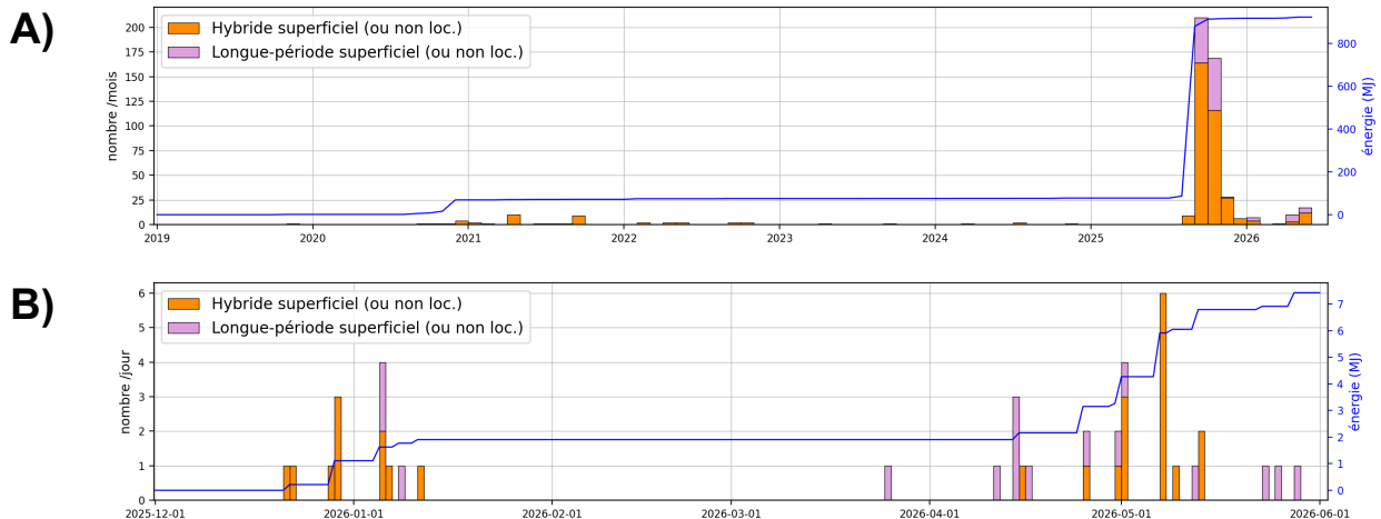
Figure 5 – Evolution du nombre de séismes superficiels de type hybride (orange) et longue-période (violet clair) détectés par l’OVSM-IPGP dans l’environnement de la Montagne Pelée : A) Nombre par mois du 1 er janvier 2019 au 31 mai 2026. B) Nombre par jour durant les 6 derniers mois (du 1 er décembre 2025 au 31 mai 2026). Les courbes bleues indiquent l’évolution de l’énergie cumulée déduite de la magnitude M_{lv} des événements localisés en sommant l’énergie des séismes superficiels de type hybride et longue-période.
