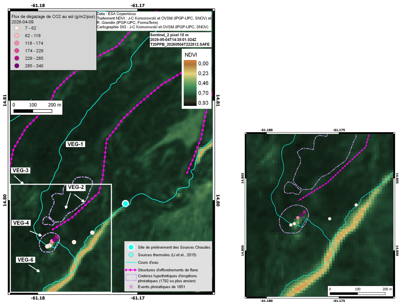
Figure 9 – Suivi du dépérissement de la végétation sur le flanc sud-ouest de la Montagne Pelée par la cartographie de l'indice NDVI à partir d'imagerie satellitale. (Gauche) Cette image du 04 mai 2026 (Sentinel-2) a été traitée pour montrer l'indice NDVI qui varie entre 0 (absence de végétation) et 1 (végétation saine). Les mesures du flux de dégazage diffus de CO 2 (en g/m 2 /jour) au sol réalisées avec la chambre d'accumulation West Systems le 9 avril 2026 sont indiquées par des cercles dans la gamme de couleur blanc-rose-magenta. Les zones dont le flux est > 25 g/m 2 /jour indiquent des flux de CO 2 qui comportent nécessairement une composante non-biogénique qui est d'origine volcanique et donc magmatique. (Droite) Agrandissement des zones VEG-3 à VEG-6 encadrées en blanc sur la carte principale. Traitement imagerie NDVI : J Corbeau et J-C Komorowski, OVSM-IPGP, UPC, SNOV (INSU-CNRS) et R. Grandin, IPGP-UPC, FormaTerre (INSU-CNRS). Cartographie SIG : J. Corbeau et J-C Komorowski, OVSM-IPGP, UPC, SNOV (INSU-CNRS). Données CO 2 : T. Abauzit, F. Jadelus, D. Melezan, OVSM-IPGP.
