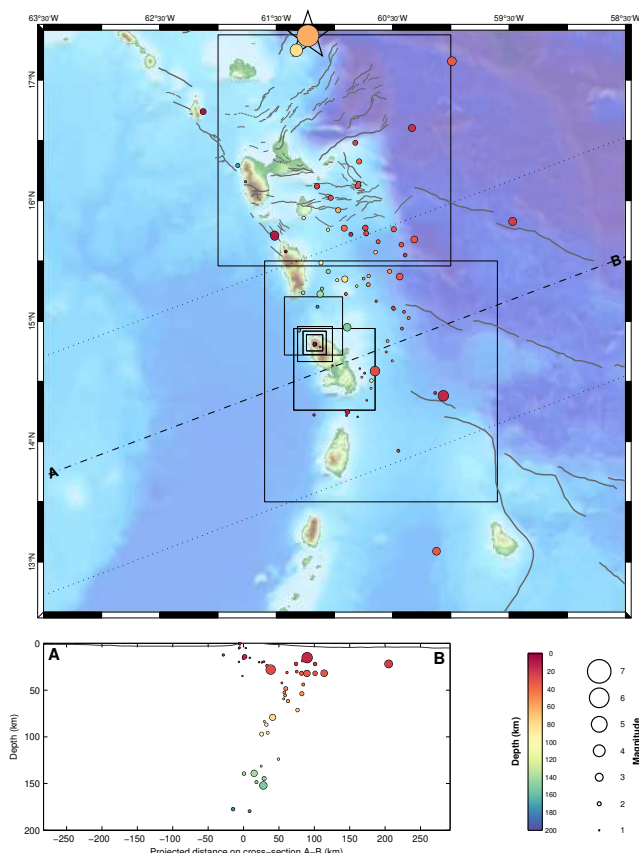
Figure 10 – Partie supérieure : carte des hypocentres des séismes enregistrés et localisés par l'OVSM-IPGP au cours du mois de mai 2026 sur l'arc antillais. La présence d'une étoile indique un séisme ressenti. Partie inférieure : représentation des séismes en profondeur le long du profil A-B et situés dans la zone comprises entre les deux lignes en pointillé (source WebObs/OVSM).
