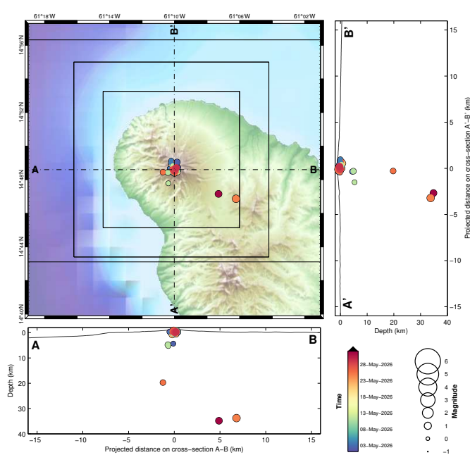
Figure 1 – Carte de localisation manuelle de la sismicité d'origine volcanique du mois de mai 2026, et coupes est-ouest et nord-sud indiquant la localisation en profondeur des hypocentres (source WebObs/OVSM).
