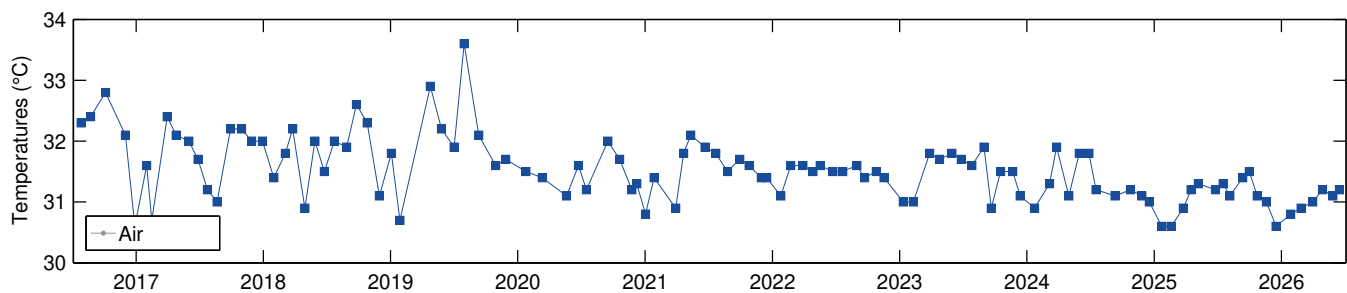
Figure 8 – Évolution de la température du forage Puits Chaud (points bleus foncés) de juin 2016 à mai 2026 inclus (mesures manuelles mensuelles, source WebObs/OVSM).
