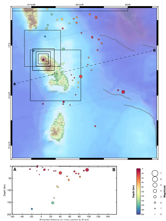
Figure 11 – Partie supérieure : carte des hypocentres des séismes enregistrés et localisés par l'OVSM-IPGP au cours du mois de mai 2026 autour de la Martinique. La présence d'une étoile indique un séisme ressenti. Partie inférieure : représentation des séismes en profondeur le long du profil A-B et situés dans la zone comprises entre les deux lignes en pointillé (source WebObs/OVSM).
