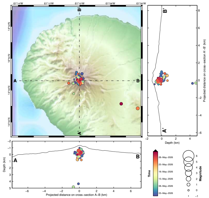
Figure 2 – Sismicité d'origine volcanique du mois de mai 2026 ayant pu être localisée au niveau de la partie superficielle de la Montagne Pelée, et coupes est-ouest et nord-sud indiquant la localisation en profondeur des hypocentres (source WebObs/OVSM).
