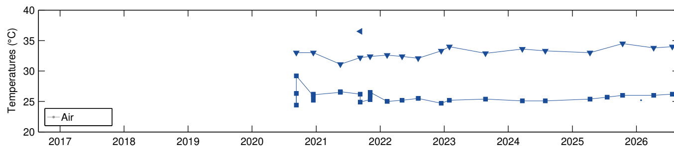
Figure 9 – Évolution de la température des sources chaudes de la Rivière Chaude (triangles bleus) et des eaux de la rivière (carrés bleus) de 2016 à juillet 2026 sur la base des mesures manuelles (source WebObs/OVSM).
