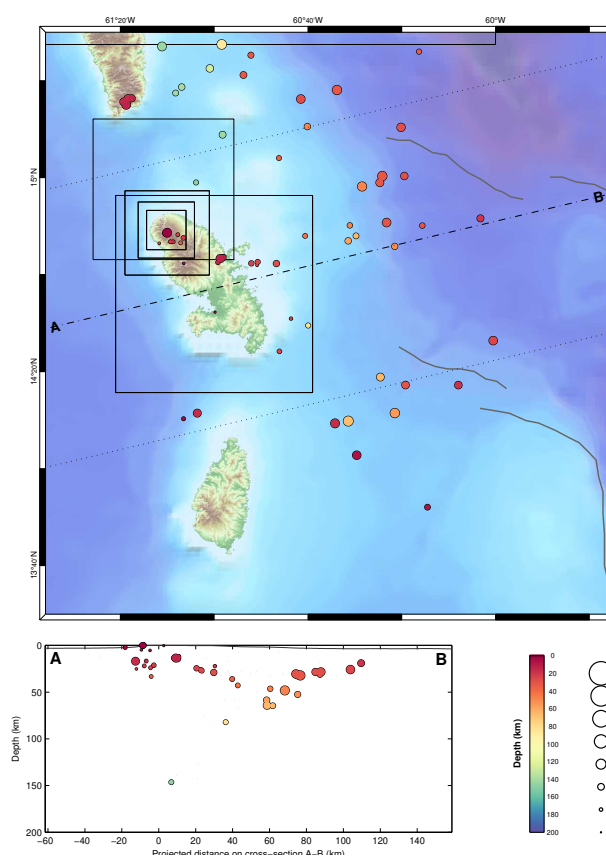
Figure 12 – Partie supérieure : carte des hypocentres des séismes enregistrés et localisés par l'OVSM-IPGP au cours du mois de juillet 2026 autour de la Martinique. La présence d'une étoile indique un séisme ressenti. Partie inférieure : représentation des séismes en profondeur le long du profil A-B et situés dans la zone comprises entre les deux lignes en pointillé (source WebObs/OVSM).
