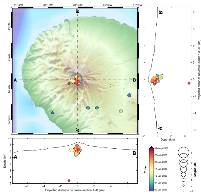
Figure 2 – Sismicité d'origine volcanique du mois de juillet 2026 ayant pu être localisée au niveau de la partie superficielle de la Montagne Pelée, et coupes est-ouest et nord-sud indiquant la localisation en profondeur des hypocentres (source WebObs/OVSM).
