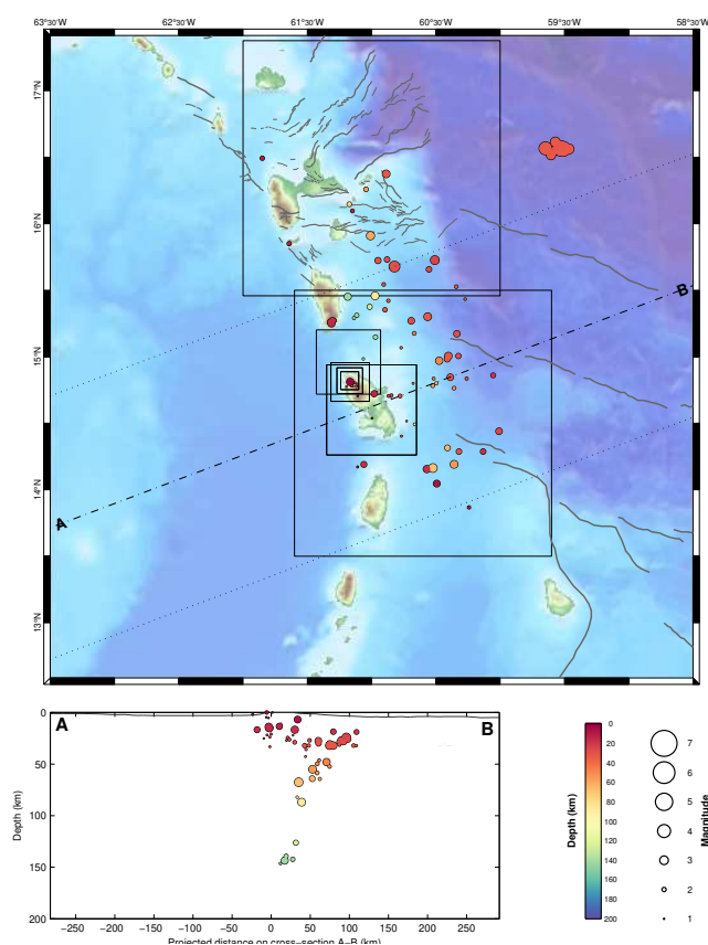
Figure 11 – Partie supérieure : carte des hypocentres des séismes enregistrés et localisés par l'OVSM-IPGP au cours du mois de juillet 2026 sur l'arc antillais. La présence d'une étoile indique un séisme ressenti. Partie inférieure : représentation des séismes en profondeur le long du profil A-B et situés dans la zone comprises entre les deux lignes en pointillé (source WebObs/OVSM).
