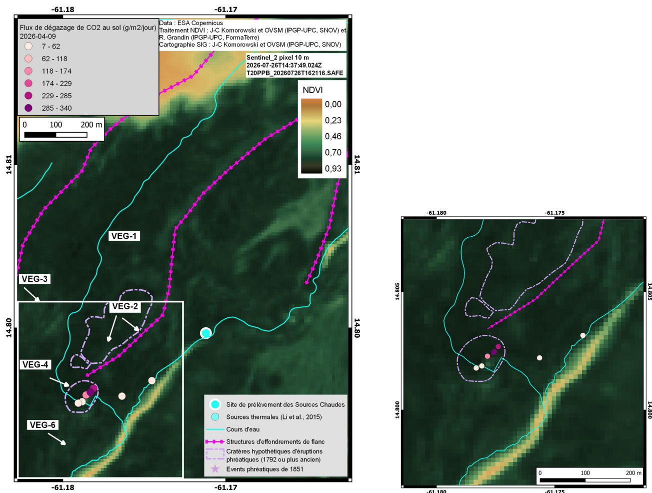
Figure 10 – Suivi du dépérissement de la végétation sur le flanc sud-ouest de la Montagne Pelée par la cartographie de l'indice NDVI à partir d'imagerie satellitale. (Gauche) Cette image du 26 juillet 2026 (Sentinel-2) a été traitée pour montrer l'indice NDVI qui varie entre 0 (absence de végétation) et 1 (végétation saine). Les mesures du flux de dégazage diffus de \text{CO}_2 (en \text{g/m}^2/\text{jour} ) au sol réalisées avec la chambre d'accumulation West Systems le 9 avril 2026 sont indiquées par des cercles dans la gamme de couleur blanc-rose-magenta. Les zones dont le flux est > 25 \text{ g/m}^2/\text{jour} indiquent des flux de \text{CO}_2 qui comportent nécessairement une composante non-biogénique qui est d'origine volcanique et donc magmatique. (Droite) Agrandissement des zones VEG-3 à VEG-6 encadrées en blanc sur la carte principale. Traitement imagerie NDVI : J Corbeau et J-C Komorowski, OVSM-IPGP, UPC, SNOV (INSU-CNRS) et R. Grandin, IPGP-UPC, FormaTerre (INSU-CNRS). Cartographie SIG : J. Corbeau et J-C Komorowski, OVSM-IPGP, UPC, SNOV (INSU-CNRS). Données \text{CO}_2 : F. Jadelus, A.-S. Leygnac, OVSM-IPGP.
