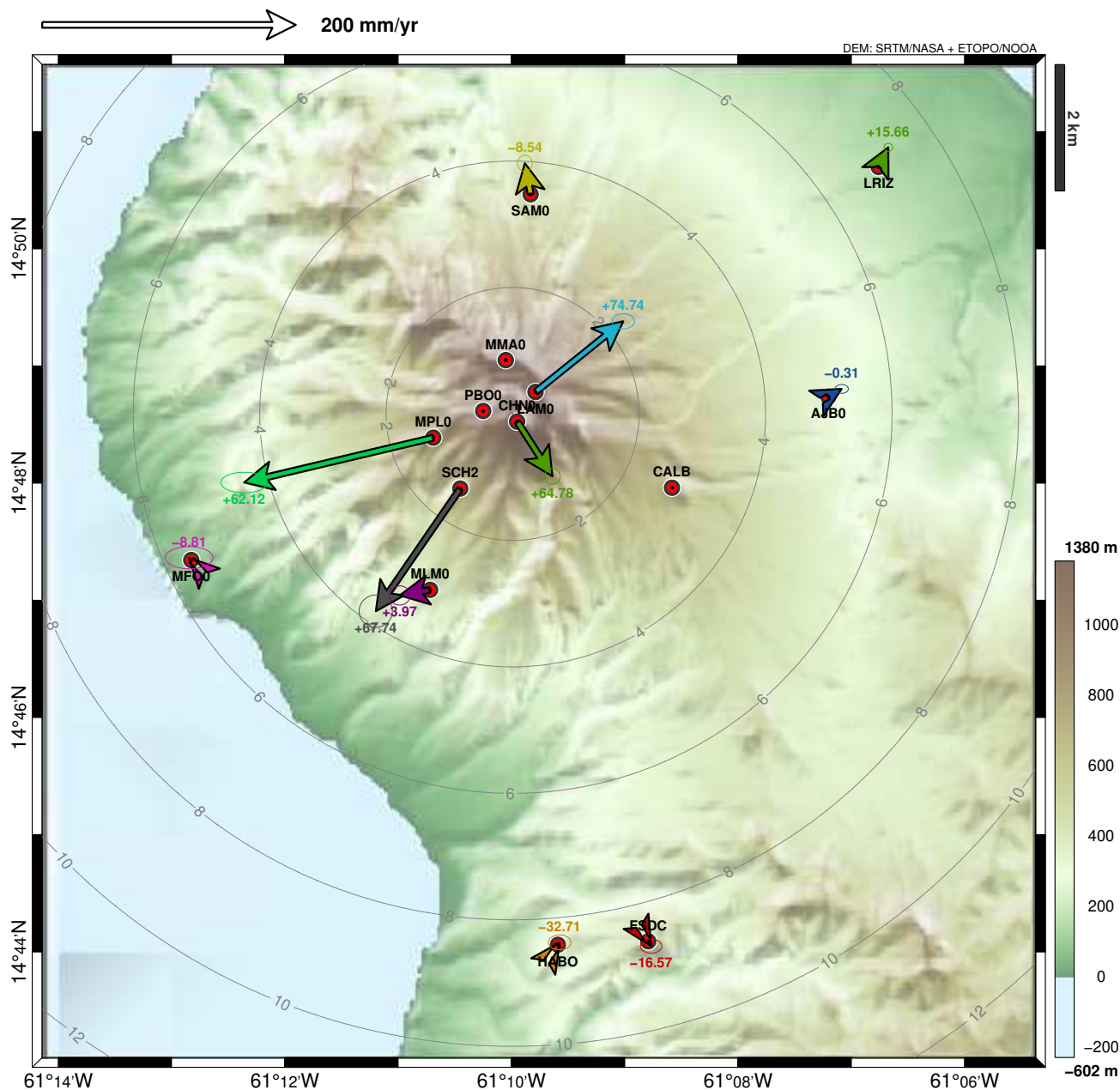
Figure 6 – Vecteurs des vitesses moyennes de déformations horizontales mesurées entre le 1 er février 2026 et le 31 juillet 2026 (six mois) sur la Montagne Pelée (échelle donnée par la flèche en haut à gauche en mm par an). Chaque vecteur est associé à une ellipse d'erreur ainsi qu'à une indication de la vitesse verticale (non significative). Ces vitesses sont calculées de façon relative par rapport à un référentiel local et les ellipses d'erreur sont évaluées par rapport à l'écart-type des données relatifs à une tendance linéaire. Les cercles concentriques gris indiquent les distances en km depuis le sommet (calculs préliminaires. Source WebObs / OVSM).
