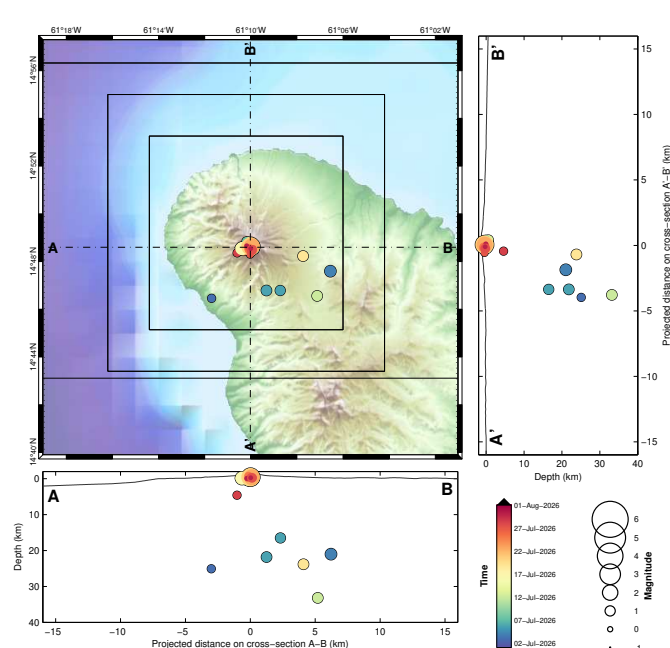
Figure 1 – Carte de localisation manuelle de la sismicité d'origine volcanique du mois de juillet 2026, et coupes est-ouest et nord-sud indiquant la localisation en profondeur des hypocentres (source WebObs/OVSM).
