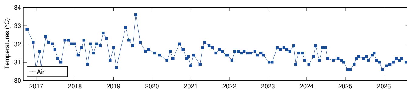
Figure 8 – Évolution de la température du forage Puits Chaud (points bleus foncés) de août 2016 à juillet 2026 inclus (mesures manuelles mensuelles, source WebObs/OVSM).
